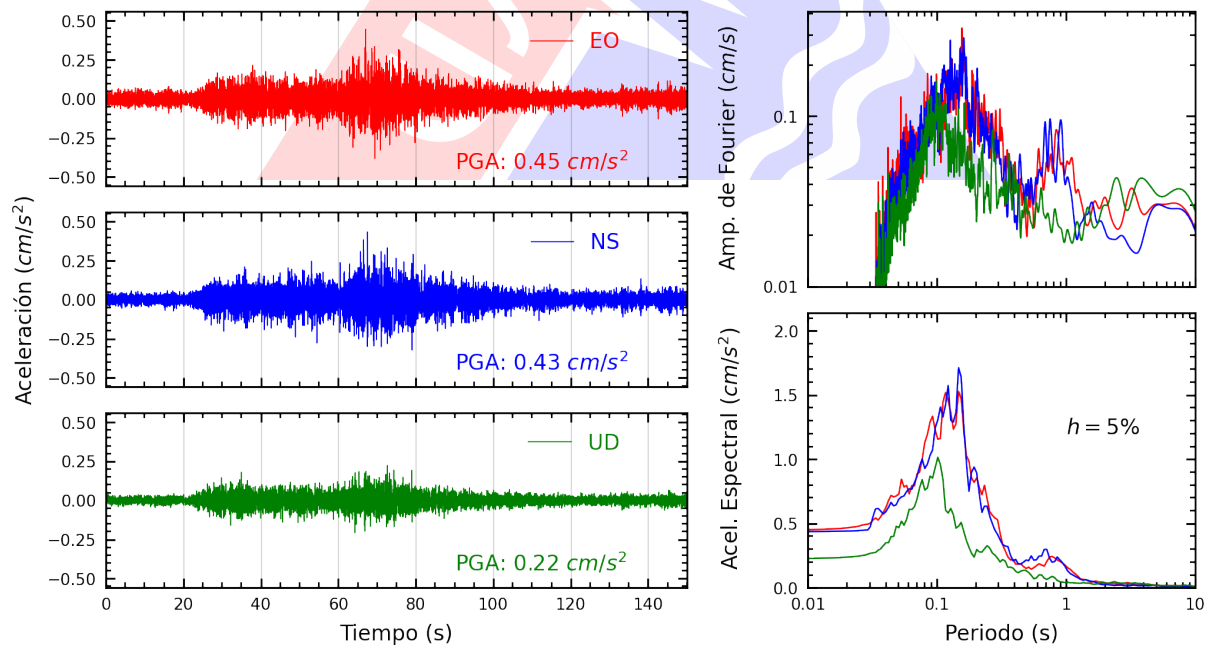
Figura A.4: Registros tiempo-historia, espectros de Fourier y de respuesta en las direcciones EO, NS y vertical de la estación USILM. Sismo de Puerto Bermudez, Oxapampa - Pasco del 2024-05-24, 04:58:47 (Hora local)
