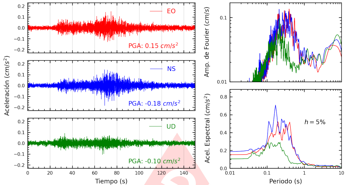
Figura A.13: Registros tiempo-historia, espectros de Fourier y de respuesta en las direcciones EO, NS y vertical de la estación VHAYA. Sismo de Puerto Bermudez, Oxapampa - Pasco del 2024-05-24, 04:58:47 (Hora local)
