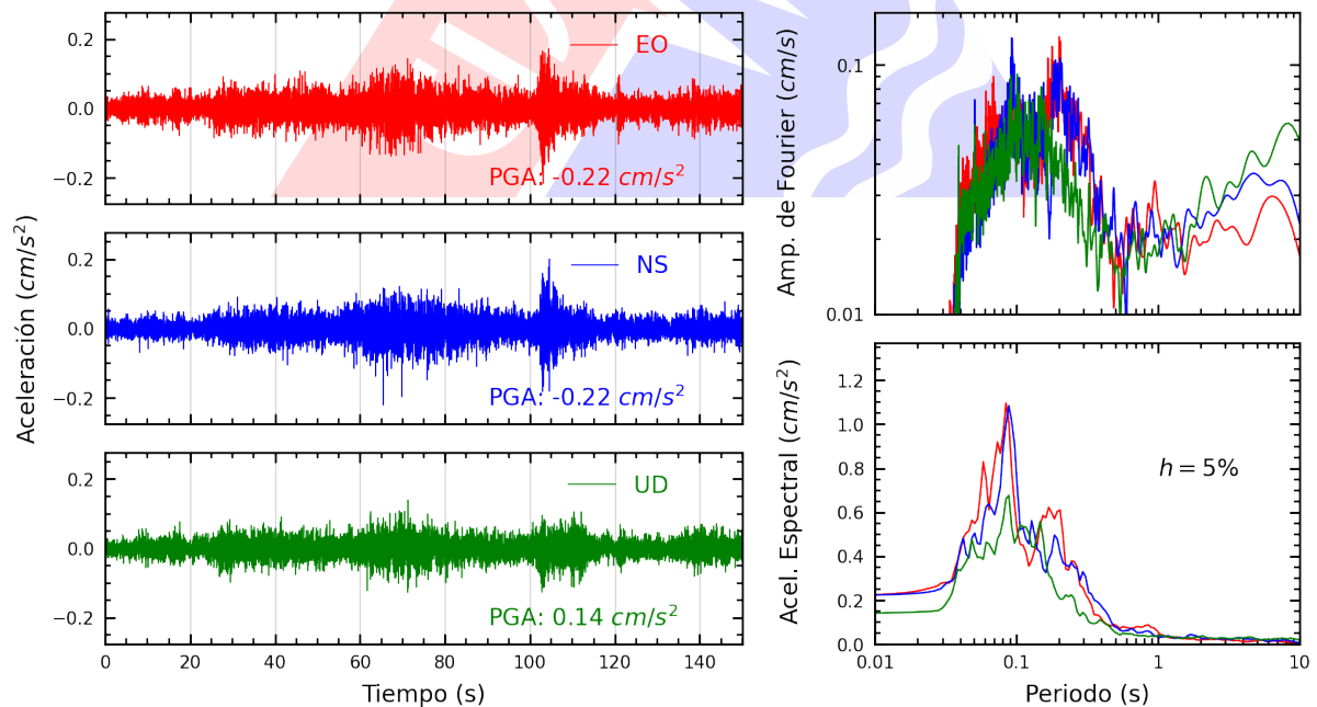
Figura A.10: Registros tiempo-historia, espectros de Fourier y de respuesta en las direcciones EO, NS y vertical de la estación INDEP. Sismo de Puerto Bermudez, Oxapampa - Pasco del 2024-05-24, 04:58:47 (Hora local)
