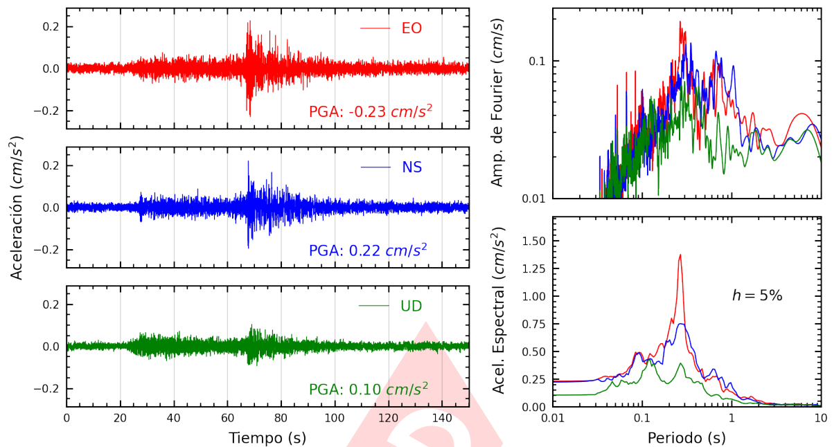
Figura A.9: Registros tiempo-historia, espectros de Fourier y de respuesta en las direcciones EO, NS y vertical de la estación USILP. Sismo de Puerto Bermudez, Oxapampa - Pasco del 2024-05-24, 04:58:47 (Hora local)
