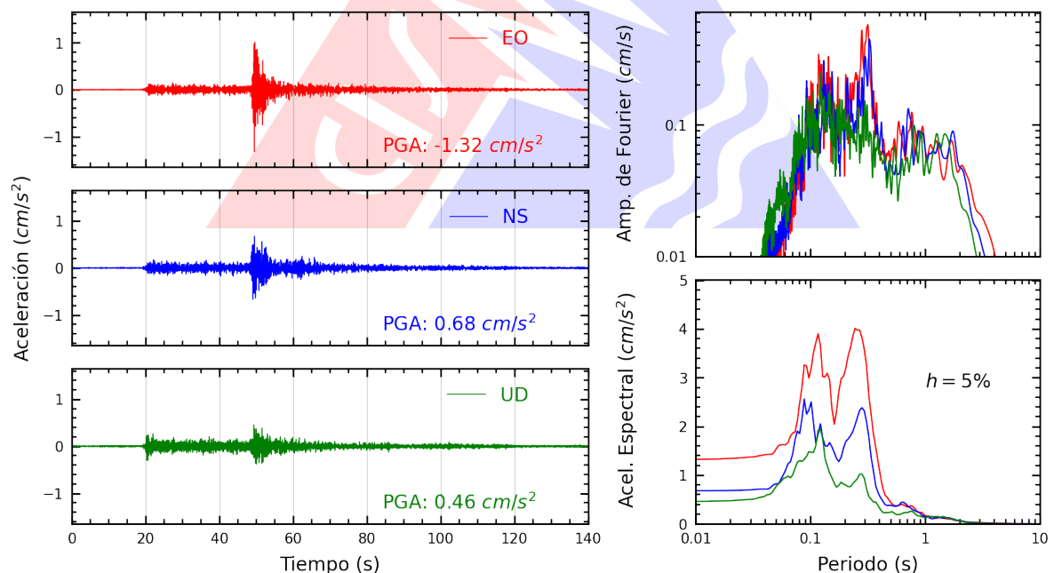
Figura A.2: Registros tiempo-historia, espectros de Fourier y de respuesta en las direcciones EO, NS y vertical de la estación SCHYO. Sismo de Puerto Bermudez, Oxapampa - Pasco del 2024-05-24, 04:58:47 (Hora local)
