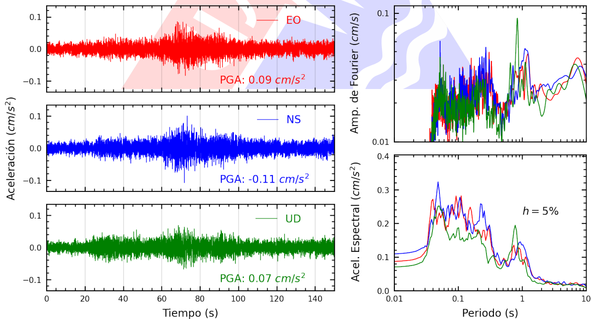
Figura A.20: Registros tiempo-historia, espectros de Fourier y de respuesta en las direcciones EO, NS y vertical de la estación CENEP. Sismo de Puerto Bermudez, Oxapampa - Pasco del 2024-05-24, 04:58:47 (Hora local)
