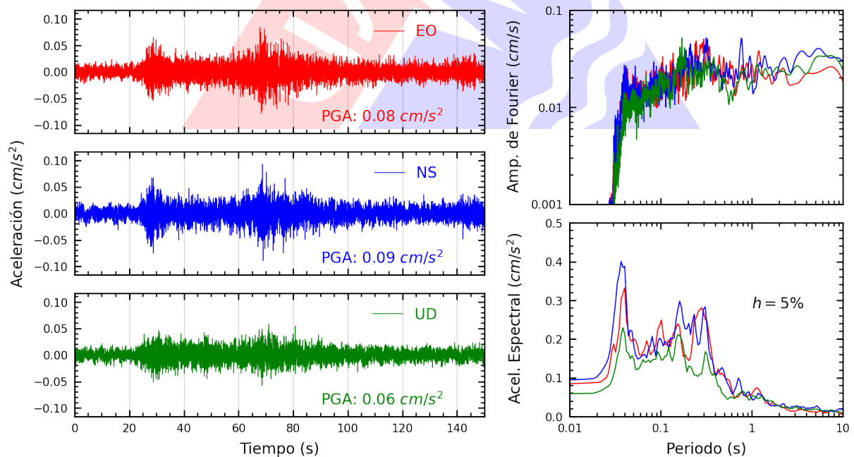
Figura A.24: Registros tiempo-historia, espectros de Fourier y de respuesta en las direcciones EO, NS y vertical de la estación CEPRE. Sismo de Puerto Bermudez, Oxapampa - Pasco del 2024-05-24, 04:58:47 (Hora local)
