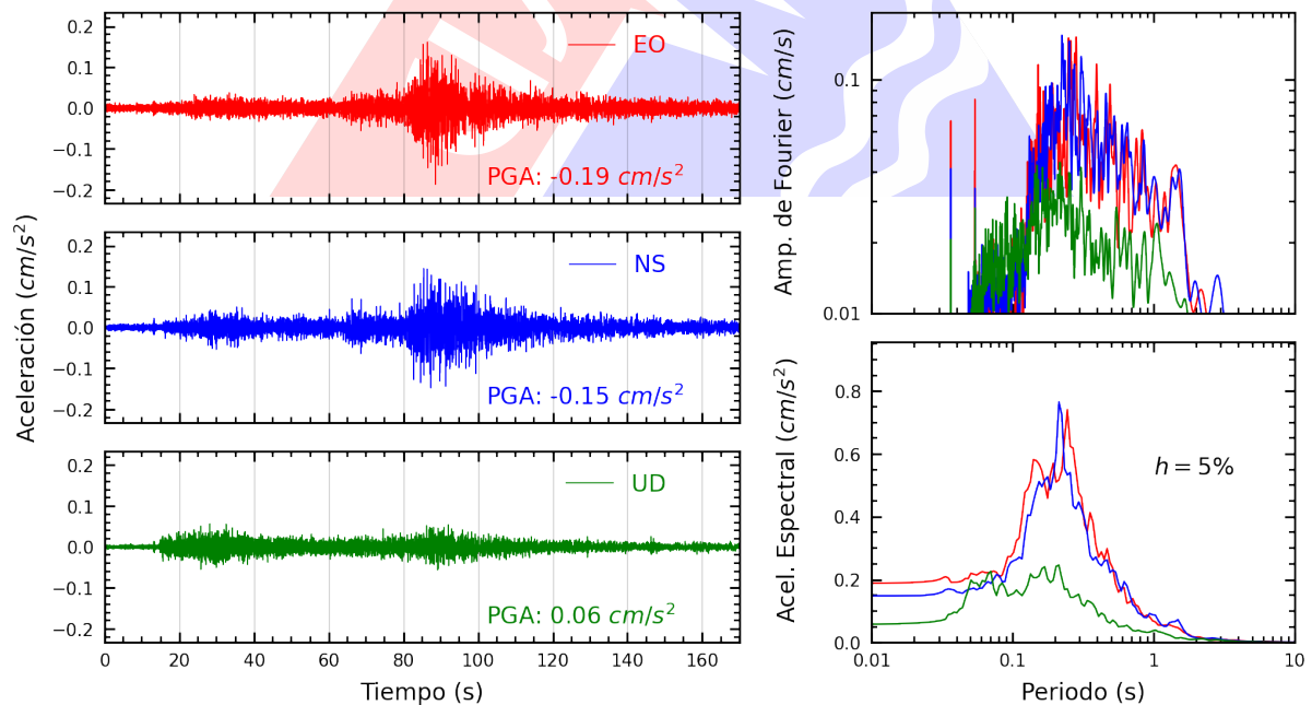
Figura A.12: Registros tiempo-historia, espectros de Fourier y de respuesta en las direcciones EO, NS y vertical de la estación UNAAA. Sismo de Puerto Bermudez, Oxapampa - Pasco del 2024-05-24, 04:58:47 (Hora local)
