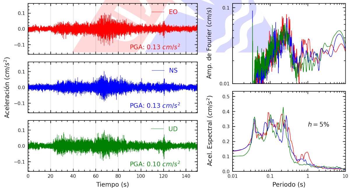
Figura A.18: Registros tiempo-historia, espectros de Fourier y de respuesta en las direcciones EO, NS y vertical de la estación USMP. Sismo de Puerto Bermudez, Oxapampa - Pasco del 2024-05-24, 04:58:47 (Hora local)
