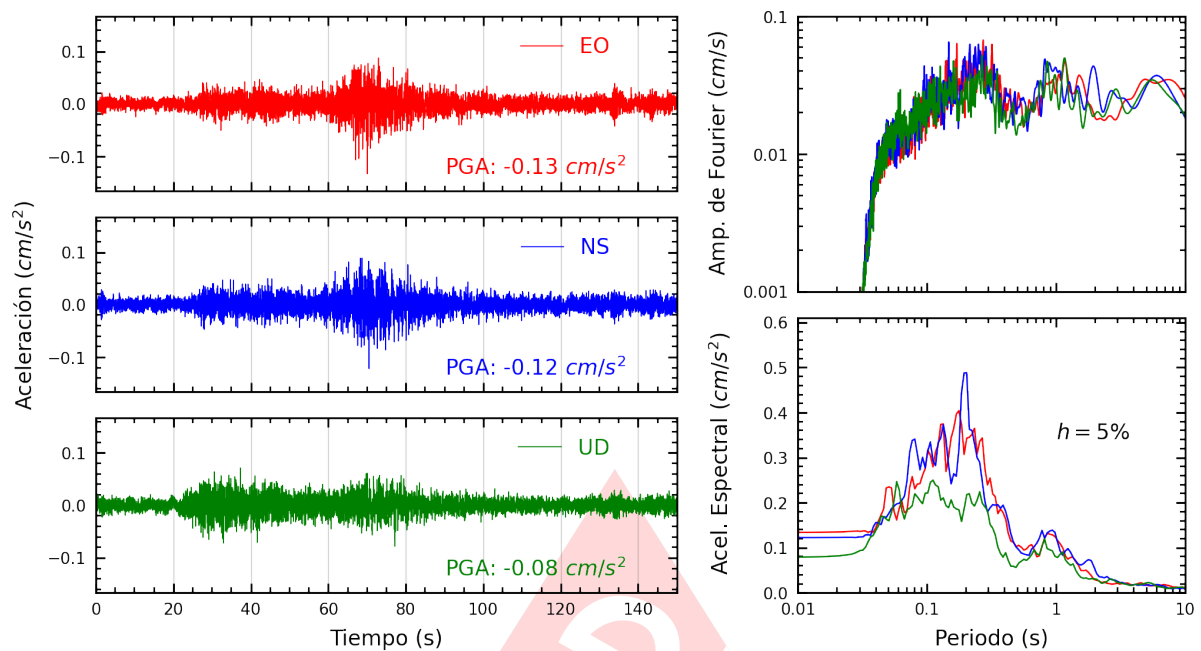
Figura A.17: Registros tiempo-historia, espectros de Fourier y de respuesta en las direcciones EO, NS y vertical de la estación SERVI. Sismo de Puerto Bermudez, Oxapampa - Pasco del 2024-05-24, 04:58:47 (Hora local)
