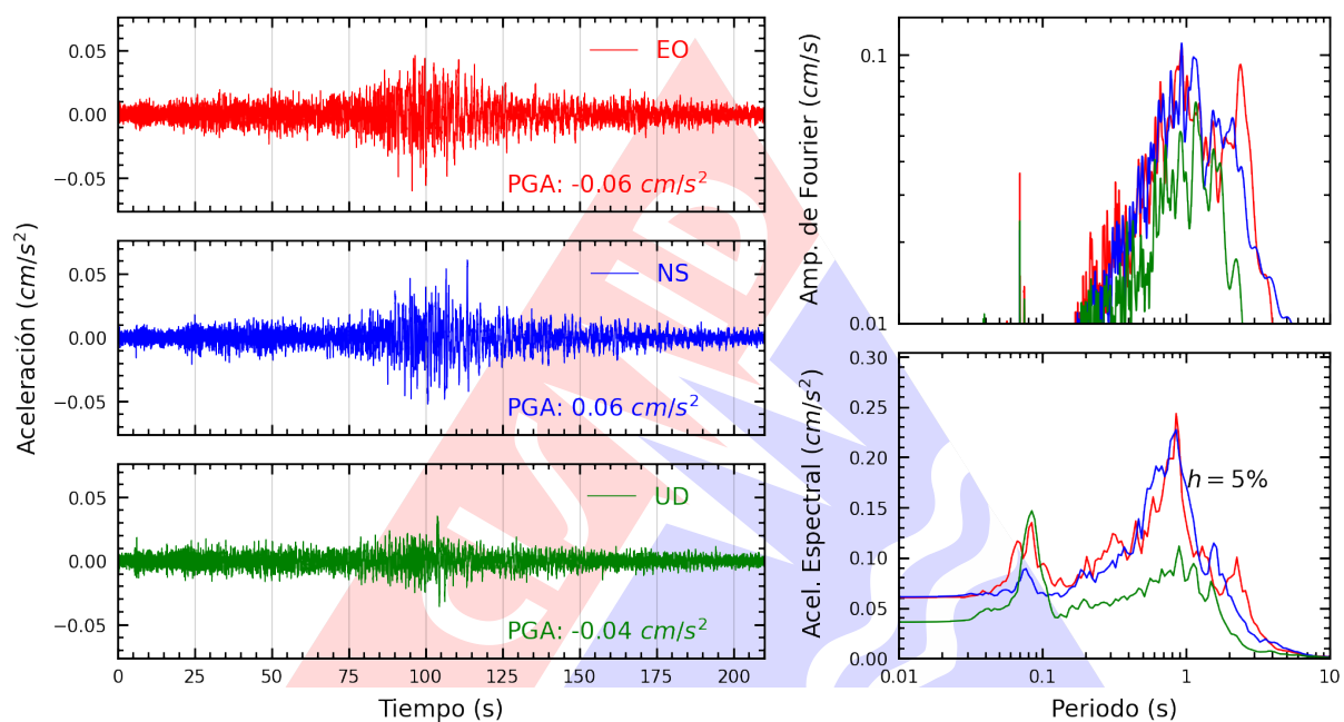
Figura A.25: Registros tiempo-historia, espectros de Fourier y de respuesta en las direcciones EO, NS y vertical de la estación UNC. Sismo de Puerto Bermudez, Oxapampa - Pasco del 2024-05-24, 04:58:47 (Hora local)
