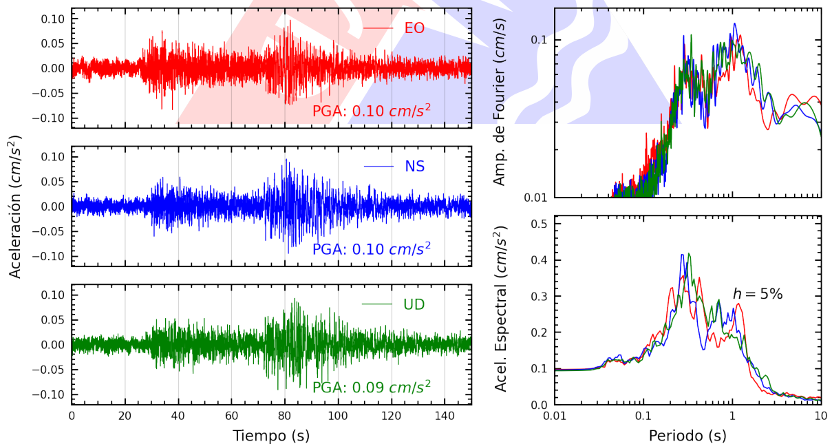
Figura A.22: Registros tiempo-historia, espectros de Fourier y de respuesta en las direcciones EO, NS y vertical de la estación UNSCH. Sismo de Puerto Bermudez, Oxapampa - Pasco del 2024-05-24, 04:58:47 (Hora local)
