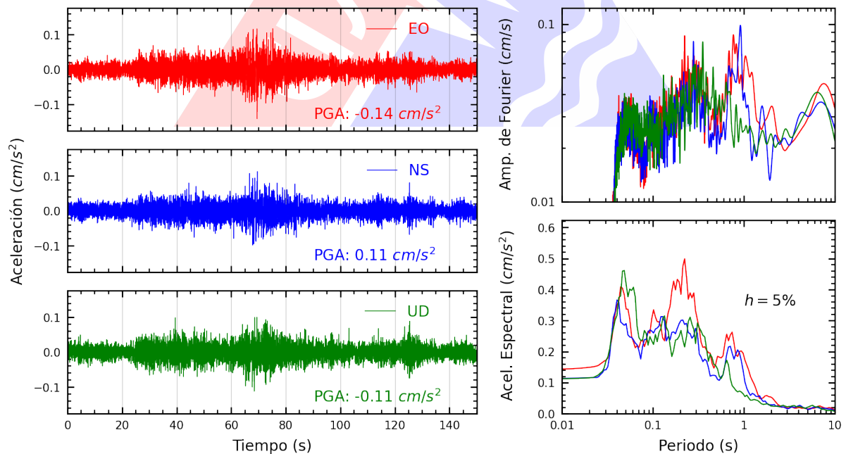
Figura A.16: Registros tiempo-historia, espectros de Fourier y de respuesta en las direcciones EO, NS y vertical de la estación IMCA. Sismo de Puerto Bermudez, Oxapampa - Pasco del 2024-05-24, 04:58:47 (Hora local)
