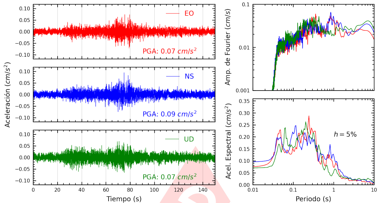
Figura A.23: Registros tiempo-historia, espectros de Fourier y de respuesta en las direcciones EO, NS y vertical de la estación UNFV. Sismo de Puerto Bermudez, Oxapampa - Pasco del 2024-05-24, 04:58:47 (Hora local)
