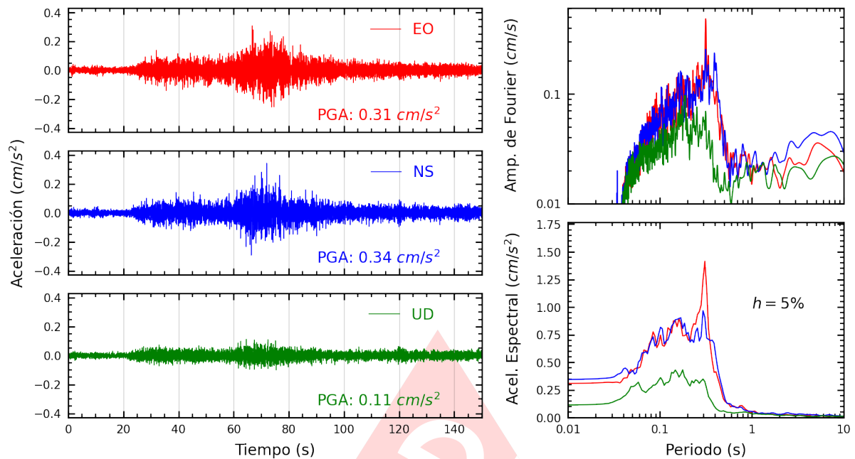
Figura A.7: Registros tiempo-historia, espectros de Fourier y de respuesta en las direcciones EO, NS y vertical de la estación DEFEN. Sismo de Puerto Bermudez, Oxapampa - Pasco del 2024-05-24, 04:58:47 (Hora local)
