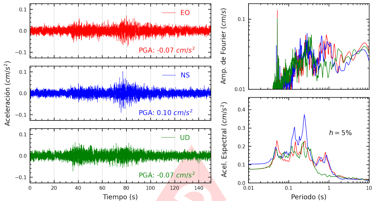
Figura A.21: Registros tiempo-historia, espectros de Fourier y de respuesta en las direcciones EO, NS y vertical de la estación UNMSM. Sismo de Puerto Bermudez, Oxapampa - Pasco del 2024-05-24, 04:58:47 (Hora local)
