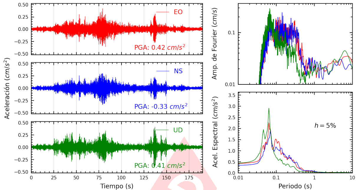
Figura A.5: Registros tiempo-historia, espectros de Fourier y de respuesta en las direcciones EO, NS y vertical de la estación ANCON. Sismo de Puerto Bermudez, Oxapampa - Pasco del 2024-05-24, 04:58:47 (Hora local)
