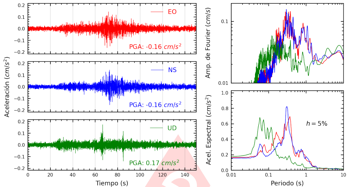
Figura A.15: Registros tiempo-historia, espectros de Fourier y de respuesta en las direcciones EO, NS y vertical de la estación ACAPU. Sismo de Puerto Bermudez, Oxapampa - Pasco del 2024-05-24, 04:58:47 (Hora local)
