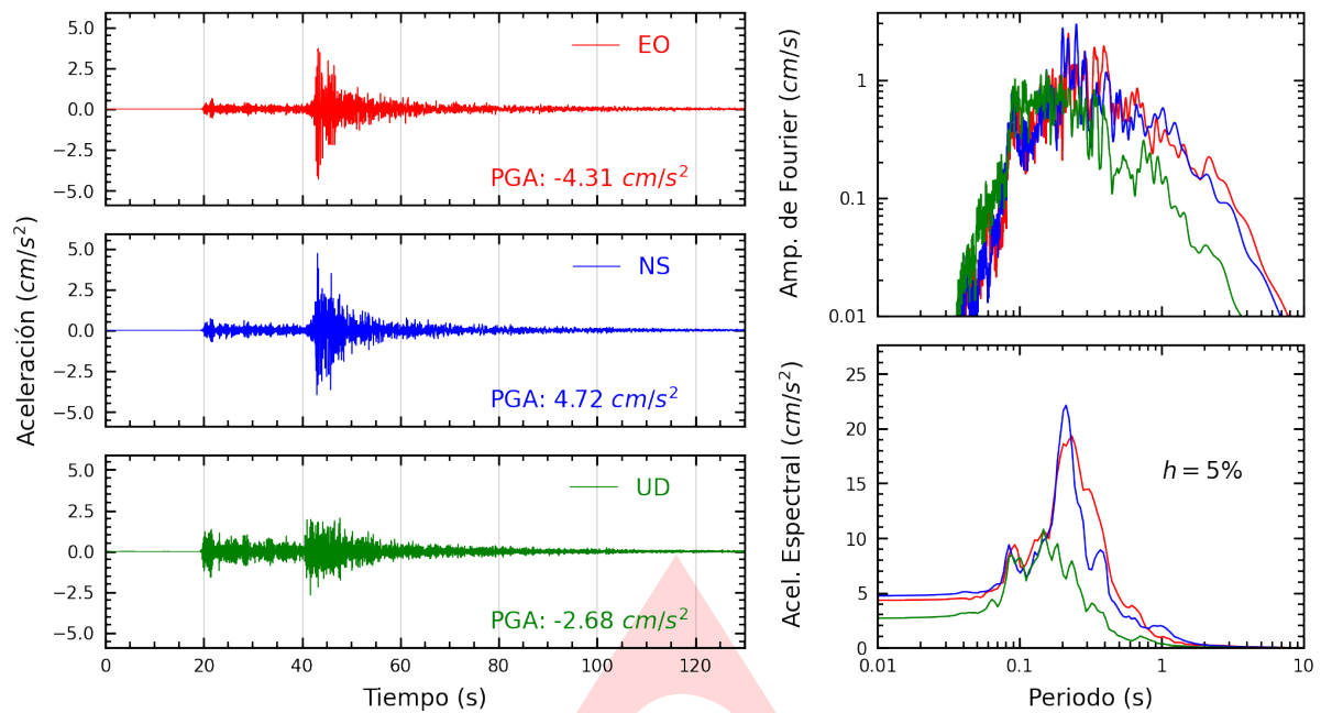
Figura A.1: Registros tiempo-historia, espectros de Fourier y de respuesta en las direcciones EO, NS y vertical de la estación UNIA. Sismo de Puerto Bermudez, Oxapampa - Pasco del 2024-05-24, 04:58:47 (Hora local)
