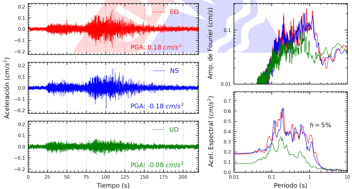
Figura A.14: Registros tiempo-historia, espectros de Fourier y de respuesta en las direcciones EO, NS y vertical de la estación UNTRM. Sismo de Puerto Bermudez, Oxapampa - Pasco del 2024-05-24, 04:58:47 (Hora local)
