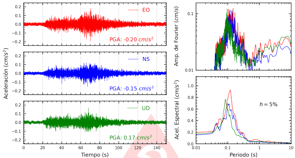
Figura A.11: Registros tiempo-historia, espectros de Fourier y de respuesta en las direcciones EO, NS y vertical de la estación AMORE. Sismo de Puerto Bermudez, Oxapampa - Pasco del 2024-05-24, 04:58:47 (Hora local)
