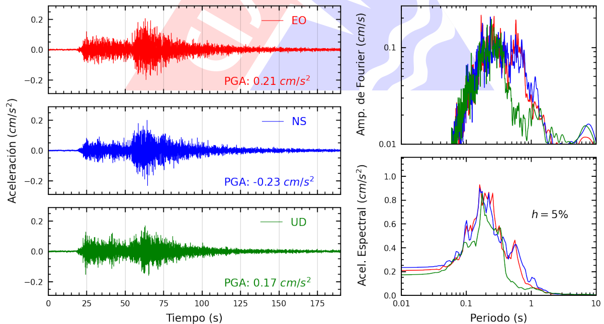
Figura A.8: Registros tiempo-historia, espectros de Fourier y de respuesta en las direcciones EO, NS y vertical de la estación CARAL. Sismo de Puerto Bermudez, Oxapampa - Pasco del 2024-05-24, 04:58:47 (Hora local)
