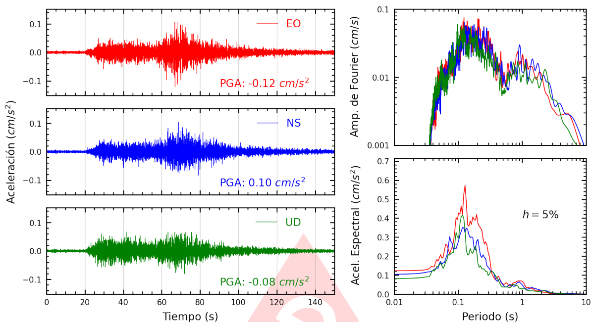
Figura A.19: Registros tiempo-historia, espectros de Fourier y de respuesta en las direcciones EO, NS y vertical de la estación JALV2. Sismo de Puerto Bermudez, Oxapampa - Pasco del 2024-05-24, 04:58:47 (Hora local)
