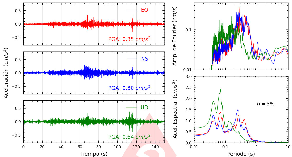
Figura A.3: Registros tiempo-historia, espectros de Fourier y de respuesta en las direcciones EO, NS y vertical de la estación MDPP. Sismo de Puerto Bermudez, Oxapampa - Pasco del 2024-05-24, 04:58:47 (Hora local)
