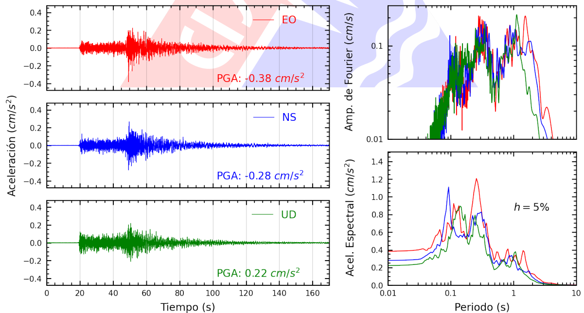
Figura A.6: Registros tiempo-historia, espectros de Fourier y de respuesta en las direcciones EO, NS y vertical de la estación UNCP. Sismo de Puerto Bermudez, Oxapampa - Pasco del 2024-05-24, 04:58:47 (Hora local)
