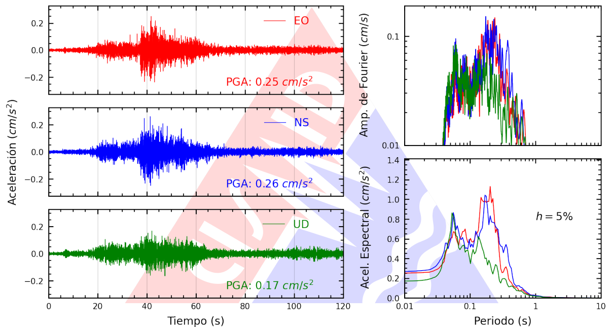
Figura A.3: Registros tiempo-historia, espectros de Fourier y de respuesta en las direcciones EO, NS y vertical de la estación ASIA. Sismo de Ica, Ica - Ica del 2024-05-28, 09:44:41 (Hora local)
