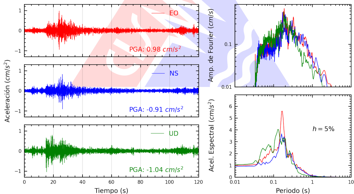
Figura A.2: Registros tiempo-historia, espectros de Fourier y de respuesta en las direcciones EO, NS y vertical de la estación SCICA. Sismo de Ica, Ica - Ica del 2024-05-28, 09:44:41 (Hora local)
