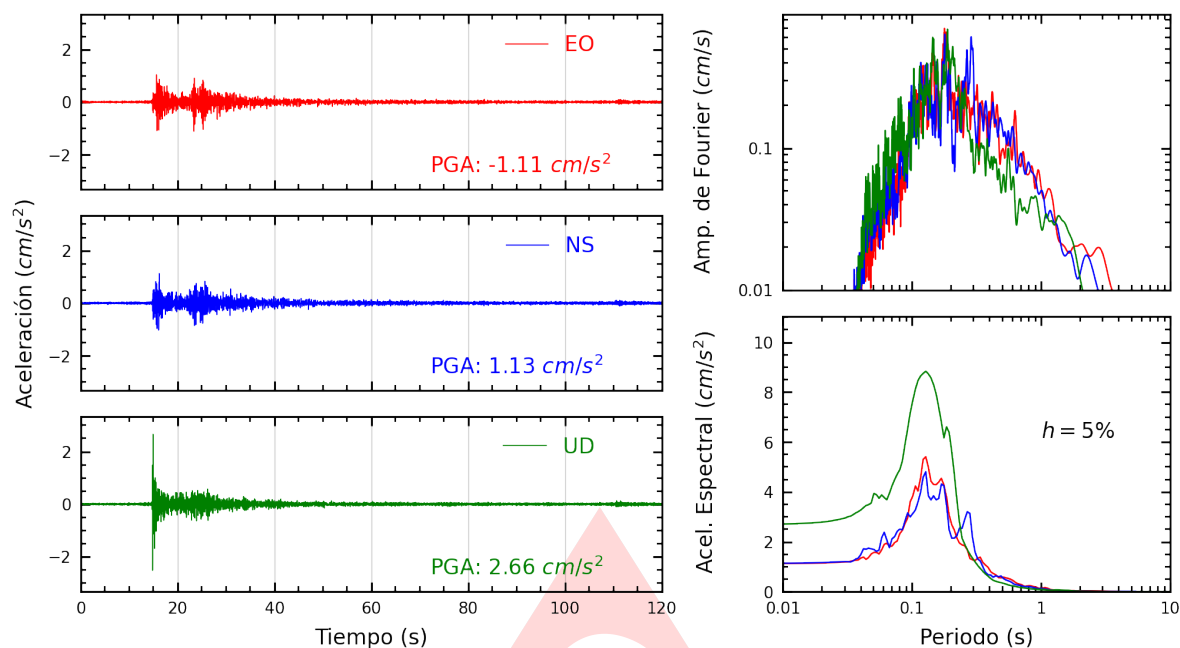
Figura A.1: Registros tiempo-historia, espectros de Fourier y de respuesta en las direcciones EO, NS y vertical de la estación UNICA. Sismo de Ica, Ica - Ica del 2024-05-28, 09:44:41 (Hora local)
