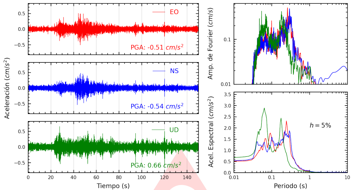
Figura A.1: Registros tiempo-historia, espectros de Fourier y de respuesta en las direcciones EO, NS y vertical de la estación SCTAC. Sismo de Ilo, Ilo - Moquegua del 2024-05-29, 14:34:43 (Hora local)
