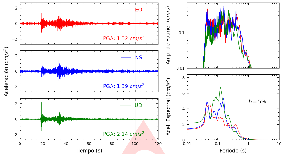
Figura A.1: Registros tiempo-historia, espectros de Fourier y de respuesta en las direcciones EO, NS y vertical de la estación SCTR. Sismo de San Pedro De Lloc, Pacasmayo - La Libertad del 2024-06-08, 07:06:46 (Hora local)
