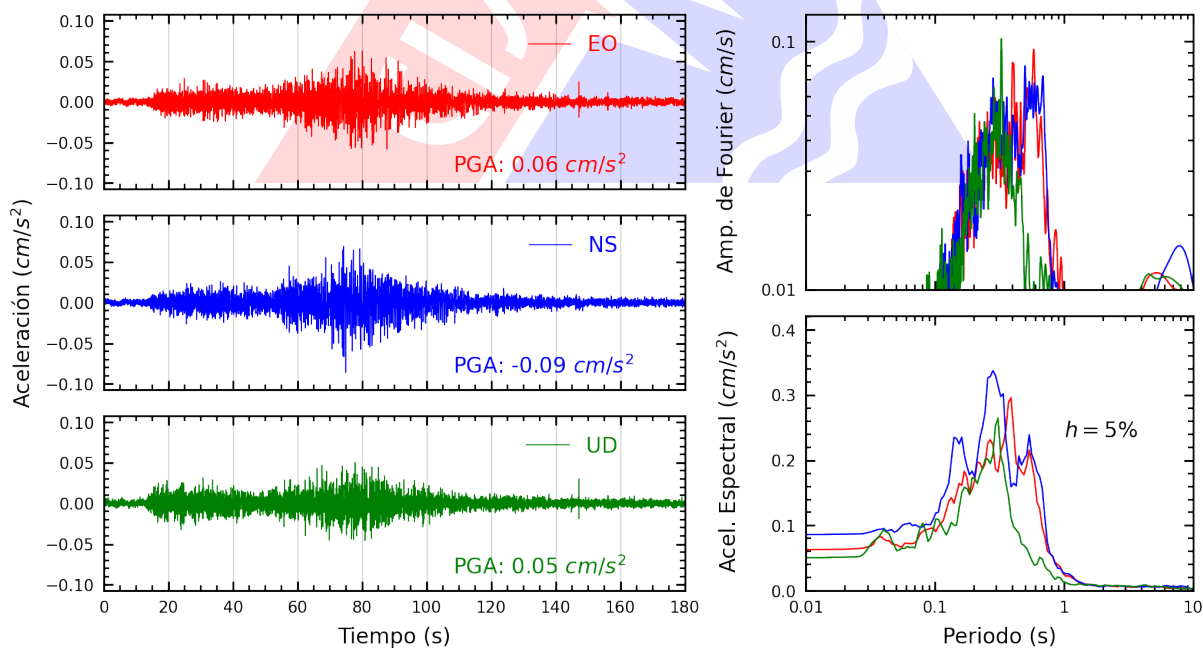
Figura A.4: Registros tiempo-historia, espectros de Fourier y de respuesta en las direcciones EO, NS y vertical de la estación CARAL. Sismo de San Pedro De Lloc, Pacasmayo - La Libertad del 2024-06-08, 07:06:46 (Hora local)
