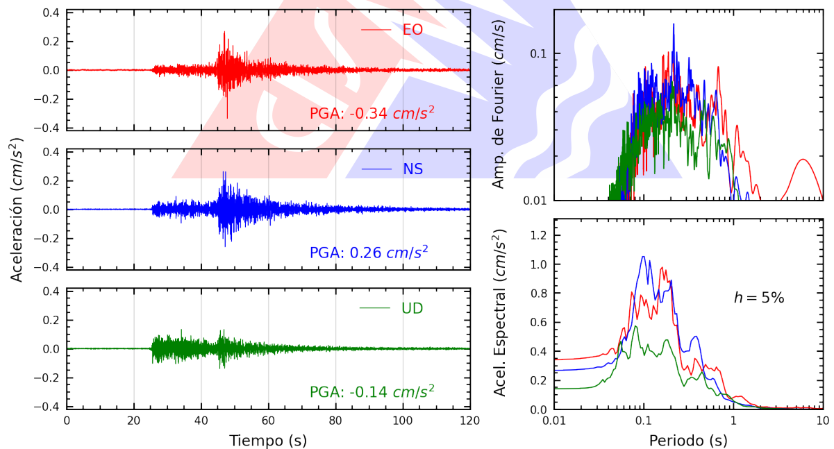
Figura A.2: Registros tiempo-historia, espectros de Fourier y de respuesta en las direcciones EO, NS y vertical de la estación SCCH. Sismo de San Pedro De Lloc, Pacasmayo - La Libertad del 2024-06-08, 07:06:46 (Hora local)
