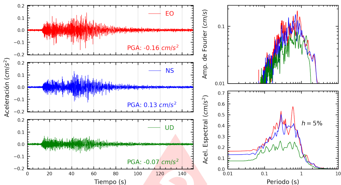
Figura A.3: Registros tiempo-historia, espectros de Fourier y de respuesta en las direcciones EO, NS y vertical de la estación UNC. Sismo de San Pedro De Lloc, Pacasmayo - La Libertad del 2024-06-08, 07:06:46 (Hora local)
