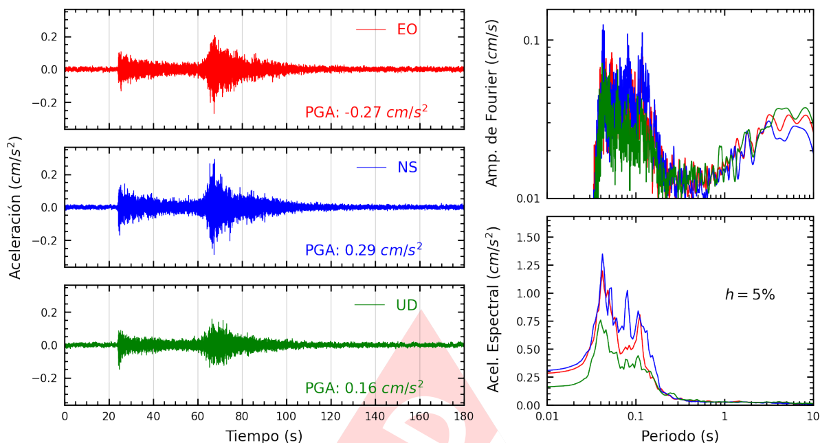
Figura A.5: Registros tiempo-historia, espectros de Fourier y de respuesta en las direcciones EO, NS y vertical de la estación JOSEO. Sismo de Chimbote, Santa - Ancash del 2024-06-11, 02:34:17 (Hora local)
