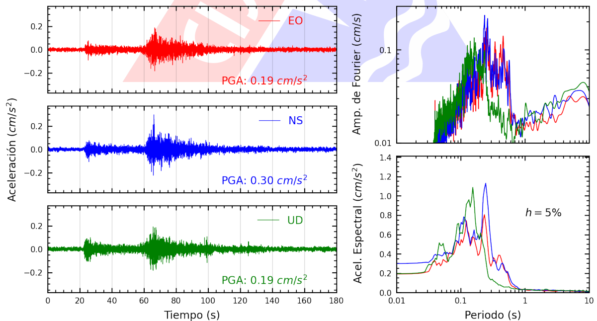
Figura A.4: Registros tiempo-historia, espectros de Fourier y de respuesta en las direcciones EO, NS y vertical de la estación MDPP. Sismo de Chimbote, Santa - Ancash del 2024-06-11, 02:34:17 (Hora local)
