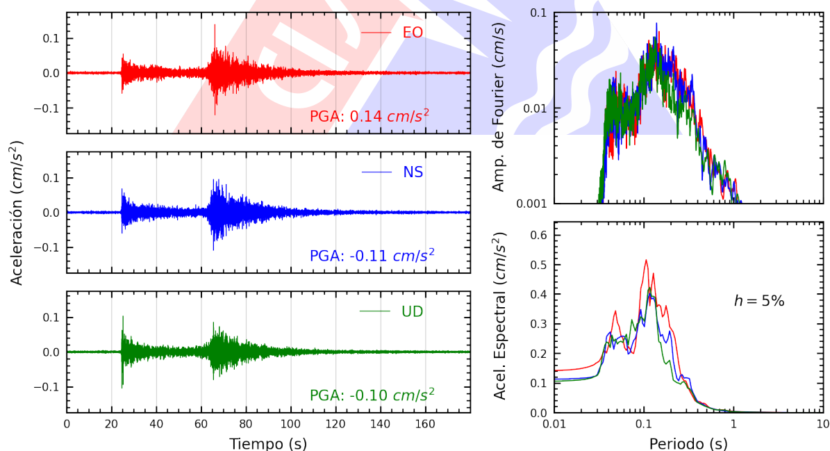
Figura A.10: Registros tiempo-historia, espectros de Fourier y de respuesta en las direcciones EO, NS y vertical de la estación JALV2. Sismo de Chimbote, Santa - Ancash del 2024-06-11, 02:34:17 (Hora local)
