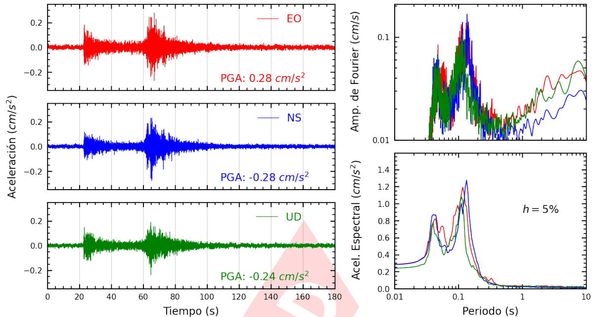
Figura A.7: Registros tiempo-historia, espectros de Fourier y de respuesta en las direcciones EO, NS y vertical de la estación AMORE. Sismo de Chimbote, Santa - Ancash del 2024-06-11, 02:34:17 (Hora local)
