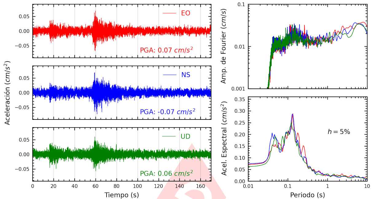
Figura A.15: Registros tiempo-historia, espectros de Fourier y de respuesta en las direcciones EO, NS y vertical de la estación SERVI. Sismo de Chimbote, Santa - Ancash del 2024-06-11, 02:34:17 (Hora local)
