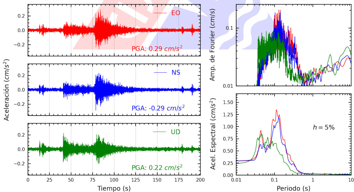
Figura A.6: Registros tiempo-historia, espectros de Fourier y de respuesta en las direcciones EO, NS y vertical de la estación ANCON. Sismo de Chimbote, Santa - Ancash del 2024-06-11, 02:34:17 (Hora local)
