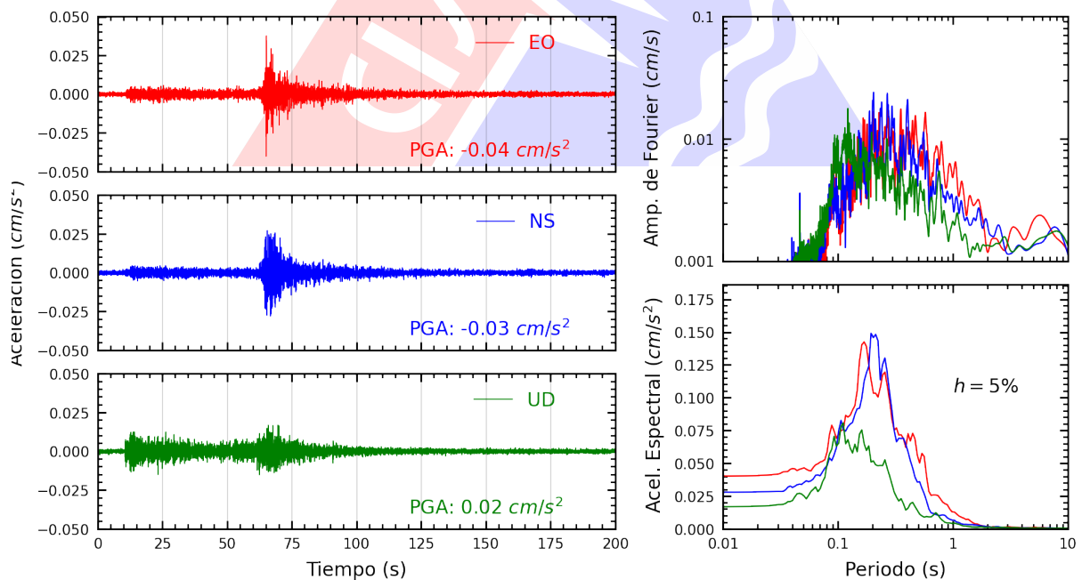
Figura A.18: Registros tiempo-historia, espectros de Fourier y de respuesta en las direcciones EO, NS y vertical de la estación UNIA. Sismo de Chimbote, Santa - Ancash del 2024-06-11, 02:34:17 (Hora local)
