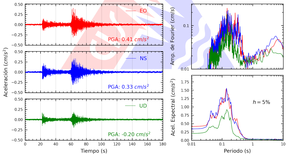
Figura A.2: Registros tiempo-historia, espectros de Fourier y de respuesta en las direcciones EO, NS y vertical de la estación DEFEN. Sismo de Chimbote, Santa - Ancash del 2024-06-11, 02:34:17 (Hora local)
