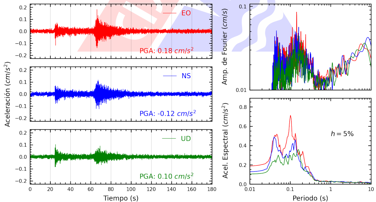
Figura A.8: Registros tiempo-historia, espectros de Fourier y de respuesta en las direcciones EO, NS y vertical de la estación FICPE. Sismo de Chimbote, Santa - Ancash del 2024-06-11, 02:34:17 (Hora local)
