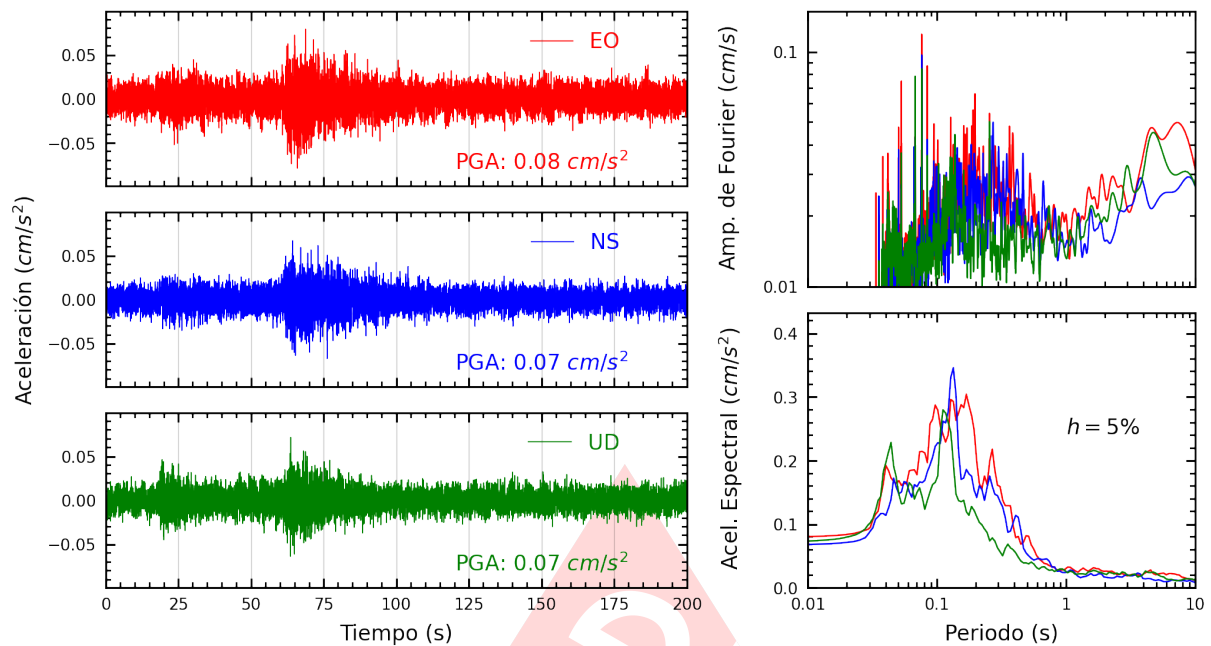
Figura A.13: Registros tiempo-historia, espectros de Fourier y de respuesta en las direcciones EO, NS y vertical de la estación USILP. Sismo de Chimbote, Santa - Ancash del 2024-06-11, 02:34:17 (Hora local)
