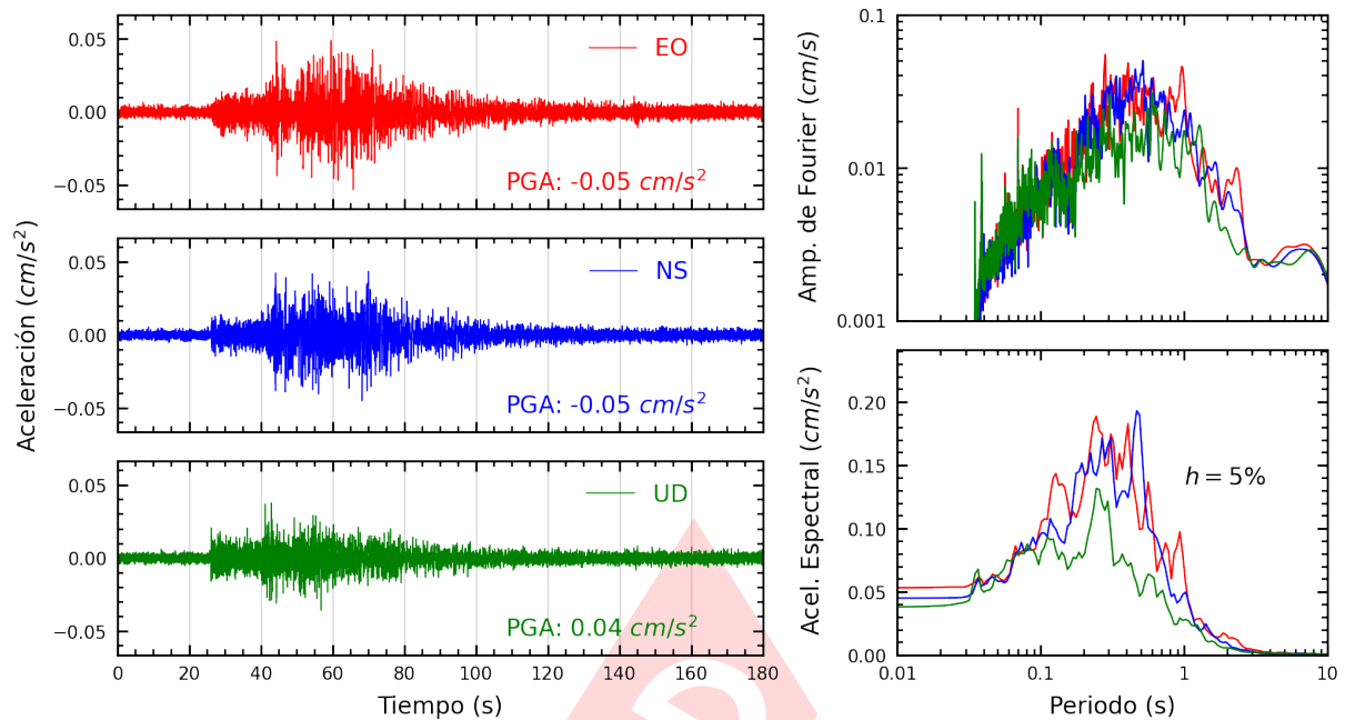
Figura A.17: Registros tiempo-historia, espectros de Fourier y de respuesta en las direcciones EO, NS y vertical de la estación UNC. Sismo de Chimbote, Santa - Ancash del 2024-06-11, 02:34:17 (Hora local)
