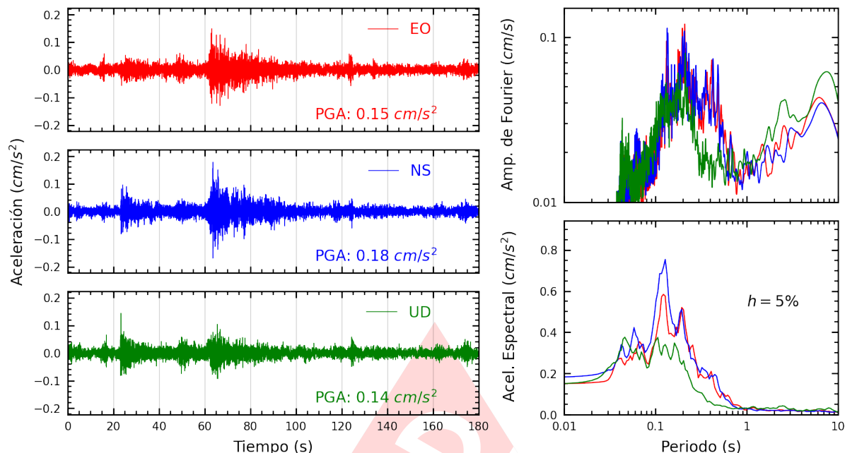
Figura A.9: Registros tiempo-historia, espectros de Fourier y de respuesta en las direcciones EO, NS y vertical de la estación VHAYA. Sismo de Chimbote, Santa - Ancash del 2024-06-11, 02:34:17 (Hora local)
