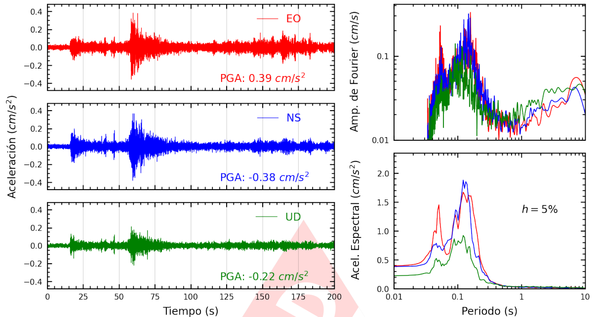
Figura A.3: Registros tiempo-historia, espectros de Fourier y de respuesta en las direcciones EO, NS y vertical de la estación USILM. Sismo de Chimbote, Santa - Ancash del 2024-06-11, 02:34:17 (Hora local)
