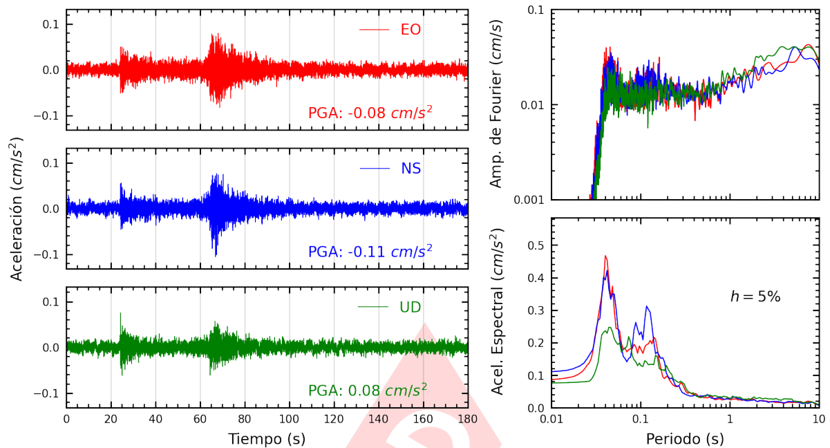
Figura A.11: Registros tiempo-historia, espectros de Fourier y de respuesta en las direcciones EO, NS y vertical de la estación UCSS. Sismo de Chimbote, Santa - Ancash del 2024-06-11, 02:34:17 (Hora local)
