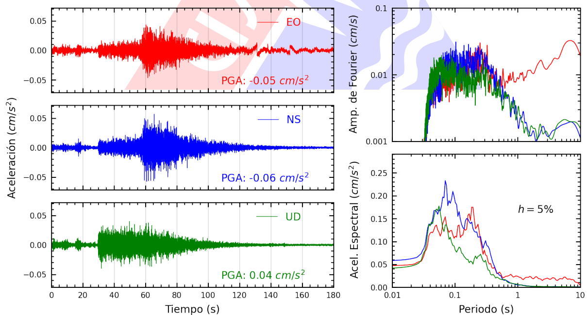
Figura A.16: Registros tiempo-historia, espectros de Fourier y de respuesta en las direcciones EO, NS y vertical de la estación SCCHI. Sismo de Chimbote, Santa - Ancash del 2024-06-11, 02:34:17 (Hora local)
