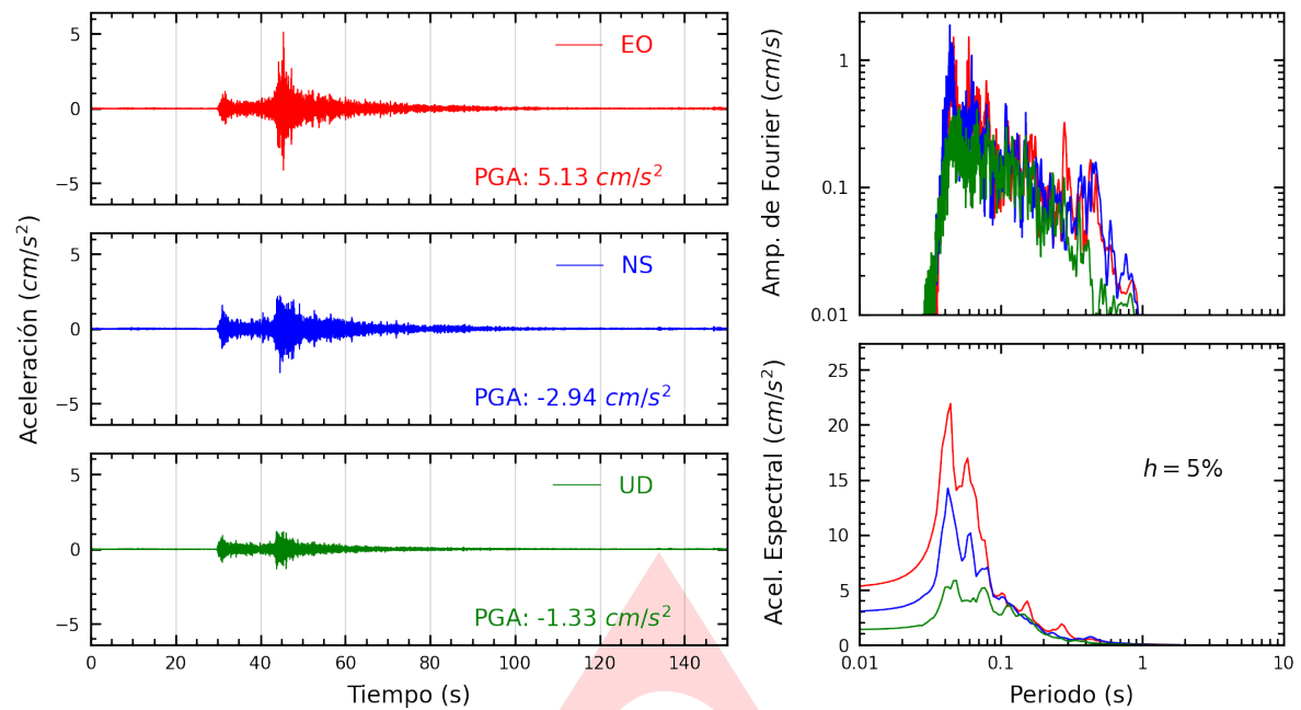
Figura A.1: Registros tiempo-historia, espectros de Fourier y de respuesta en las direcciones EO, NS y vertical de la estación SCTRU. Sismo de Chimbote, Santa - Ancash del 2024-06-11, 02:34:17 (Hora local)
