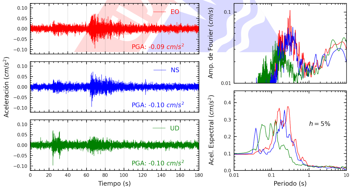
Figura A.12: Registros tiempo-historia, espectros de Fourier y de respuesta en las direcciones EO, NS y vertical de la estación ACAPU. Sismo de Chimbote, Santa - Ancash del 2024-06-11, 02:34:17 (Hora local)
