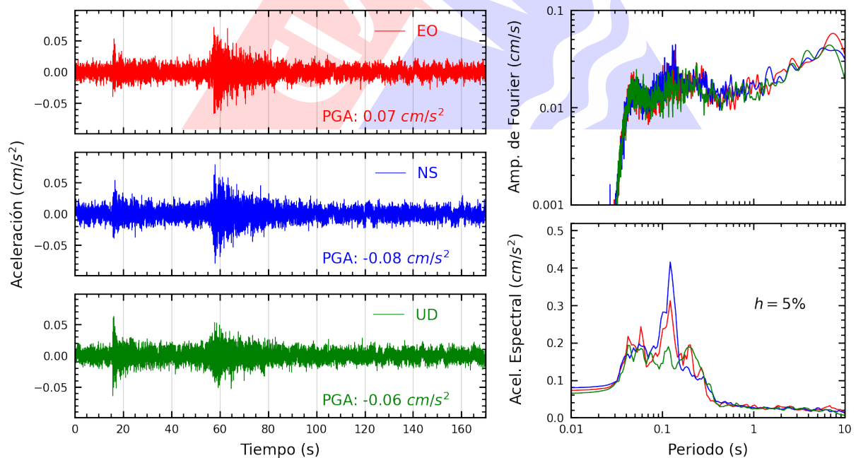
Figura A.14: Registros tiempo-historia, espectros de Fourier y de respuesta en las direcciones EO, NS y vertical de la estación CENEP. Sismo de Chimbote, Santa - Ancash del 2024-06-11, 02:34:17 (Hora local)
