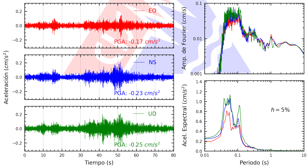
Figura A.2: Registros tiempo-historia, espectros de Fourier y de respuesta en las direcciones EO, NS y vertical de la estación UNICA. Sismo de Marcona, Nazca - Ica del 2024-06-11, 14:03:41 (Hora local)
