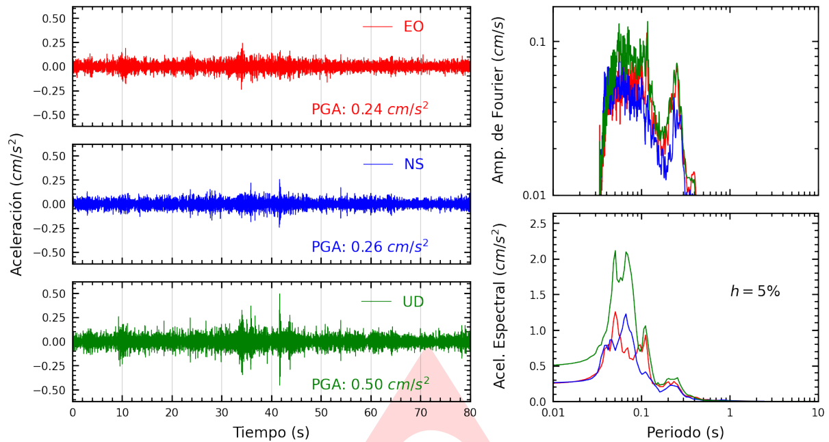
Figura A.1: Registros tiempo-historia, espectros de Fourier y de respuesta en las direcciones EO, NS y vertical de la estación SCICA. Sismo de Marcona, Nazca - Ica del 2024-06-11, 14:03:41 (Hora local)
