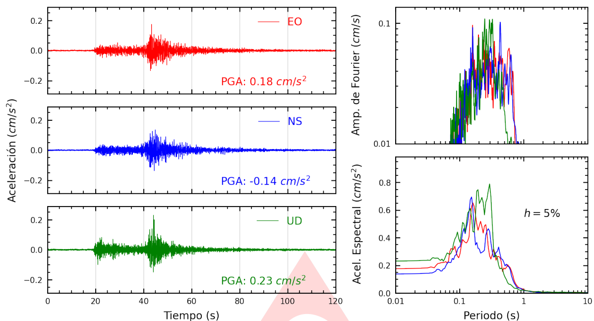
Figura A.1: Registros tiempo-historia, espectros de Fourier y de respuesta en las direcciones EO, NS y vertical de la estación CARAL. Sismo de Huarney, Huarney - Ancash del 2024-06-15, 04:53:26 (Hora local)
