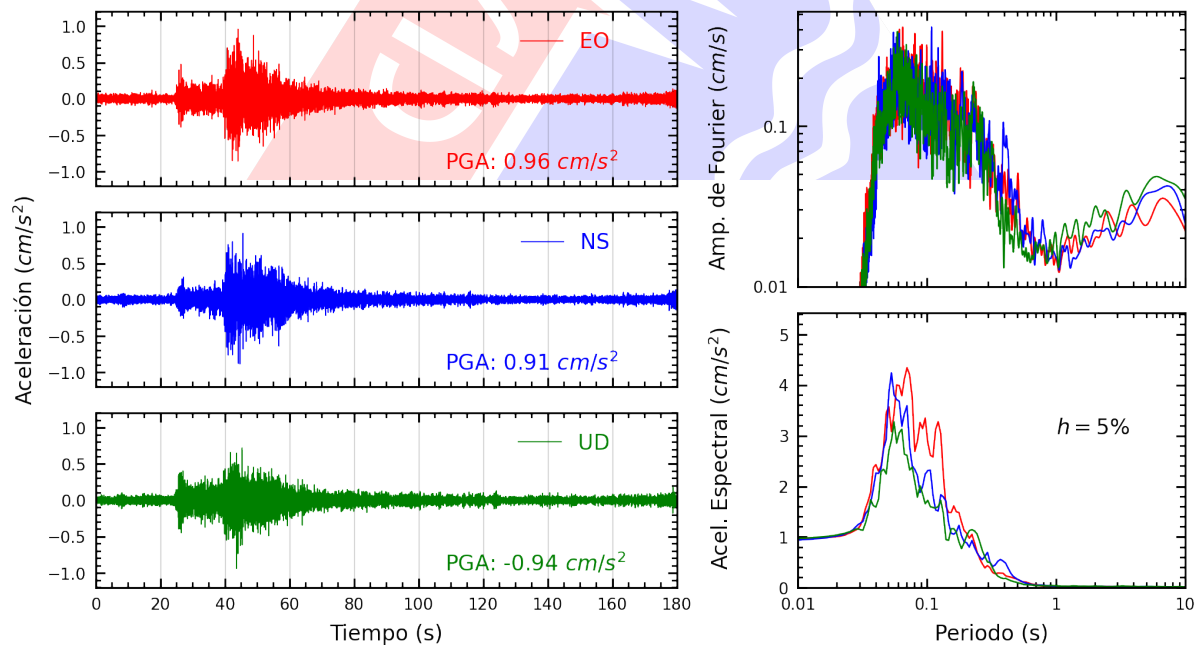
Figura A.16: Registros tiempo-historia, espectros de Fourier y de respuesta en las direcciones EO, NS y vertical de la estación URPE. Sismo de San Vicente De Cañete, Cañete - Lima del 2024-06-18, 19:48:13 (Hora local)
