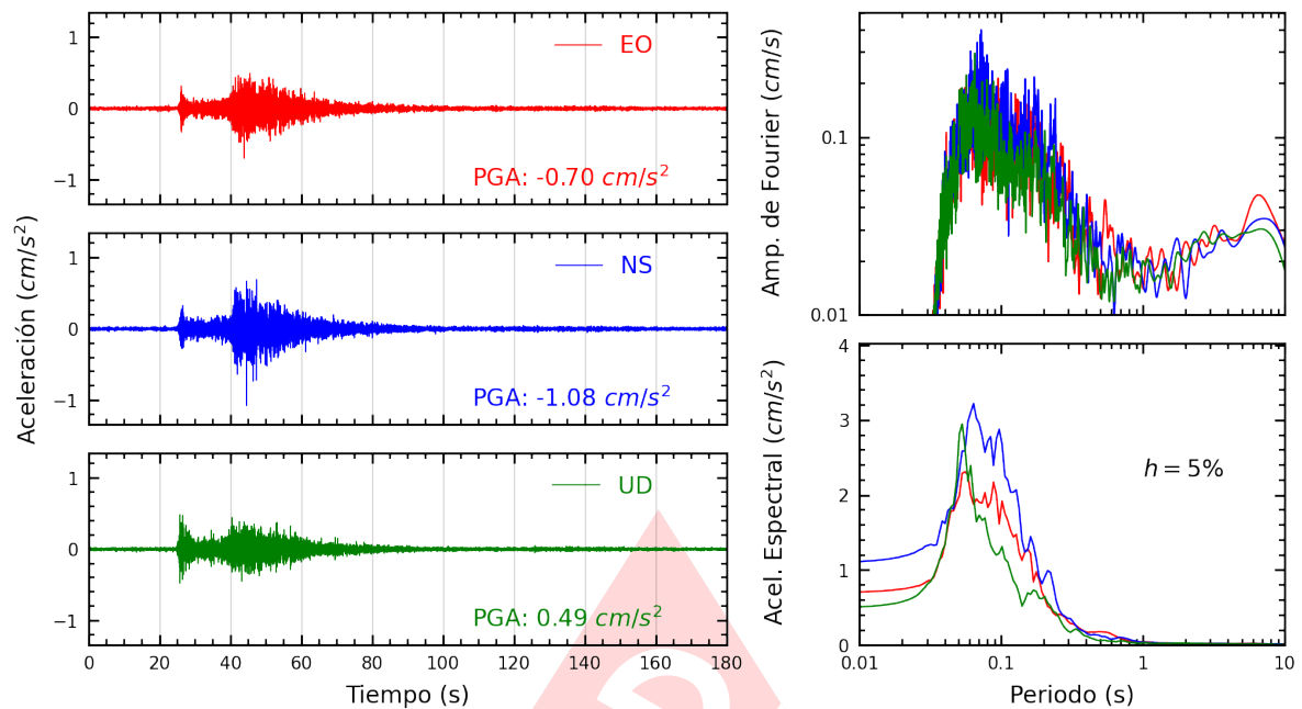
Figura A.13: Registros tiempo-historia, espectros de Fourier y de respuesta en las direcciones EO, NS y vertical de la estación SERVI. Sismo de San Vicente De Cañete, Cañete - Lima del 2024-06-18, 19:48:13 (Hora local)
