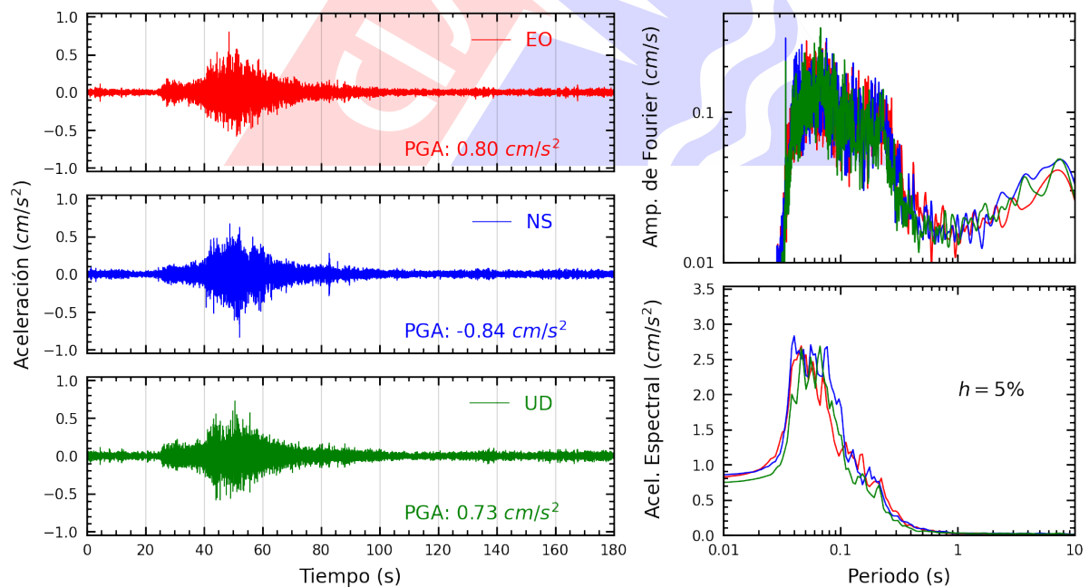
Figura A.20: Registros tiempo-historia, espectros de Fourier y de respuesta en las direcciones EO, NS y vertical de la estación USMP. Sismo de San Vicente De Cañete, Cañete - Lima del 2024-06-18, 19:48:13 (Hora local)
