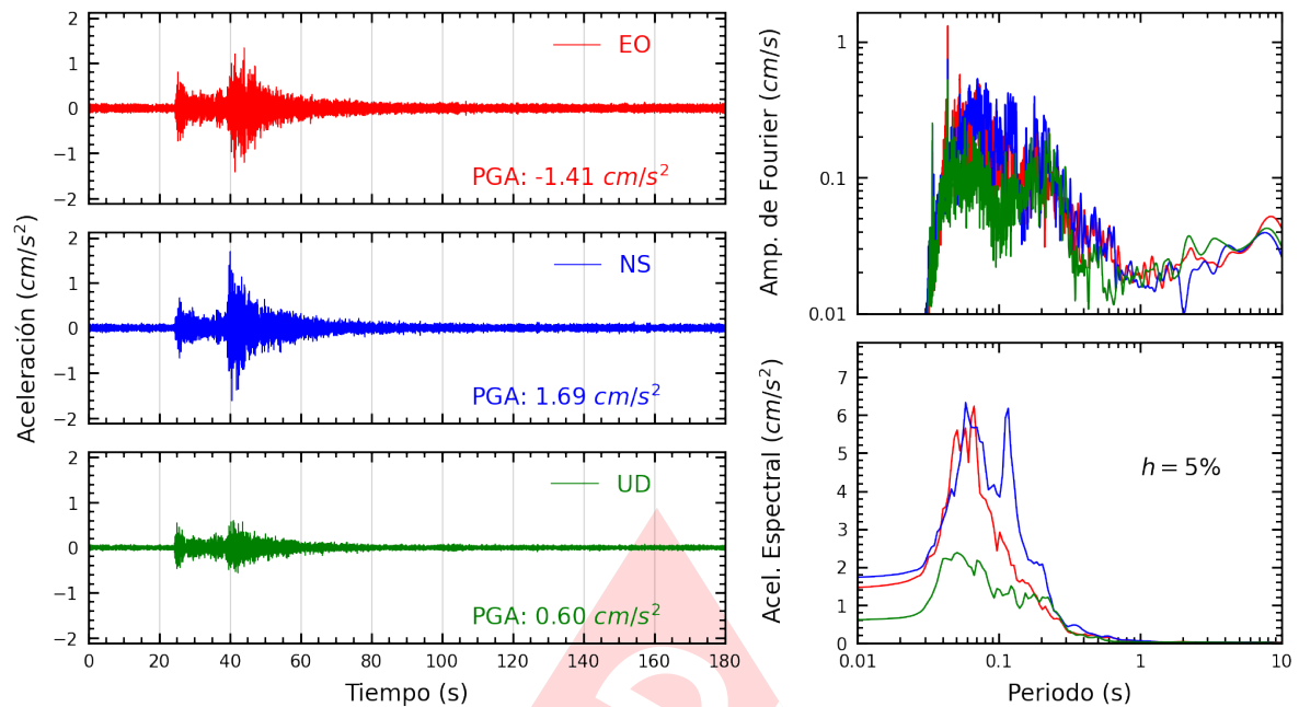
Figura A.9: Registros tiempo-historia, espectros de Fourier y de respuesta en las direcciones EO, NS y vertical de la estación UPCVI. Sismo de San Vicente De Cañete, Cañete - Lima del 2024-06-18, 19:48:13 (Hora local)
