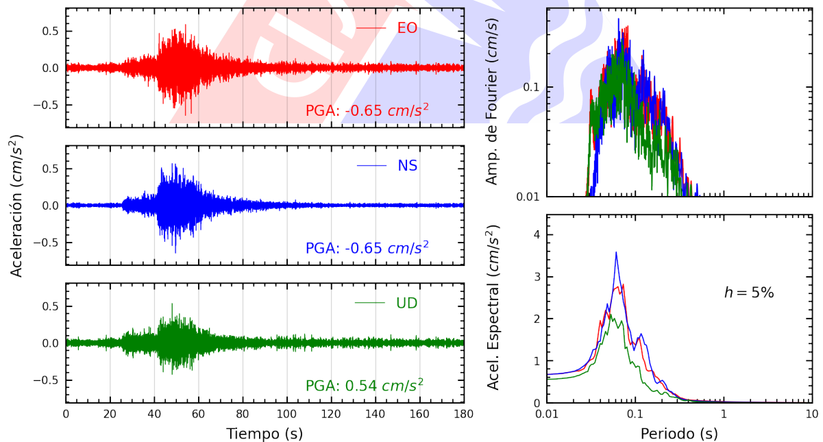
Figura A.26: Registros tiempo-historia, espectros de Fourier y de respuesta en las direcciones EO, NS y vertical de la estación ATARJ. Sismo de San Vicente De Cañete, Cañete - Lima del 2024-06-18, 19:48:13 (Hora local)
