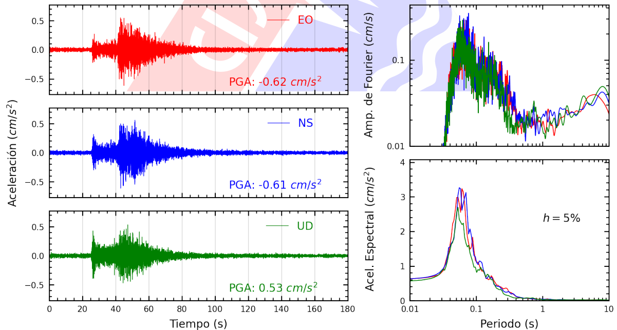
Figura A.28: Registros tiempo-historia, espectros de Fourier y de respuesta en las direcciones EO, NS y vertical de la estación CENEP. Sismo de San Vicente De Cañete, Cañete - Lima del 2024-06-18, 19:48:13 (Hora local)
