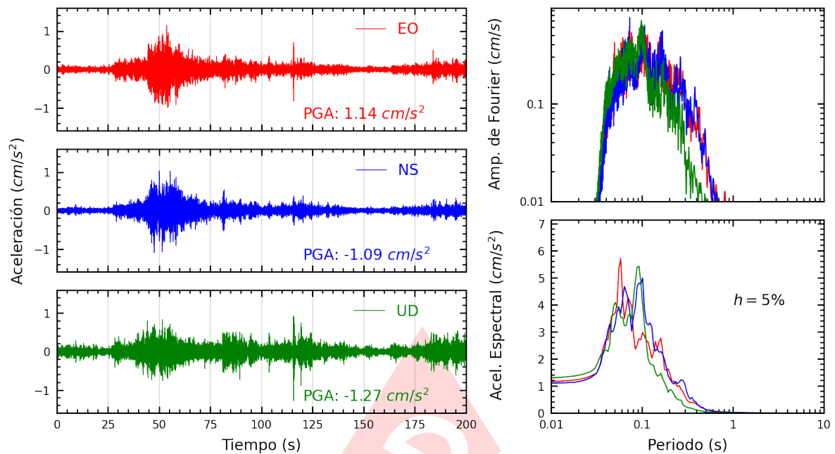
Figura A.11: Registros tiempo-historia, espectros de Fourier y de respuesta en las direcciones EO, NS y vertical de la estación SCOLI. Sismo de San Vicente De Cañete, Cañete - Lima del 2024-06-18, 19:48:13 (Hora local)
