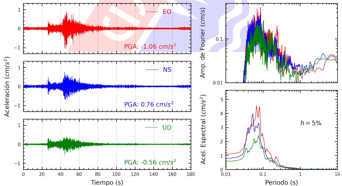
Figura A.14: Registros tiempo-historia, espectros de Fourier y de respuesta en las direcciones EO, NS y vertical de la estación CEPRE. Sismo de San Vicente De Cañete, Cañete - Lima del 2024-06-18, 19:48:13 (Hora local)
