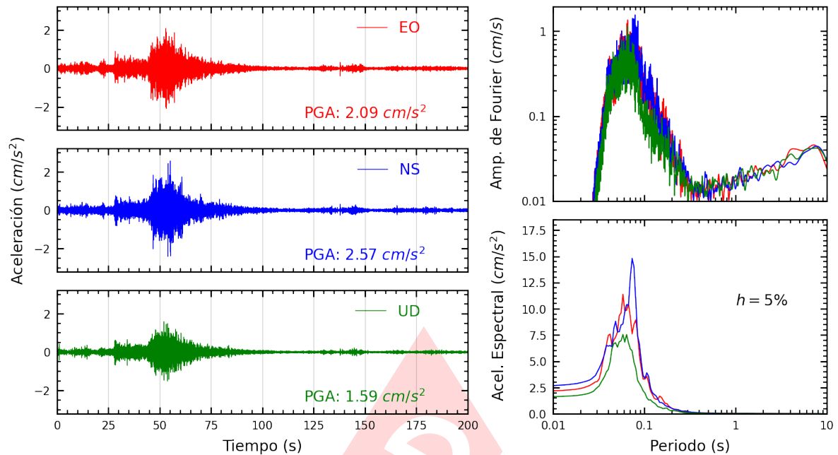
Figura A.3: Registros tiempo-historia, espectros de Fourier y de respuesta en las direcciones EO, NS y vertical de la estación JOSEO. Sismo de San Vicente De Cañete, Cañete - Lima del 2024-06-18, 19:48:13 (Hora local)
