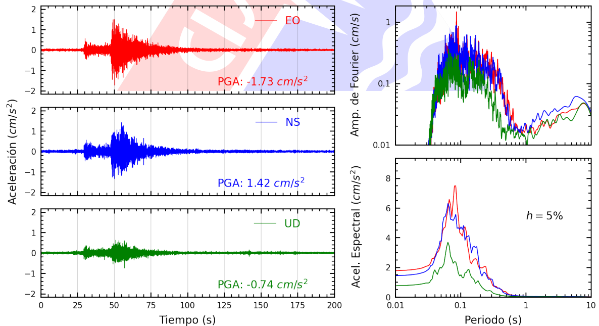
Figura A.8: Registros tiempo-historia, espectros de Fourier y de respuesta en las direcciones EO, NS y vertical de la estación DEFEN. Sismo de San Vicente De Cañete, Cañete - Lima del 2024-06-18, 19:48:13 (Hora local)
