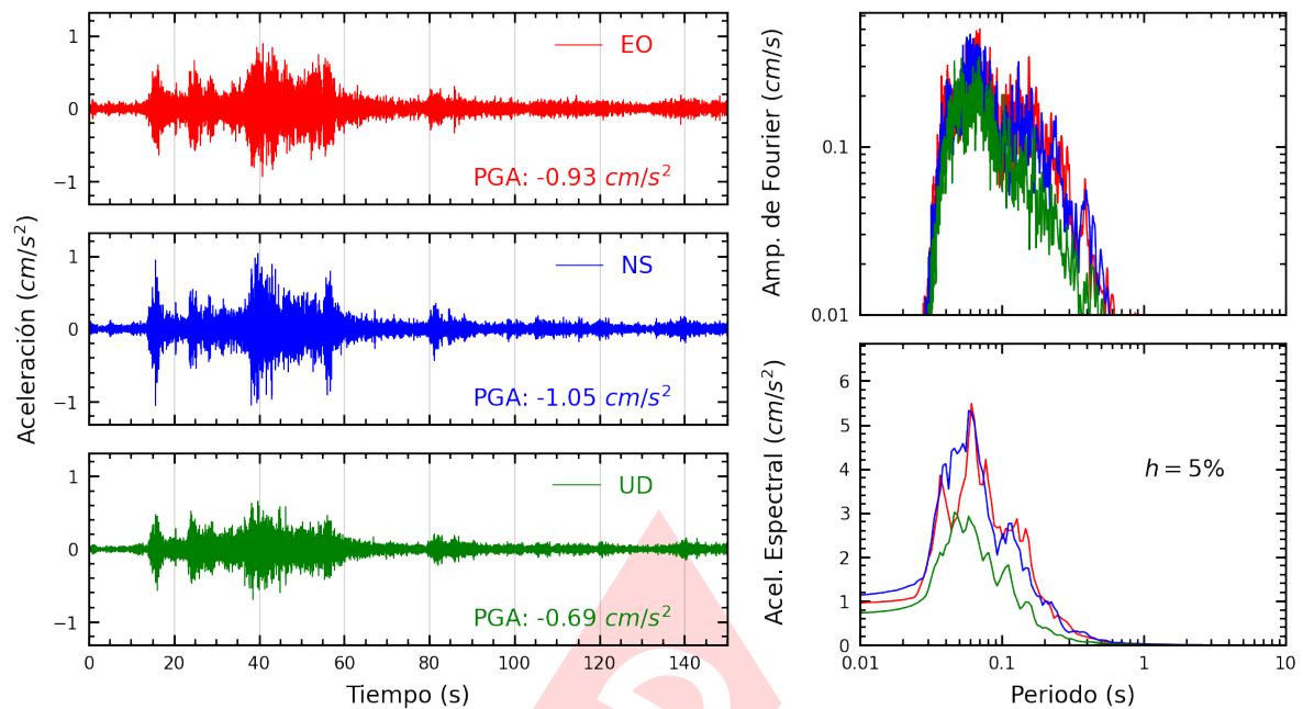
Figura A.15: Registros tiempo-historia, espectros de Fourier y de respuesta en las direcciones EO, NS y vertical de la estación PACHA. Sismo de San Vicente De Cañete, Cañete - Lima del 2024-06-18, 19:48:13 (Hora local)
