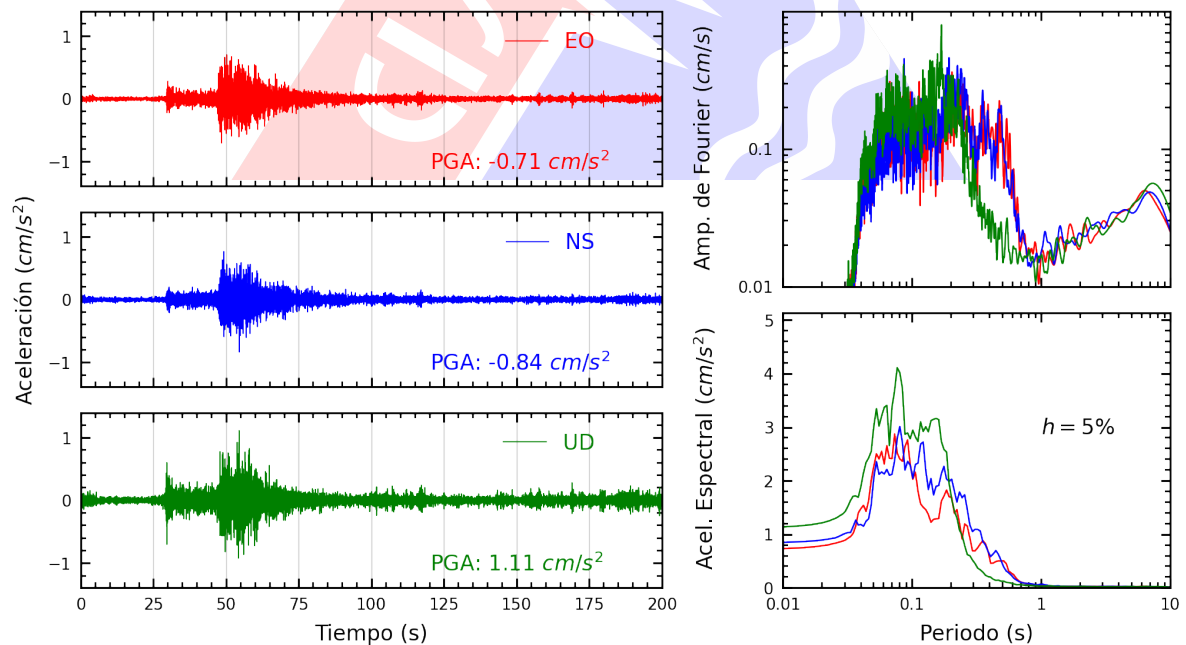
Figura A.12: Registros tiempo-historia, espectros de Fourier y de respuesta en las direcciones EO, NS y vertical de la estación MDPP. Sismo de San Vicente De Cañete, Cañete - Lima del 2024-06-18, 19:48:13 (Hora local)
