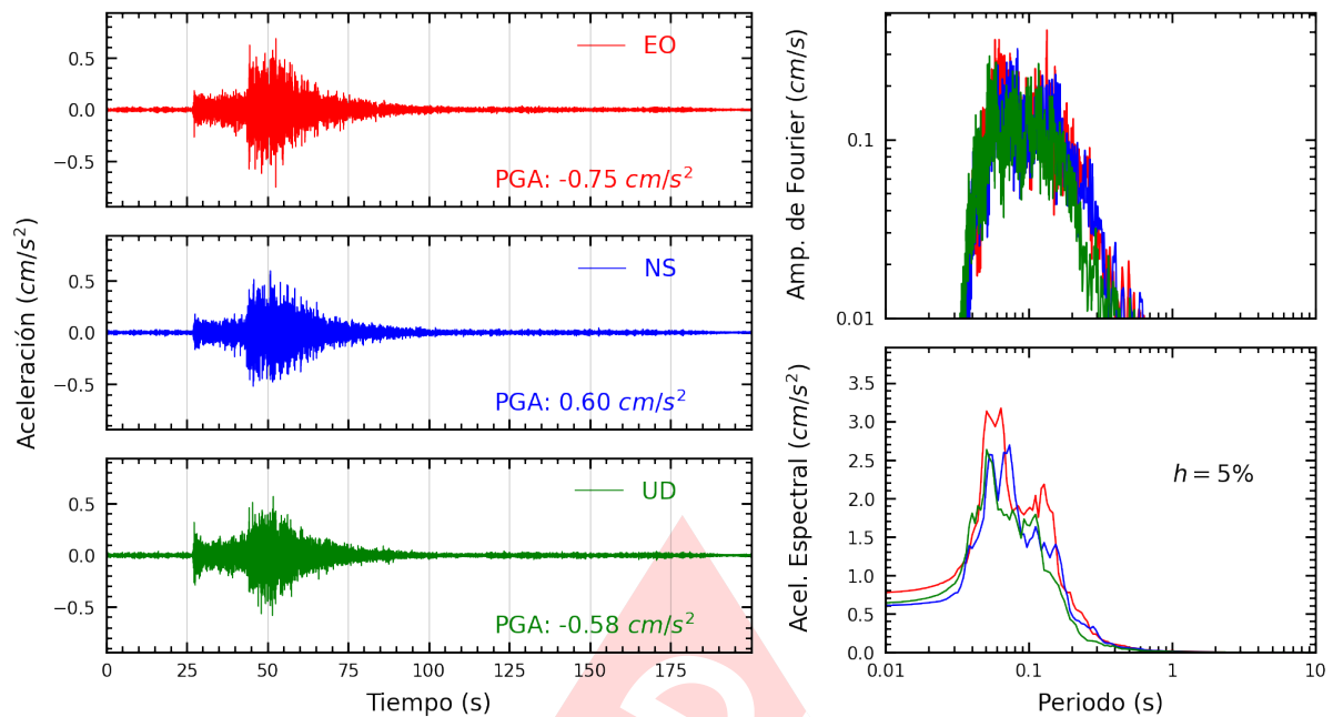
Figura A.21: Registros tiempo-historia, espectros de Fourier y de respuesta en las direcciones EO, NS y vertical de la estación JALV2. Sismo de San Vicente De Cañete, Cañete - Lima del 2024-06-18, 19:48:13 (Hora local)
