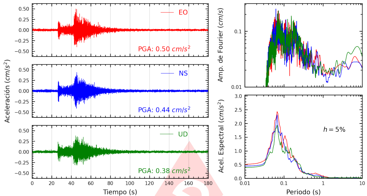
Figura A.33: Registros tiempo-historia, espectros de Fourier y de respuesta en las direcciones EO, NS y vertical de la estación UNFV. Sismo de San Vicente De Cañete, Cañete - Lima del 2024-06-18, 19:48:13 (Hora local)
