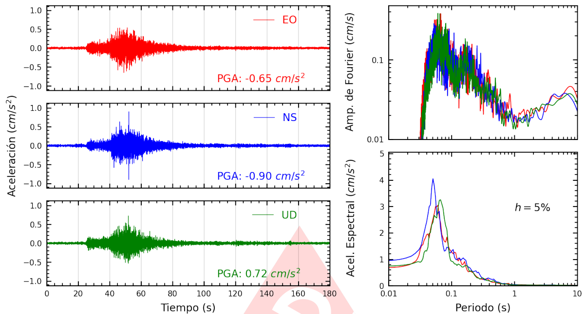
Figura A.19: Registros tiempo-historia, espectros de Fourier y de respuesta en las direcciones EO, NS y vertical de la estación IMCA. Sismo de San Vicente De Cañete, Cañete - Lima del 2024-06-18, 19:48:13 (Hora local)
