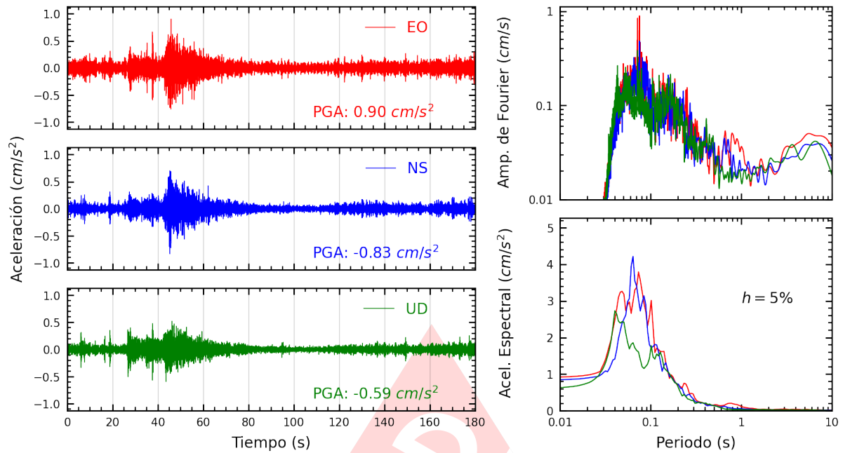
Figura A.17: Registros tiempo-historia, espectros de Fourier y de respuesta en las direcciones EO, NS y vertical de la estación UPCS. Sismo de San Vicente De Cañete, Cañete - Lima del 2024-06-18, 19:48:13 (Hora local)
