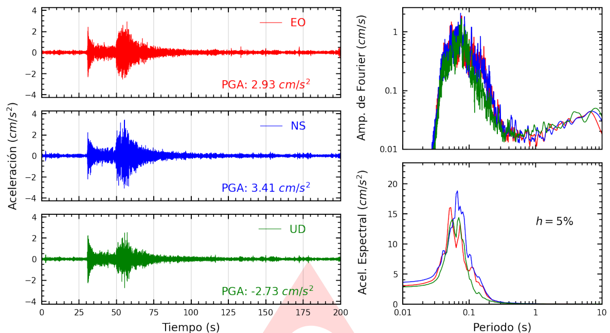
Figura A.1: Registros tiempo-historia, espectros de Fourier y de respuesta en las direcciones EO, NS y vertical de la estación SROSA. Sismo de San Vicente De Cañete, Cañete - Lima del 2024-06-18, 19:48:13 (Hora local)
