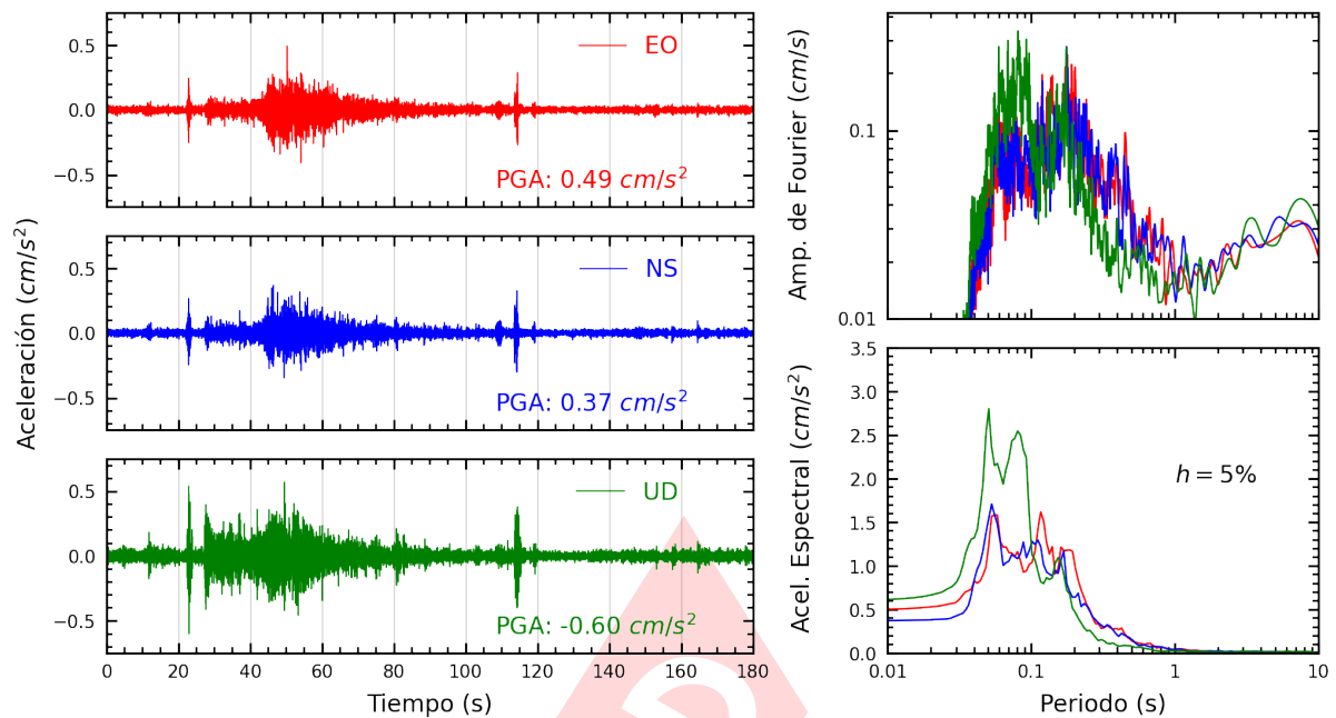
Figura A.29: Registros tiempo-historia, espectros de Fourier y de respuesta en las direcciones EO, NS y vertical de la estación RAMON. Sismo de San Vicente De Cañete, Cañete - Lima del 2024-06-18, 19:48:13 (Hora local)
