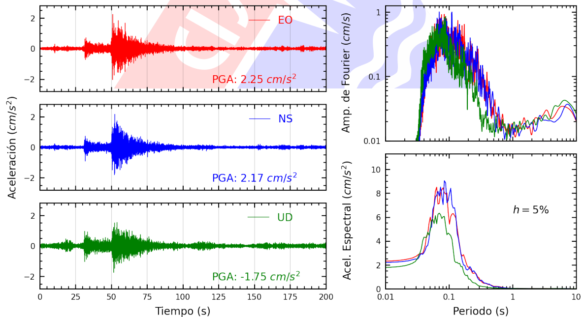
Figura A.4: Registros tiempo-historia, espectros de Fourier y de respuesta en las direcciones EO, NS y vertical de la estación ANCON. Sismo de San Vicente De Cañete, Cañete - Lima del 2024-06-18, 19:48:13 (Hora local)
