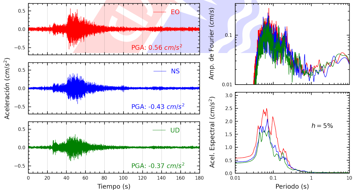
Figura A.30: Registros tiempo-historia, espectros de Fourier y de respuesta en las direcciones EO, NS y vertical de la estación INICT. Sismo de San Vicente De Cañete, Cañete - Lima del 2024-06-18, 19:48:13 (Hora local)
