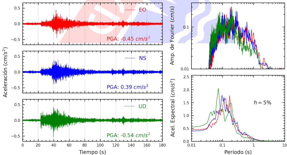
Figura A.32: Registros tiempo-historia, espectros de Fourier y de respuesta en las direcciones EO, NS y vertical de la estación UNICA. Sismo de San Vicente De Cañete, Cañete - Lima del 2024-06-18, 19:48:13 (Hora local)
