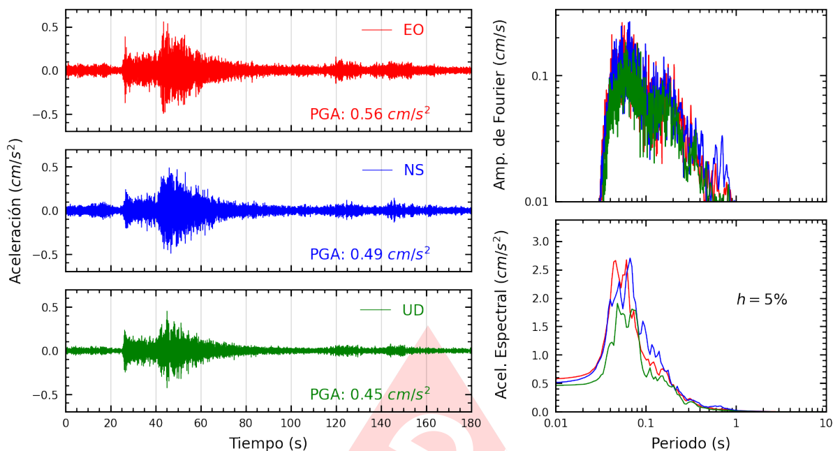
Figura A.31: Registros tiempo-historia, espectros de Fourier y de respuesta en las direcciones EO, NS y vertical de la estación BORJA. Sismo de San Vicente De Cañete, Cañete - Lima del 2024-06-18, 19:48:13 (Hora local)
