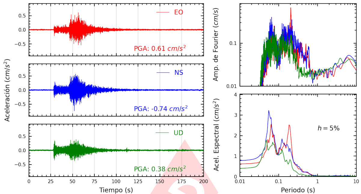
Figura A.23: Registros tiempo-historia, espectros de Fourier y de respuesta en las direcciones EO, NS y vertical de la estación VHAYA. Sismo de San Vicente De Cañete, Cañete - Lima del 2024-06-18, 19:48:13 (Hora local)
