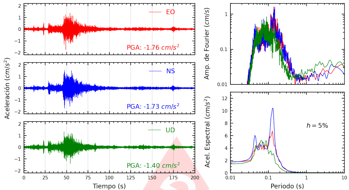
Figura A.7: Registros tiempo-historia, espectros de Fourier y de respuesta en las direcciones EO, NS y vertical de la estación CARAB. Sismo de San Vicente De Cañete, Cañete - Lima del 2024-06-18, 19:48:13 (Hora local)
