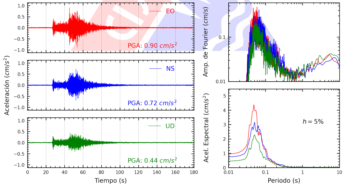
Figura A.18: Registros tiempo-historia, espectros de Fourier y de respuesta en las direcciones EO, NS y vertical de la estación UCSS. Sismo de San Vicente De Cañete, Cañete - Lima del 2024-06-18, 19:48:13 (Hora local)
