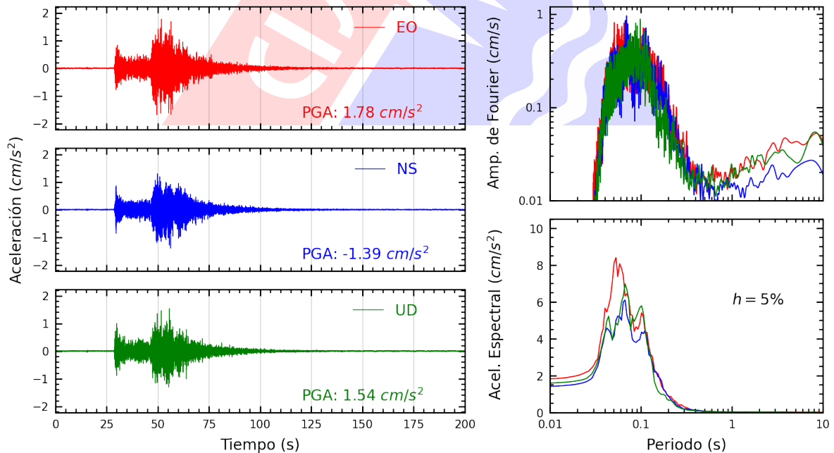
Figura A.6: Registros tiempo-historia, espectros de Fourier y de respuesta en las direcciones EO, NS y vertical de la estación AMORE. Sismo de San Vicente De Cañete, Cañete - Lima del 2024-06-18, 19:48:13 (Hora local)
