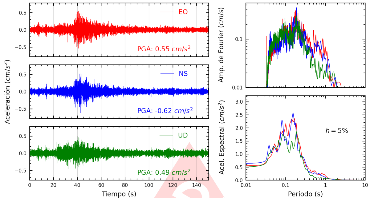
Figura A.27: Registros tiempo-historia, espectros de Fourier y de respuesta en las direcciones EO, NS y vertical de la estación SCICA. Sismo de San Vicente De Cañete, Cañete - Lima del 2024-06-18, 19:48:13 (Hora local)
