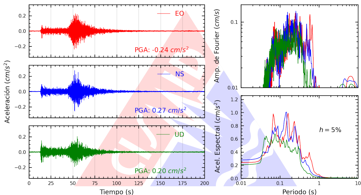
Figura A.35: Registros tiempo-historia, espectros de Fourier y de respuesta en las direcciones EO, NS y vertical de la estación CARAL. Sismo de San Vicente De Cañete, Cañete - Lima del 2024-06-18, 19:48:13 (Hora local)
