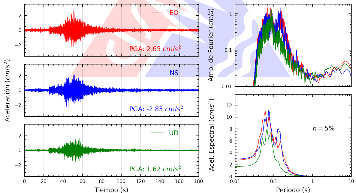
Figura A.2: Registros tiempo-historia, espectros de Fourier y de respuesta en las direcciones EO, NS y vertical de la estación USILM. Sismo de San Vicente De Cañete, Cañete - Lima del 2024-06-18, 19:48:13 (Hora local)
