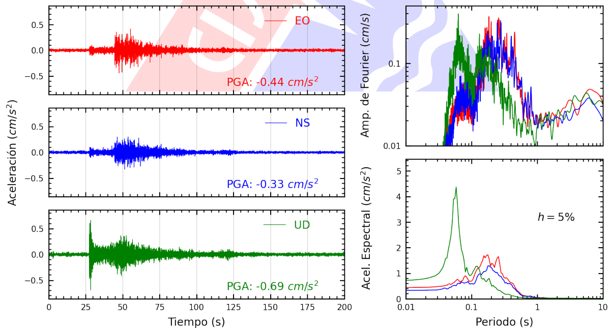
Figura A.24: Registros tiempo-historia, espectros de Fourier y de respuesta en las direcciones EO, NS y vertical de la estación ACAPU. Sismo de San Vicente De Cañete, Cañete - Lima del 2024-06-18, 19:48:13 (Hora local)
