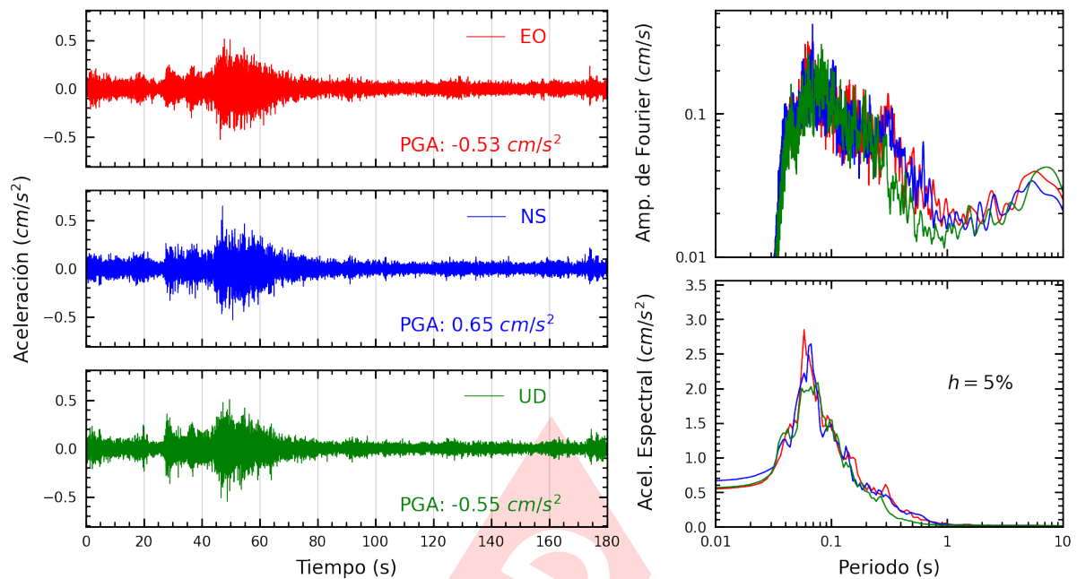
Figura A.25: Registros tiempo-historia, espectros de Fourier y de respuesta en las direcciones EO, NS y vertical de la estación MADRE. Sismo de San Vicente De Cañete, Cañete - Lima del 2024-06-18, 19:48:13 (Hora local)
