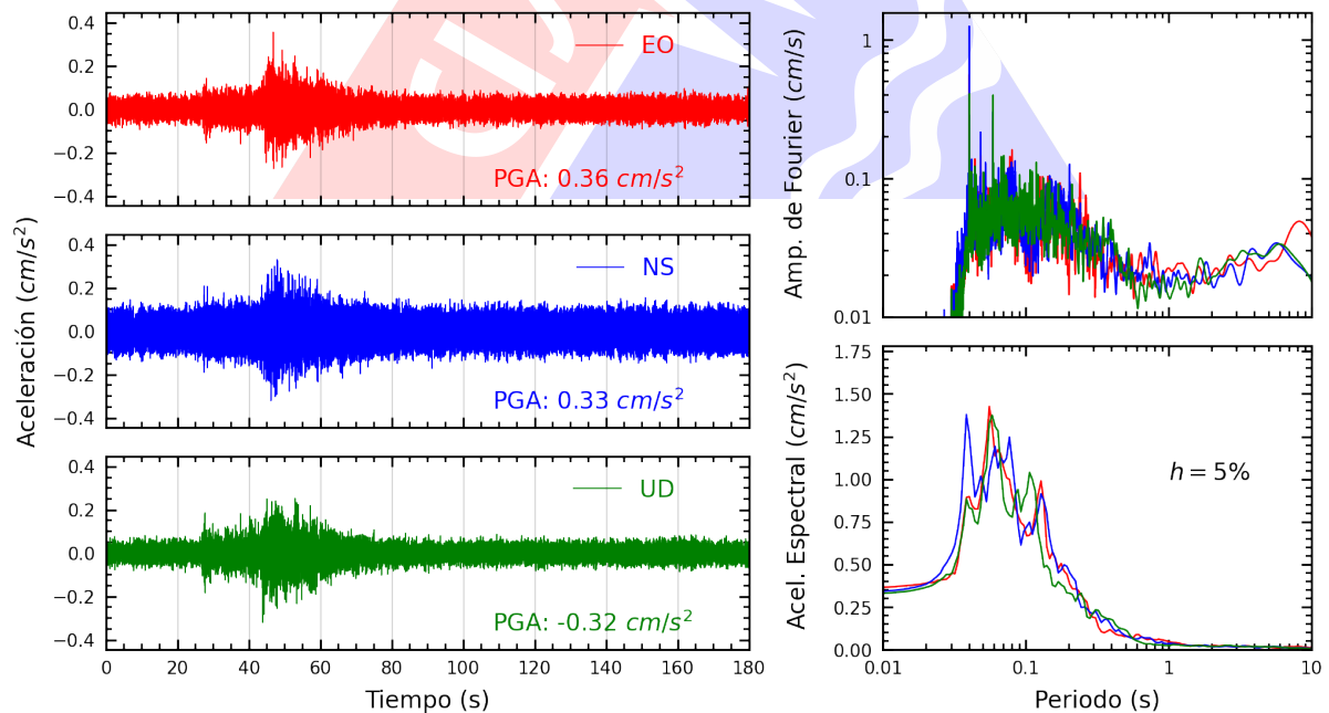
Figura A.34: Registros tiempo-historia, espectros de Fourier y de respuesta en las direcciones EO, NS y vertical de la estación BONDY. Sismo de San Vicente De Cañete, Cañete - Lima del 2024-06-18, 19:48:13 (Hora local)
