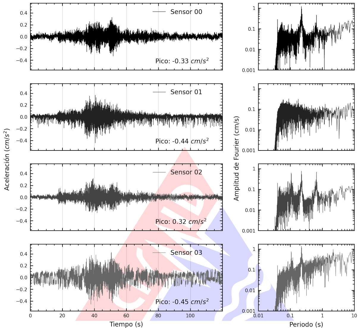
Figura A.1: Registros tiempo-historia y espectros de Fourier en la dirección EW de la edificación Centro de Información e Investigación de la FIC-UNI. Sismo de San Vicente De Cañete, Cañete - Lima del 2024-06-18, 19:48:13 (Hora local)
