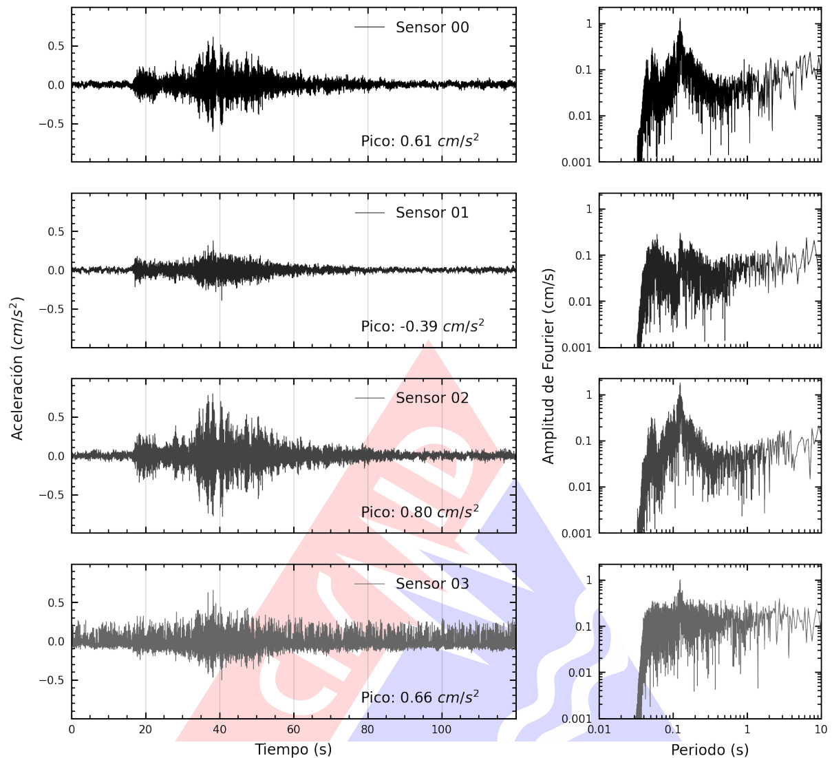
Figura A.3: Registros tiempo-historia y espectros de Fourier en la dirección vertical de la edificación Centro de Información e Investigación de la FIC-UNI. Sismo de San Vicente De Cañete, Cañete - Lima del 2024-06-18, 19:48:13 (Hora local)
