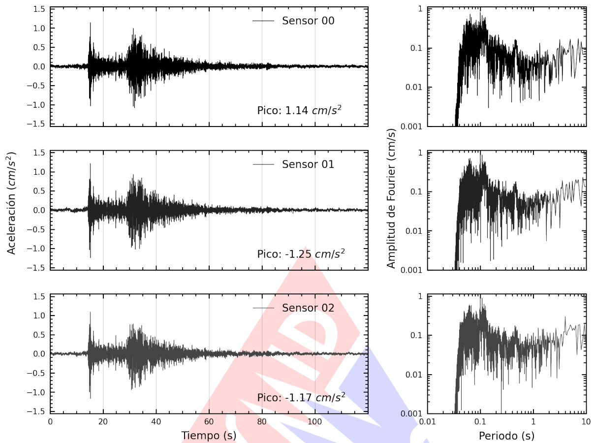
Figura A.3: Registros tiempo-historia y espectros de Fourier en la dirección vertical de la edificación Vivienda. Sismo de San Vicente De Cañete, Cañete - Lima del 2024-06-18, 19:48:13 (Hora local)
