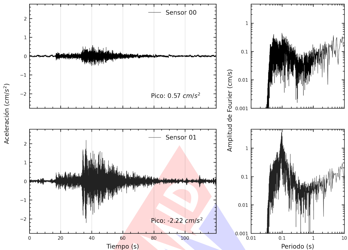
Figura A.1: Registros tiempo-historia y espectros de Fourier en la dirección EW de la edificación Laboratorio de Estructuras del CISMID-FIC-UNI. Sismo de San Vicente De Cañete, Cañete - Lima del 2024-06-18, 19:48:13 (Hora local)
