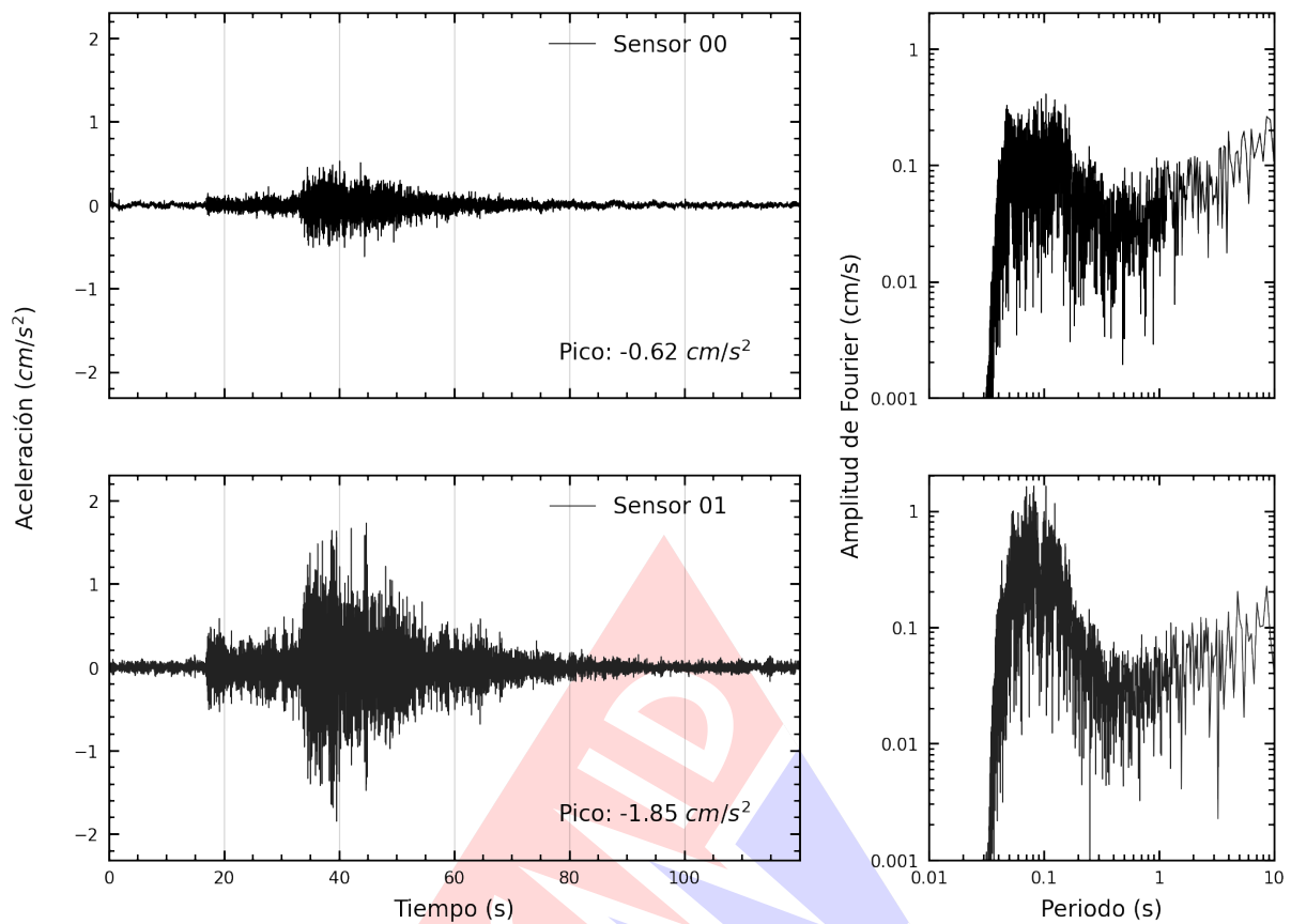
Figura A.2: Registros tiempo-historia y espectros de Fourier en la dirección NS de la edificación Laboratorio de Estructuras del CISMID-FIC-UNI. Sismo de San Vicente De Cañete, Cañete - Lima del 2024-06-18, 19:48:13 (Hora local)
