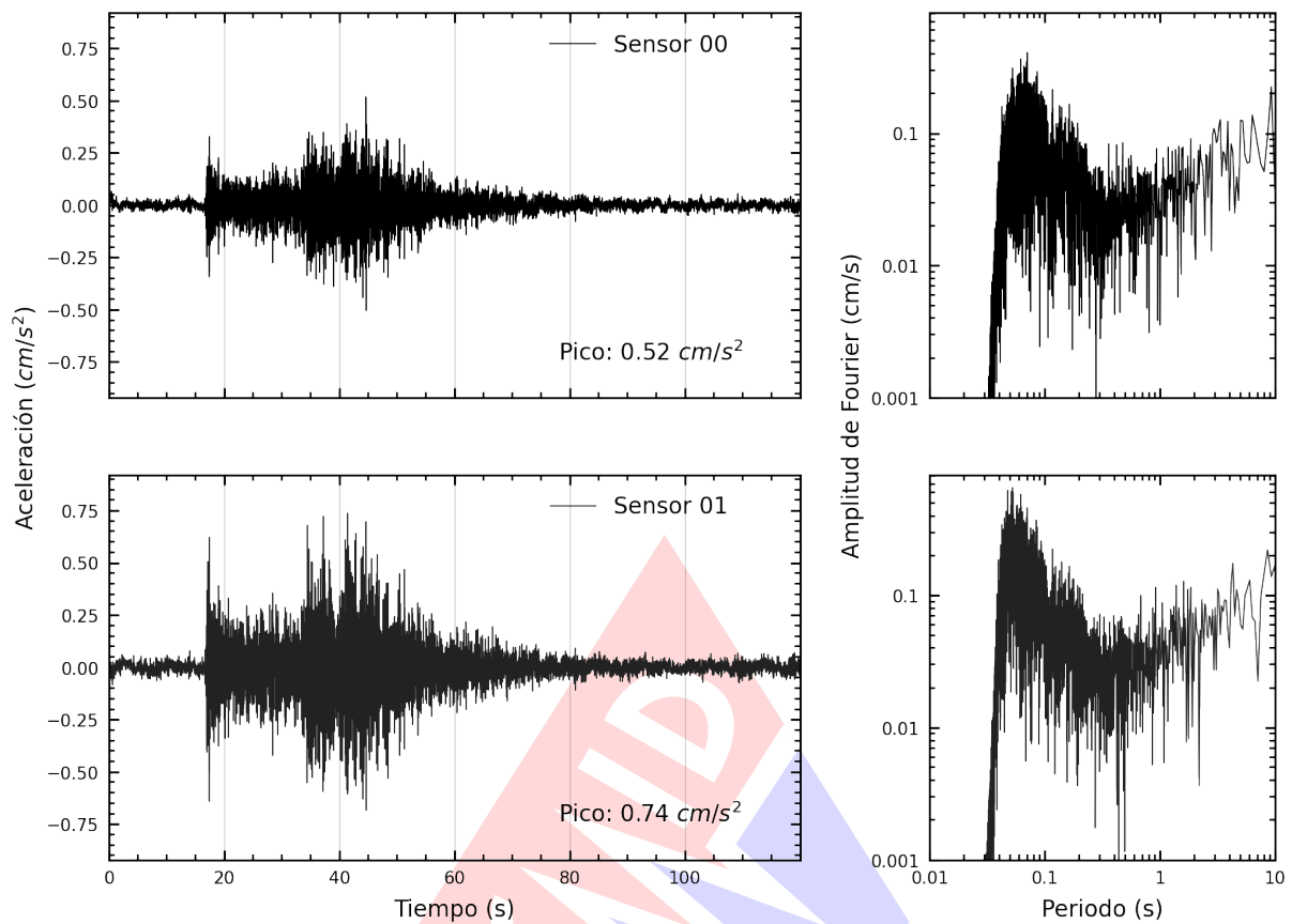
Figura A.3: Registros tiempo-historia y espectros de Fourier en la dirección vertical de la edificación Laboratorio de Estructuras del CISMID-FIC-UNI. Sismo de San Vicente De Cañete, Cañete - Lima del 2024-06-18, 19:48:13 (Hora local)
