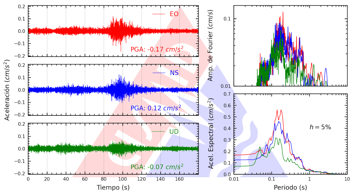
Figura A.9: Registros tiempo-historia, espectros de Fourier y de respuesta en las direcciones EO, NS y vertical de la estación JALV2. Sismo de Yauca, Caraveli - Arequipa del 2024-06-22, 15:46:43 (Hora local)
