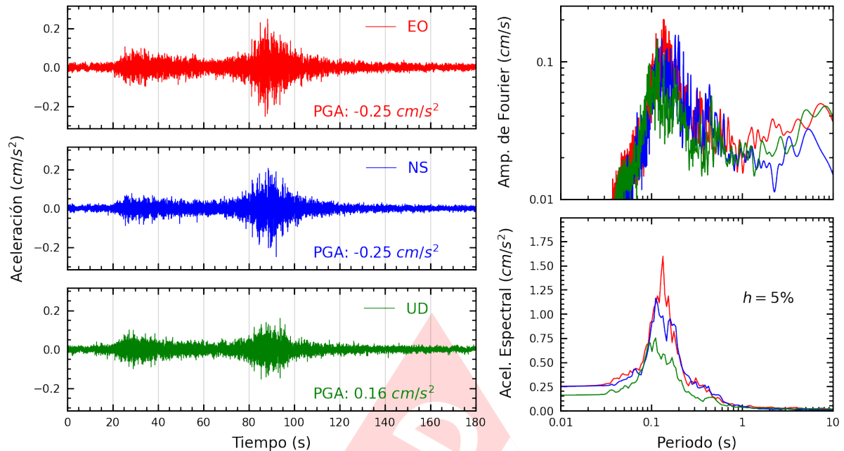
Figura A.7: Registros tiempo-historia, espectros de Fourier y de respuesta en las direcciones EO, NS y vertical de la estación AMORE. Sismo de Yauca, Caraveli - Arequipa del 2024-06-22, 15:46:43 (Hora local)
