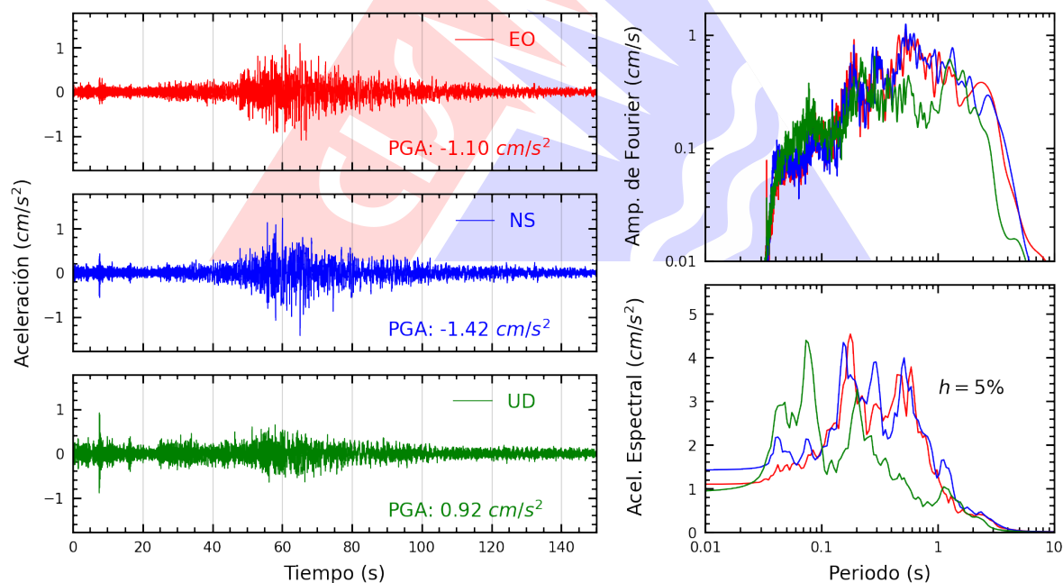
Figura A.2: Registros tiempo-historia, espectros de Fourier y de respuesta en las direcciones EO, NS y vertical de la estación SCICA. Sismo de Yauca, Caraveli - Arequipa del 2024-06-22, 15:46:43 (Hora local)
