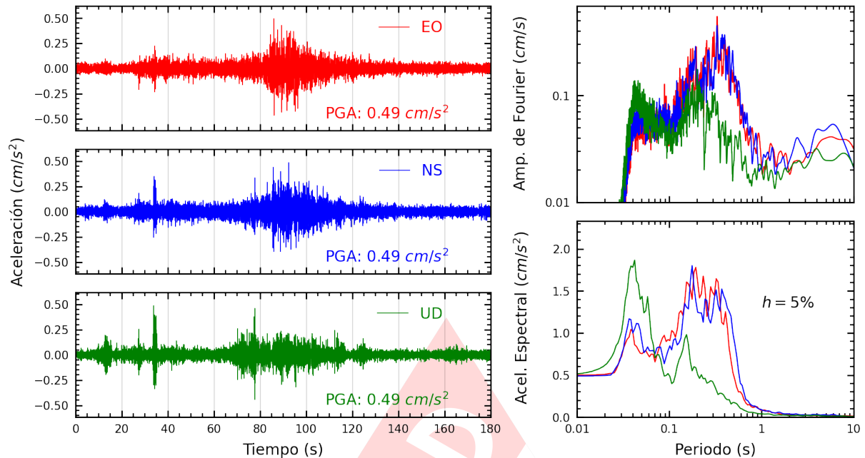
Figura A.3: Registros tiempo-historia, espectros de Fourier y de respuesta en las direcciones EO, NS y vertical de la estación DEFEN. Sismo de Yauca, Caraveli - Arequipa del 2024-06-22, 15:46:43 (Hora local)
