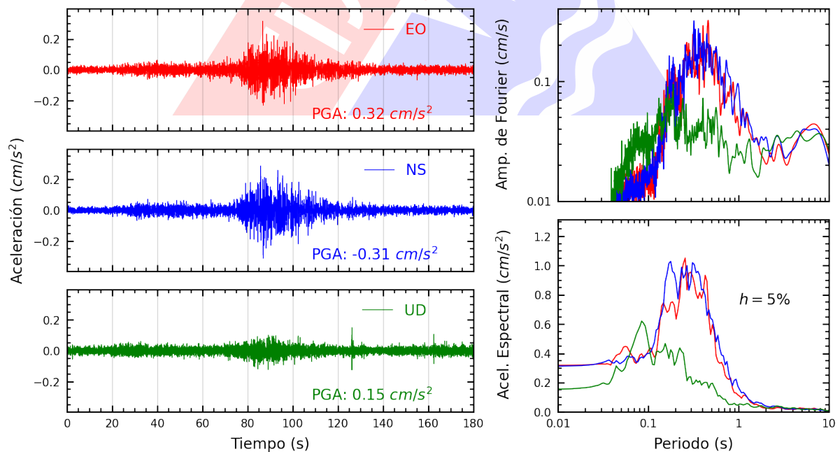
Figura A.4: Registros tiempo-historia, espectros de Fourier y de respuesta en las direcciones EO, NS y vertical de la estación ACAPU. Sismo de Yauca, Caraveli - Arequipa del 2024-06-22, 15:46:43 (Hora local)
