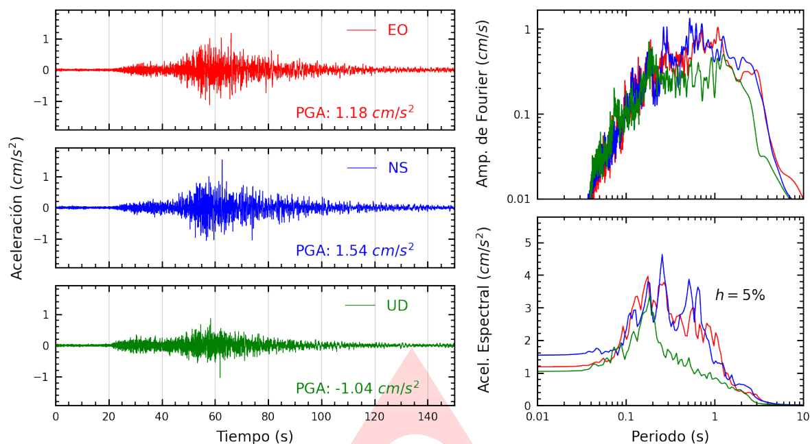
Figura A.1: Registros tiempo-historia, espectros de Fourier y de respuesta en las direcciones EO, NS y vertical de la estación UNICA. Sismo de Yauca, Caraveli - Arequipa del 2024-06-22, 15:46:43 (Hora local)
