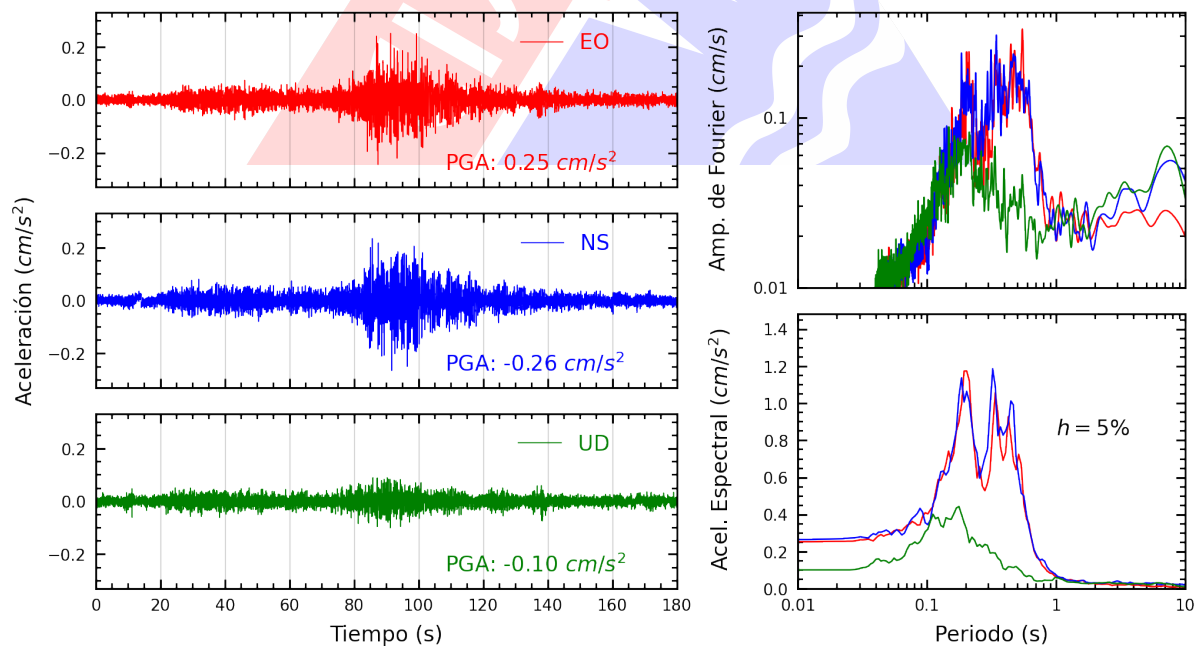
Figura A.6: Registros tiempo-historia, espectros de Fourier y de respuesta en las direcciones EO, NS y vertical de la estación VHAYA. Sismo de Yauca, Caraveli - Arequipa del 2024-06-22, 15:46:43 (Hora local)
