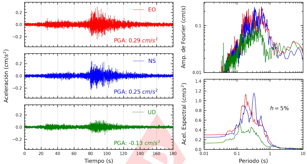
Figura A.5: Registros tiempo-historia, espectros de Fourier y de respuesta en las direcciones EO, NS y vertical de la estación USILP. Sismo de Yauca, Caraveli - Arequipa del 2024-06-22, 15:46:43 (Hora local)
