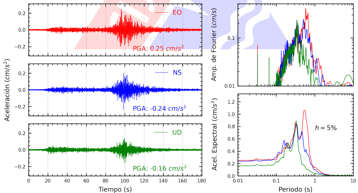
Figura A.8: Registros tiempo-historia, espectros de Fourier y de respuesta en las direcciones EO, NS y vertical de la estación CARAL. Sismo de Yauca, Caraveli - Arequipa del 2024-06-22, 15:46:43 (Hora local)
