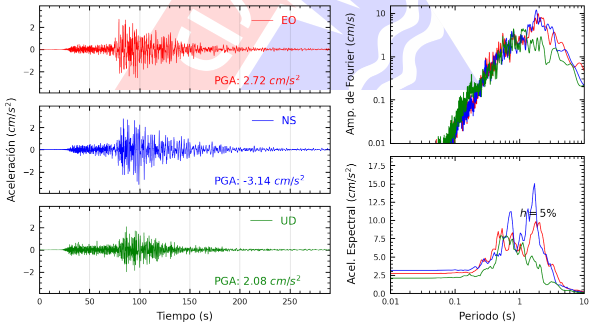
Figura A.34: Registros tiempo-historia, espectros de Fourier y de respuesta en las direcciones EO, NS y vertical de la estación UNCP. Sismo de Yauca, Caraveli - Arequipa del 2024-06-28, 00:36:27 (Hora local)
