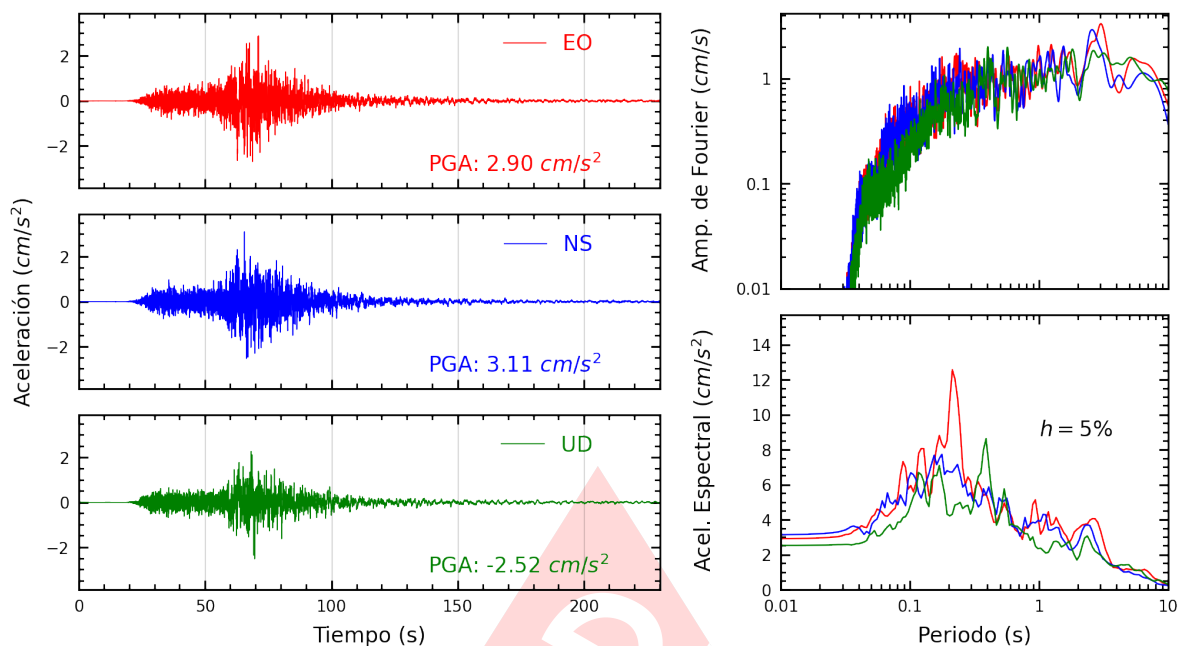
Figura A.35: Registros tiempo-historia, espectros de Fourier y de respuesta en las direcciones EO, NS y vertical de la estación UNSA. Sismo de Yauca, Caraveli - Arequipa del 2024-06-28, 00:36:27 (Hora local)
