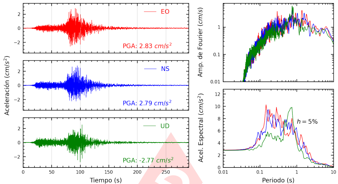
Figura A.37: Registros tiempo-historia, espectros de Fourier y de respuesta en las direcciones EO, NS y vertical de la estación CENEP. Sismo de Yauca, Caraveli - Arequipa del 2024-06-28, 00:36:27 (Hora local)
