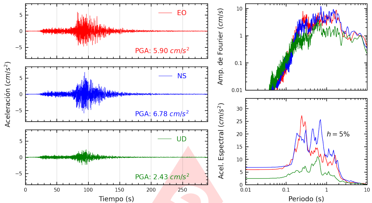
Figura A.15: Registros tiempo-historia, espectros de Fourier y de respuesta en las direcciones EO, NS y vertical de la estación DDMI. Sismo de Yauca, Caraveli - Arequipa del 2024-06-28, 00:36:27 (Hora local)
