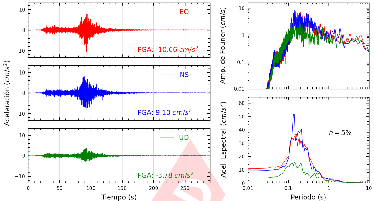
Figura A.5: Registros tiempo-historia, espectros de Fourier y de respuesta en las direcciones EO, NS y vertical de la estación CARAB. Sismo de Yauca, Caraveli - Arequipa del 2024-06-28, 00:36:27 (Hora local)
