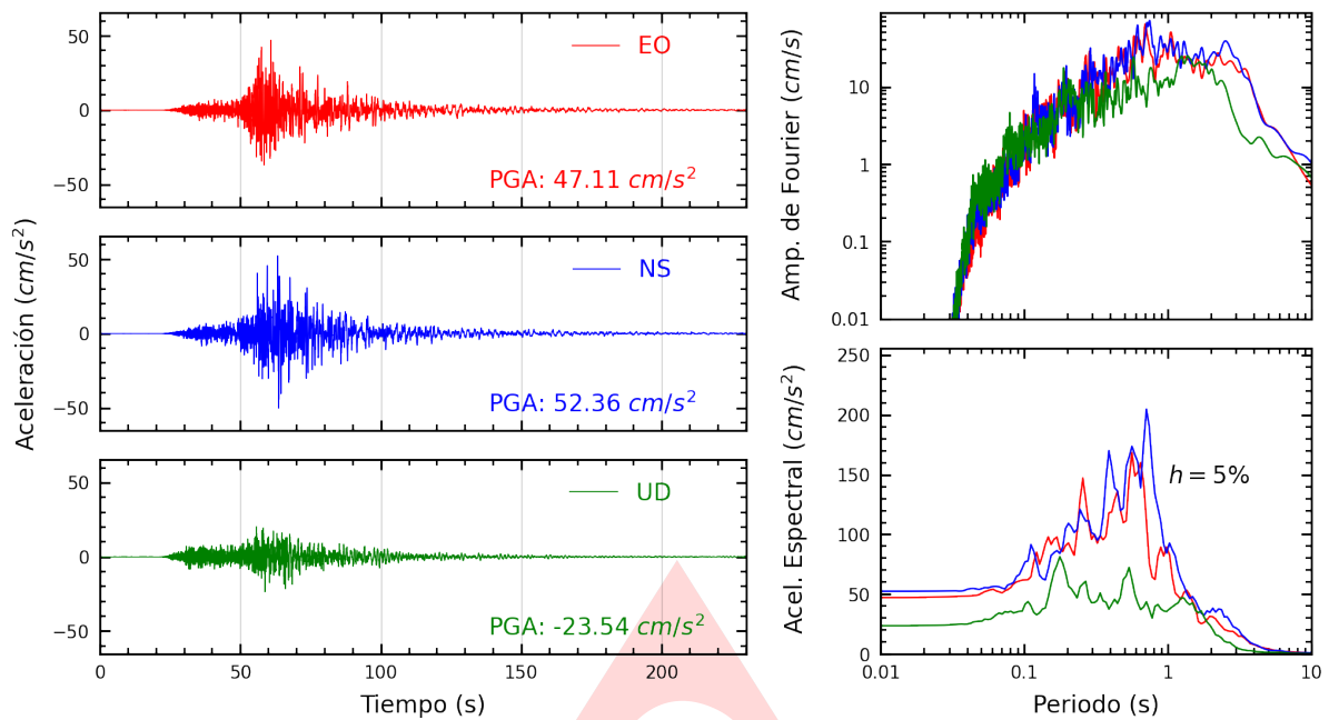
Figura A.1: Registros tiempo-historia, espectros de Fourier y de respuesta en las direcciones EO, NS y vertical de la estación UNICA. Sismo de Yauca, Caraveli - Arequipa del 2024-06-28, 00:36:27 (Hora local)
