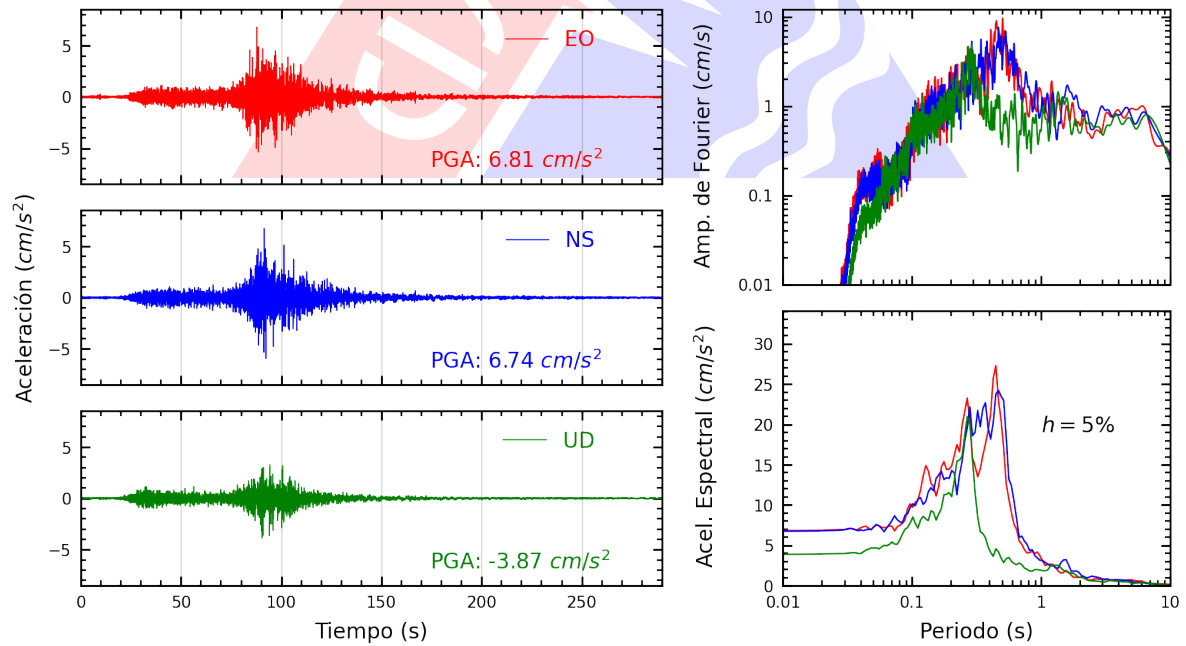
Figura A.14: Registros tiempo-historia, espectros de Fourier y de respuesta en las direcciones EO, NS y vertical de la estación OLIVO. Sismo de Yauca, Caraveli - Arequipa del 2024-06-28, 00:36:27 (Hora local)
