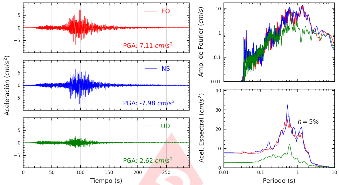
Figura A.13: Registros tiempo-historia, espectros de Fourier y de respuesta en las direcciones EO, NS y vertical de la estación DHN2. Sismo de Yauca, Caraveli - Arequipa del 2024-06-28, 00:36:27 (Hora local)
