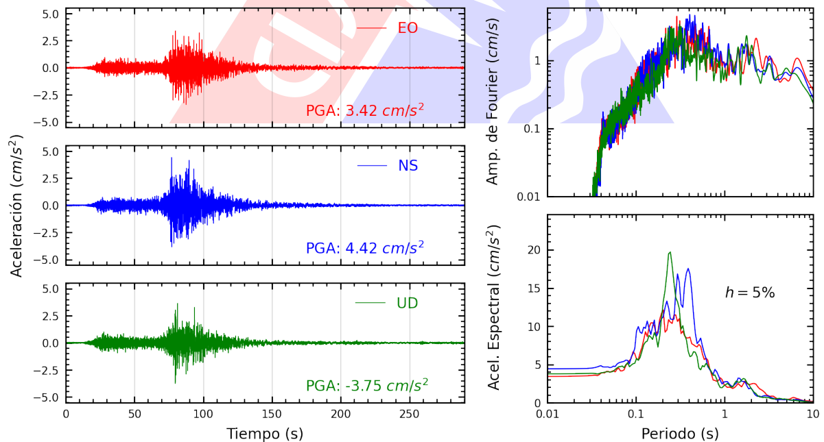
Figura A.24: Registros tiempo-historia, espectros de Fourier y de respuesta en las direcciones EO, NS y vertical de la estación URPPE. Sismo de Yauca, Caraveli - Arequipa del 2024-06-28, 00:36:27 (Hora local)
