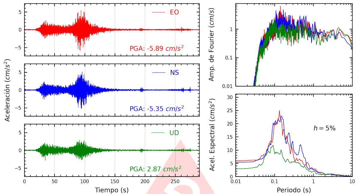
Figura A.17: Registros tiempo-historia, espectros de Fourier y de respuesta en las direcciones EO, NS y vertical de la estación SROSA. Sismo de Yauca, Caraveli - Arequipa del 2024-06-28, 00:36:27 (Hora local)
