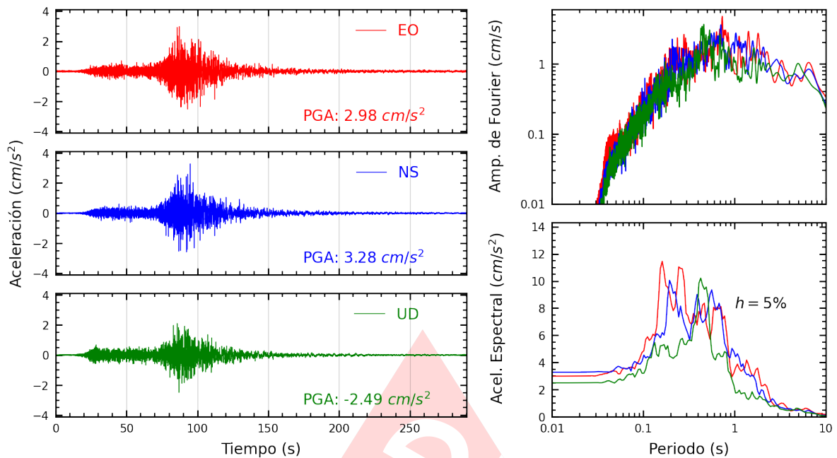
Figura A.33: Registros tiempo-historia, espectros de Fourier y de respuesta en las direcciones EO, NS y vertical de la estación INICT. Sismo de Yauca, Caraveli - Arequipa del 2024-06-28, 00:36:27 (Hora local)
