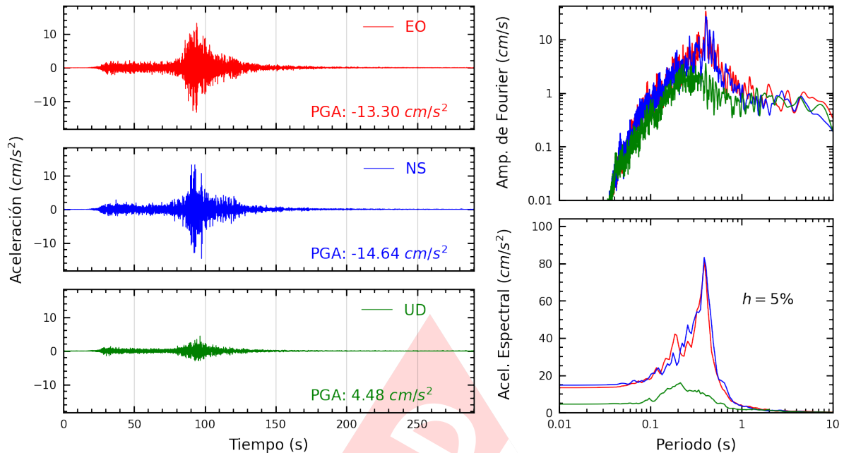
Figura A.3: Registros tiempo-historia, espectros de Fourier y de respuesta en las direcciones EO, NS y vertical de la estación DEFEN. Sismo de Yauca, Caraveli - Arequipa del 2024-06-28, 00:36:27 (Hora local)
