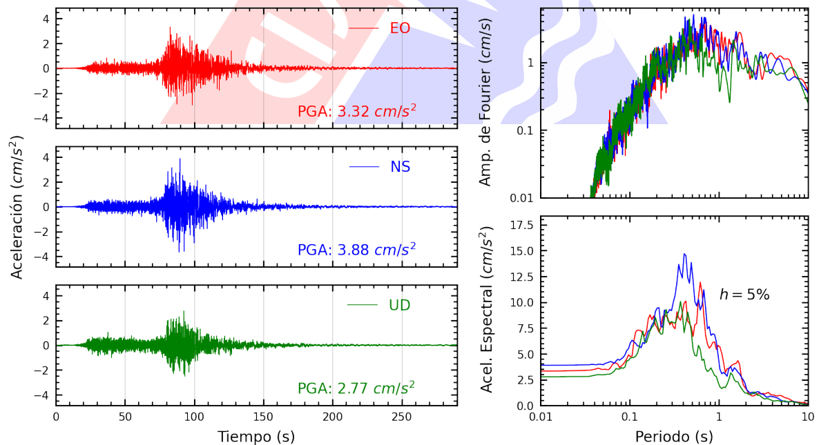
Figura A.28: Registros tiempo-historia, espectros de Fourier y de respuesta en las direcciones EO, NS y vertical de la estación UNFV. Sismo de Yauca, Caraveli - Arequipa del 2024-06-28, 00:36:27 (Hora local)
