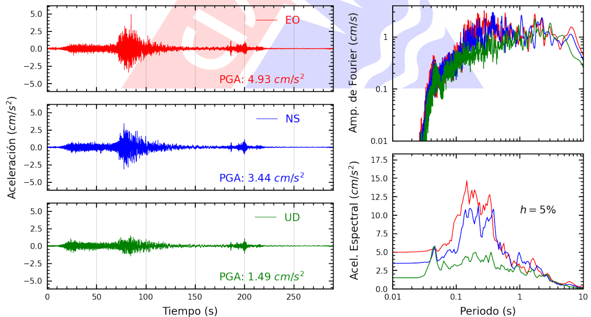
Figura A.20: Registros tiempo-historia, espectros de Fourier y de respuesta en las direcciones EO, NS y vertical de la estación PACHA. Sismo de Yauca, Caraveli - Arequipa del 2024-06-28, 00:36:27 (Hora local)
