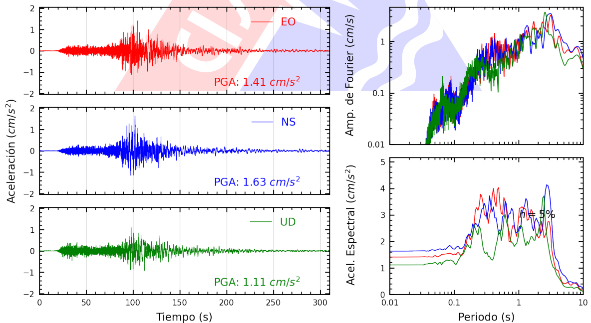
Figura A.42: Registros tiempo-historia, espectros de Fourier y de respuesta en las direcciones EO, NS y vertical de la estación CREY. Sismo de Yauca, Caraveli - Arequipa del 2024-06-28, 00:36:27 (Hora local)
