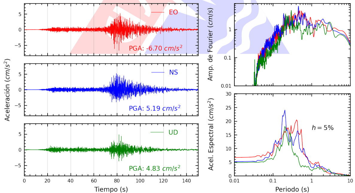
Figura A.16: Registros tiempo-historia, espectros de Fourier y de respuesta en las direcciones EO, NS y vertical de la estación UPCVI. Sismo de Yauca, Caraveli - Arequipa del 2024-06-28, 00:36:27 (Hora local)
