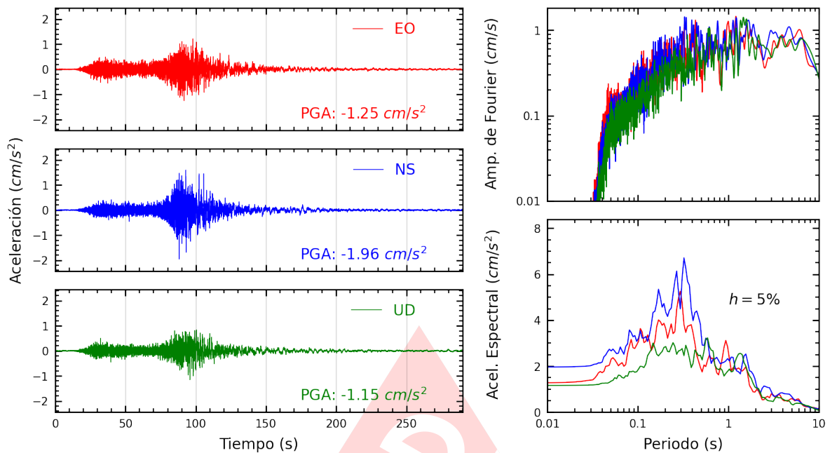
Figura A.41: Registros tiempo-historia, espectros de Fourier y de respuesta en las direcciones EO, NS y vertical de la estación UCSS. Sismo de Yauca, Caraveli - Arequipa del 2024-06-28, 00:36:27 (Hora local)
