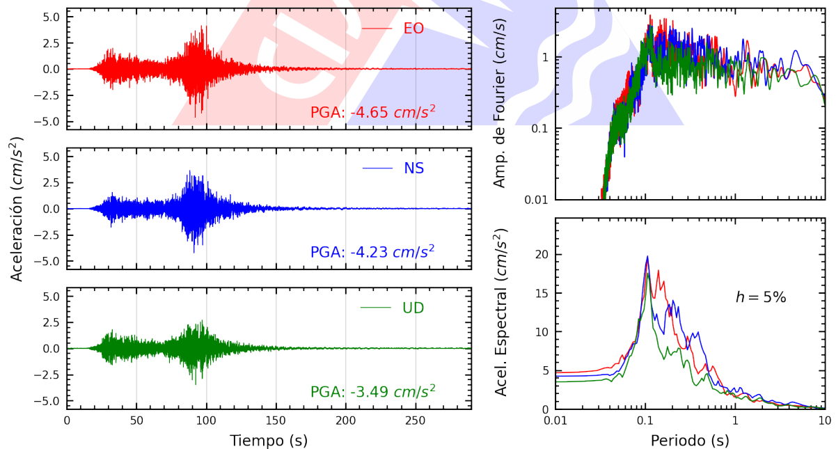
Figura A.22: Registros tiempo-historia, espectros de Fourier y de respuesta en las direcciones EO, NS y vertical de la estación AMORE. Sismo de Yauca, Caraveli - Arequipa del 2024-06-28, 00:36:27 (Hora local)
