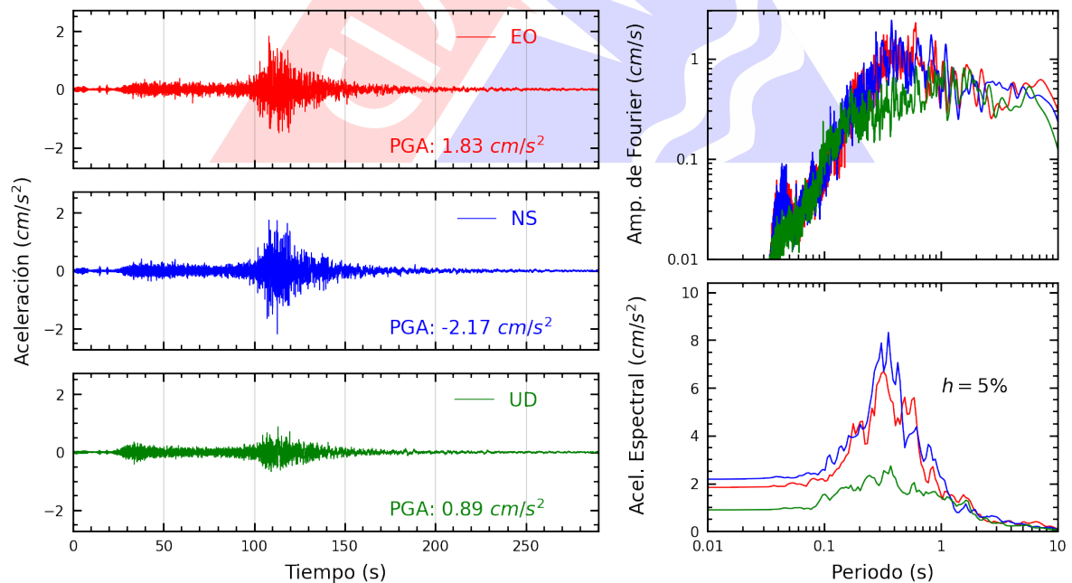
Figura A.40: Registros tiempo-historia, espectros de Fourier y de respuesta en las direcciones EO, NS y vertical de la estación UNAB. Sismo de Yauca, Caraveli - Arequipa del 2024-06-28, 00:36:27 (Hora local)
