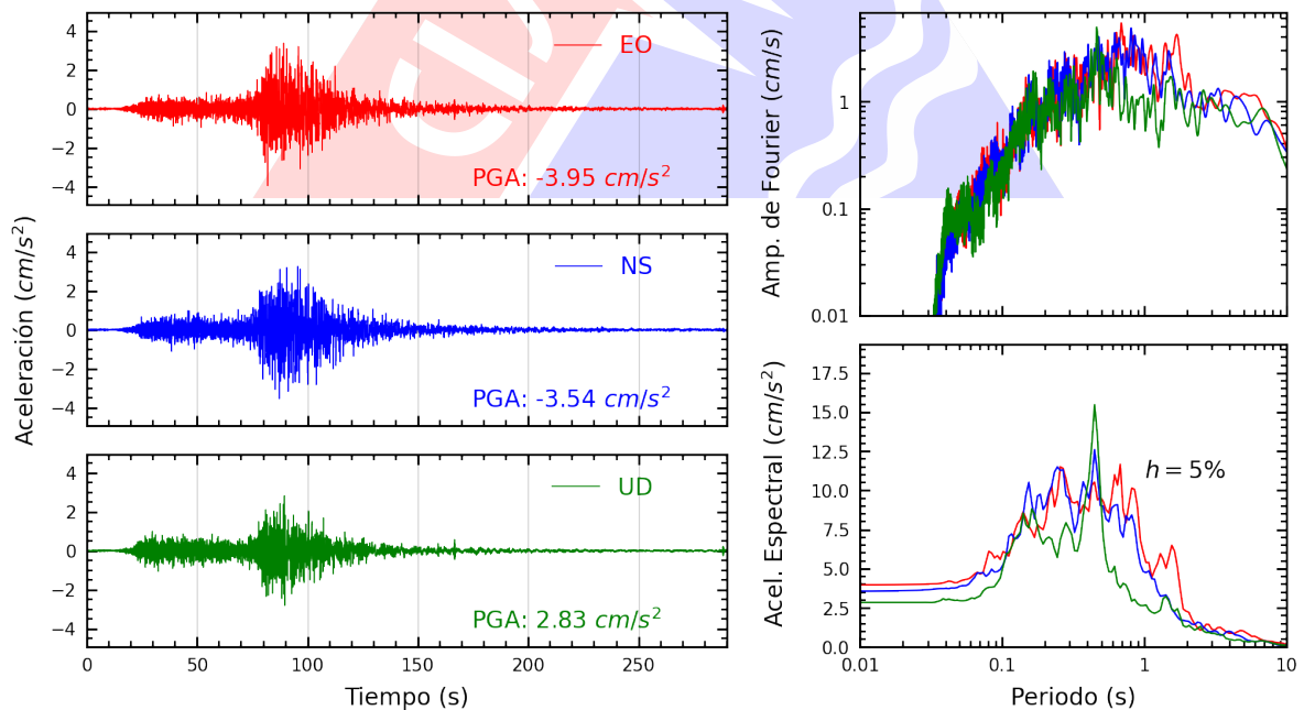
Figura A.26: Registros tiempo-historia, espectros de Fourier y de respuesta en las direcciones EO, NS y vertical de la estación UPCSM. Sismo de Yauca, Caraveli - Arequipa del 2024-06-28, 00:36:27 (Hora local)
