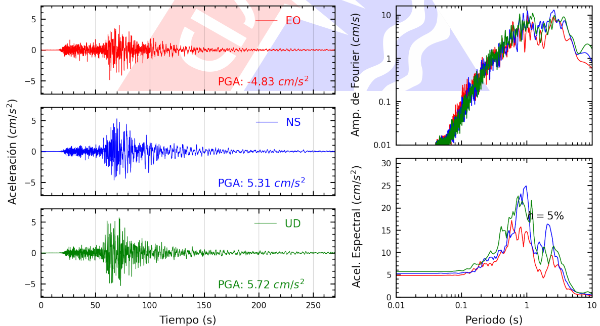
Figura A.18: Registros tiempo-historia, espectros de Fourier y de respuesta en las direcciones EO, NS y vertical de la estación UNSCH. Sismo de Yauca, Caraveli - Arequipa del 2024-06-28, 00:36:27 (Hora local)
