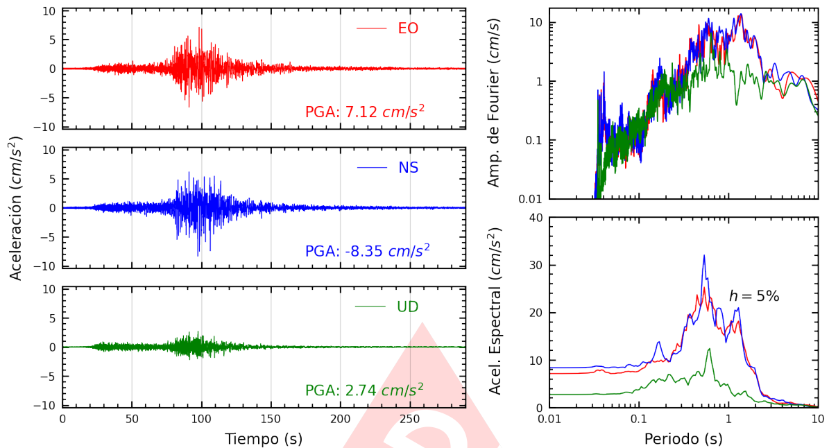
Figura A.11: Registros tiempo-historia, espectros de Fourier y de respuesta en las direcciones EO, NS y vertical de la estación DHNPE. Sismo de Yauca, Caraveli - Arequipa del 2024-06-28, 00:36:27 (Hora local)
