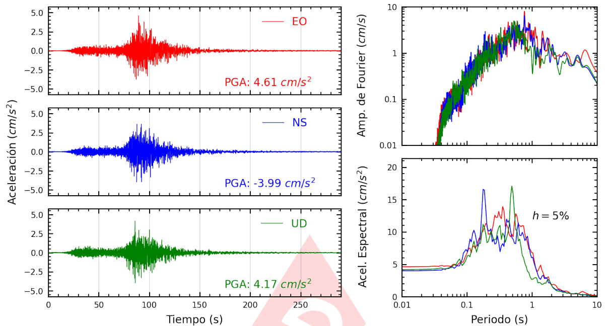
Figura A.23: Registros tiempo-historia, espectros de Fourier y de respuesta en las direcciones EO, NS y vertical de la estación IMCA. Sismo de Yauca, Caraveli - Arequipa del 2024-06-28, 00:36:27 (Hora local)
