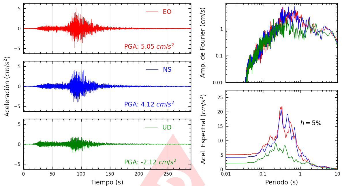
Figura A.19: Registros tiempo-historia, espectros de Fourier y de respuesta en las direcciones EO, NS y vertical de la estación MADRE. Sismo de Yauca, Caraveli - Arequipa del 2024-06-28, 00:36:27 (Hora local)
