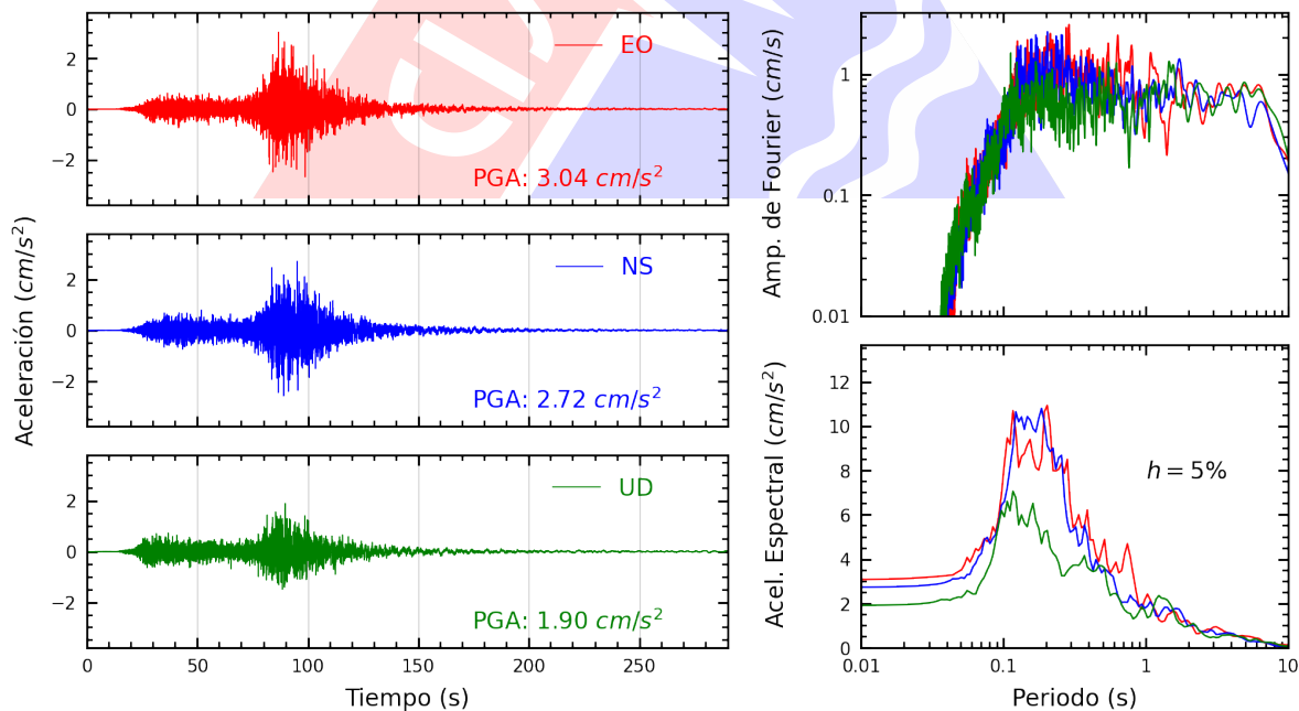
Figura A.36: Registros tiempo-historia, espectros de Fourier y de respuesta en las direcciones EO, NS y vertical de la estación JALV2. Sismo de Yauca, Caraveli - Arequipa del 2024-06-28, 00:36:27 (Hora local)
