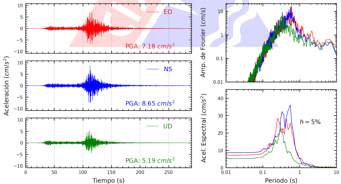
Figura A.8: Registros tiempo-historia, espectros de Fourier y de respuesta en las direcciones EO, NS y vertical de la estación CARAL. Sismo de Yauca, Caraveli - Arequipa del 2024-06-28, 00:36:27 (Hora local)
