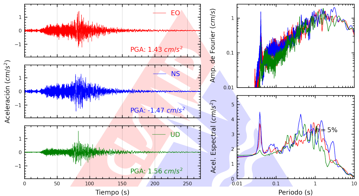
Figura A.43: Registros tiempo-historia, espectros de Fourier y de respuesta en las direcciones EO, NS y vertical de la estación UNAM. Sismo de Yauca, Caraveli - Arequipa del 2024-06-28, 00:36:27 (Hora local)
