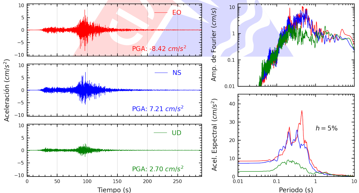
Figura A.10: Registros tiempo-historia, espectros de Fourier y de respuesta en las direcciones EO, NS y vertical de la estación VHAYA. Sismo de Yauca, Caraveli - Arequipa del 2024-06-28, 00:36:27 (Hora local)
