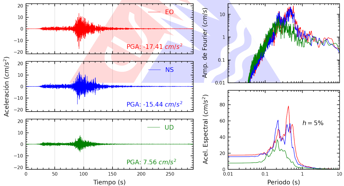
Figura A.2: Registros tiempo-historia, espectros de Fourier y de respuesta en las direcciones EO, NS y vertical de la estación MDPP. Sismo de Yauca, Caraveli - Arequipa del 2024-06-28, 00:36:27 (Hora local)
