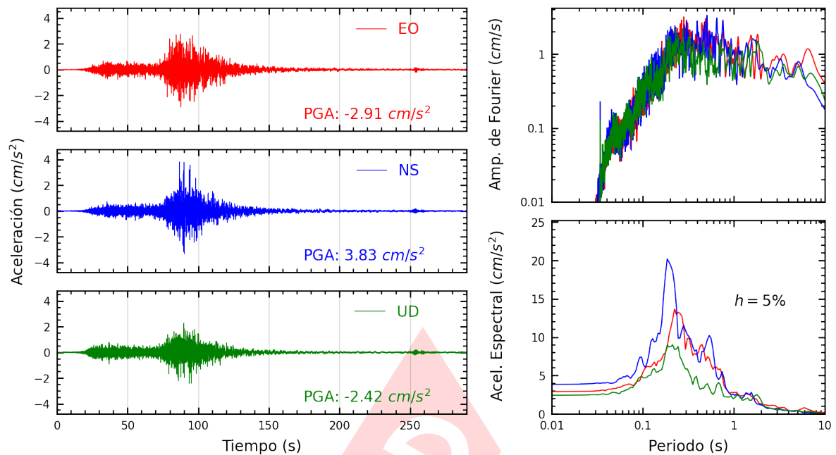
Figura A.29: Registros tiempo-historia, espectros de Fourier y de respuesta en las direcciones EO, NS y vertical de la estación USMP. Sismo de Yauca, Caraveli - Arequipa del 2024-06-28, 00:36:27 (Hora local)
