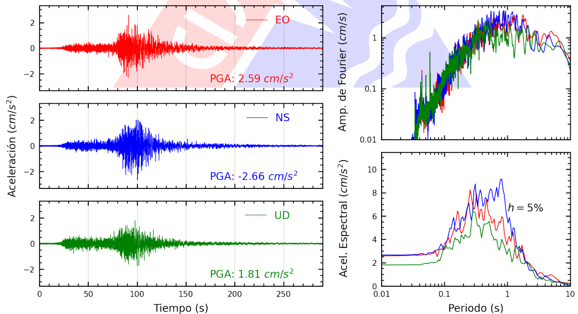
Figura A.38: Registros tiempo-historia, espectros de Fourier y de respuesta en las direcciones EO, NS y vertical de la estación BONDY. Sismo de Yauca, Caraveli - Arequipa del 2024-06-28, 00:36:27 (Hora local)
