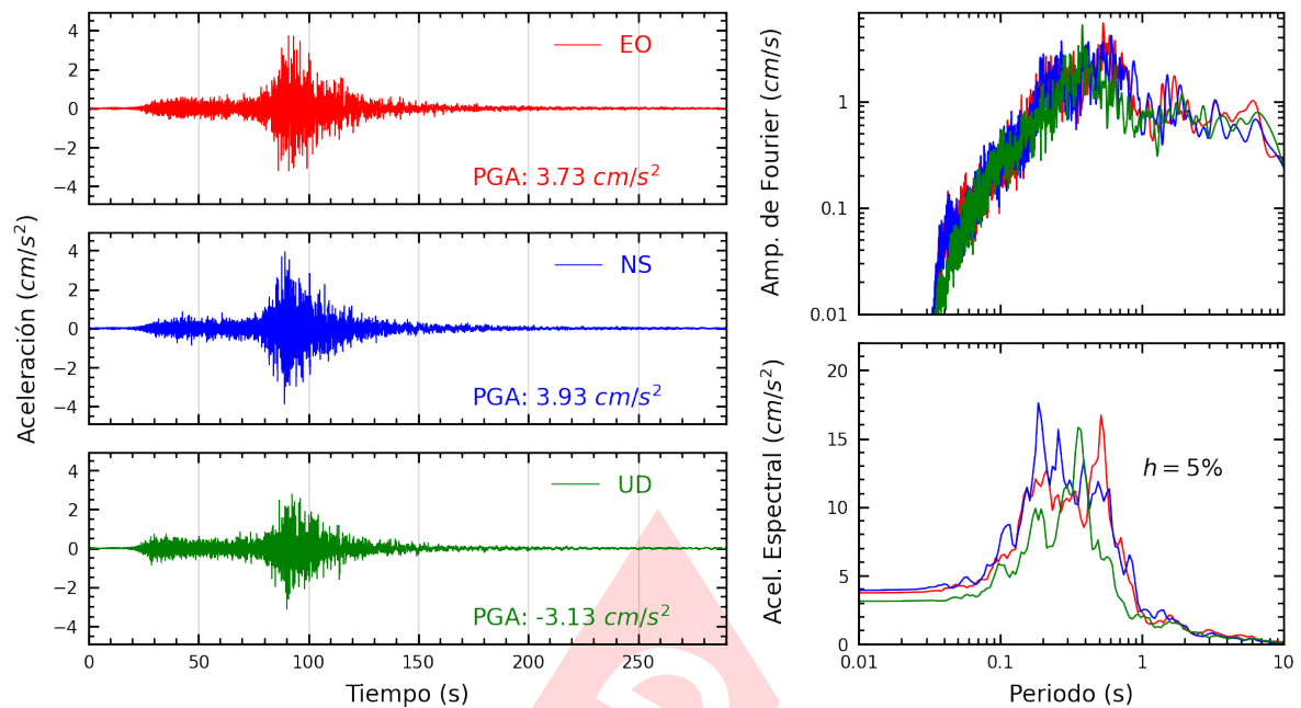
Figura A.27: Registros tiempo-historia, espectros de Fourier y de respuesta en las direcciones EO, NS y vertical de la estación COMAS. Sismo de Yauca, Caraveli - Arequipa del 2024-06-28, 00:36:27 (Hora local)
