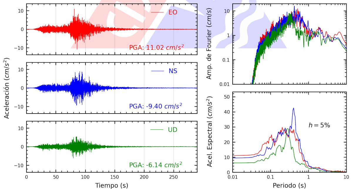
Figura A.4: Registros tiempo-historia, espectros de Fourier y de respuesta en las direcciones EO, NS y vertical de la estación UNTEL. Sismo de Yauca, Caraveli - Arequipa del 2024-06-28, 00:36:27 (Hora local)
