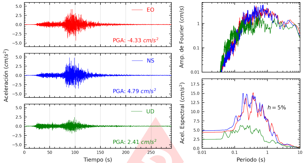
Figura A.21: Registros tiempo-historia, espectros de Fourier y de respuesta en las direcciones EO, NS y vertical de la estación RAMON. Sismo de Yauca, Caraveli - Arequipa del 2024-06-28, 00:36:27 (Hora local)
