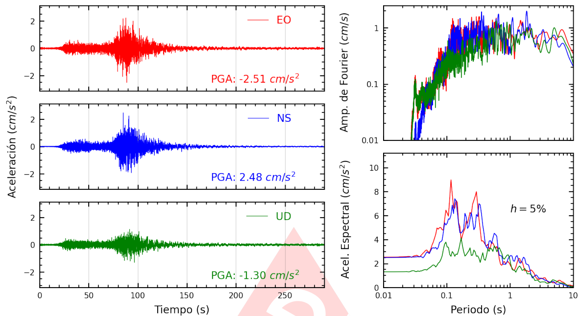
Figura A.39: Registros tiempo-historia, espectros de Fourier y de respuesta en las direcciones EO, NS y vertical de la estación ATARJ. Sismo de Yauca, Caraveli - Arequipa del 2024-06-28, 00:36:27 (Hora local)
