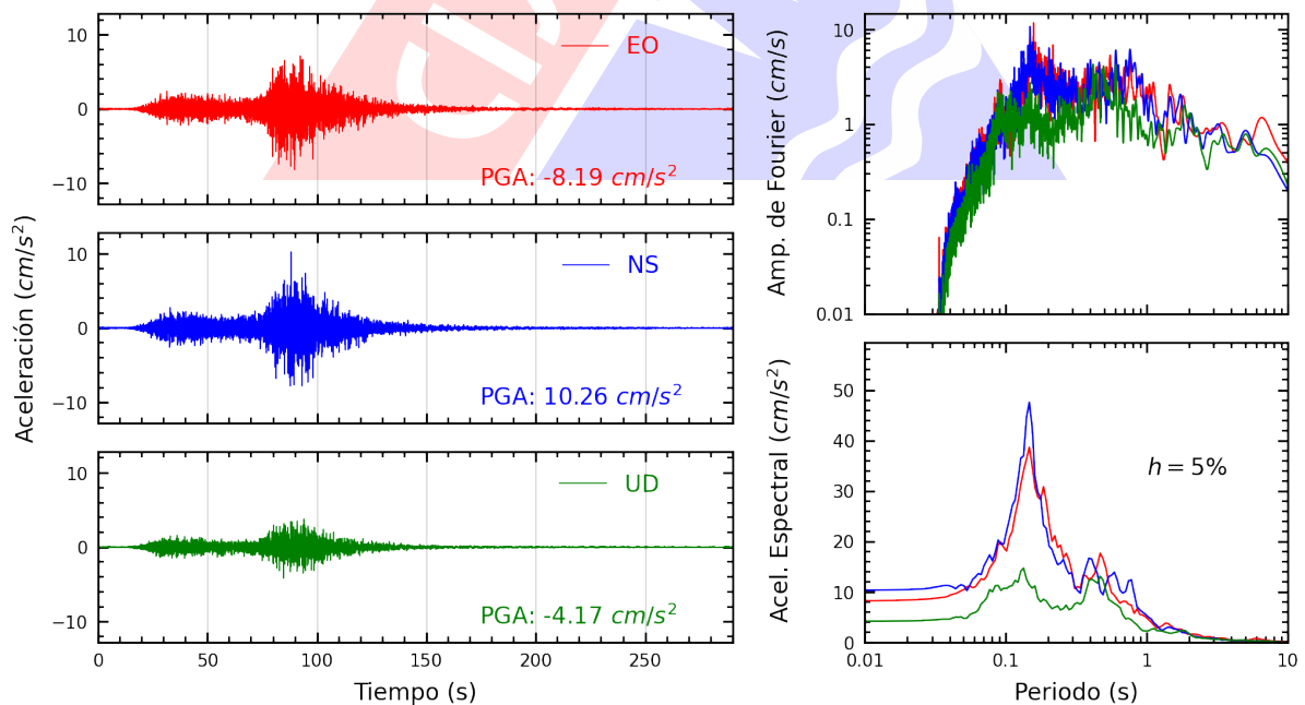
Figura A.6: Registros tiempo-historia, espectros de Fourier y de respuesta en las direcciones EO, NS y vertical de la estación USILM. Sismo de Yauca, Caraveli - Arequipa del 2024-06-28, 00:36:27 (Hora local)
