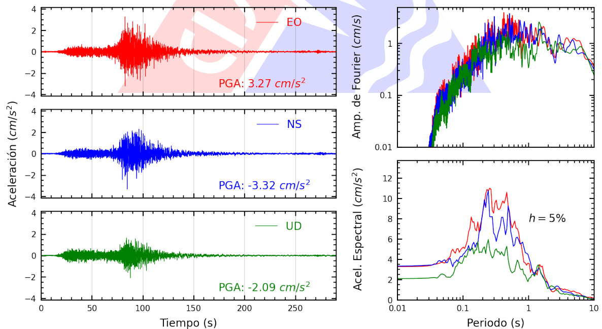
Figura A.32: Registros tiempo-historia, espectros de Fourier y de respuesta en las direcciones EO, NS y vertical de la estación CEPRE. Sismo de Yauca, Caraveli - Arequipa del 2024-06-28, 00:36:27 (Hora local)
