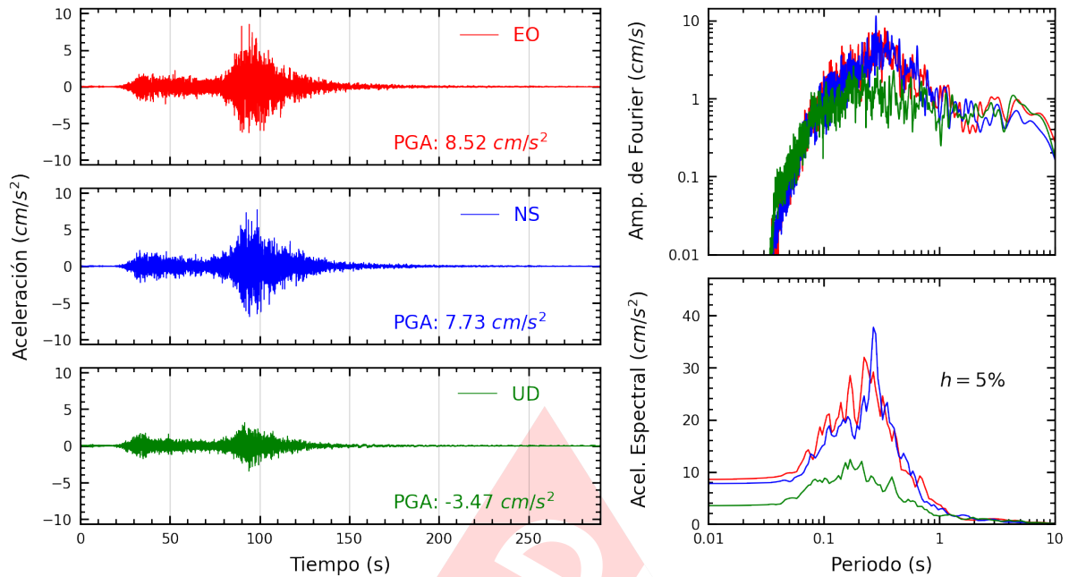
Figura A.9: Registros tiempo-historia, espectros de Fourier y de respuesta en las direcciones EO, NS y vertical de la estación ANCON. Sismo de Yauca, Caraveli - Arequipa del 2024-06-28, 00:36:27 (Hora local)
