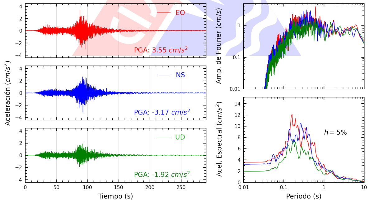
Figura A.30: Registros tiempo-historia, espectros de Fourier y de respuesta en las direcciones EO, NS y vertical de la estación FICPE. Sismo de Yauca, Caraveli - Arequipa del 2024-06-28, 00:36:27 (Hora local)
