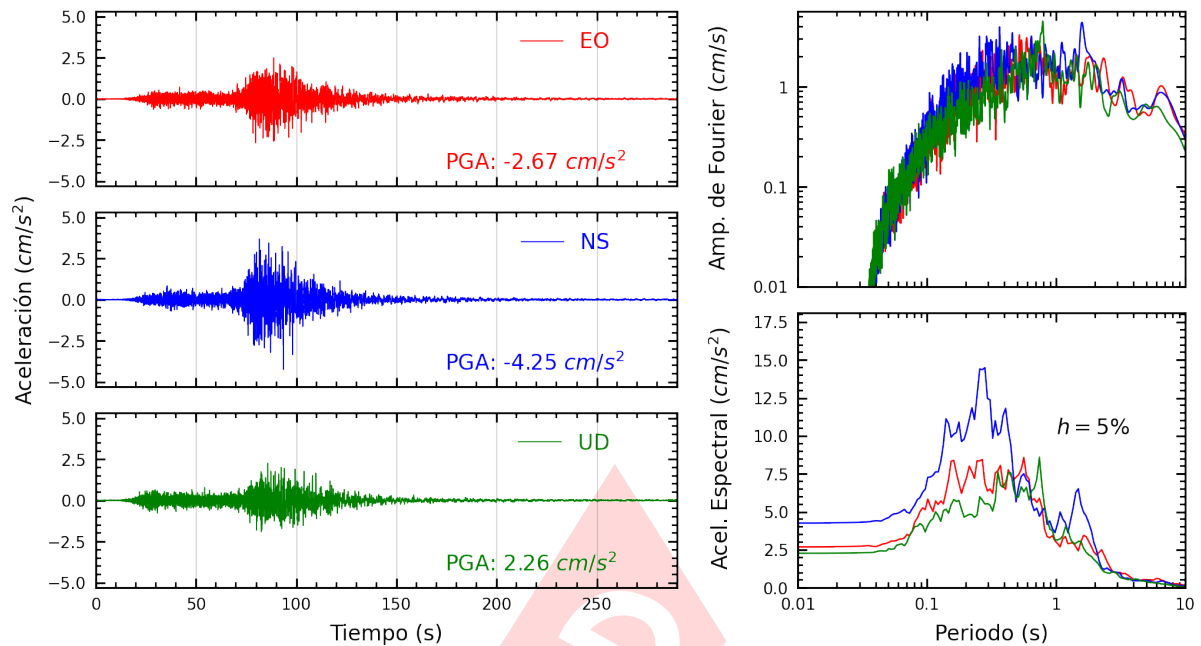
Figura A.25: Registros tiempo-historia, espectros de Fourier y de respuesta en las direcciones EO, NS y vertical de la estación SERVI. Sismo de Yauca, Caraveli - Arequipa del 2024-06-28, 00:36:27 (Hora local)
