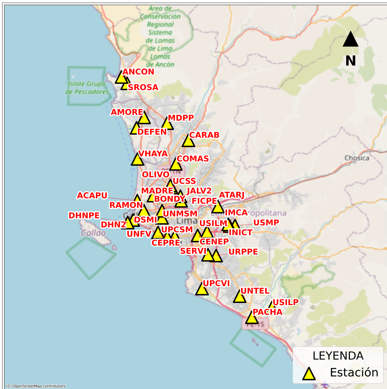
Figura 3: Mapa de ubicación de la(s) estación(es) acelerográfica(s) en Lima Metropolitana correspondiente(s) al Sismo de Yauca, Caraveli - Arequipa del 28 de junio de 2024 a las 00:36:27 (hora local)
