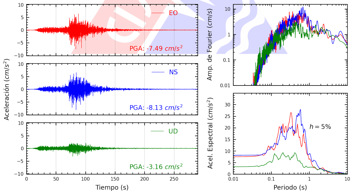
Figura A.12: Registros tiempo-historia, espectros de Fourier y de respuesta en las direcciones EO, NS y vertical de la estación USILP. Sismo de Yauca, Caraveli - Arequipa del 2024-06-28, 00:36:27 (Hora local)
