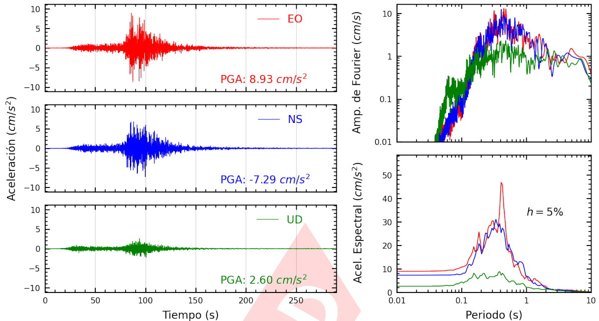
Figura A.7: Registros tiempo-historia, espectros de Fourier y de respuesta en las direcciones EO, NS y vertical de la estación ACAPU. Sismo de Yauca, Caraveli - Arequipa del 2024-06-28, 00:36:27 (Hora local)
