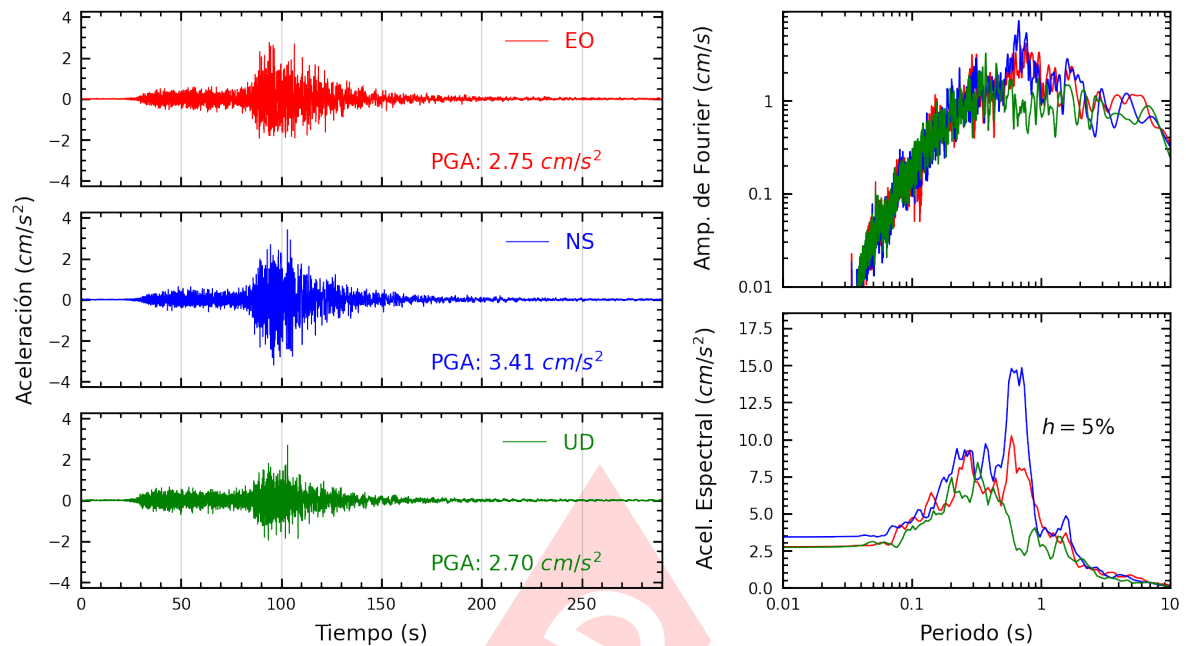
Figura A.31: Registros tiempo-historia, espectros de Fourier y de respuesta en las direcciones EO, NS y vertical de la estación UNMSM. Sismo de Yauca, Caraveli - Arequipa del 2024-06-28, 00:36:27 (Hora local)
