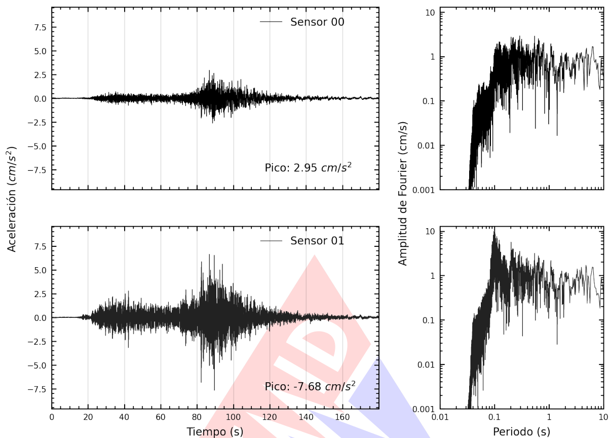
Figura A.1: Registros tiempo-historia y espectros de Fourier en la dirección EW de la edificación Laboratorio de Estructuras del CISMID-FIC-UNI. Sismo de Yauca, Caraveli - Arequipa del 2024-06-28, 00:36:27 (Hora local)
