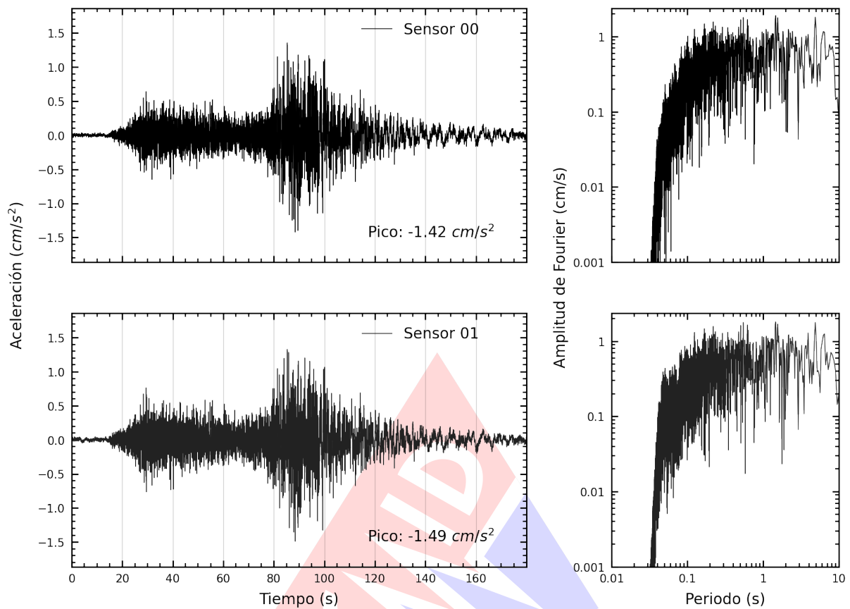
Figura A.3: Registros tiempo-historia y espectros de Fourier en la dirección vertical de la edificación Laboratorio de Estructuras del CISMID-FIC-UNI. Sismo de Yauca, Caraveli - Arequipa del 2024-06-28, 00:36:27 (Hora local)
