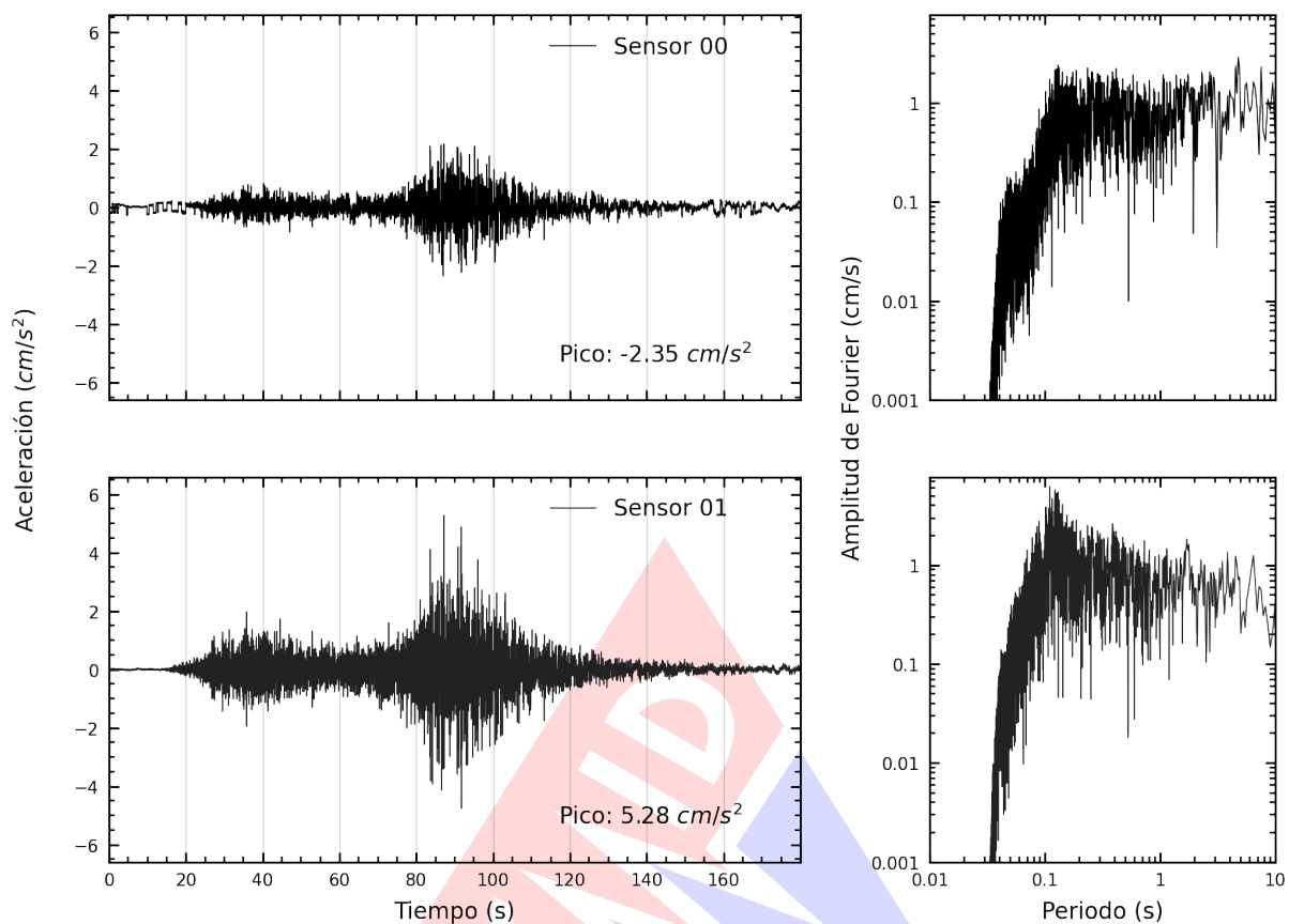
Figura A.2: Registros tiempo-historia y espectros de Fourier en la dirección NS de la edificación Laboratorio de Estructuras del CISMID-FIC-UNI. Sismo de Yauca, Caraveli - Arequipa del 2024-06-28, 00:36:27 (Hora local)
