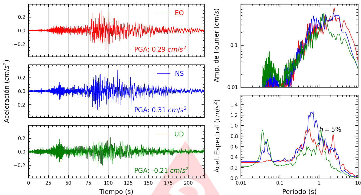
Figura A.49: Registros tiempo-historia, espectros de Fourier y de respuesta en las direcciones EO, NS y vertical de la estación SCHYO. Sismo de Chala, Caraveli - Arequipa del 2024-06-29, 02:05:31 (Hora local)
