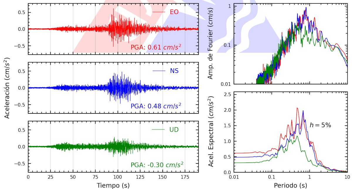
Figura A.30: Registros tiempo-historia, espectros de Fourier y de respuesta en las direcciones EO, NS y vertical de la estación UNFV. Sismo de Chala, Caraveli - Arequipa del 2024-06-29, 02:05:31 (Hora local)
