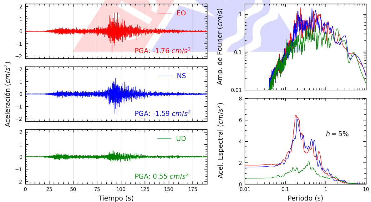
Figura A.8: Registros tiempo-historia, espectros de Fourier y de respuesta en las direcciones EO, NS y vertical de la estación SCCHO. Sismo de Chala, Caraveli - Arequipa del 2024-06-29, 02:05:31 (Hora local)
