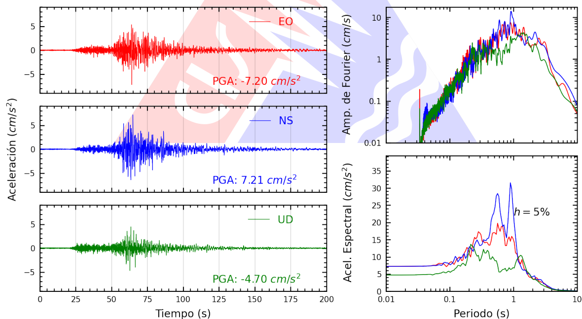
Figura A.2: Registros tiempo-historia, espectros de Fourier y de respuesta en las direcciones EO, NS y vertical de la estación SCICA. Sismo de Chala, Caraveli - Arequipa del 2024-06-29, 02:05:31 (Hora local)
