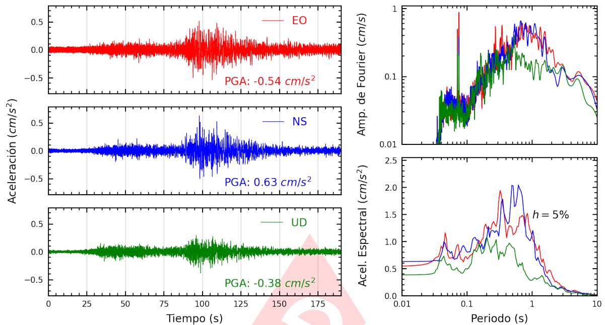
Figura A.29: Registros tiempo-historia, espectros de Fourier y de respuesta en las direcciones EO, NS y vertical de la estación UPCSM. Sismo de Chala, Caraveli - Arequipa del 2024-06-29, 02:05:31 (Hora local)
