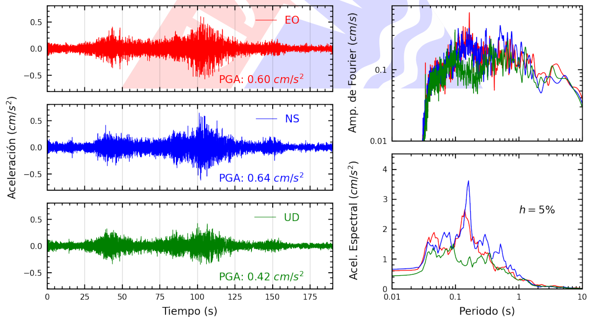
Figura A.28: Registros tiempo-historia, espectros de Fourier y de respuesta en las direcciones EO, NS y vertical de la estación SROSA. Sismo de Chala, Caraveli - Arequipa del 2024-06-29, 02:05:31 (Hora local)
