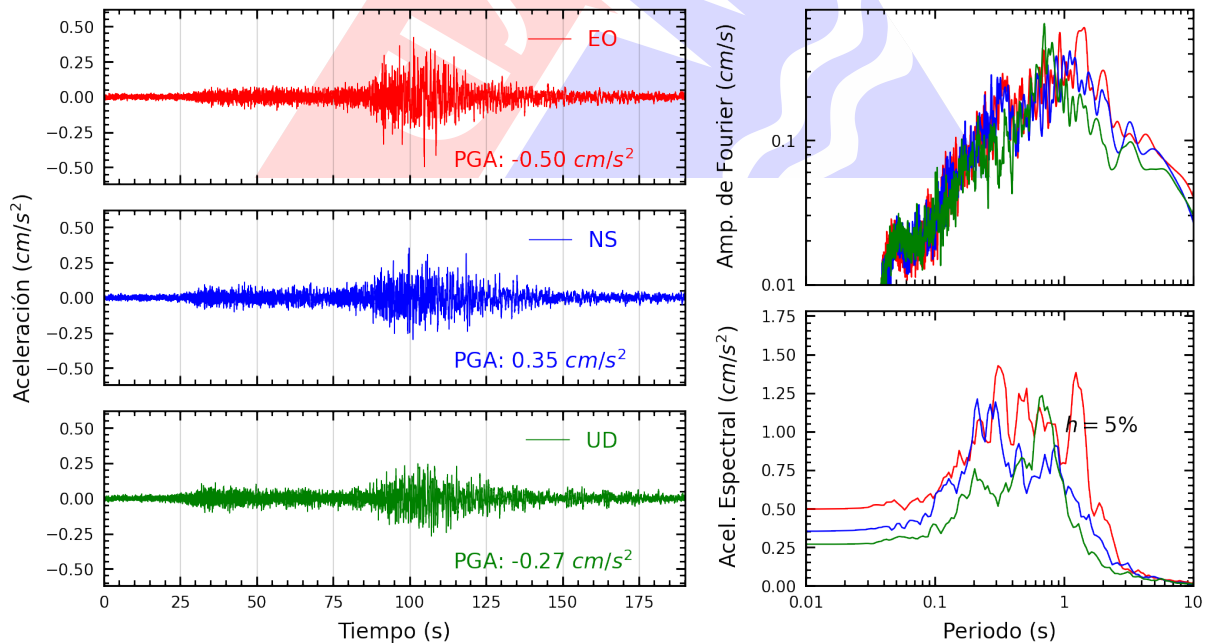
Figura A.36: Registros tiempo-historia, espectros de Fourier y de respuesta en las direcciones EO, NS y vertical de la estación CENEP. Sismo de Chala, Caraveli - Arequipa del 2024-06-29, 02:05:31 (Hora local)
