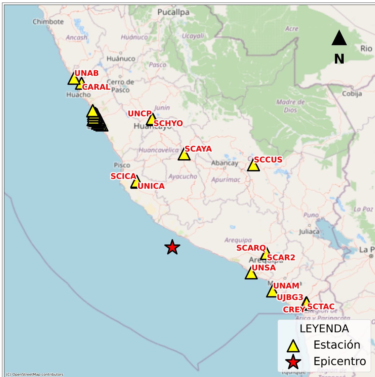
Figura 2: Mapa de ubicación de la(s) estación(es) acelerográfica(s) a nivel nacional correspondiente(s) al Sismo de Chala, Caraveli - Arequipa del 29 de junio de 2024 a las 02:05:31 (hora local)
