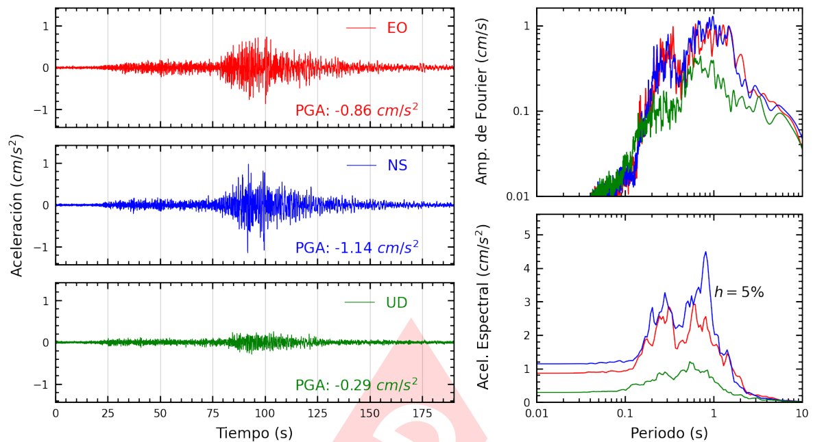
Figura A.15: Registros tiempo-historia, espectros de Fourier y de respuesta en las direcciones EO, NS y vertical de la estación DSMI. Sismo de Chala, Caraveli - Arequipa del 2024-06-29, 02:05:31 (Hora local)
