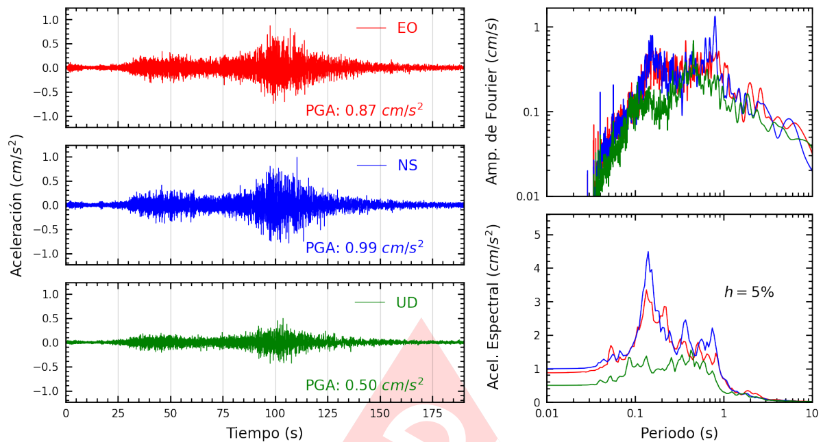
Figura A.17: Registros tiempo-historia, espectros de Fourier y de respuesta en las direcciones EO, NS y vertical de la estación USILM. Sismo de Chala, Caraveli - Arequipa del 2024-06-29, 02:05:31 (Hora local)
