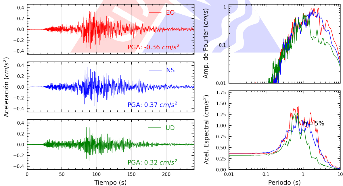
Figura A.46: Registros tiempo-historia, espectros de Fourier y de respuesta en las direcciones EO, NS y vertical de la estación UNCP. Sismo de Chala, Caraveli - Arequipa del 2024-06-29, 02:05:31 (Hora local)
