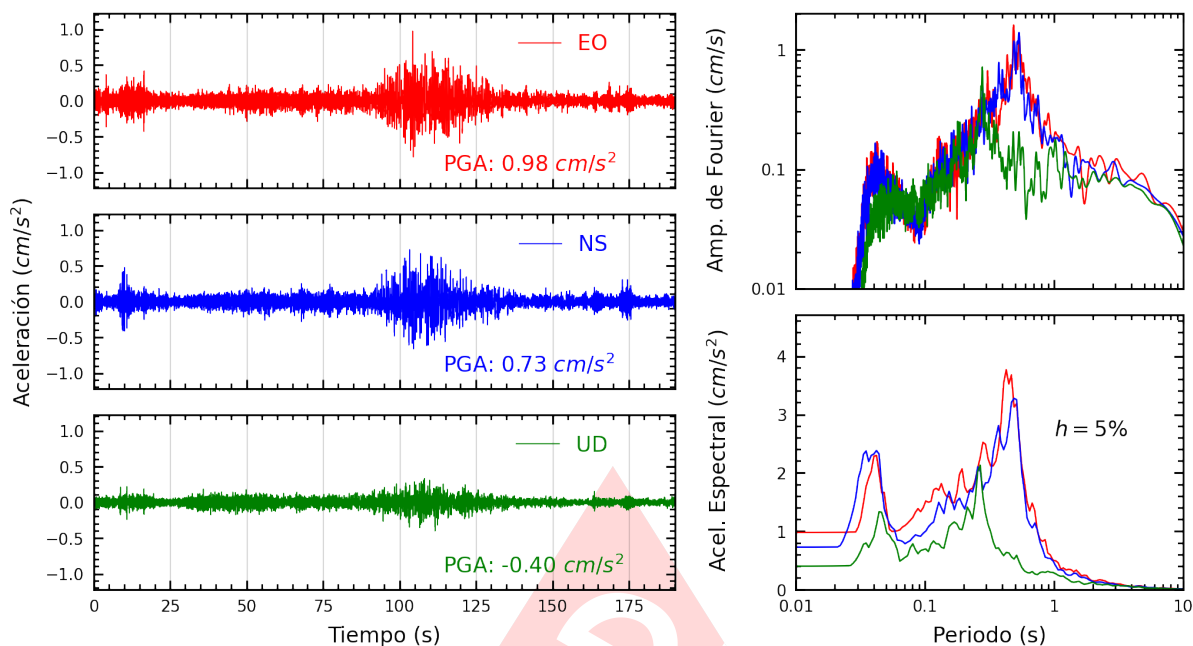
Figura A.19: Registros tiempo-historia, espectros de Fourier y de respuesta en las direcciones EO, NS y vertical de la estación OLIVO. Sismo de Chala, Caraveli - Arequipa del 2024-06-29, 02:05:31 (Hora local)
