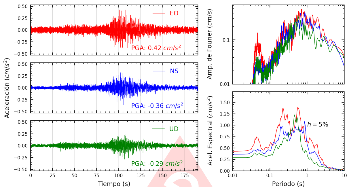
Figura A.41: Registros tiempo-historia, espectros de Fourier y de respuesta en las direcciones EO, NS y vertical de la estación INICT. Sismo de Chala, Caraveli - Arequipa del 2024-06-29, 02:05:31 (Hora local)
