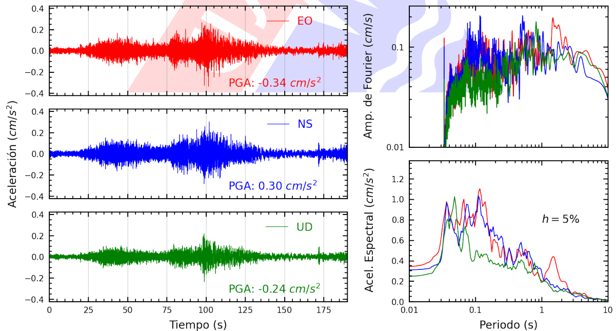
Figura A.48: Registros tiempo-historia, espectros de Fourier y de respuesta en las direcciones EO, NS y vertical de la estación JOSEO. Sismo de Chala, Caraveli - Arequipa del 2024-06-29, 02:05:31 (Hora local)
