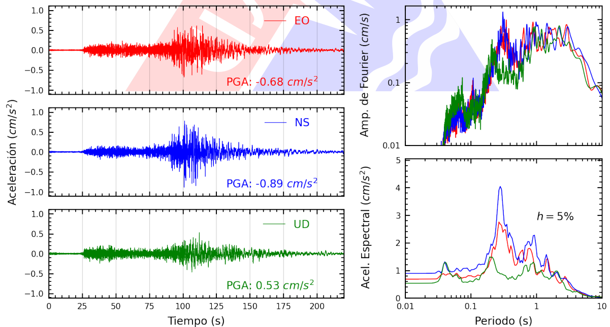
Figura A.24: Registros tiempo-historia, espectros de Fourier y de respuesta en las direcciones EO, NS y vertical de la estación SCTAC. Sismo de Chala, Caraveli - Arequipa del 2024-06-29, 02:05:31 (Hora local)
