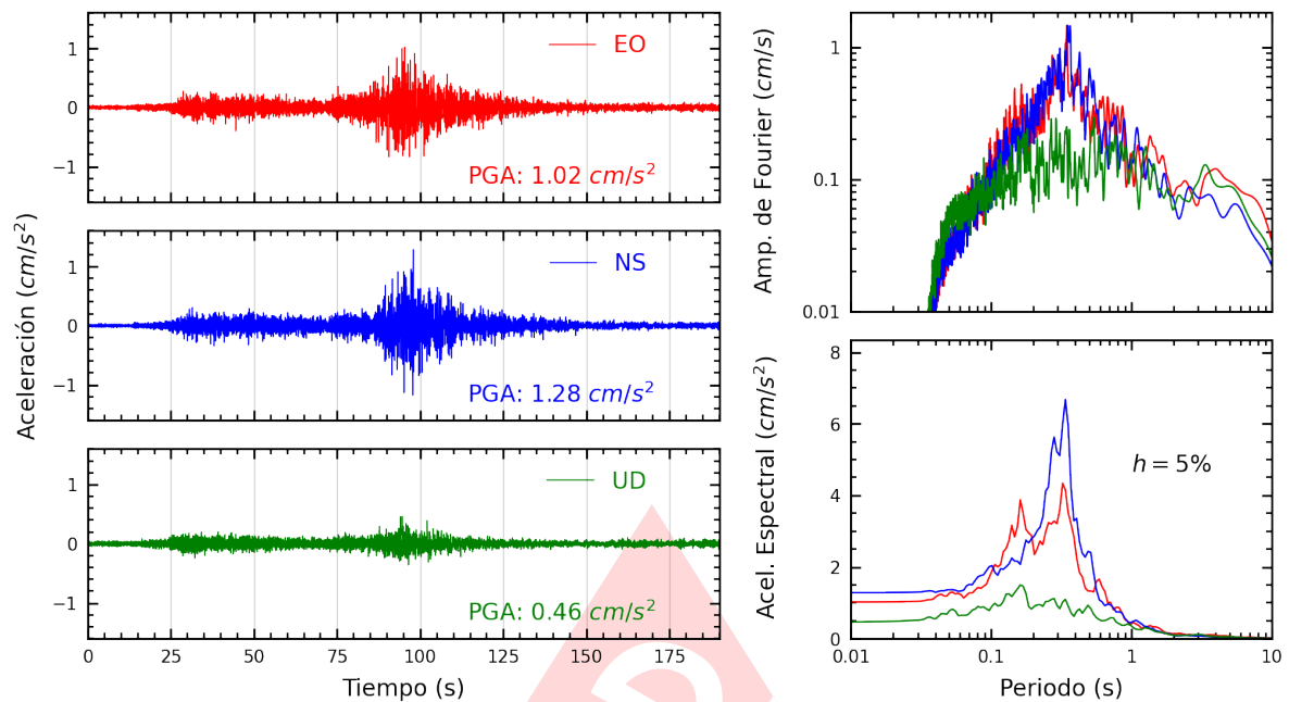
Figura A.11: Registros tiempo-historia, espectros de Fourier y de respuesta en las direcciones EO, NS y vertical de la estación ANCON. Sismo de Chala, Caraveli - Arequipa del 2024-06-29, 02:05:31 (Hora local)
