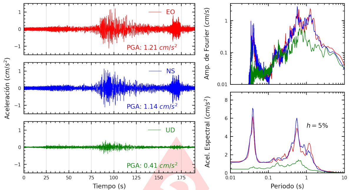
Figura A.13: Registros tiempo-historia, espectros de Fourier y de respuesta en las direcciones EO, NS y vertical de la estación DHNPE. Sismo de Chala, Caraveli - Arequipa del 2024-06-29, 02:05:31 (Hora local)
