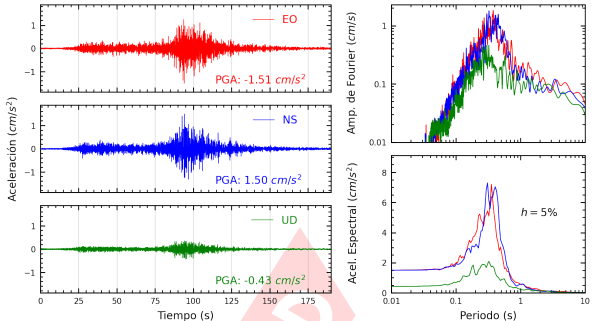
Figura A.9: Registros tiempo-historia, espectros de Fourier y de respuesta en las direcciones EO, NS y vertical de la estación DEFEN. Sismo de Chala, Caraveli - Arequipa del 2024-06-29, 02:05:31 (Hora local)
