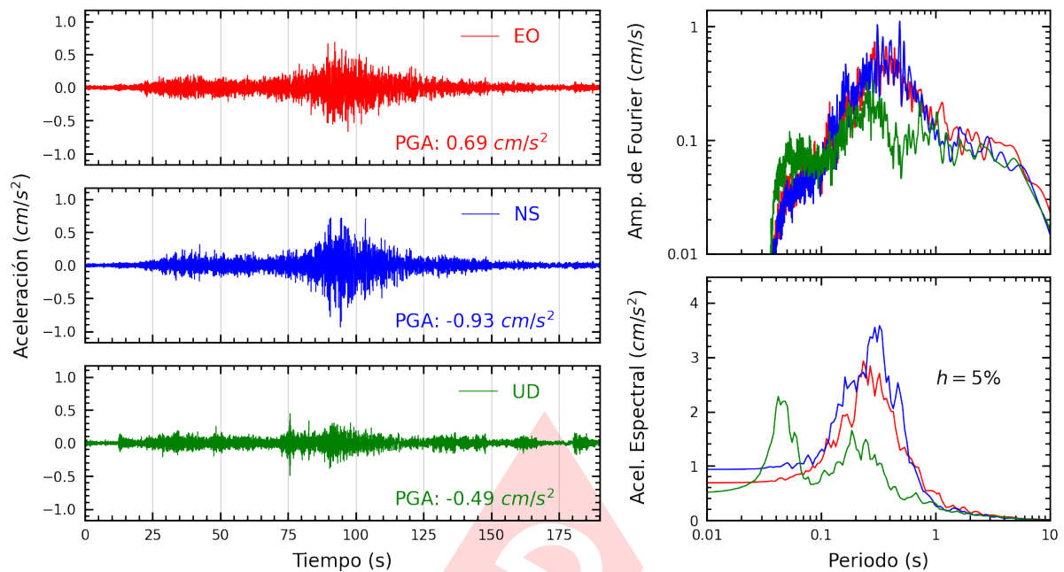
Figura A.21: Registros tiempo-historia, espectros de Fourier y de respuesta en las direcciones EO, NS y vertical de la estación SCOLI. Sismo de Chala, Caraveli - Arequipa del 2024-06-29, 02:05:31 (Hora local)
