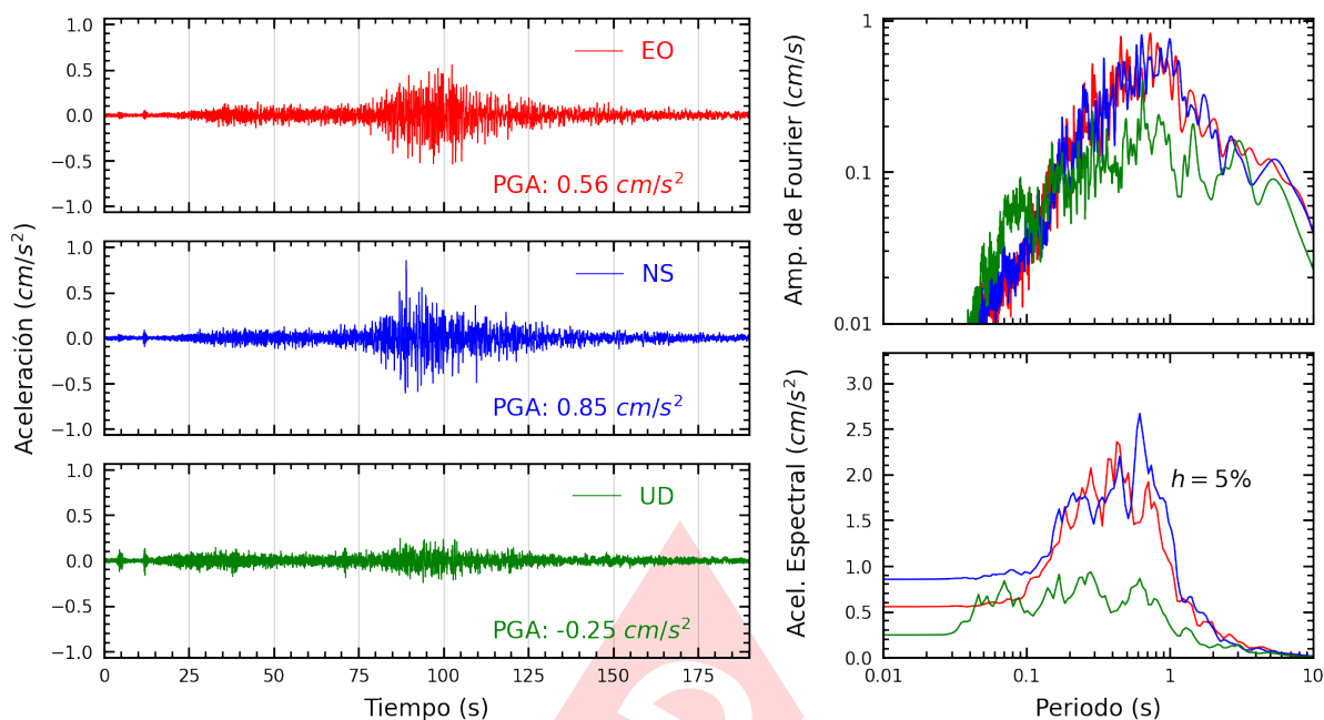
Figura A.25: Registros tiempo-historia, espectros de Fourier y de respuesta en las direcciones EO, NS y vertical de la estación RAMON. Sismo de Chala, Caraveli - Arequipa del 2024-06-29, 02:05:31 (Hora local)
