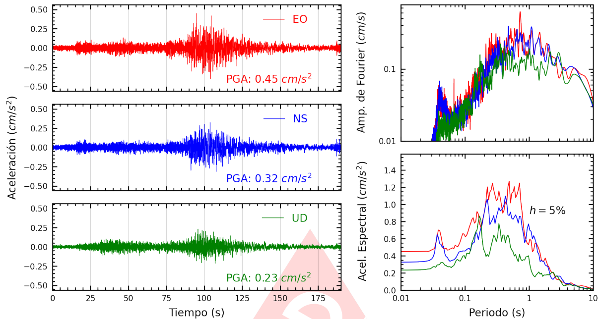
Figura A.39: Registros tiempo-historia, espectros de Fourier y de respuesta en las direcciones EO, NS y vertical de la estación CEPRE. Sismo de Chala, Caraveli - Arequipa del 2024-06-29, 02:05:31 (Hora local)
