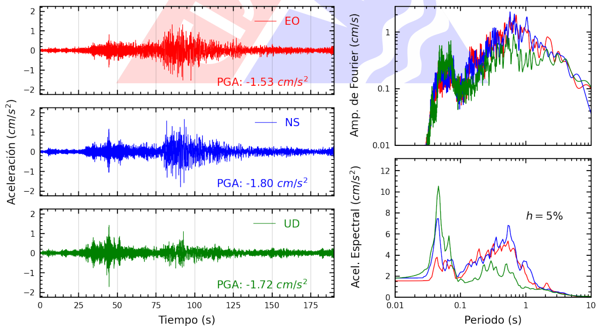
Figura A.6: Registros tiempo-historia, espectros de Fourier y de respuesta en las direcciones EO, NS y vertical de la estación SCAR2. Sismo de Chala, Caraveli - Arequipa del 2024-06-29, 02:05:31 (Hora local)
