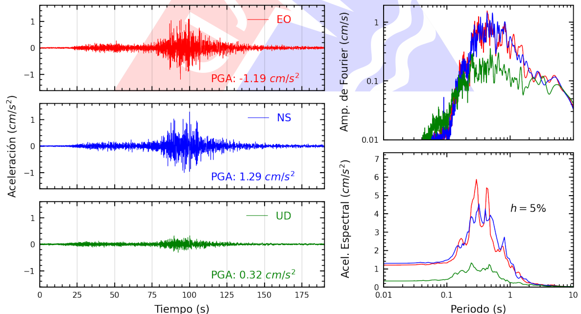
Figura A.10: Registros tiempo-historia, espectros de Fourier y de respuesta en las direcciones EO, NS y vertical de la estación ACAPU. Sismo de Chala, Caraveli - Arequipa del 2024-06-29, 02:05:31 (Hora local)
