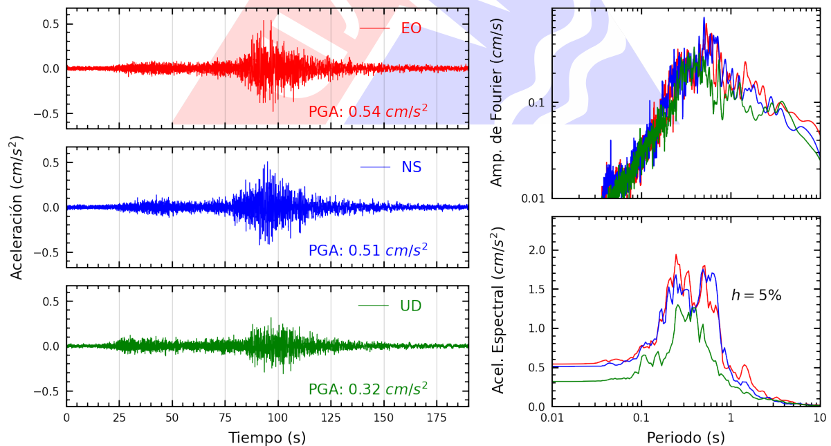
Figura A.34: Registros tiempo-historia, espectros de Fourier y de respuesta en las direcciones EO, NS y vertical de la estación COMAS. Sismo de Chala, Caraveli - Arequipa del 2024-06-29, 02:05:31 (Hora local)
