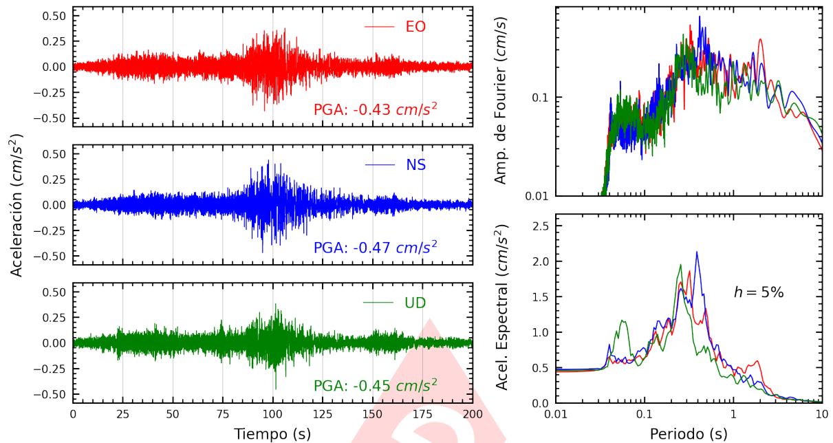
Figura A.37: Registros tiempo-historia, espectros de Fourier y de respuesta en las direcciones EO, NS y vertical de la estación URPPE. Sismo de Chala, Caraveli - Arequipa del 2024-06-29, 02:05:31 (Hora local)
