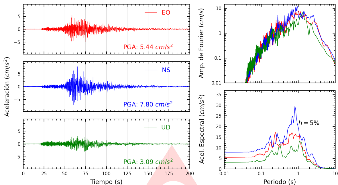
Figura A.1: Registros tiempo-historia, espectros de Fourier y de respuesta en las direcciones EO, NS y vertical de la estación UNICA. Sismo de Chala, Caraveli - Arequipa del 2024-06-29, 02:05:31 (Hora local)
