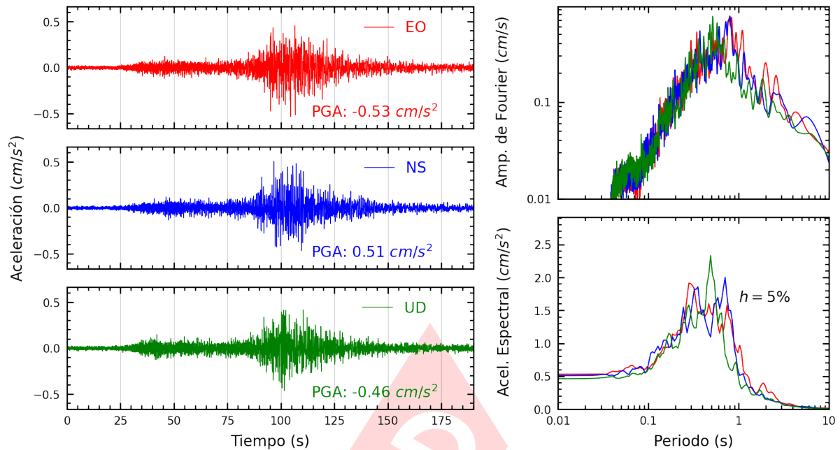
Figura A.35: Registros tiempo-historia, espectros de Fourier y de respuesta en las direcciones EO, NS y vertical de la estación IMCA. Sismo de Chala, Caraveli - Arequipa del 2024-06-29, 02:05:31 (Hora local)
