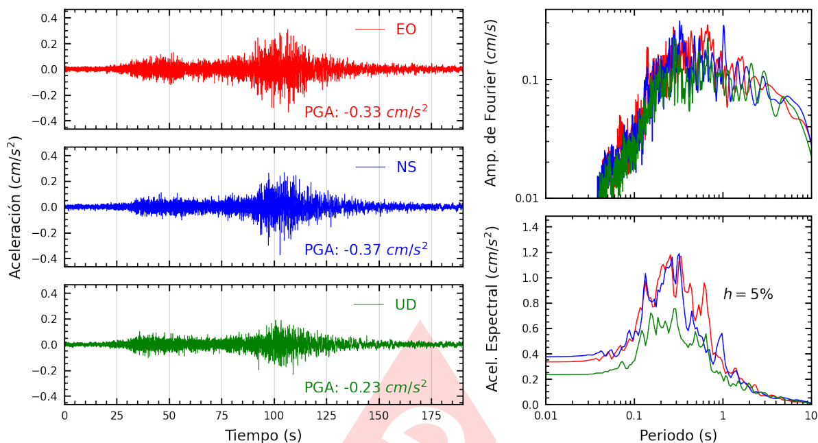
Figura A.45: Registros tiempo-historia, espectros de Fourier y de respuesta en las direcciones EO, NS y vertical de la estación FICPE. Sismo de Chala, Caraveli - Arequipa del 2024-06-29, 02:05:31 (Hora local)
