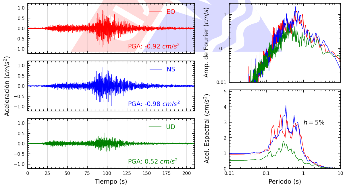
Figura A.18: Registros tiempo-historia, espectros de Fourier y de respuesta en las direcciones EO, NS y vertical de la estación USILP. Sismo de Chala, Caraveli - Arequipa del 2024-06-29, 02:05:31 (Hora local)
