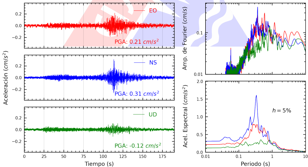
Figura A.50: Registros tiempo-historia, espectros de Fourier y de respuesta en las direcciones EO, NS y vertical de la estación UNAB. Sismo de Chala, Caraveli - Arequipa del 2024-06-29, 02:05:31 (Hora local)
