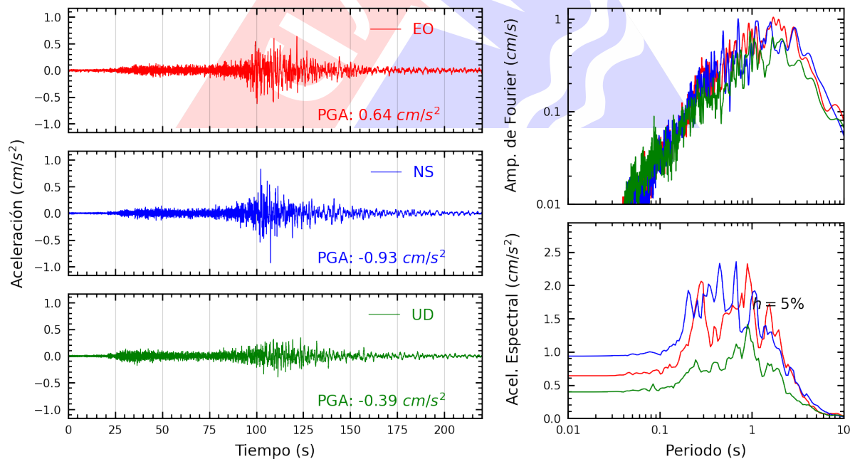
Figura A.22: Registros tiempo-historia, espectros de Fourier y de respuesta en las direcciones EO, NS y vertical de la estación UJBG3. Sismo de Chala, Caraveli - Arequipa del 2024-06-29, 02:05:31 (Hora local)
