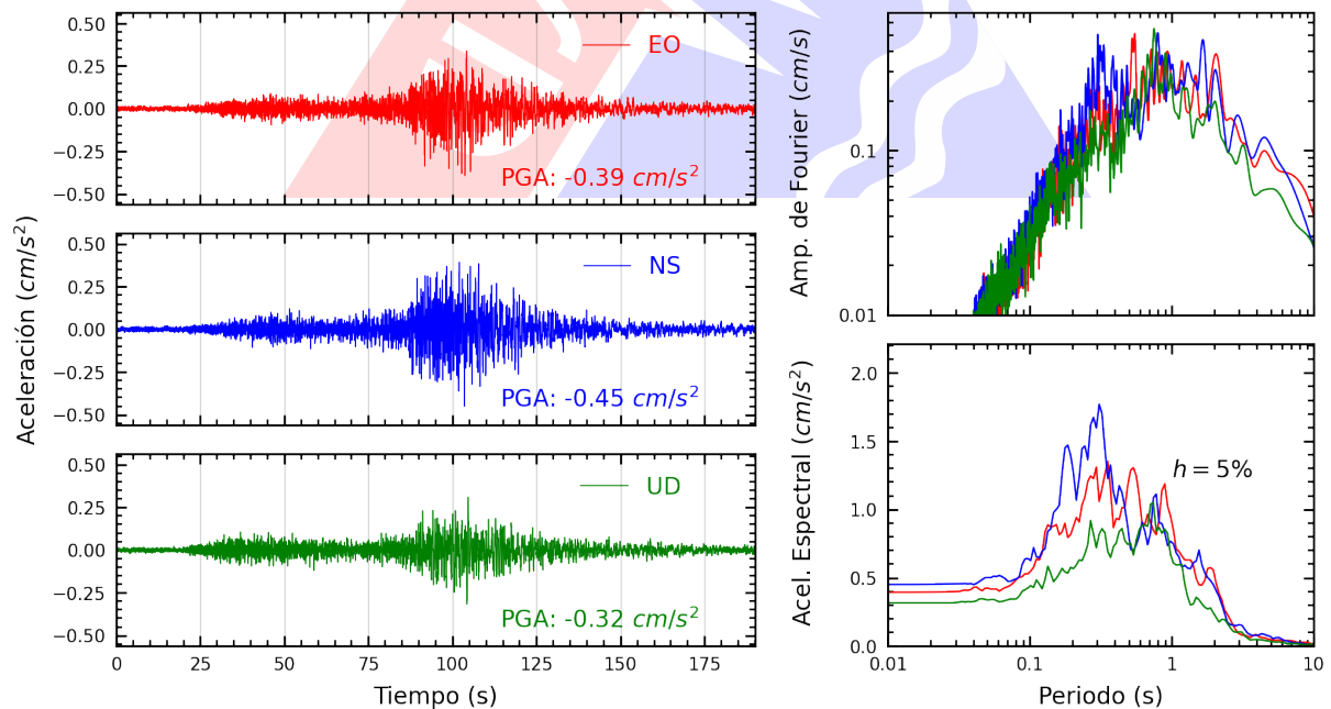
Figura A.38: Registros tiempo-historia, espectros de Fourier y de respuesta en las direcciones EO, NS y vertical de la estación SERVI. Sismo de Chala, Caraveli - Arequipa del 2024-06-29, 02:05:31 (Hora local)
