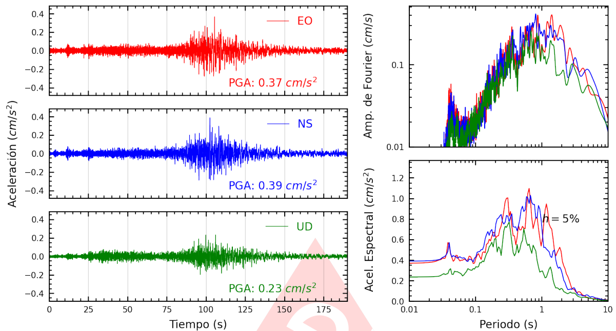
Figura A.43: Registros tiempo-historia, espectros de Fourier y de respuesta en las direcciones EO, NS y vertical de la estación BORJA. Sismo de Chala, Caraveli - Arequipa del 2024-06-29, 02:05:31 (Hora local)
