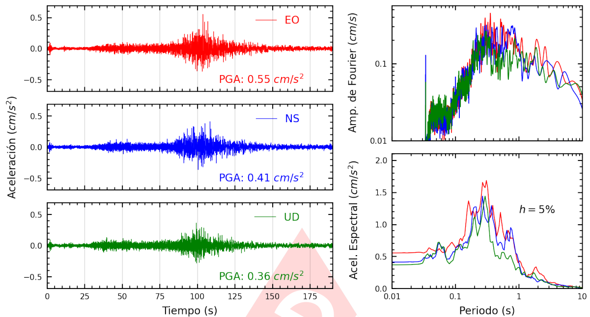
Figura A.33: Registros tiempo-historia, espectros de Fourier y de respuesta en las direcciones EO, NS y vertical de la estación USMP. Sismo de Chala, Caraveli - Arequipa del 2024-06-29, 02:05:31 (Hora local)
