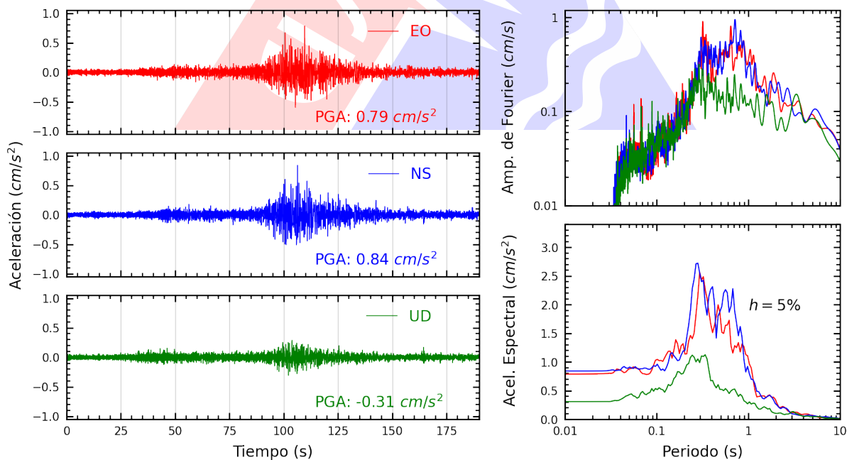
Figura A.26: Registros tiempo-historia, espectros de Fourier y de respuesta en las direcciones EO, NS y vertical de la estación MADRE. Sismo de Chala, Caraveli - Arequipa del 2024-06-29, 02:05:31 (Hora local)
