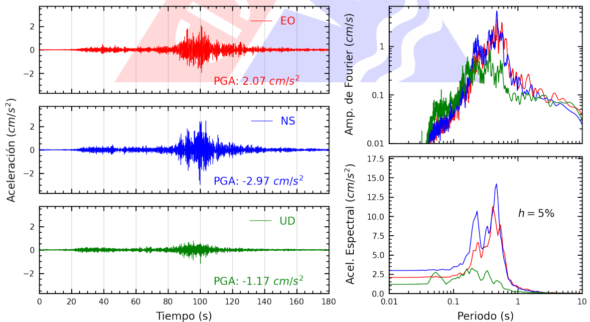
Figura A.4: Registros tiempo-historia, espectros de Fourier y de respuesta en las direcciones EO, NS y vertical de la estación MDPP. Sismo de Chala, Caraveli - Arequipa del 2024-06-29, 02:05:31 (Hora local)
