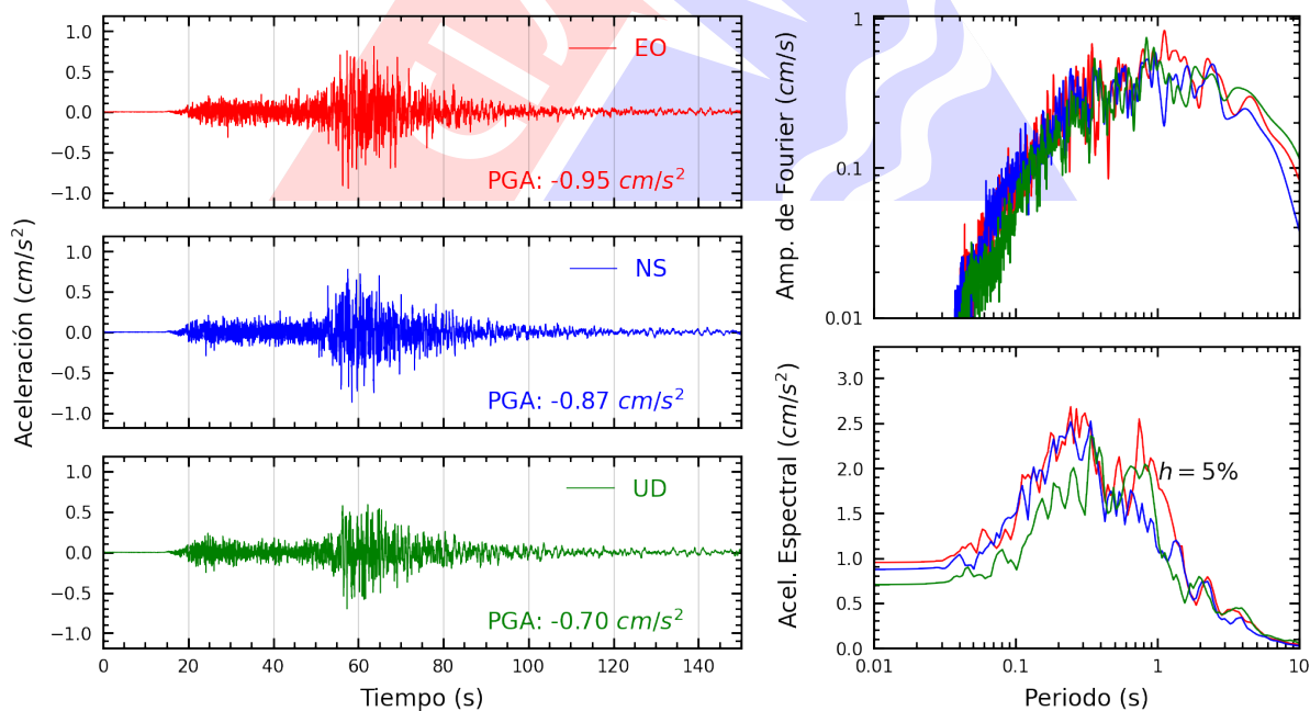
Figura A.20: Registros tiempo-historia, espectros de Fourier y de respuesta en las direcciones EO, NS y vertical de la estación UNSA. Sismo de Chala, Caraveli - Arequipa del 2024-06-29, 02:05:31 (Hora local)
