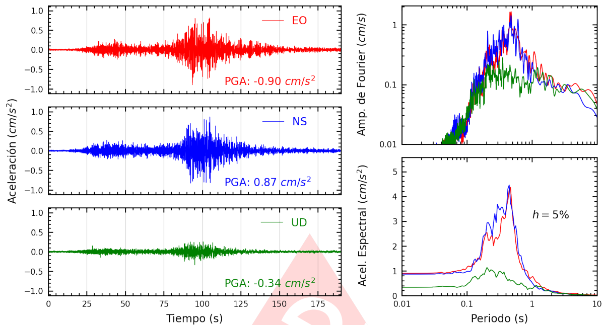
Figura A.23: Registros tiempo-historia, espectros de Fourier y de respuesta en las direcciones EO, NS y vertical de la estación VHAYA. Sismo de Chala, Caraveli - Arequipa del 2024-06-29, 02:05:31 (Hora local)
