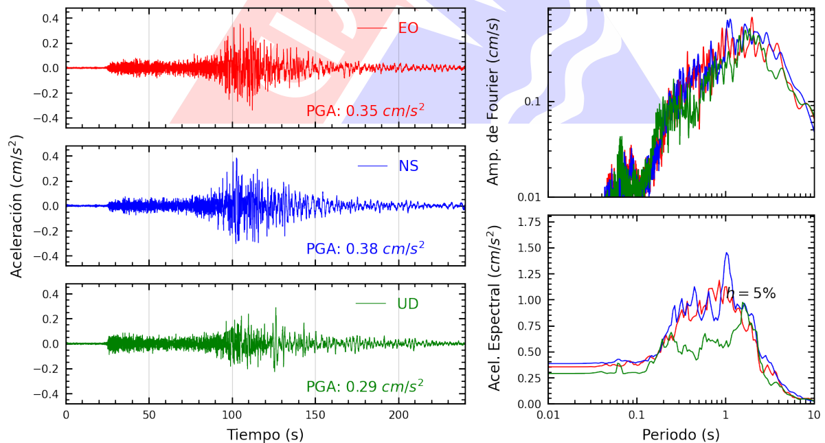
Figura A.44: Registros tiempo-historia, espectros de Fourier y de respuesta en las direcciones EO, NS y vertical de la estación CREY. Sismo de Chala, Caraveli - Arequipa del 2024-06-29, 02:05:31 (Hora local)
