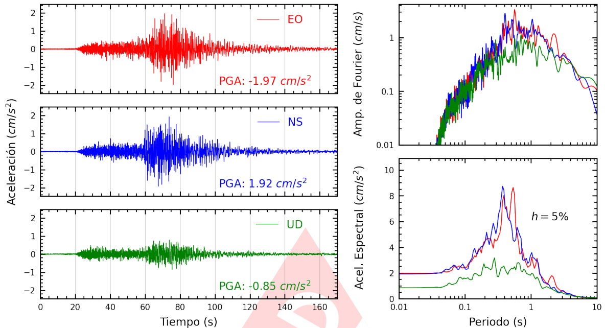
Figura A.5: Registros tiempo-historia, espectros de Fourier y de respuesta en las direcciones EO, NS y vertical de la estación SCARQ. Sismo de Chala, Caraveli - Arequipa del 2024-06-29, 02:05:31 (Hora local)
