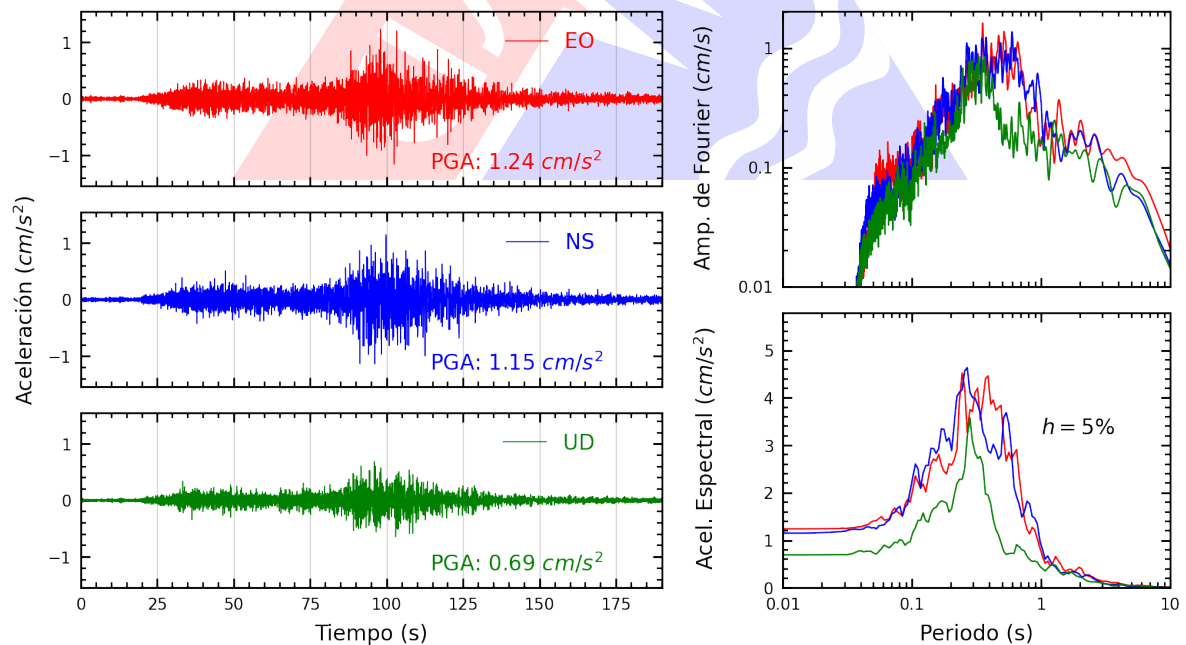
Figura A.12: Registros tiempo-historia, espectros de Fourier y de respuesta en las direcciones EO, NS y vertical de la estación UNTEL. Sismo de Chala, Caraveli - Arequipa del 2024-06-29, 02:05:31 (Hora local)
