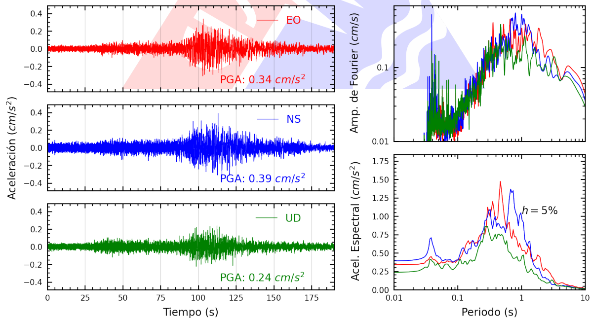
Figura A.42: Registros tiempo-historia, espectros de Fourier y de respuesta en las direcciones EO, NS y vertical de la estación BONDY. Sismo de Chala, Caraveli - Arequipa del 2024-06-29, 02:05:31 (Hora local)
