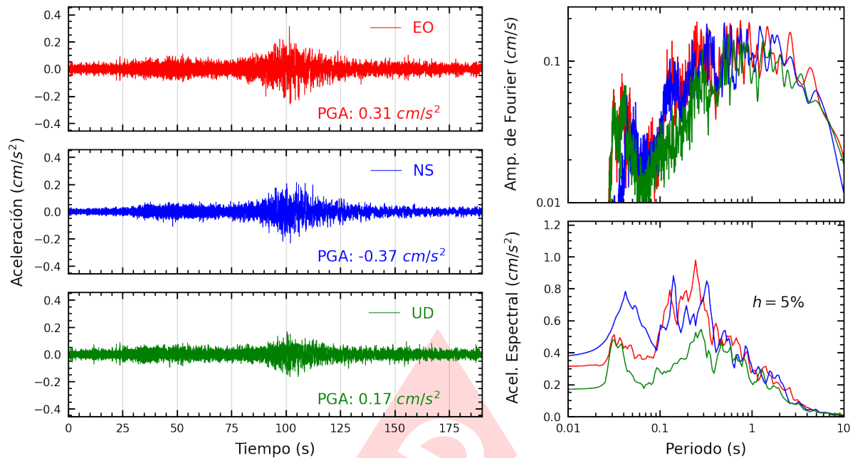
Figura A.47: Registros tiempo-historia, espectros de Fourier y de respuesta en las direcciones EO, NS y vertical de la estación ATARJ. Sismo de Chala, Caraveli - Arequipa del 2024-06-29, 02:05:31 (Hora local)
