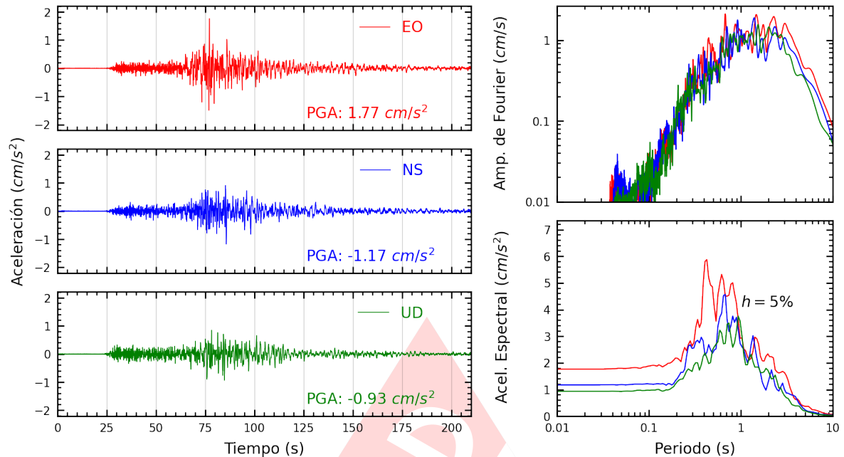
Figura A.7: Registros tiempo-historia, espectros de Fourier y de respuesta en las direcciones EO, NS y vertical de la estación SCAYA. Sismo de Chala, Caraveli - Arequipa del 2024-06-29, 02:05:31 (Hora local)
