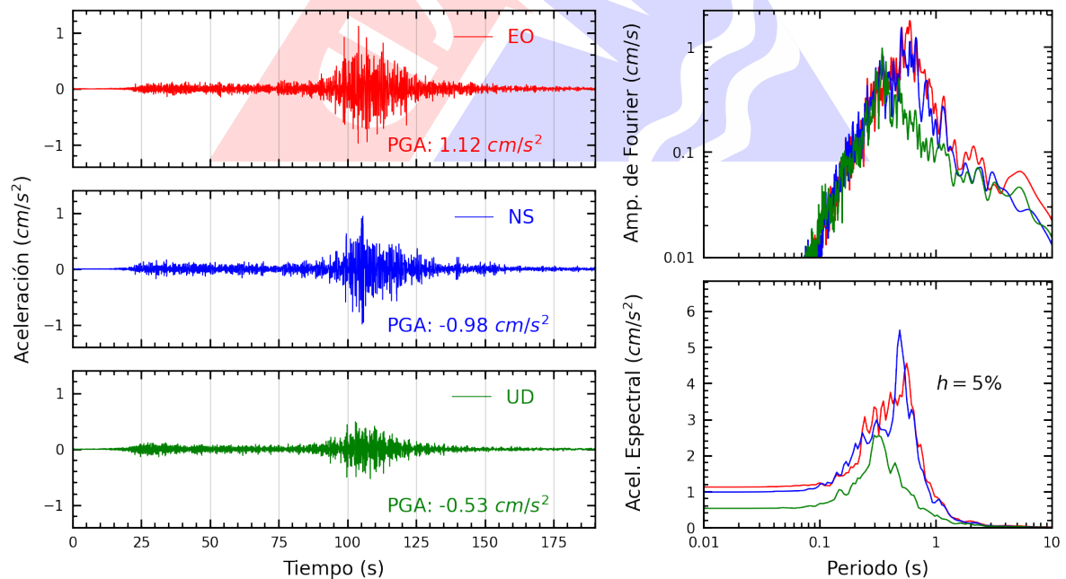
Figura A.16: Registros tiempo-historia, espectros de Fourier y de respuesta en las direcciones EO, NS y vertical de la estación CARAL. Sismo de Chala, Caraveli - Arequipa del 2024-06-29, 02:05:31 (Hora local)
