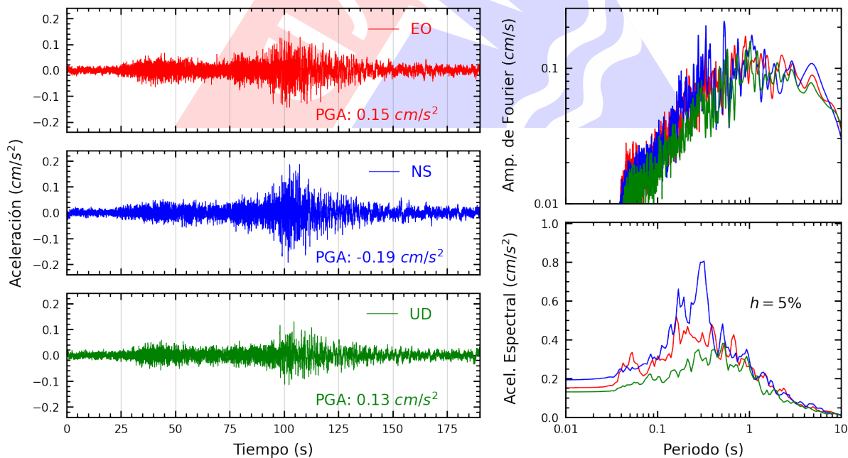
Figura A.52: Registros tiempo-historia, espectros de Fourier y de respuesta en las direcciones EO, NS y vertical de la estación UCSS. Sismo de Chala, Caraveli - Arequipa del 2024-06-29, 02:05:31 (Hora local)
