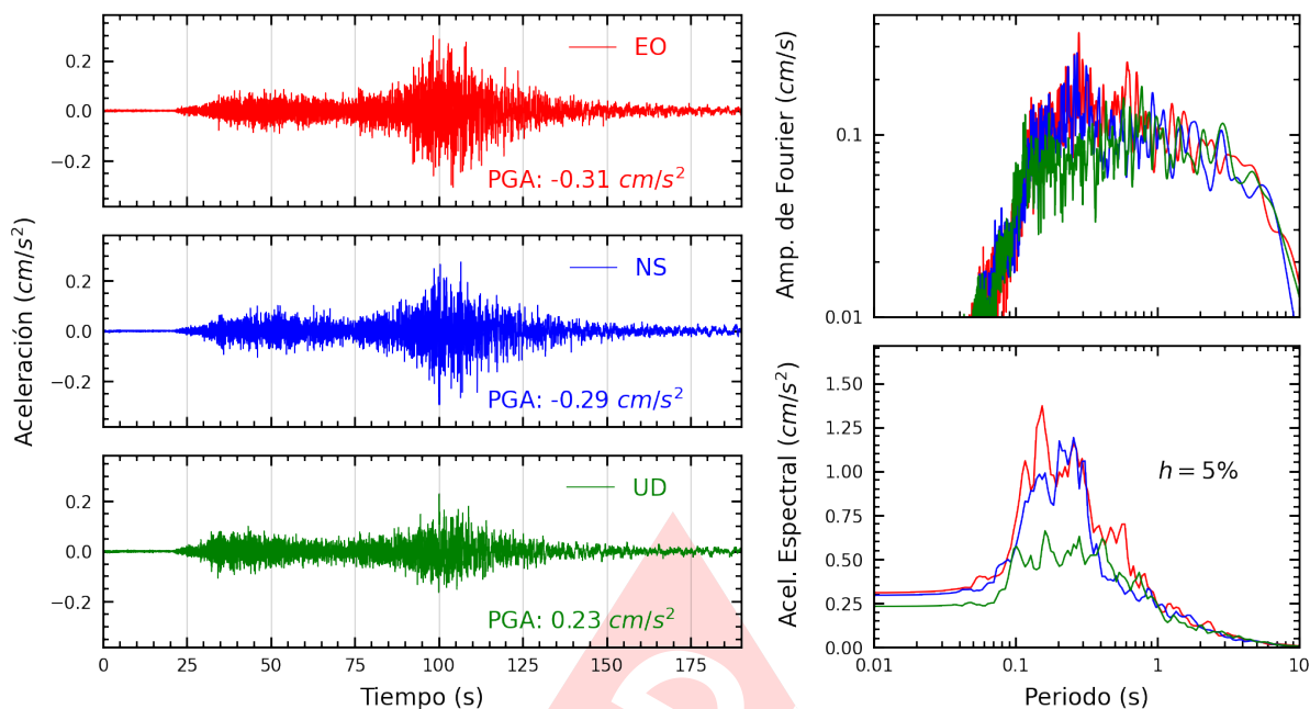
Figura A.51: Registros tiempo-historia, espectros de Fourier y de respuesta en las direcciones EO, NS y vertical de la estación JALV2. Sismo de Chala, Caraveli - Arequipa del 2024-06-29, 02:05:31 (Hora local)
