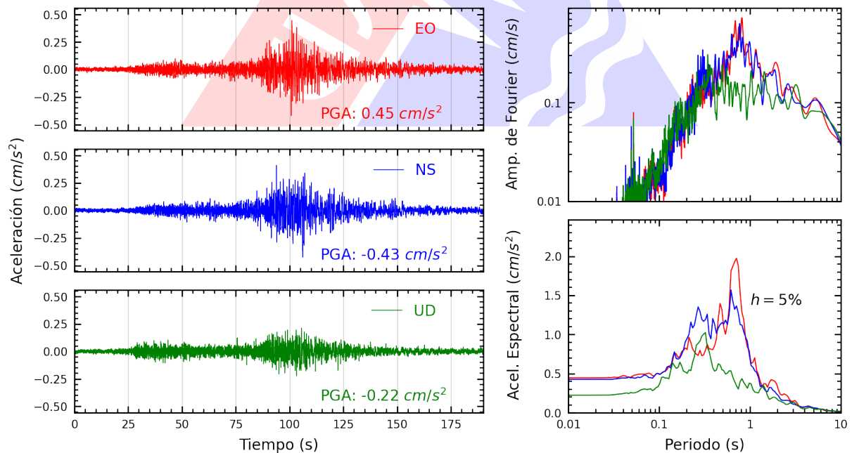
Figura A.40: Registros tiempo-historia, espectros de Fourier y de respuesta en las direcciones EO, NS y vertical de la estación UNMSM. Sismo de Chala, Caraveli - Arequipa del 2024-06-29, 02:05:31 (Hora local)
