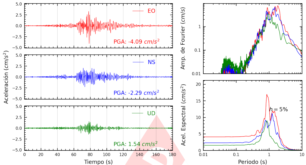
Figura A.3: Registros tiempo-historia, espectros de Fourier y de respuesta en las direcciones EO, NS y vertical de la estación SCCUS. Sismo de Chala, Caraveli - Arequipa del 2024-06-29, 02:05:31 (Hora local)
