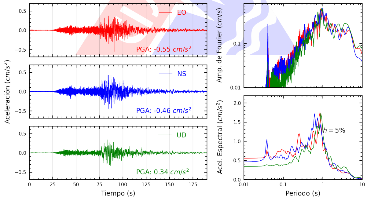
Figura A.32: Registros tiempo-historia, espectros de Fourier y de respuesta en las direcciones EO, NS y vertical de la estación UNAM. Sismo de Chala, Caraveli - Arequipa del 2024-06-29, 02:05:31 (Hora local)
