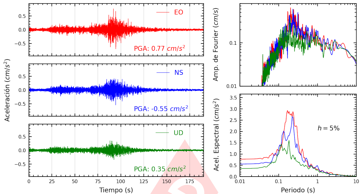
Figura A.27: Registros tiempo-historia, espectros de Fourier y de respuesta en las direcciones EO, NS y vertical de la estación INDEP. Sismo de Chala, Caraveli - Arequipa del 2024-06-29, 02:05:31 (Hora local)
