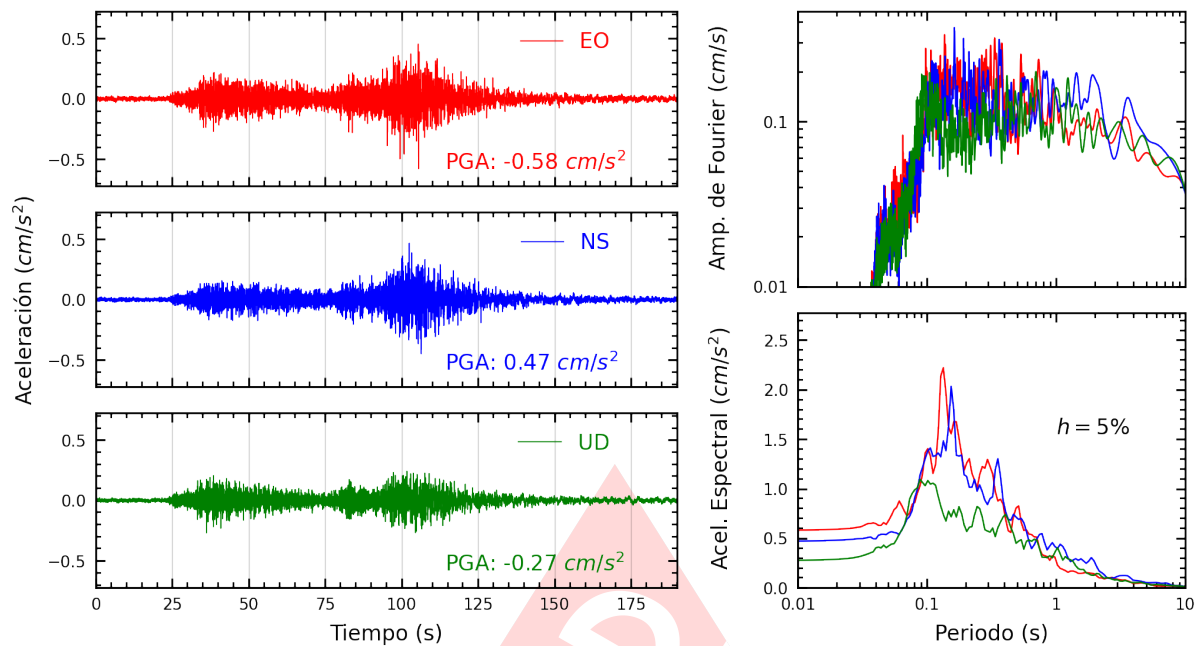
Figura A.31: Registros tiempo-historia, espectros de Fourier y de respuesta en las direcciones EO, NS y vertical de la estación AMORE. Sismo de Chala, Caraveli - Arequipa del 2024-06-29, 02:05:31 (Hora local)
