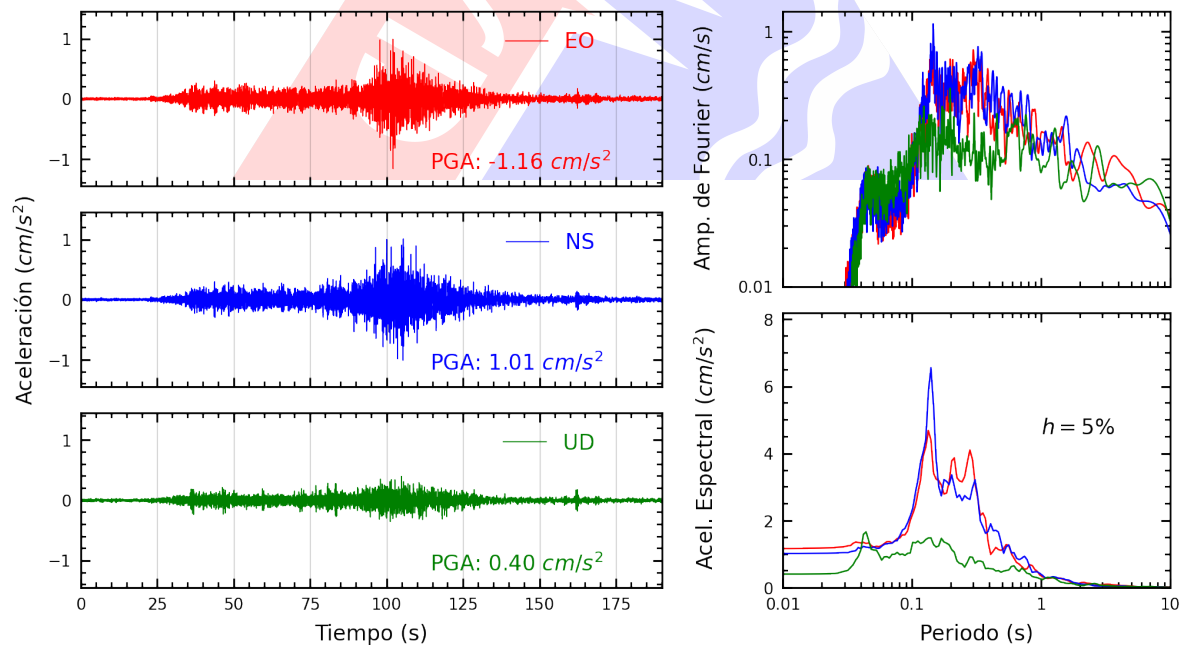
Figura A.14: Registros tiempo-historia, espectros de Fourier y de respuesta en las direcciones EO, NS y vertical de la estación CARAB. Sismo de Chala, Caraveli - Arequipa del 2024-06-29, 02:05:31 (Hora local)
