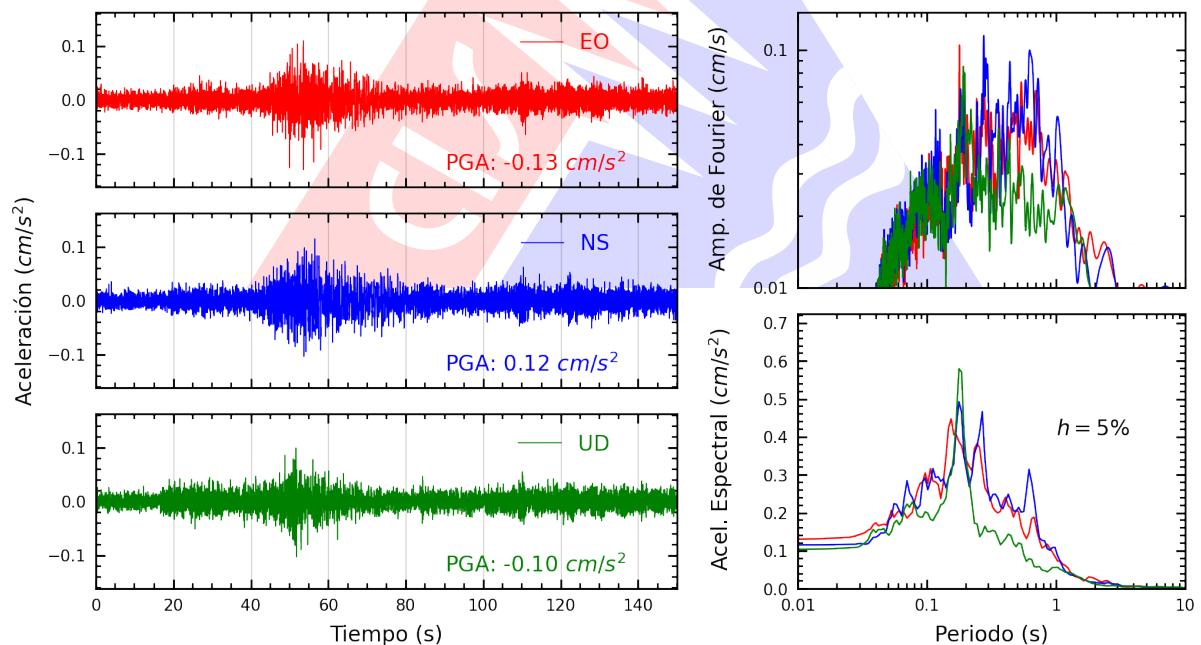
Figura A.2: Registros tiempo-historia, espectros de Fourier y de respuesta en las direcciones EO, NS y vertical de la estación UNICA. Sismo de Yauca, Caraveli - Arequipa del 2024-06-29, 04:08:30 (Hora local)
