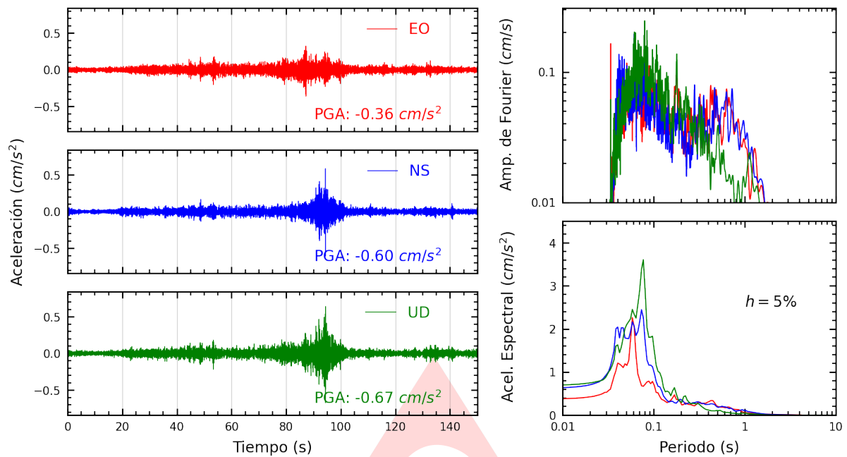
Figura A.1: Registros tiempo-historia, espectros de Fourier y de respuesta en las direcciones EO, NS y vertical de la estación SCICA. Sismo de Yauca, Caraveli - Arequipa del 2024-06-29, 04:08:30 (Hora local)
