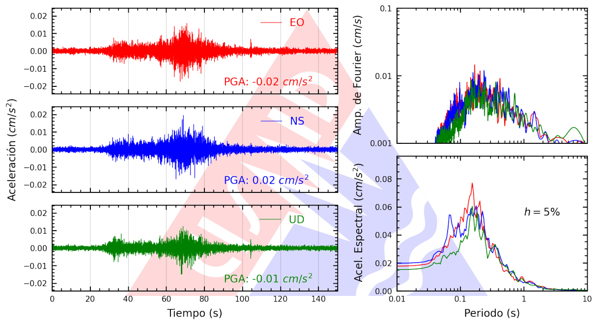
Figura A.3: Registros tiempo-historia, espectros de Fourier y de respuesta en las direcciones EO, NS y vertical de la estación UNSA. Sismo de Yauca, Caraveli - Arequipa del 2024-06-29, 04:08:30 (Hora local)
