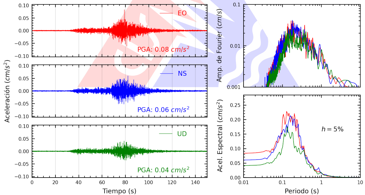
Figura A.2: Registros tiempo-historia, espectros de Fourier y de respuesta en las direcciones EO, NS y vertical de la estación UNSA. Sismo de Lomas, Caraveli - Arequipa del 2024-06-29, 07:24:43 (Hora local)
