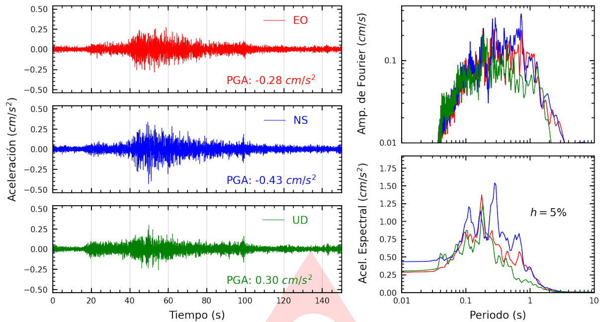
Figura A.1: Registros tiempo-historia, espectros de Fourier y de respuesta en las direcciones EO, NS y vertical de la estación UNICA. Sismo de Lomas, Caraveli - Arequipa del 2024-06-29, 07:24:43 (Hora local)
