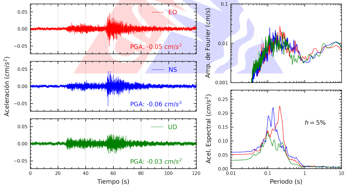
Figura A.2: Registros tiempo-historia, espectros de Fourier y de respuesta en las direcciones EO, NS y vertical de la estación CARAL. Sismo de Codo Del Pozuzo, Puerto Inca - Huanuco del 2024-06-29, 16:30:47 (Hora local)
