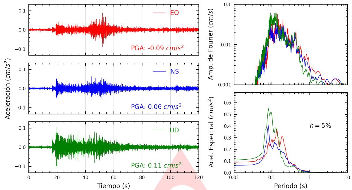
Figura A.1: Registros tiempo-historia, espectros de Fourier y de respuesta en las direcciones EO, NS y vertical de la estación UNIA. Sismo de Codo Del Pozuzo, Puerto Inca - Huanuco del 2024-06-29, 16:30:47 (Hora local)
