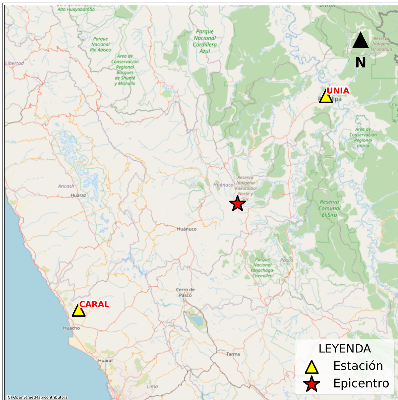
Figura 2: Mapa de ubicación de la(s) estación(es) acelerográfica(s) correspondiente(s) al Sismo de Codo Del Pozuzo, Puerto Inca - Huanuco del 29 de junio de 2024 a las 16:30:47 (hora local)
