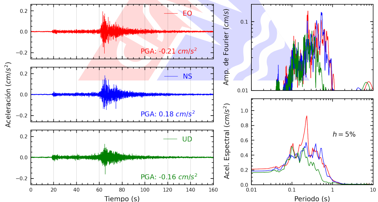
Figura A.2: Registros tiempo-historia, espectros de Fourier y de respuesta en las direcciones EO, NS y vertical de la estación CARAL. Sismo de Pucallpa, Coronel Portillo - Ucayali del 2024-06-30, 15:47:37 (Hora local)
