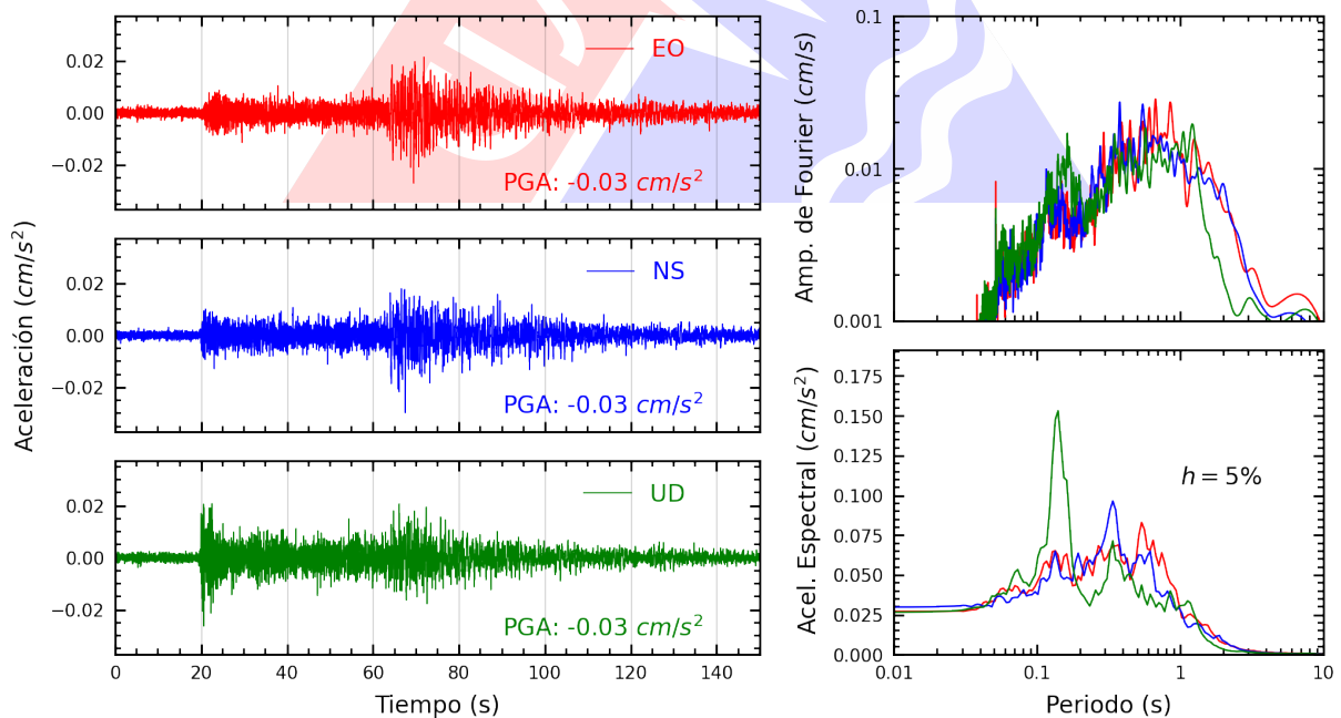
Figura A.4: Registros tiempo-historia, espectros de Fourier y de respuesta en las direcciones EO, NS y vertical de la estación UNCP. Sismo de Pucallpa, Coronel Portillo - Ucayali del 2024-06-30, 15:47:37 (Hora local)
