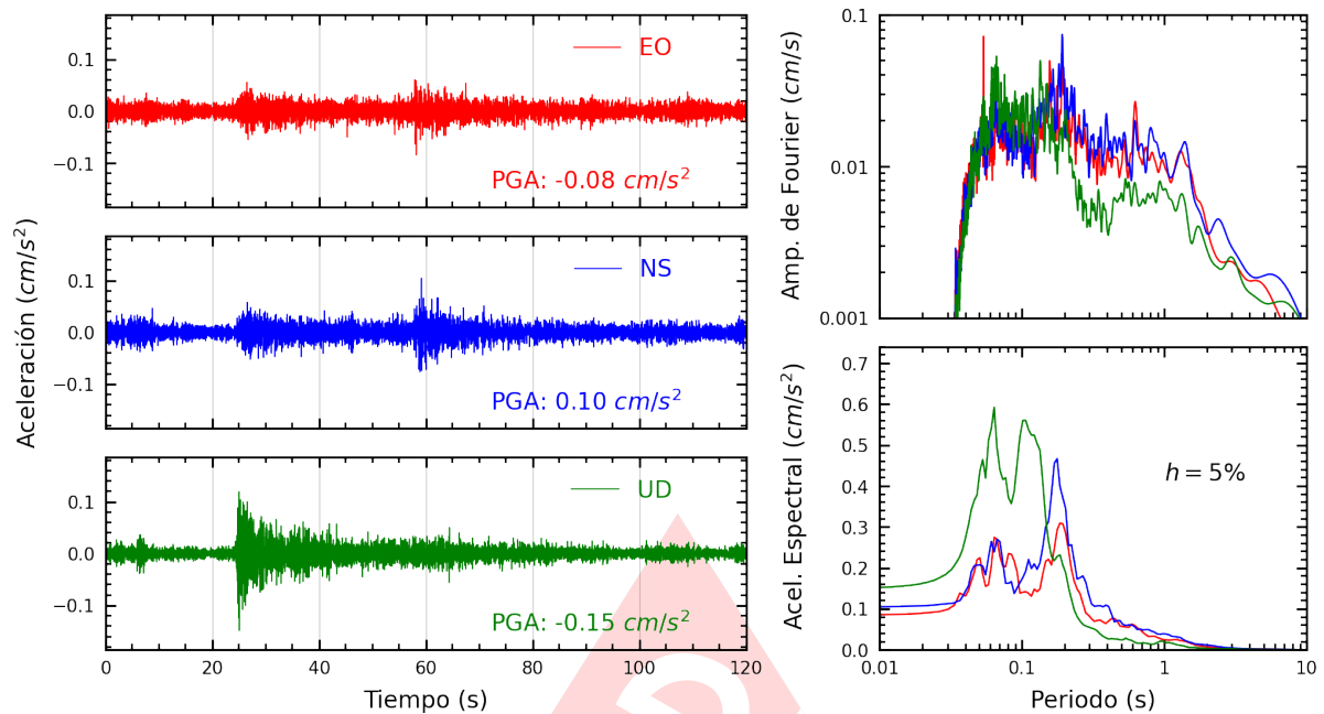
Figura A.3: Registros tiempo-historia, espectros de Fourier y de respuesta en las direcciones EO, NS y vertical de la estación UNAAA. Sismo de Pucallpa, Coronel Portillo - Ucayali del 2024-06-30, 15:47:37 (Hora local)
