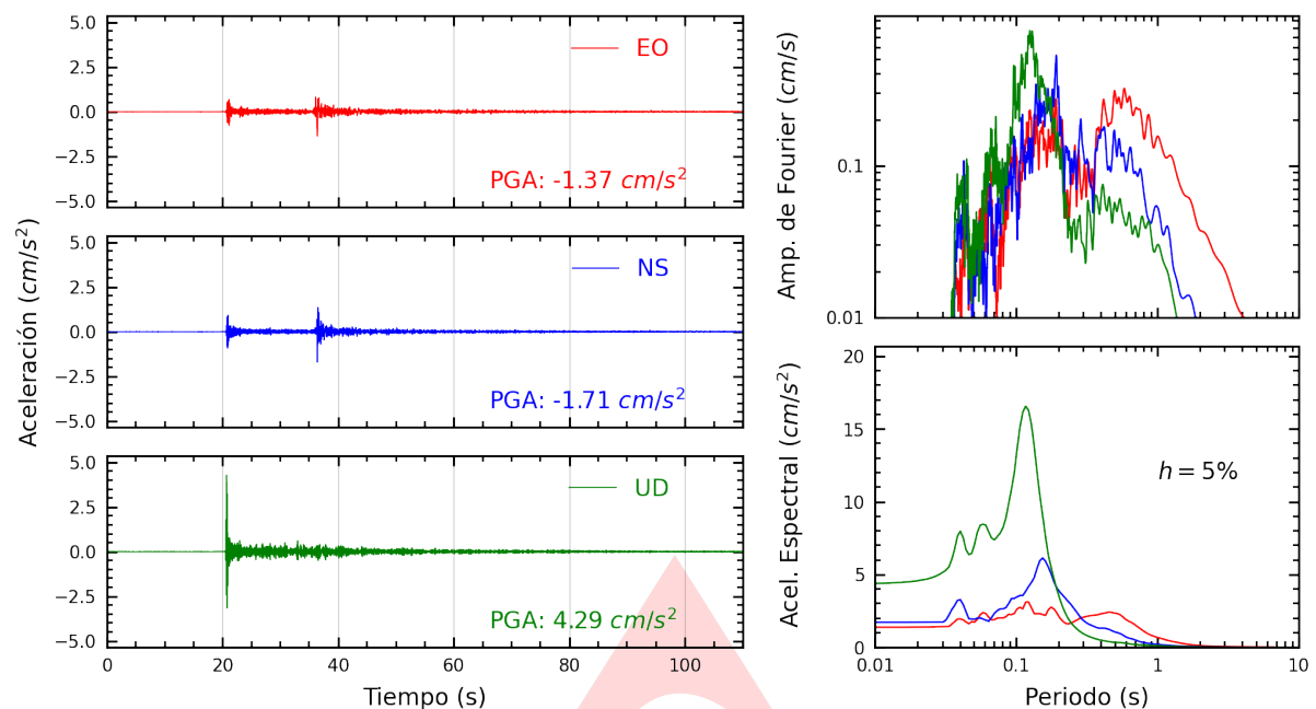
Figura A.1: Registros tiempo-historia, espectros de Fourier y de respuesta en las direcciones EO, NS y vertical de la estación UNIA. Sismo de Pucallpa, Coronel Portillo - Ucayali del 2024-06-30, 15:47:37 (Hora local)
