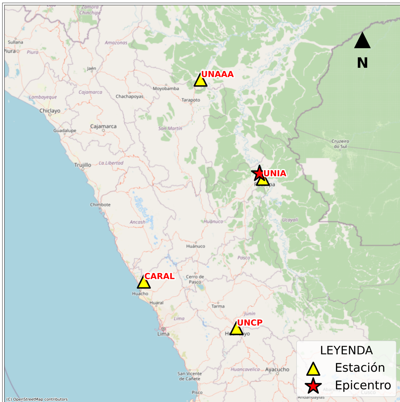
Figura 2: Mapa de ubicación de la(s) estación(es) acelerográfica(s) correspondiente(s) al Sismo de Pucallpa, Coronel Portillo - Ucayali del 30 de junio de 2024 a las 15:47:37 (hora local)
