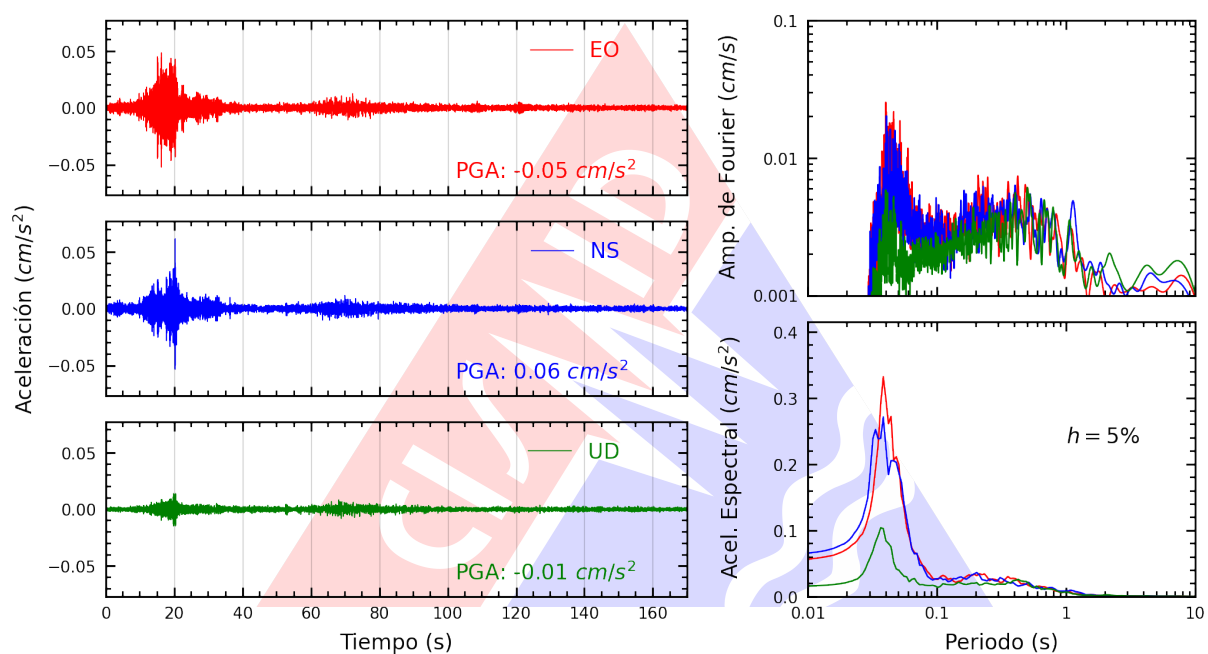
Figura A.3: Registros tiempo-historia, espectros de Fourier y de respuesta en las direcciones EO, NS y vertical de la estación UNSA. Sismo de Yauca, Caraveli - Arequipa del 2024-07-04, 14:33:26 (Hora local)
