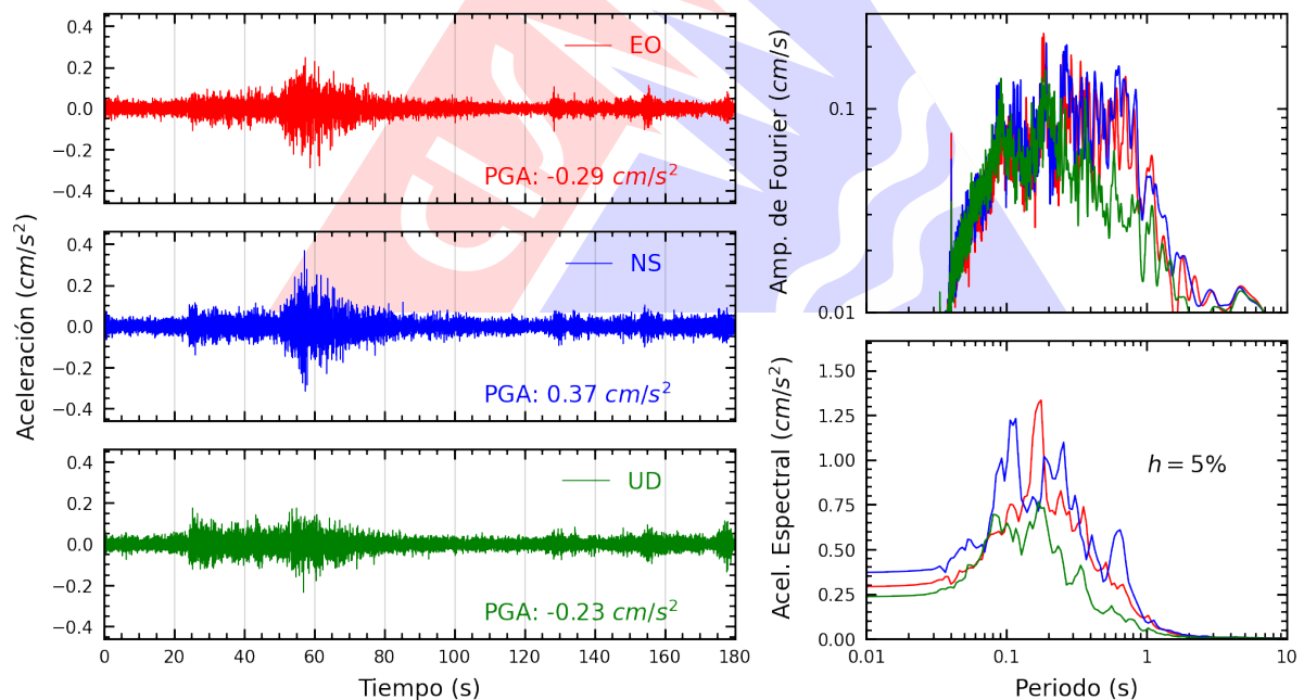
Figura A.2: Registros tiempo-historia, espectros de Fourier y de respuesta en las direcciones EO, NS y vertical de la estación UNICA. Sismo de Yauca, Caraveli - Arequipa del 2024-07-04, 14:33:26 (Hora local)
