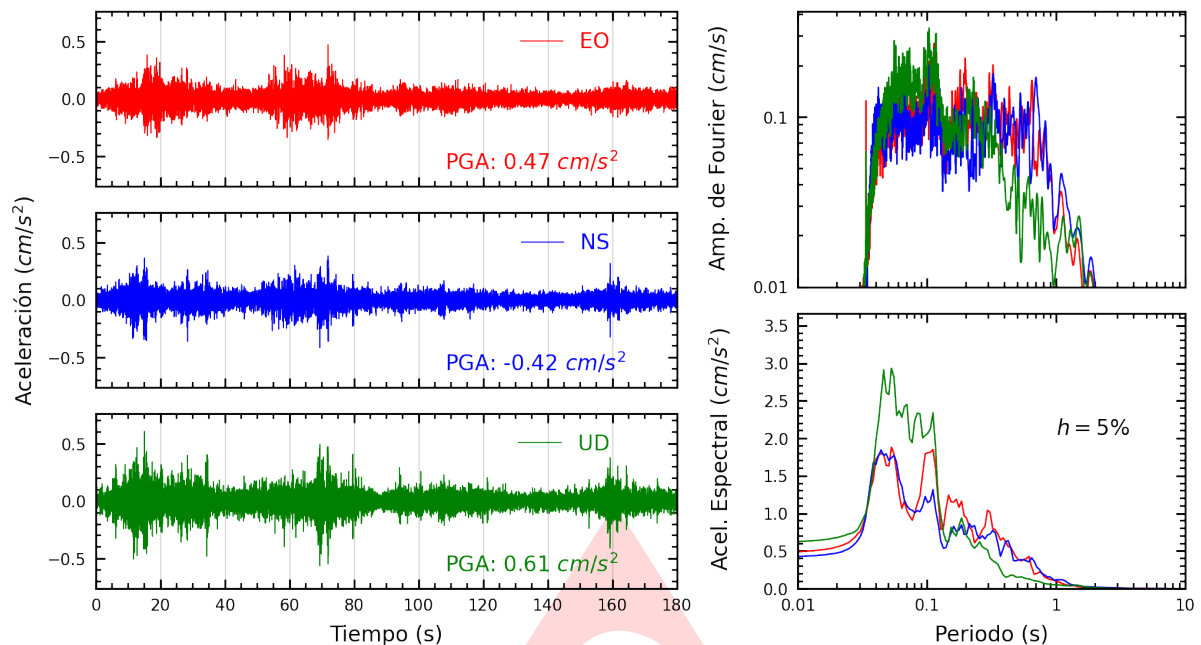
Figura A.1: Registros tiempo-historia, espectros de Fourier y de respuesta en las direcciones EO, NS y vertical de la estación SCICA. Sismo de Yauca, Caraveli - Arequipa del 2024-07-04, 14:33:26 (Hora local)
