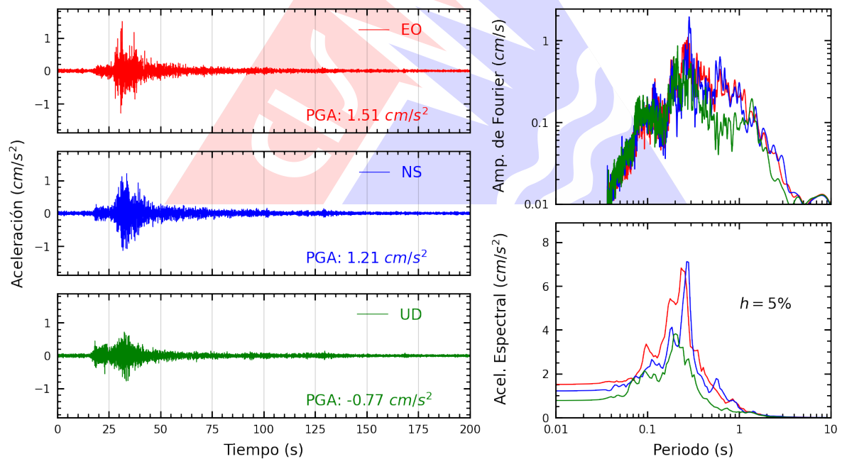
Figura A.2: Registros tiempo-historia, espectros de Fourier y de respuesta en las direcciones EO, NS y vertical de la estación UNICA. Sismo de Ica, Ica - Ica del 2024-07-04, 16:56:40 (Hora local)
