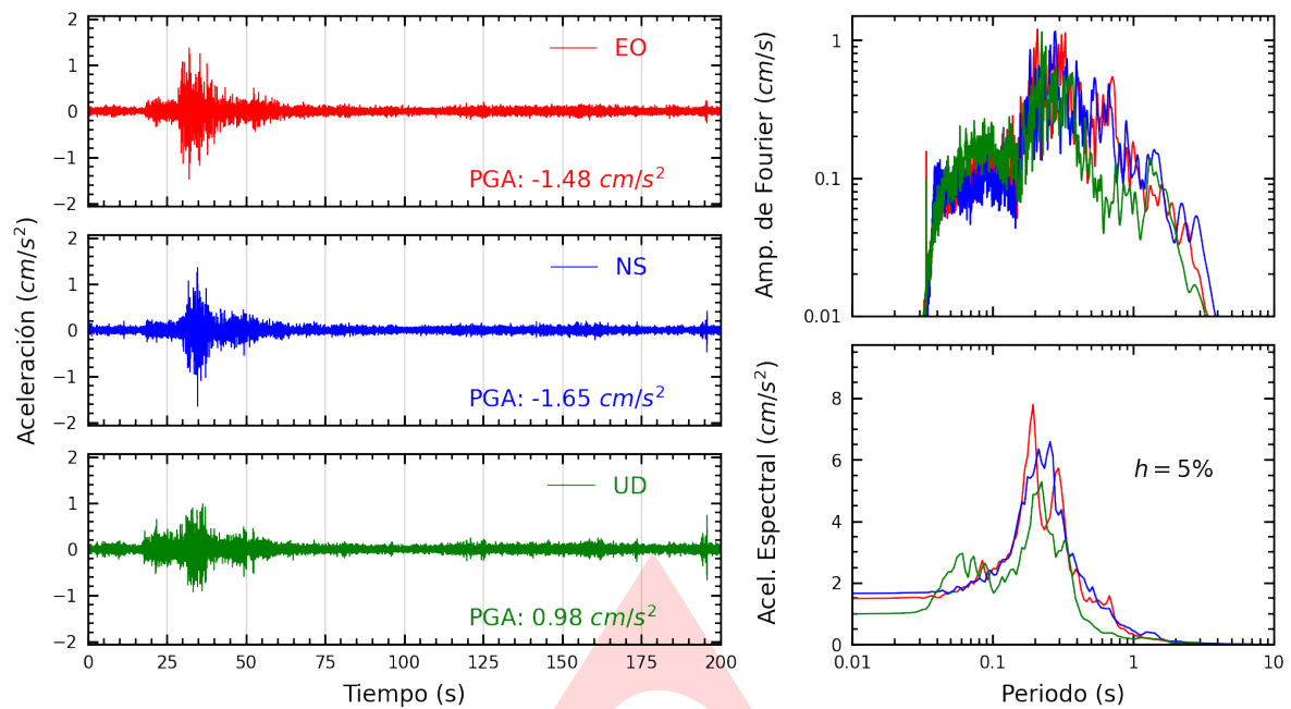
Figura A.1: Registros tiempo-historia, espectros de Fourier y de respuesta en las direcciones EO, NS y vertical de la estación SCICA. Sismo de Ica, Ica - Ica del 2024-07-04, 16:56:40 (Hora local)
