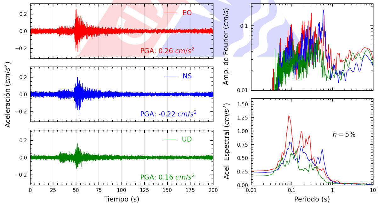
Figura A.14: Registros tiempo-historia, espectros de Fourier y de respuesta en las direcciones EO, NS y vertical de la estación USILP. Sismo de Junin, Junin - Junin del 2024-07-05, 06:27:13 (Hora local)
