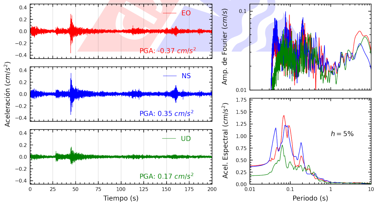
Figura A.8: Registros tiempo-historia, espectros de Fourier y de respuesta en las direcciones EO, NS y vertical de la estación COMAS. Sismo de Junin, Junin - Junin del 2024-07-05, 06:27:13 (Hora local)
