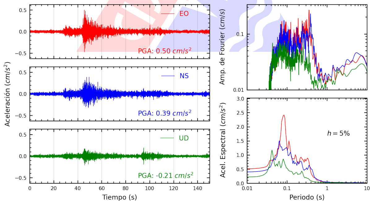
Figura A.4: Registros tiempo-historia, espectros de Fourier y de respuesta en las direcciones EO, NS y vertical de la estación DEFEN. Sismo de Junin, Junin - Junin del 2024-07-05, 06:27:13 (Hora local)
