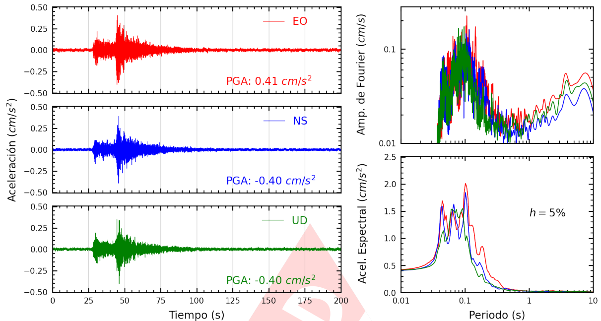
Figura A.5: Registros tiempo-historia, espectros de Fourier y de respuesta en las direcciones EO, NS y vertical de la estación AMORE. Sismo de Junin, Junin - Junin del 2024-07-05, 06:27:13 (Hora local)
