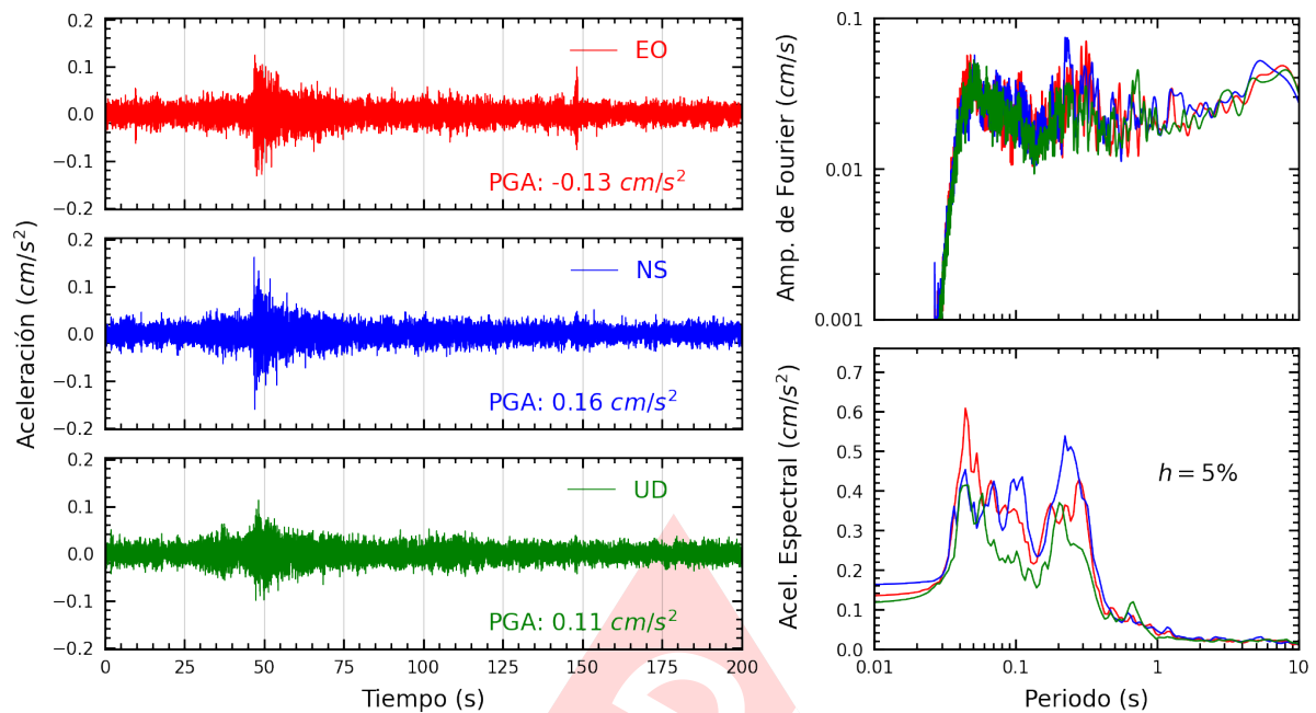
Figura A.19: Registros tiempo-historia, espectros de Fourier y de respuesta en las direcciones EO, NS y vertical de la estación CENEP. Sismo de Junin, Junin - Junin del 2024-07-05, 06:27:13 (Hora local)
