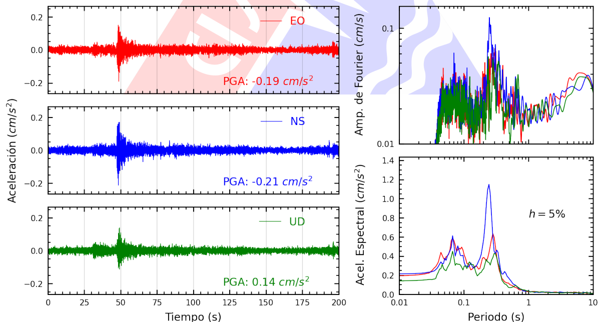
Figura A.18: Registros tiempo-historia, espectros de Fourier y de respuesta en las direcciones EO, NS y vertical de la estación SERVI. Sismo de Junin, Junin - Junin del 2024-07-05, 06:27:13 (Hora local)
