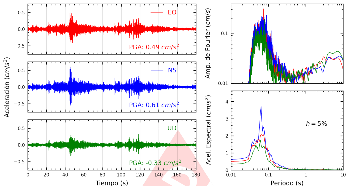
Figura A.3: Registros tiempo-historia, espectros de Fourier y de respuesta en las direcciones EO, NS y vertical de la estación JOSEO. Sismo de Junin, Junin - Junin del 2024-07-05, 06:27:13 (Hora local)
