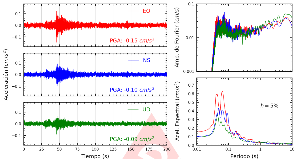
Figura A.21: Registros tiempo-historia, espectros de Fourier y de respuesta en las direcciones EO, NS y vertical de la estación UCSS. Sismo de Junin, Junin - Junin del 2024-07-05, 06:27:13 (Hora local)
