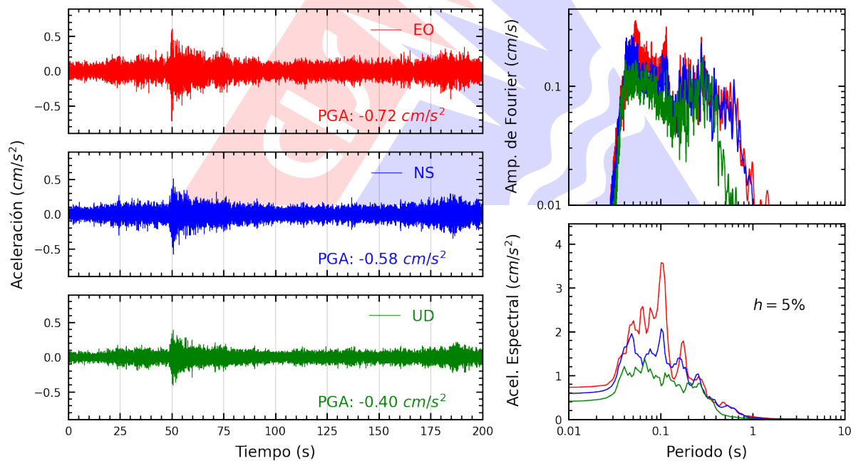
Figura A.2: Registros tiempo-historia, espectros de Fourier y de respuesta en las direcciones EO, NS y vertical de la estación UNTEL. Sismo de Junin, Junin - Junin del 2024-07-05, 06:27:13 (Hora local)
