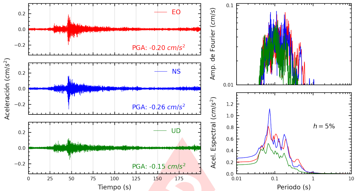
Figura A.13: Registros tiempo-historia, espectros de Fourier y de respuesta en las direcciones EO, NS y vertical de la estación JALV2. Sismo de Junin, Junin - Junin del 2024-07-05, 06:27:13 (Hora local)
