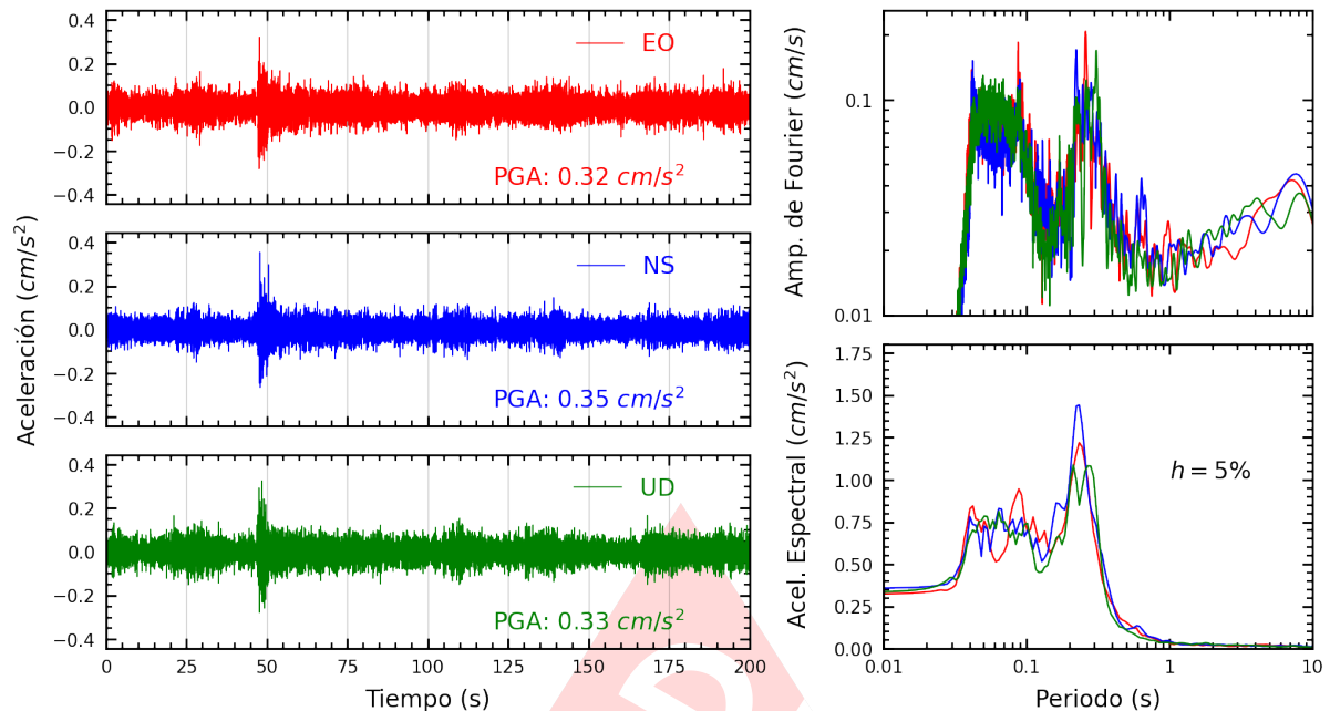
Figura A.9: Registros tiempo-historia, espectros de Fourier y de respuesta en las direcciones EO, NS y vertical de la estación URPPE. Sismo de Junin, Junin - Junin del 2024-07-05, 06:27:13 (Hora local)
