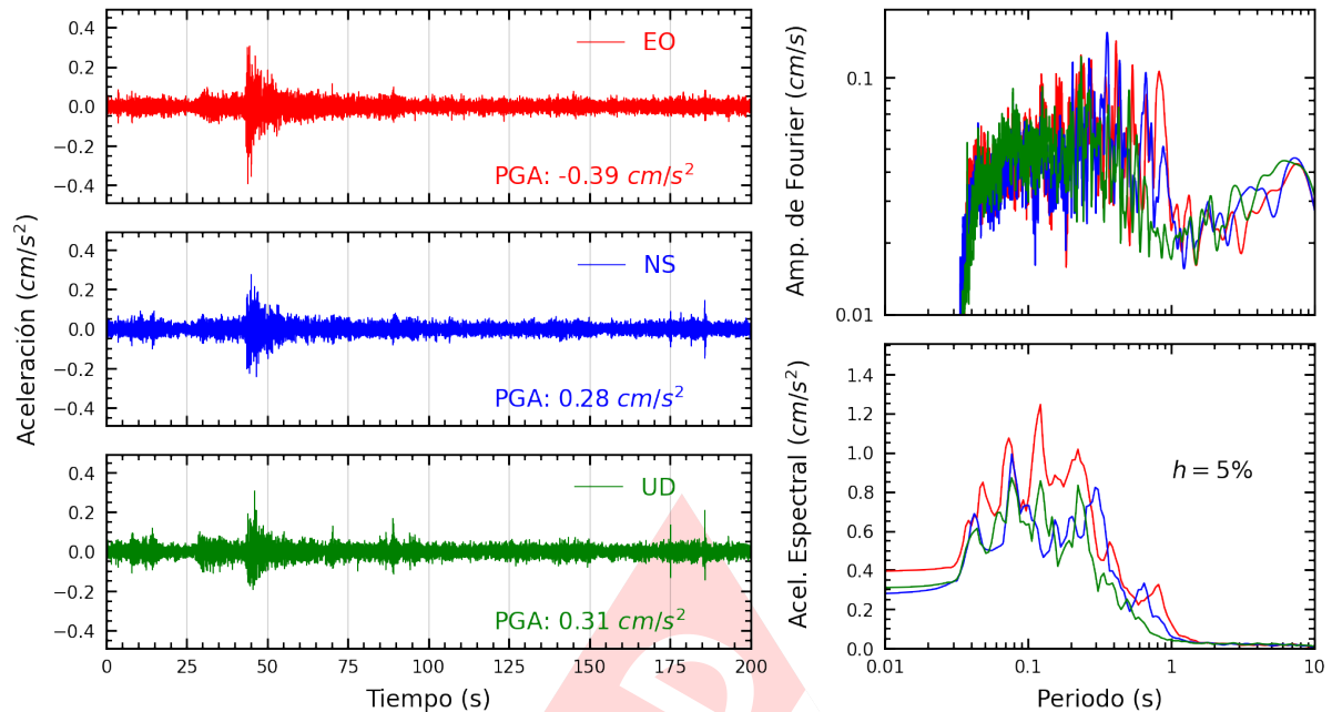
Figura A.7: Registros tiempo-historia, espectros de Fourier y de respuesta en las direcciones EO, NS y vertical de la estación UCV. Sismo de Junin, Junin - Junin del 2024-07-05, 06:27:13 (Hora local)
