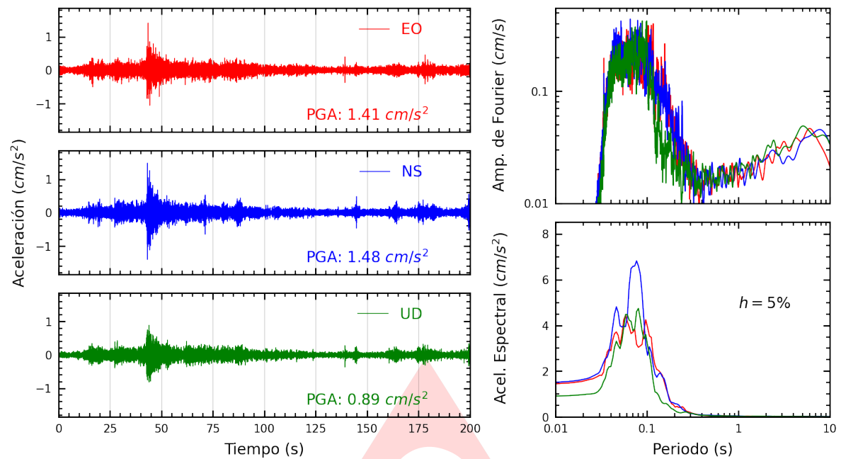
Figura A.1: Registros tiempo-historia, espectros de Fourier y de respuesta en las direcciones EO, NS y vertical de la estación SROSA. Sismo de Junin, Junin - Junin del 2024-07-05, 06:27:13 (Hora local)
