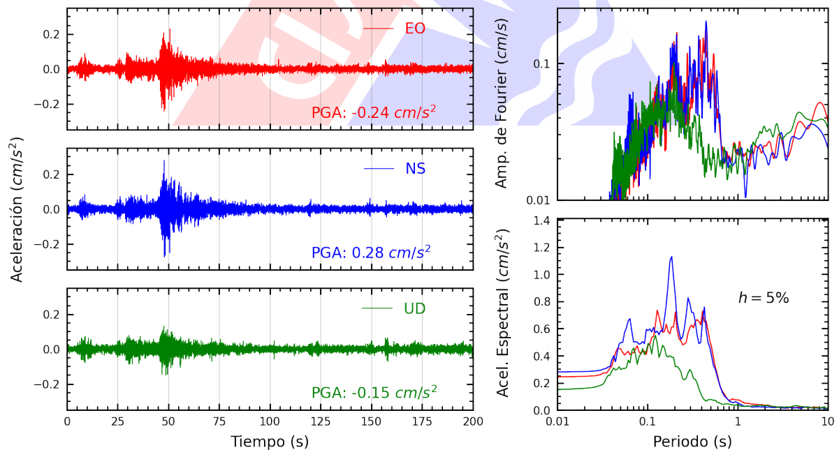
Figura A.12: Registros tiempo-historia, espectros de Fourier y de respuesta en las direcciones EO, NS y vertical de la estación VHAYA. Sismo de Junin, Junin del 2024-07-05, 06:27:13 (Hora local)
