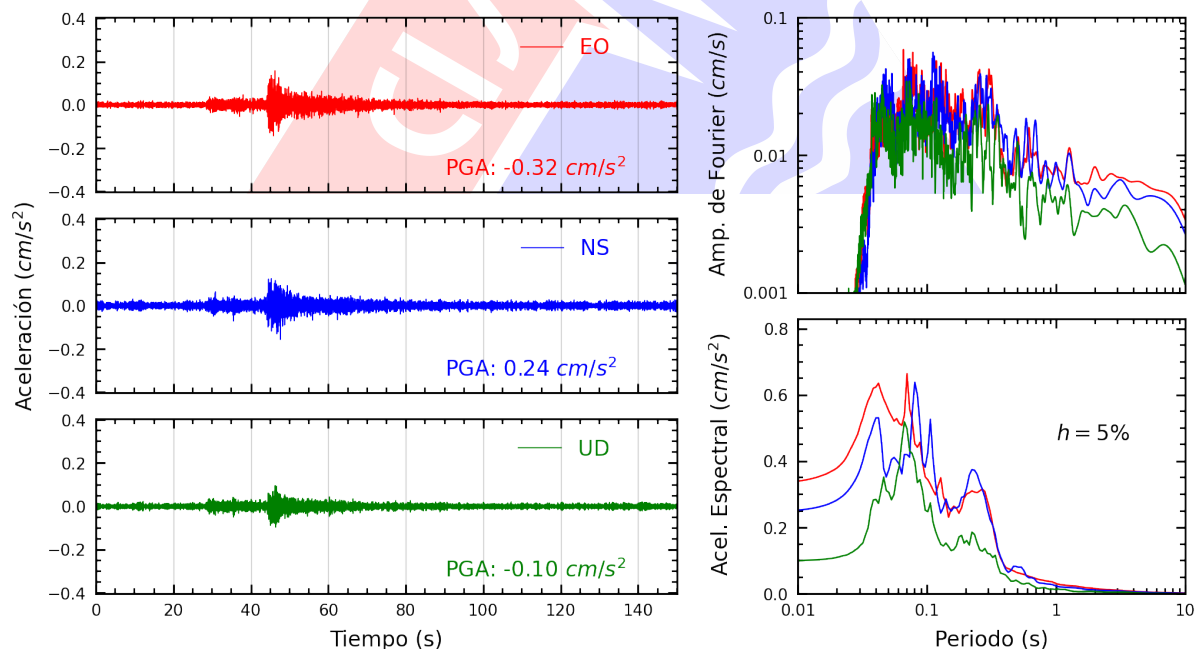
Figura A.10: Registros tiempo-historia, espectros de Fourier y de respuesta en las direcciones EO, NS y vertical de la estación ATARJ. Sismo de Junin, Junin - Junin del 2024-07-05, 06:27:13 (Hora local)
