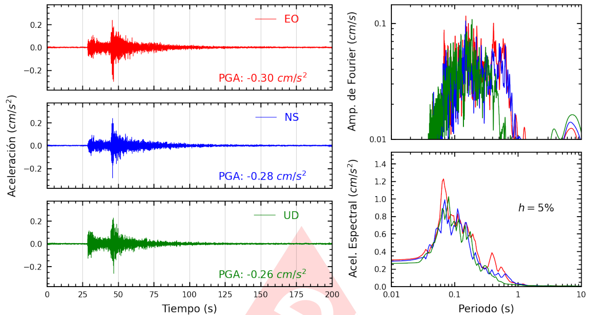
Figura A.11: Registros tiempo-historia, espectros de Fourier y de respuesta en las direcciones EO, NS y vertical de la estación CARAL. Sismo de Junin, Junin del 2024-07-05, 06:27:13 (Hora local)
