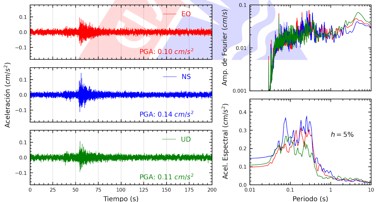
Figura A.22: Registros tiempo-historia, espectros de Fourier y de respuesta en las direcciones EO, NS y vertical de la estación UNMSM. Sismo de Junin, Junin - Junin del 2024-07-05, 06:27:13 (Hora local)
