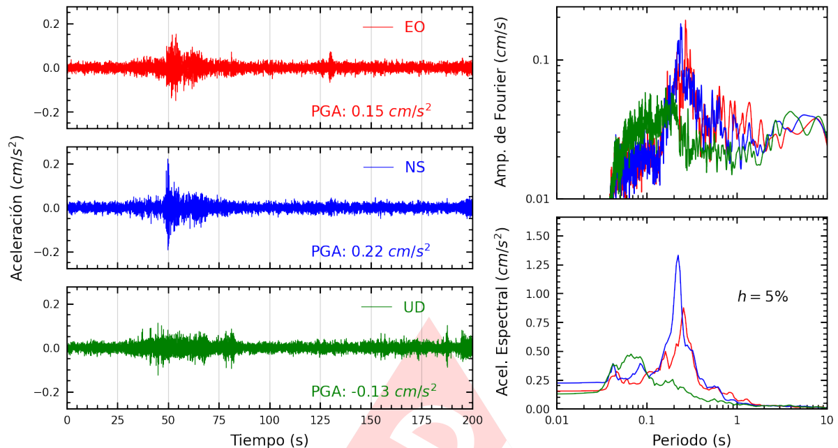
Figura A.17: Registros tiempo-historia, espectros de Fourier y de respuesta en las direcciones EO, NS y vertical de la estación DSML. Sismo de Junin, Junin - Junin del 2024-07-05, 06:27:13 (Hora local)
