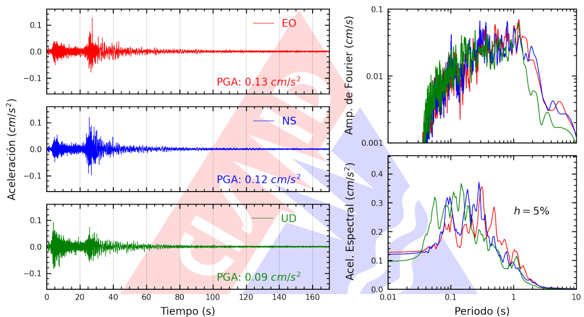
Figura A.23: Registros tiempo-historia, espectros de Fourier y de respuesta en las direcciones EO, NS y vertical de la estación UNCP. Sismo de Junin, Junin - Junin del 2024-07-05, 06:27:13 (Hora local)
