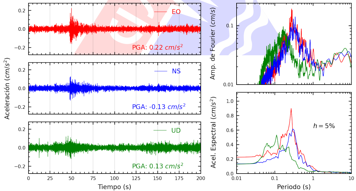
Figura A.16: Registros tiempo-historia, espectros de Fourier y de respuesta en las direcciones EO, NS y vertical de la estación ACAPU. Sismo de Junin, Junin - Junin del 2024-07-05, 06:27:13 (Hora local)
