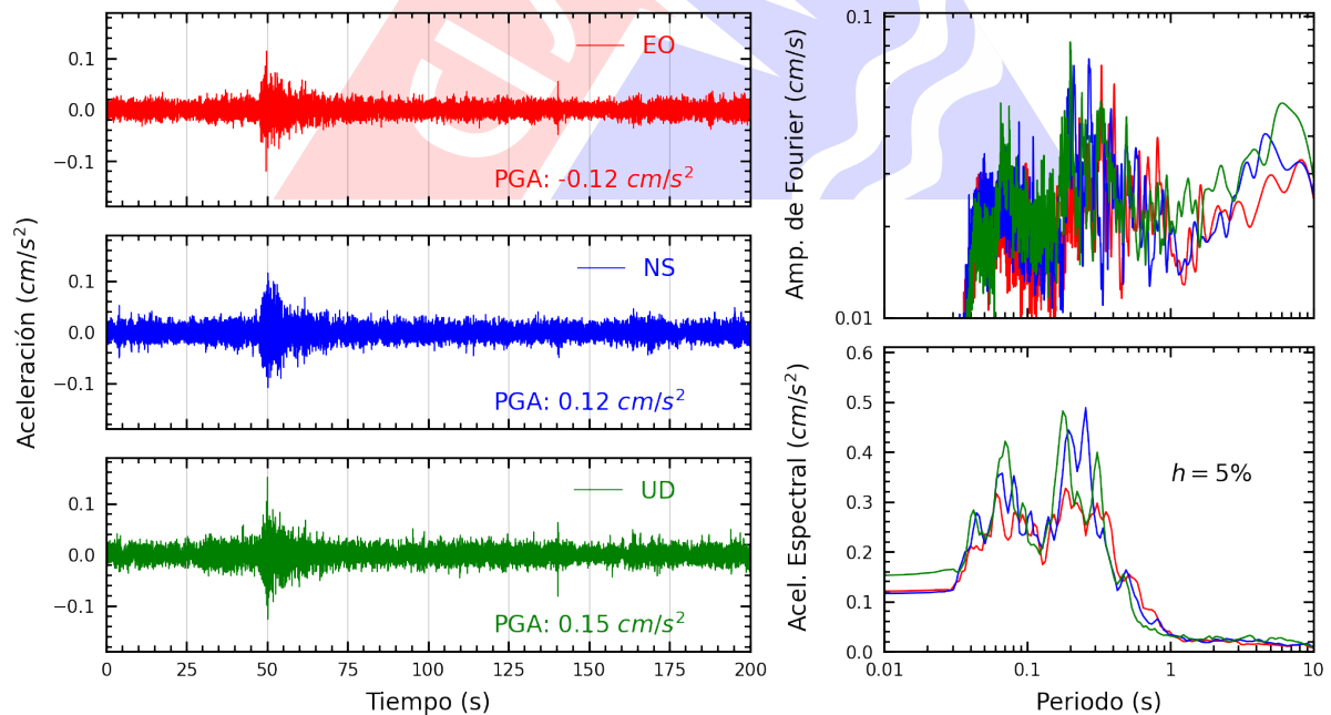
Figura A.20: Registros tiempo-historia, espectros de Fourier y de respuesta en las direcciones EO, NS y vertical de la estación UNFV. Sismo de Junin, Junin - Junin del 2024-07-05, 06:27:13 (Hora local)
