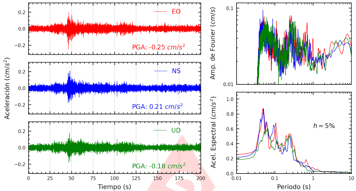
Figura A.15: Registros tiempo-historia, espectros de Fourier y de respuesta en las direcciones EO, NS y vertical de la estación IMCA. Sismo de Junin, Junin - Junin del 2024-07-05, 06:27:13 (Hora local)
