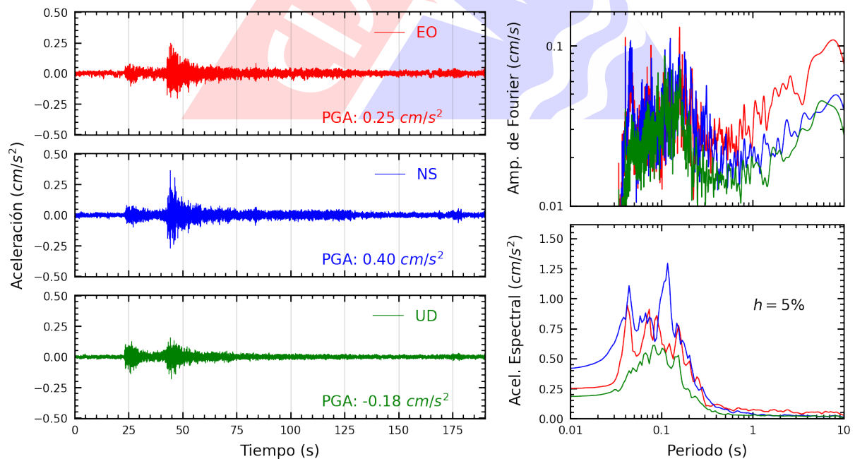
Figura A.6: Registros tiempo-historia, espectros de Fourier y de respuesta en las direcciones EO, NS y vertical de la estación UNAB. Sismo de Junin, Junin - Junin del 2024-07-05, 06:27:13 (Hora local)
