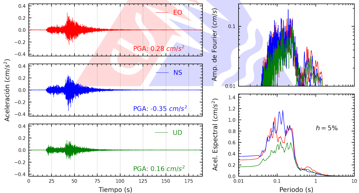
Figura A.2: Registros tiempo-historia, espectros de Fourier y de respuesta en las direcciones EO, NS y vertical de la estación UNSA. Sismo de Atico, Caraveli - Arequipa del 2024-07-05, 13:06:23 (Hora local)
