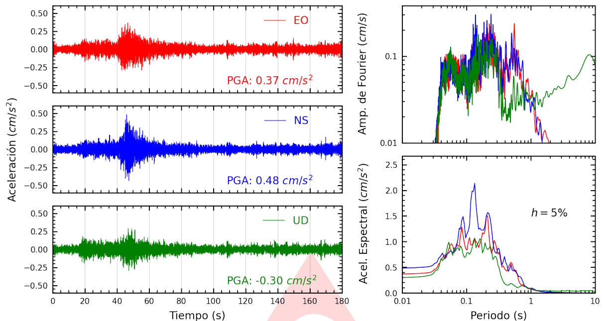
Figura A.1: Registros tiempo-historia, espectros de Fourier y de respuesta en las direcciones EO, NS y vertical de la estación SCARQ. Sismo de Atico, Caraveli - Arequipa del 2024-07-05, 13:06:23 (Hora local)
