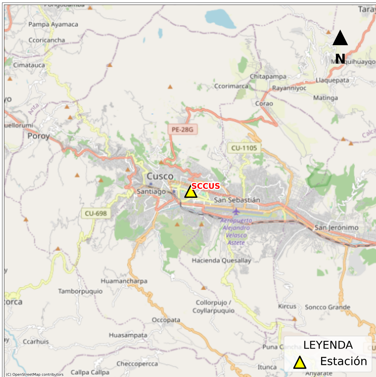
Figura 2: Mapa de ubicación de la(s) estación(es) acelerográfica(s) correspondiente(s) al Sismo de Yanaoca, Canas - Cusco del 07 de julio de 2024 a las 01:53:36 (hora local)
