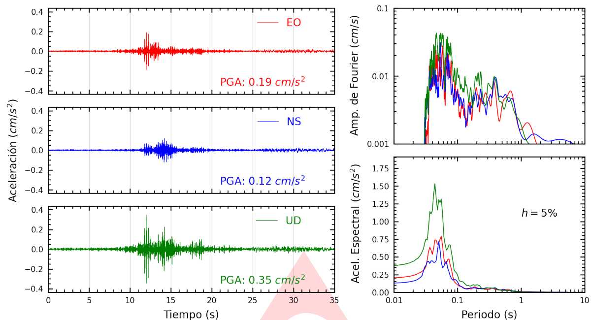
Figura A.1: Registros tiempo-historia, espectros de Fourier y de respuesta en las direcciones EO, NS y vertical de la estación SCCUS. Sismo de Yanaoca, Canas - Cusco del 2024-07-07, 01:53:36 (Hora local)
