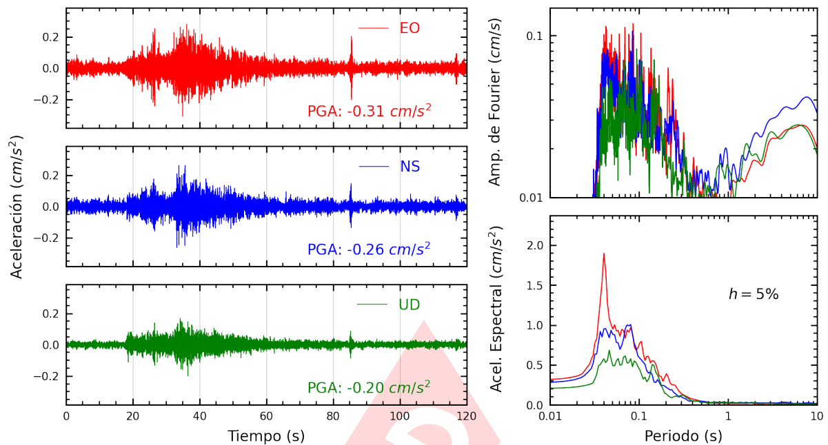
Figura A.23: Registros tiempo-historia, espectros de Fourier y de respuesta en las direcciones EO, NS y vertical de la estación CEPRE. Sismo de San Vicente De Cañete, Cañete - Lima del 2024-07-10, 20:41:16 (Hora local)
