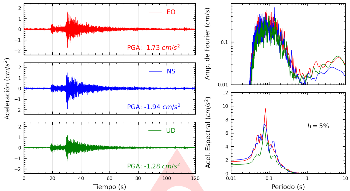
Figura A.1: Registros tiempo-historia, espectros de Fourier y de respuesta en las direcciones EO, NS y vertical de la estación PUNTA. Sismo de San Vicente De Cañete, Cañete - Lima del 2024-07-10, 20:41:16 (Hora local)
