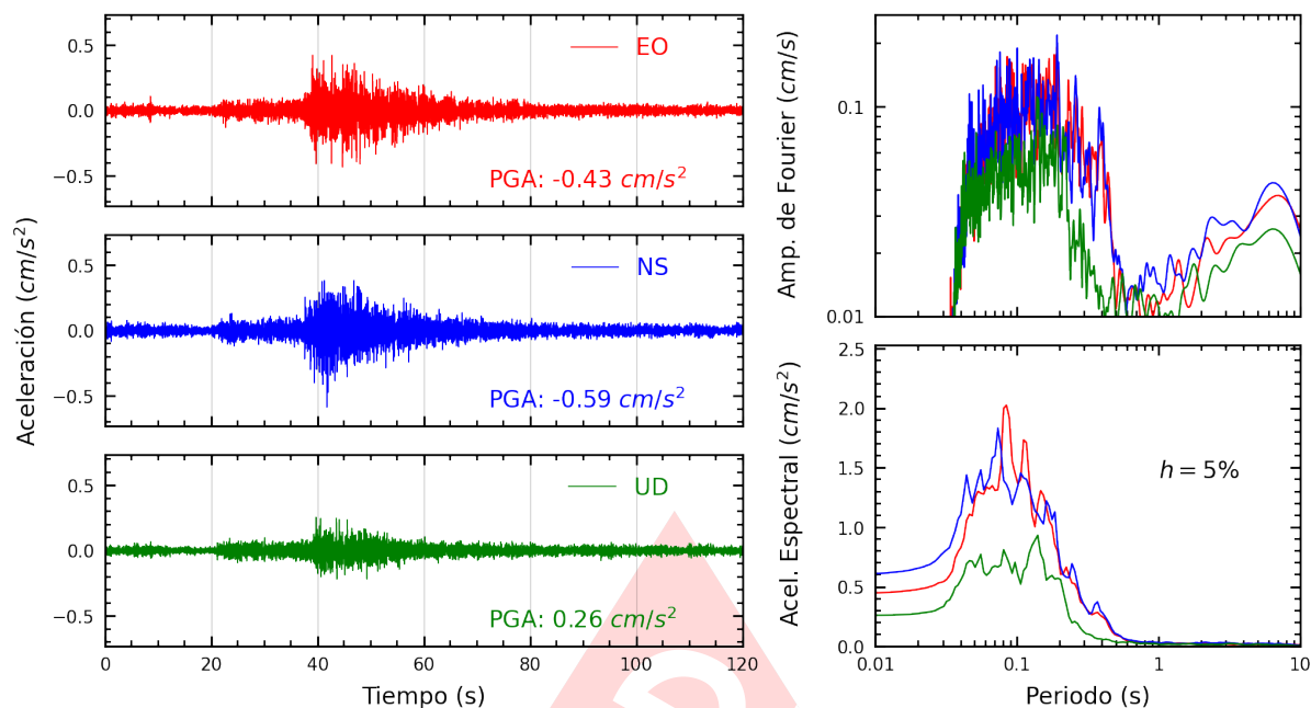
Figura A.13: Registros tiempo-historia, espectros de Fourier y de respuesta en las direcciones EO, NS y vertical de la estación DEFEN. Sismo de San Vicente De Cañete, Cañete - Lima del 2024-07-10, 20:41:16 (Hora local)
