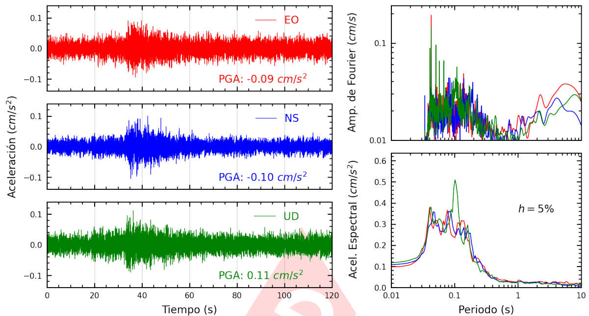
Figura A.33: Registros tiempo-historia, espectros de Fourier y de respuesta en las direcciones EO, NS y vertical de la estación BONDY. Sismo de San Vicente De Cañete, Cañete - Lima del 2024-07-10, 20:41:16 (Hora local)
