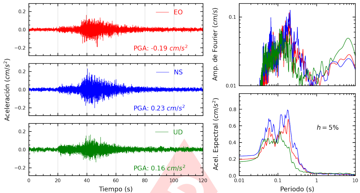
Figura A.25: Registros tiempo-historia, espectros de Fourier y de respuesta en las direcciones EO, NS y vertical de la estación VHAYA. Sismo de San Vicente De Cañete, Cañete - Lima del 2024-07-10, 20:41:16 (Hora local)
