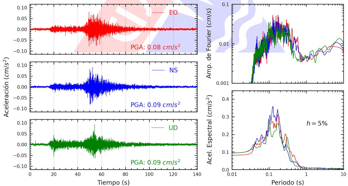
Figura A.34: Registros tiempo-historia, espectros de Fourier y de respuesta en las direcciones EO, NS y vertical de la estación CARAL. Sismo de San Vicente De Cañete, Cañete - Lima del 2024-07-10, 20:41:16 (Hora local)
