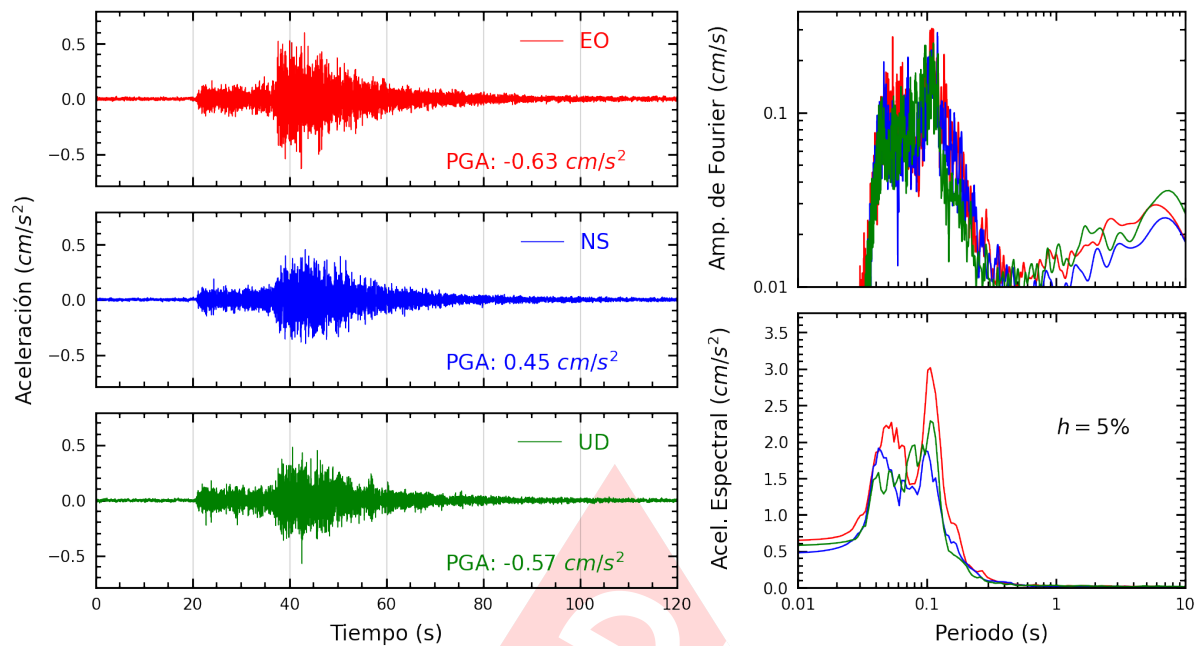
Figura A.11: Registros tiempo-historia, espectros de Fourier y de respuesta en las direcciones EO, NS y vertical de la estación AMORE. Sismo de San Vicente De Cañete, Cañete - Lima del 2024-07-10, 20:41:16 (Hora local)
