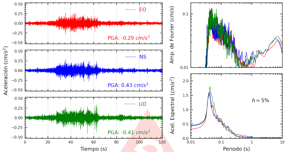
Figura A.15: Registros tiempo-historia, espectros de Fourier y de respuesta en las direcciones EO, NS y vertical de la estación USMP. Sismo de San Vicente De Cañete, Cañete - Lima del 2024-07-10, 20:41:16 (Hora local)
