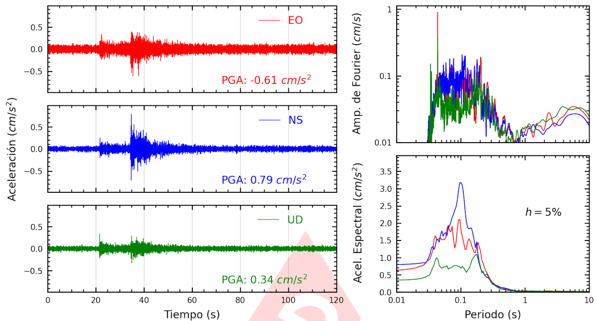
Figura A.7: Registros tiempo-historia, espectros de Fourier y de respuesta en las direcciones EO, NS y vertical de la estación UPCVI. Sismo de San Vicente De Cañete, Cañete - Lima del 2024-07-10, 20:41:16 (Hora local)
