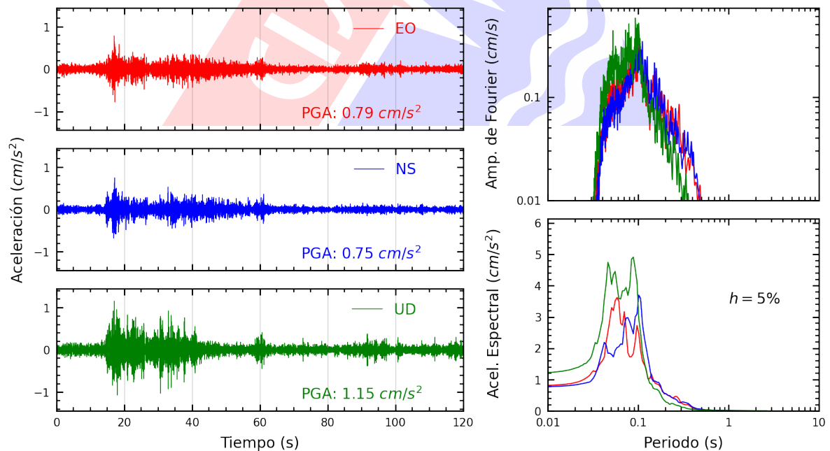
Figura A.4: Registros tiempo-historia, espectros de Fourier y de respuesta en las direcciones EO, NS y vertical de la estación SCOLI. Sismo de San Vicente De Cañete, Cañete - Lima del 2024-07-10, 20:41:16 (Hora local)
