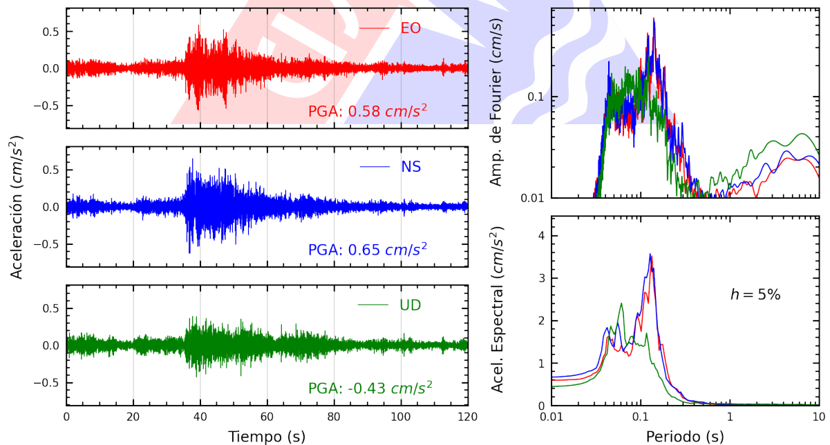
Figura A.10: Registros tiempo-historia, espectros de Fourier y de respuesta en las direcciones EO, NS y vertical de la estación CARAB. Sismo de San Vicente De Cañete, Cañete - Lima del 2024-07-10, 20:41:16 (Hora local)
