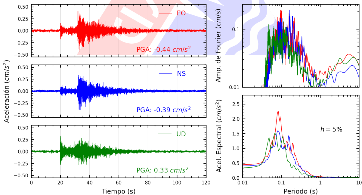
Figura A.14: Registros tiempo-historia, espectros de Fourier y de respuesta en las direcciones EO, NS y vertical de la estación USILP. Sismo de San Vicente De Cañete, Cañete - Lima del 2024-07-10, 20:41:16 (Hora local)
