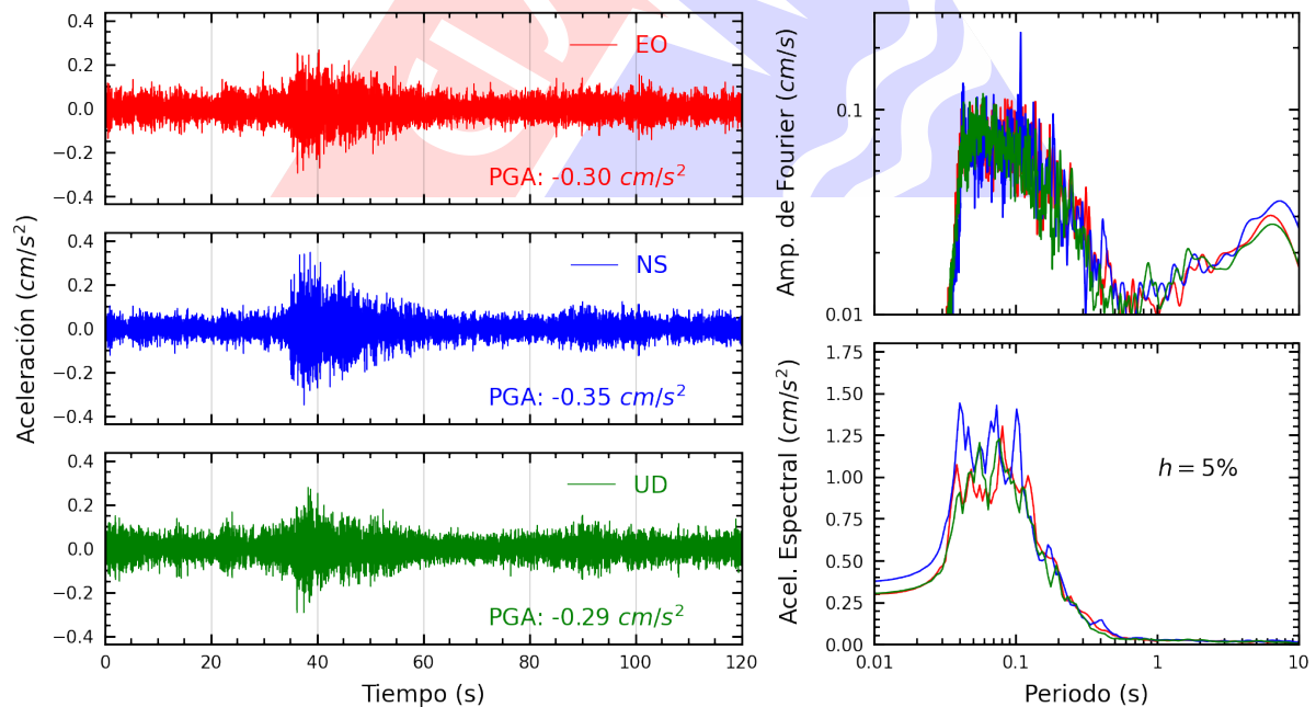
Figura A.18: Registros tiempo-historia, espectros de Fourier y de respuesta en las direcciones EO, NS y vertical de la estación URPE. Sismo de San Vicente De Cañete, Cañete - Lima del 2024-07-10, 20:41:16 (Hora local)
