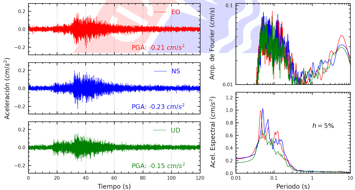
Figura A.26: Registros tiempo-historia, espectros de Fourier y de respuesta en las direcciones EO, NS y vertical de la estación CENEP. Sismo de San Vicente De Cañete, Cañete - Lima del 2024-07-10, 20:41:16 (Hora local)
