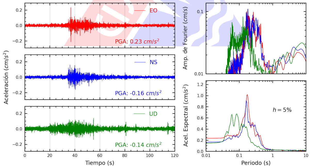
Figura A.24: Registros tiempo-historia, espectros de Fourier y de respuesta en las direcciones EO, NS y vertical de la estación ACAPU. Sismo de San Vicente De Cañete, Cañete - Lima del 2024-07-10, 20:41:16 (Hora local)
