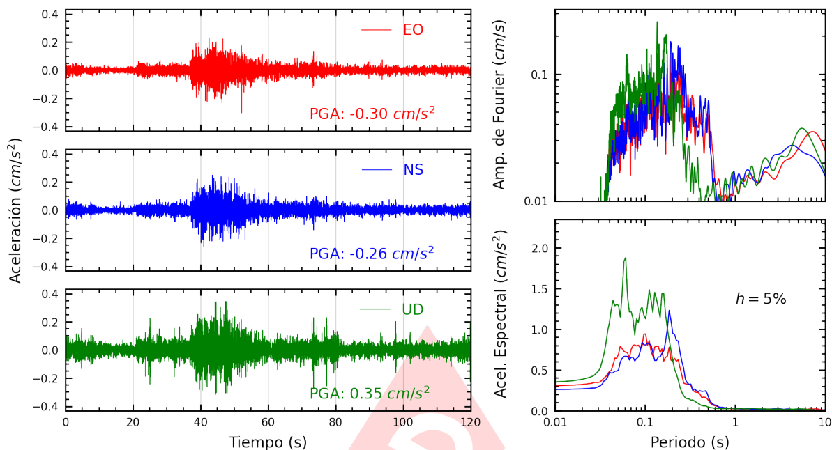
Figura A.19: Registros tiempo-historia, espectros de Fourier y de respuesta en las direcciones EO, NS y vertical de la estación MDPP. Sismo de San Vicente De Cañete, Cañete - Lima del 2024-07-10, 20:41:16 (Hora local)
