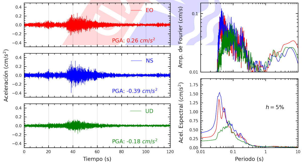
Figura A.16: Registros tiempo-historia, espectros de Fourier y de respuesta en las direcciones EO, NS y vertical de la estación COMAS. Sismo de San Vicente De Cañete, Cañete - Lima del 2024-07-10, 20:41:16 (Hora local)
