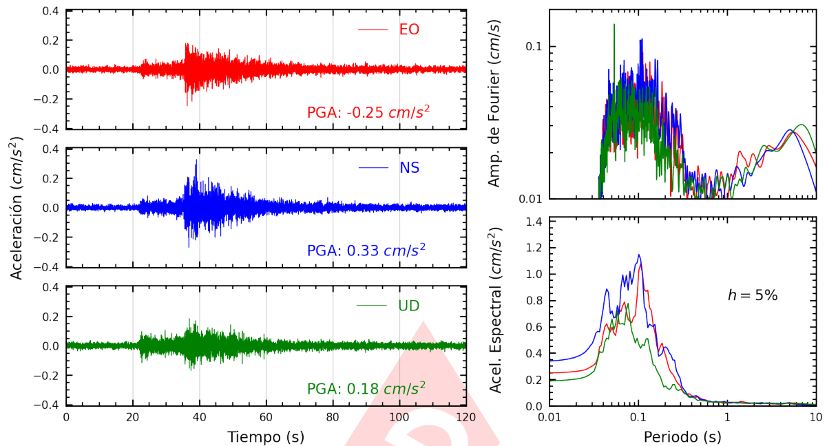
Figura A.21: Registros tiempo-historia, espectros de Fourier y de respuesta en las direcciones EO, NS y vertical de la estación SERVI. Sismo de San Vicente De Cañete, Cañete - Lima del 2024-07-10, 20:41:16 (Hora local)
