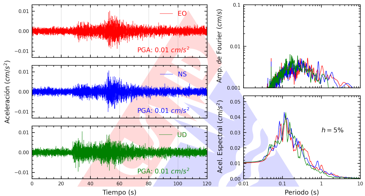
Figura A.35: Registros tiempo-historia, espectros de Fourier y de respuesta en las direcciones EO, NS y vertical de la estación UNCP. Sismo de San Vicente De Cañete, Cañete - Lima del 2024-07-10, 20:41:16 (Hora local)
