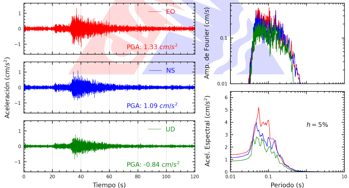
Figura A.2: Registros tiempo-historia, espectros de Fourier y de respuesta en las direcciones EO, NS y vertical de la estación UNTEL. Sismo de San Vicente De Cañete, Cañete - Lima del 2024-07-10, 20:41:16 (Hora local)
