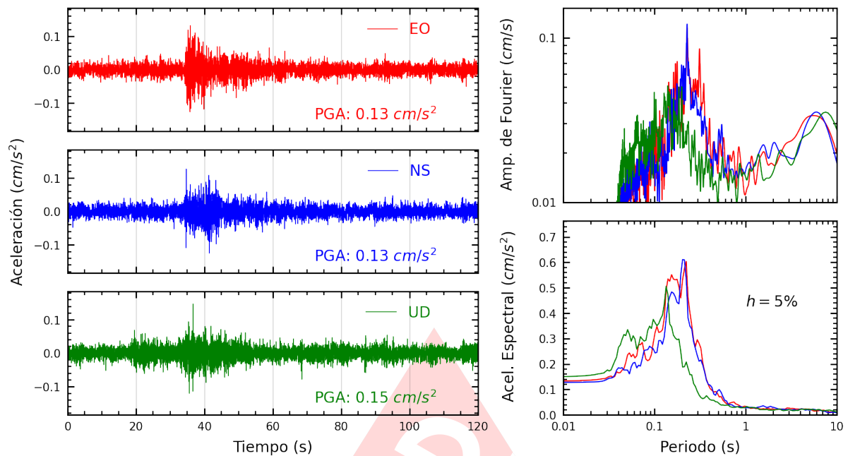
Figura A.31: Registros tiempo-historia, espectros de Fourier y de respuesta en las direcciones EO, NS y vertical de la estación DSMI. Sismo de San Vicente De Cañete, Cañete - Lima del 2024-07-10, 20:41:16 (Hora local)
