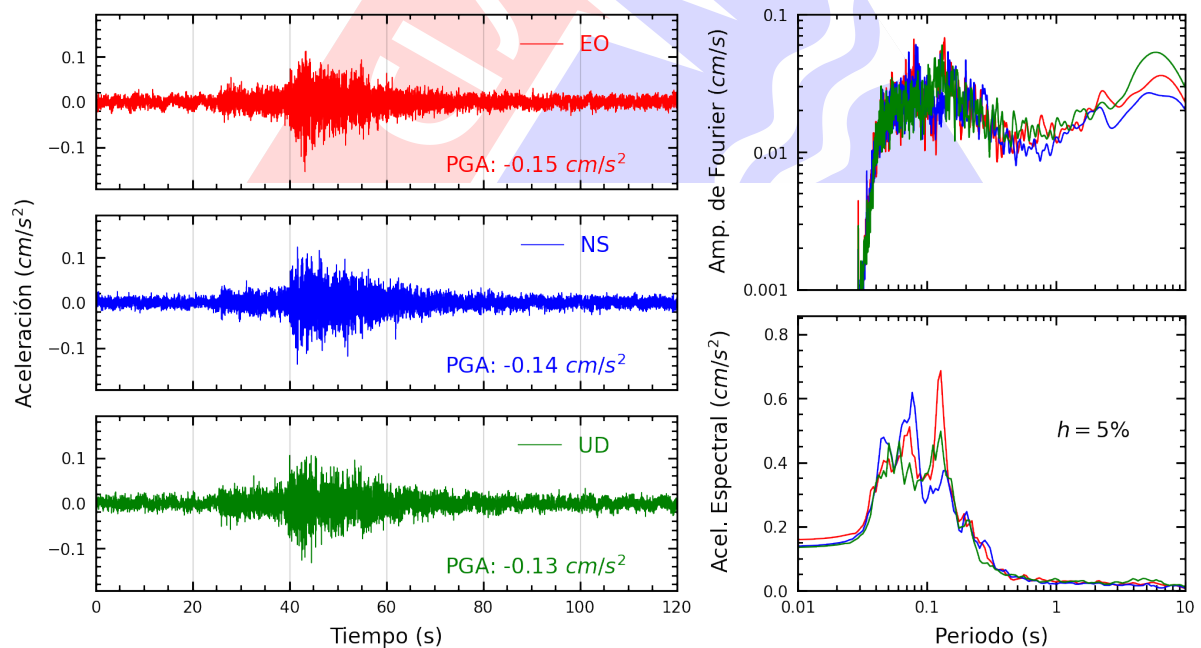
Figura A.30: Registros tiempo-historia, espectros de Fourier y de respuesta en las direcciones EO, NS y vertical de la estación UNMSM. Sismo de San Vicente De Cañete, Cañete - Lima del 2024-07-10, 20:41:16 (Hora local)
