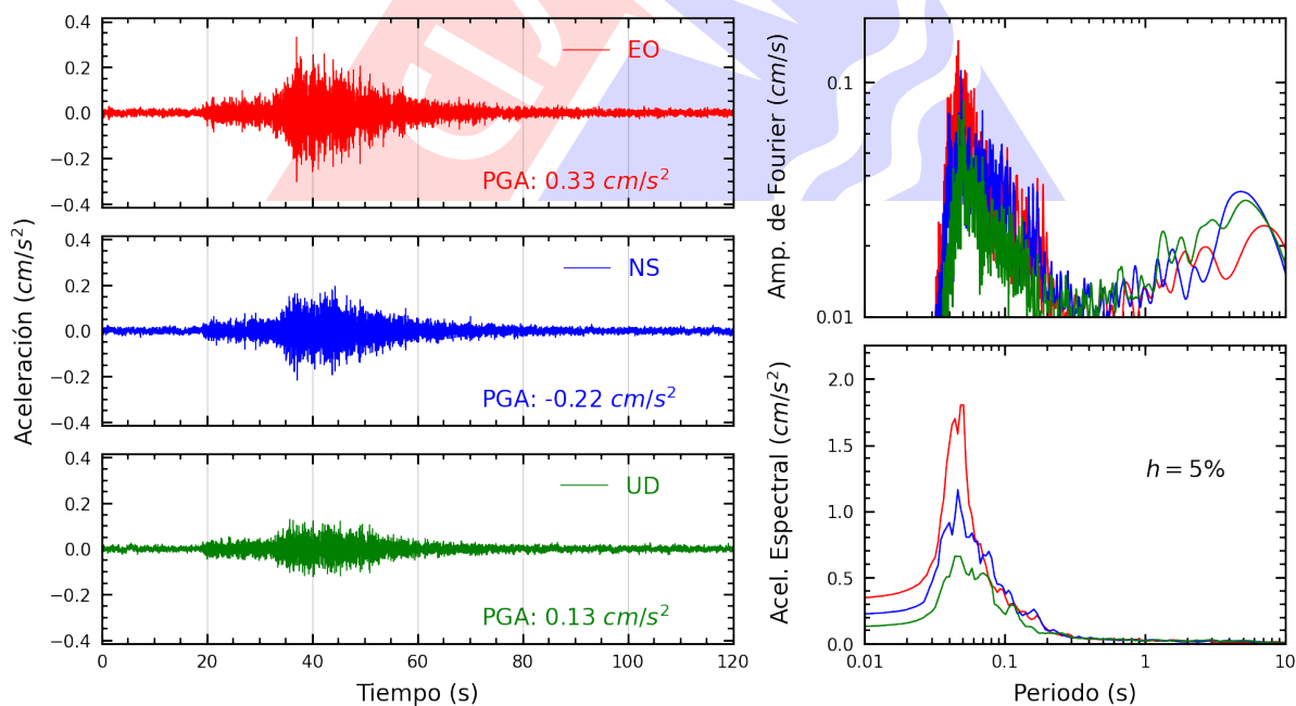
Figura A.20: Registros tiempo-historia, espectros de Fourier y de respuesta en las direcciones EO, NS y vertical de la estación UCSS. Sismo de San Vicente De Cañete, Cañete - Lima del 2024-07-10, 20:41:16 (Hora local)
