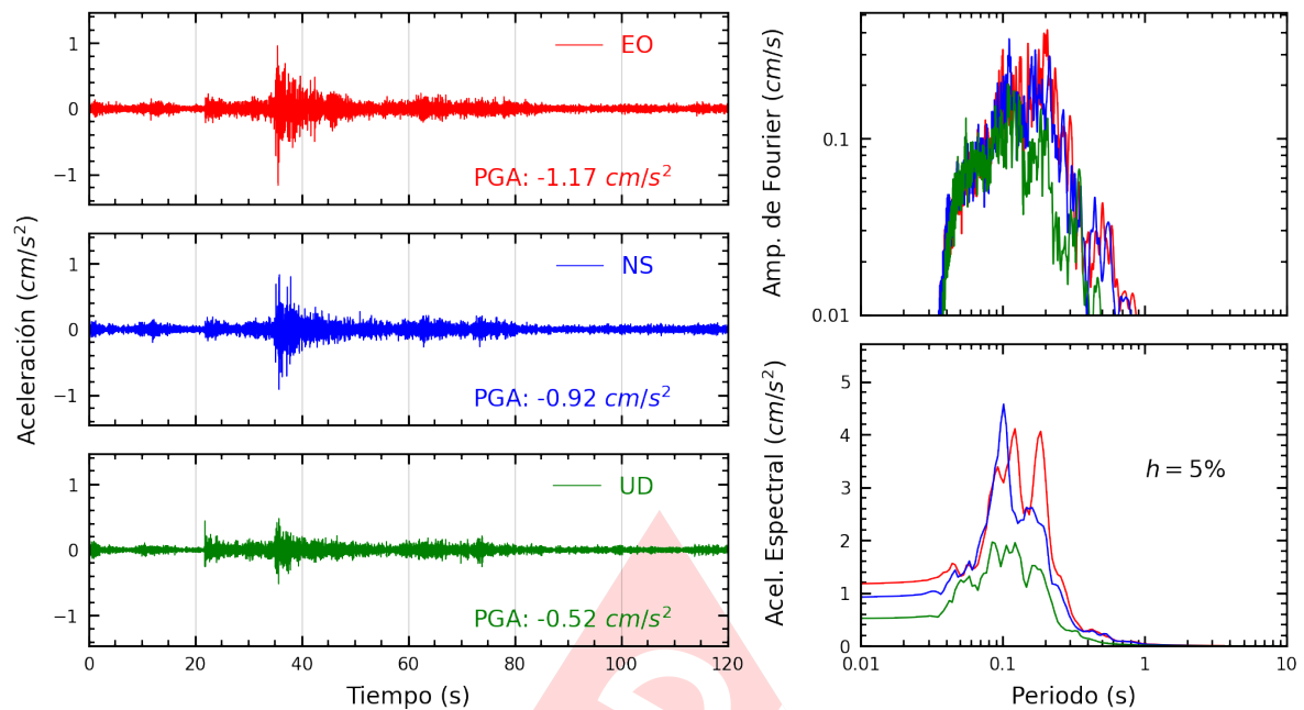
Figura A.3: Registros tiempo-historia, espectros de Fourier y de respuesta en las direcciones EO, NS y vertical de la estación SCCHO. Sismo de San Vicente De Cañete, Cañete - Lima del 2024-07-10, 20:41:16 (Hora local)
