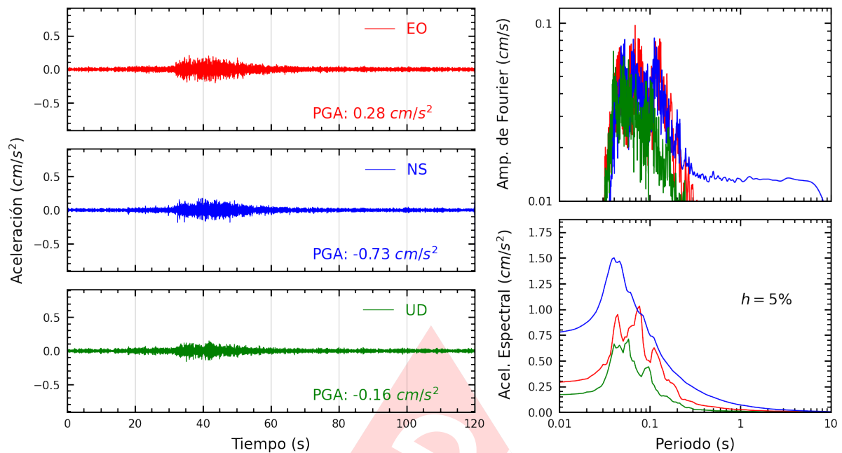
Figura A.9: Registros tiempo-historia, espectros de Fourier y de respuesta en las direcciones EO, NS y vertical de la estación ATARJ. Sismo de San Vicente De Cañete, Cañete - Lima del 2024-07-10, 20:41:16 (Hora local)
