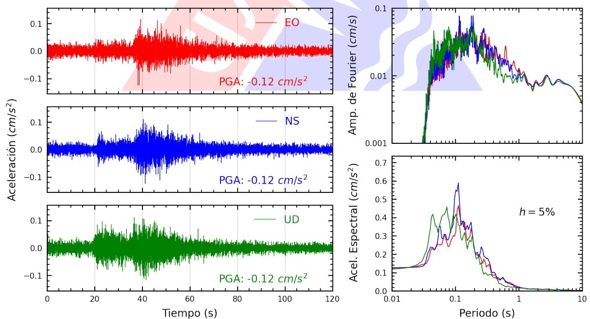
Figura A.32: Registros tiempo-historia, espectros de Fourier y de respuesta en las direcciones EO, NS y vertical de la estación UNICA. Sismo de San Vicente De Cañete, Cañete - Lima del 2024-07-10, 20:41:16 (Hora local)
