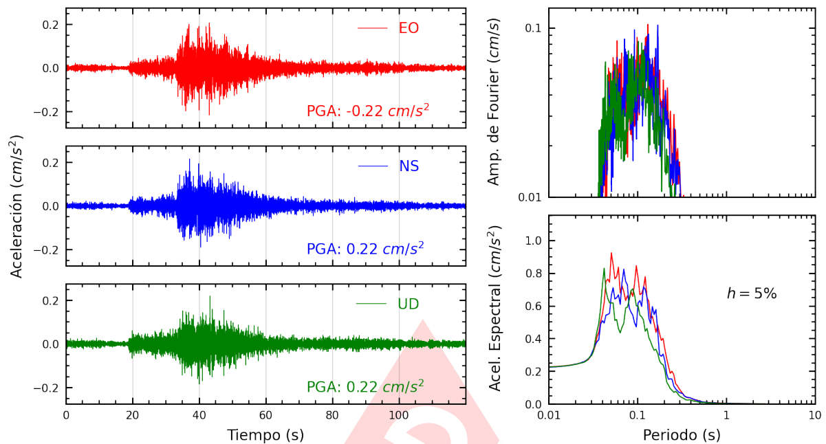
Figura A.27: Registros tiempo-historia, espectros de Fourier y de respuesta en las direcciones EO, NS y vertical de la estación JALV2. Sismo de San Vicente De Cañete, Cañete - Lima del 2024-07-10, 20:41:16 (Hora local)
