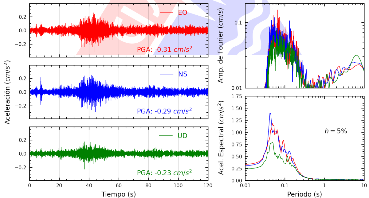
Figura A.22: Registros tiempo-historia, espectros de Fourier y de respuesta en las direcciones EO, NS y vertical de la estación FICPE. Sismo de San Vicente De Cañete, Cañete - Lima del 2024-07-10, 20:41:16 (Hora local)
