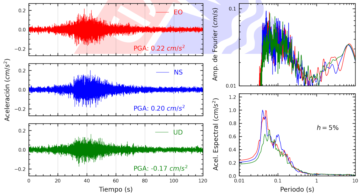
Figura A.28: Registros tiempo-historia, espectros de Fourier y de respuesta en las direcciones EO, NS y vertical de la estación IMCA. Sismo de San Vicente De Cañete, Cañete - Lima del 2024-07-10, 20:41:16 (Hora local)
