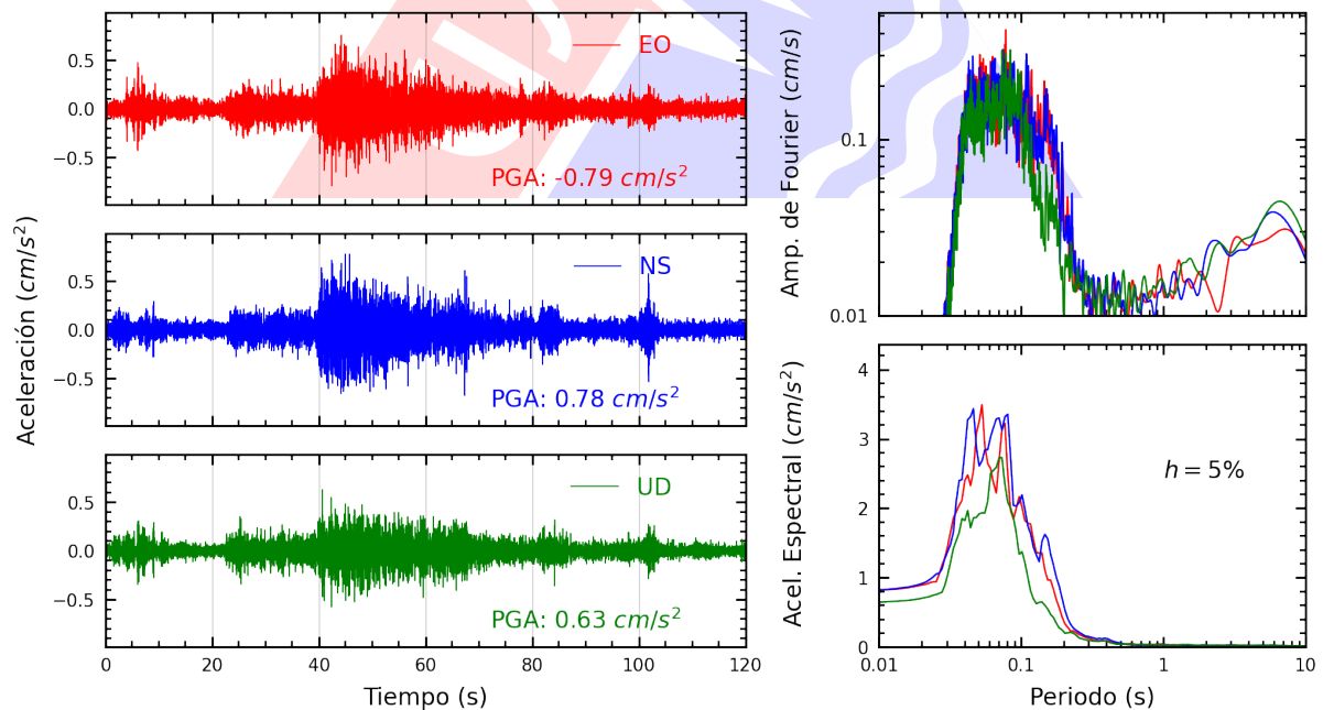
Figura A.6: Registros tiempo-historia, espectros de Fourier y de respuesta en las direcciones EO, NS y vertical de la estación SROSA. Sismo de San Vicente De Cañete, Cañete - Lima del 2024-07-10, 20:41:16 (Hora local)
