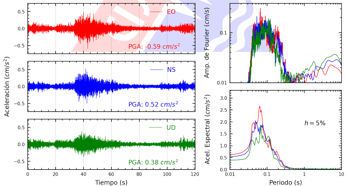
Figura A.12: Registros tiempo-historia, espectros de Fourier y de respuesta en las direcciones EO, NS y vertical de la estación INDEP. Sismo de San Vicente De Cañete, Cañete - Lima del 2024-07-10, 20:41:16 (Hora local)
