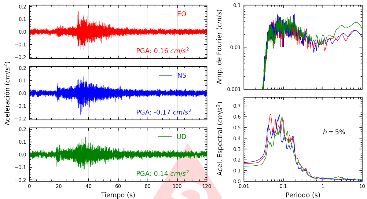
Figura A.29: Registros tiempo-historia, espectros de Fourier y de respuesta en las direcciones EO, NS y vertical de la estación UNFV. Sismo de San Vicente De Cañete, Cañete - Lima del 2024-07-10, 20:41:16 (Hora local)
