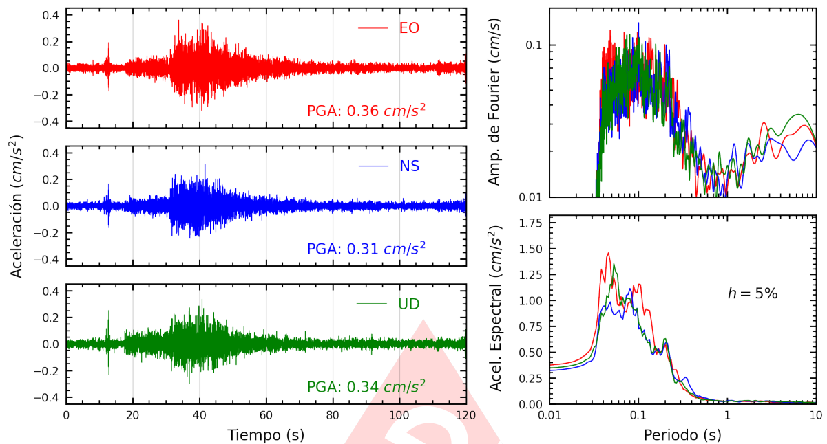
Figura A.17: Registros tiempo-historia, espectros de Fourier y de respuesta en las direcciones EO, NS y vertical de la estación UCV. Sismo de San Vicente De Cañete, Cañete - Lima del 2024-07-10, 20:41:16 (Hora local)
