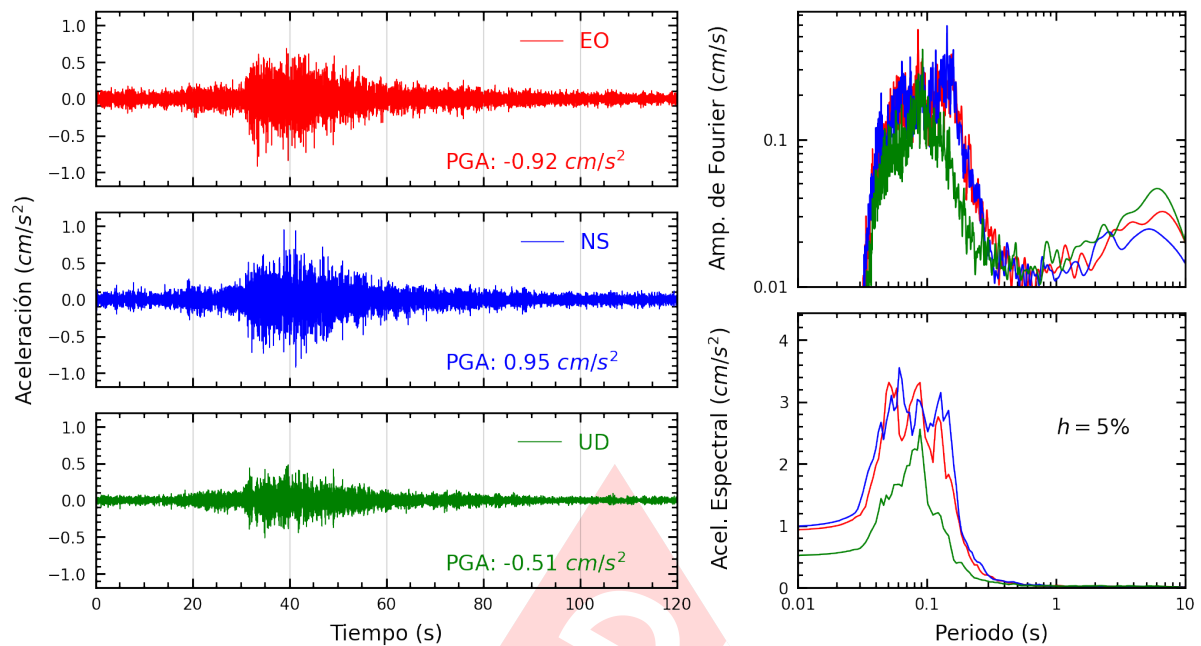
Figura A.5: Registros tiempo-historia, espectros de Fourier y de respuesta en las direcciones EO, NS y vertical de la estación USILM. Sismo de San Vicente De Cañete, Cañete - Lima del 2024-07-10, 20:41:16 (Hora local)
