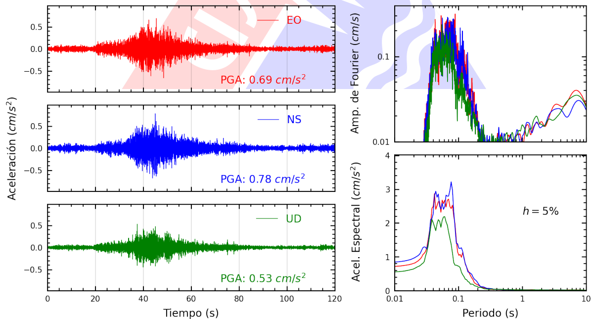
Figura A.8: Registros tiempo-historia, espectros de Fourier y de respuesta en las direcciones EO, NS y vertical de la estación JOSEO. Sismo de San Vicente De Cañete, Cañete - Lima del 2024-07-10, 20:41:16 (Hora local)
