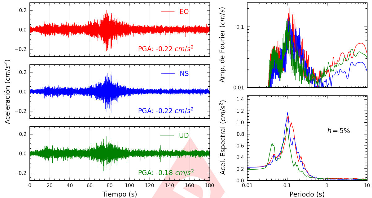
Figura A.3: Registros tiempo-historia, espectros de Fourier y de respuesta en las direcciones EO, NS y vertical de la estación AMORE. Sismo de Yauca, Caraveli - Arequipa del 2024-07-11, 12:55:26 (Hora local)
