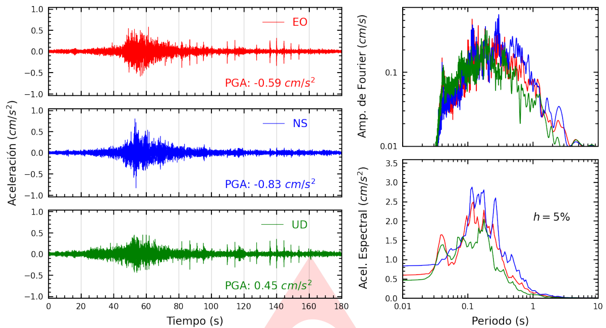
Figura A.1: Registros tiempo-historia, espectros de Fourier y de respuesta en las direcciones EO, NS y vertical de la estación UNICA. Sismo de Yauca, Caraveli - Arequipa del 2024-07-11, 12:55:26 (Hora local)
