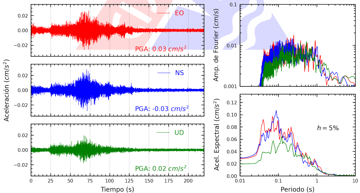
Figura A.4: Registros tiempo-historia, espectros de Fourier y de respuesta en las direcciones EO, NS y vertical de la estación UNSA. Sismo de Yauca, Caraveli - Arequipa del 2024-07-11, 12:55:26 (Hora local)
