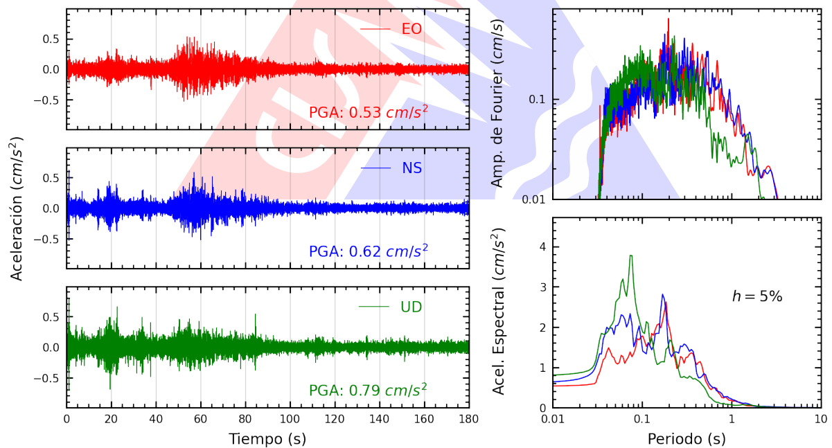
Figura A.2: Registros tiempo-historia, espectros de Fourier y de respuesta en las direcciones EO, NS y vertical de la estación SCICA. Sismo de Yauca, Caraveli - Arequipa del 2024-07-11, 12:55:26 (Hora local)
