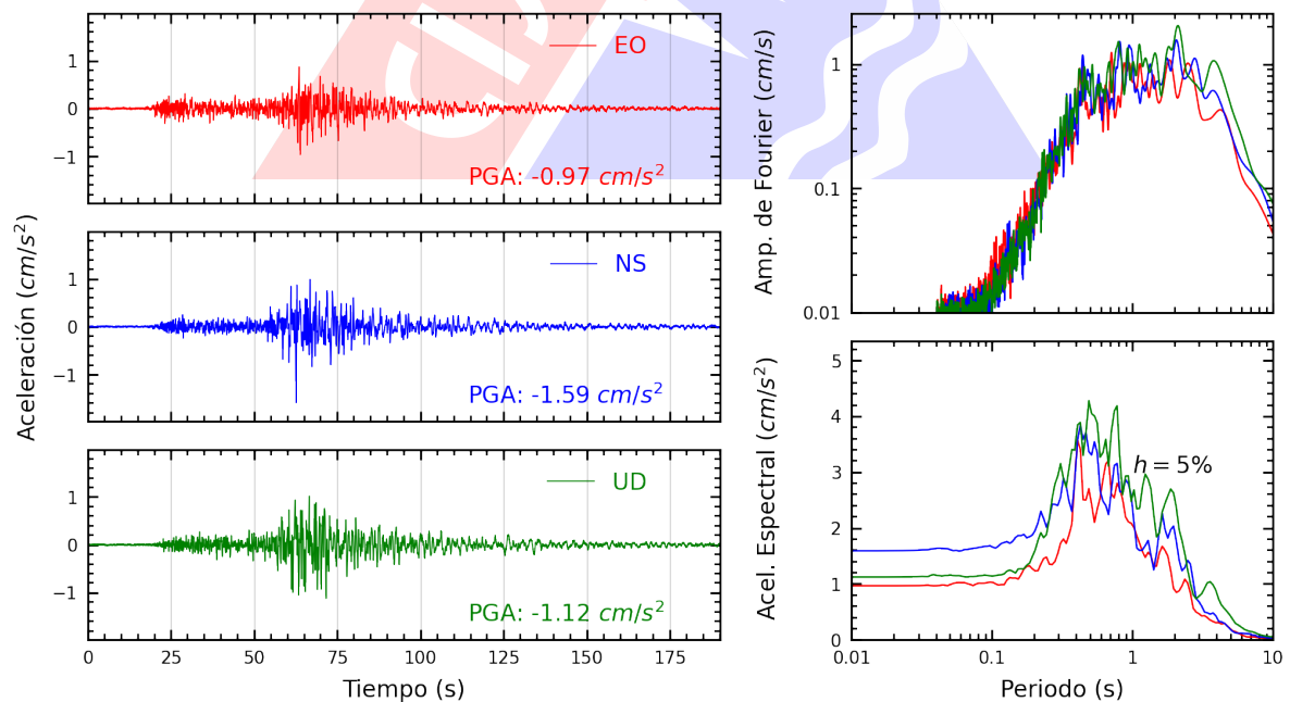
Figura A.4: Registros tiempo-historia, espectros de Fourier y de respuesta en las direcciones EO, NS y vertical de la estación UNSCH. Sismo de Lomas, Caraveli - Arequipa del 2024-07-12, 04:30:32 (Hora local)
