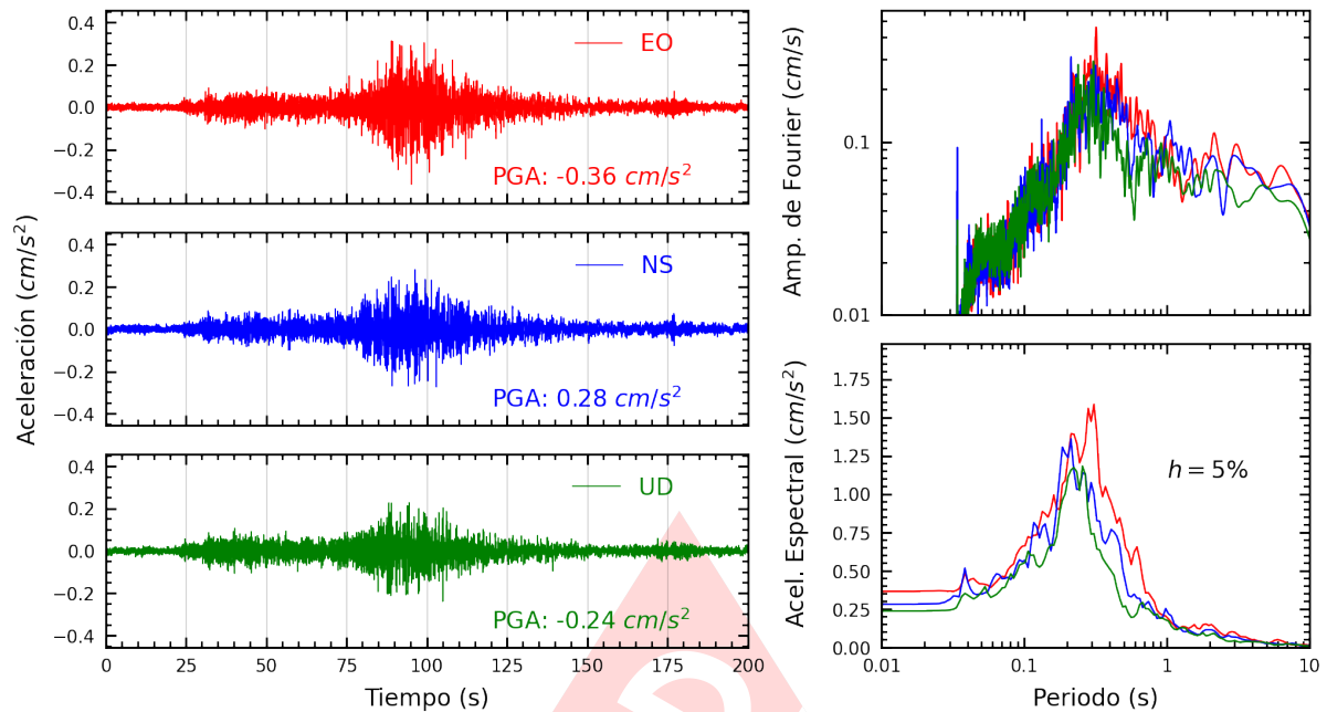
Figura A.31: Registros tiempo-historia, espectros de Fourier y de respuesta en las direcciones EO, NS y vertical de la estación USMP. Sismo de Lomas, Caraveli - Arequipa del 2024-07-12, 04:30:32 (Hora local)
