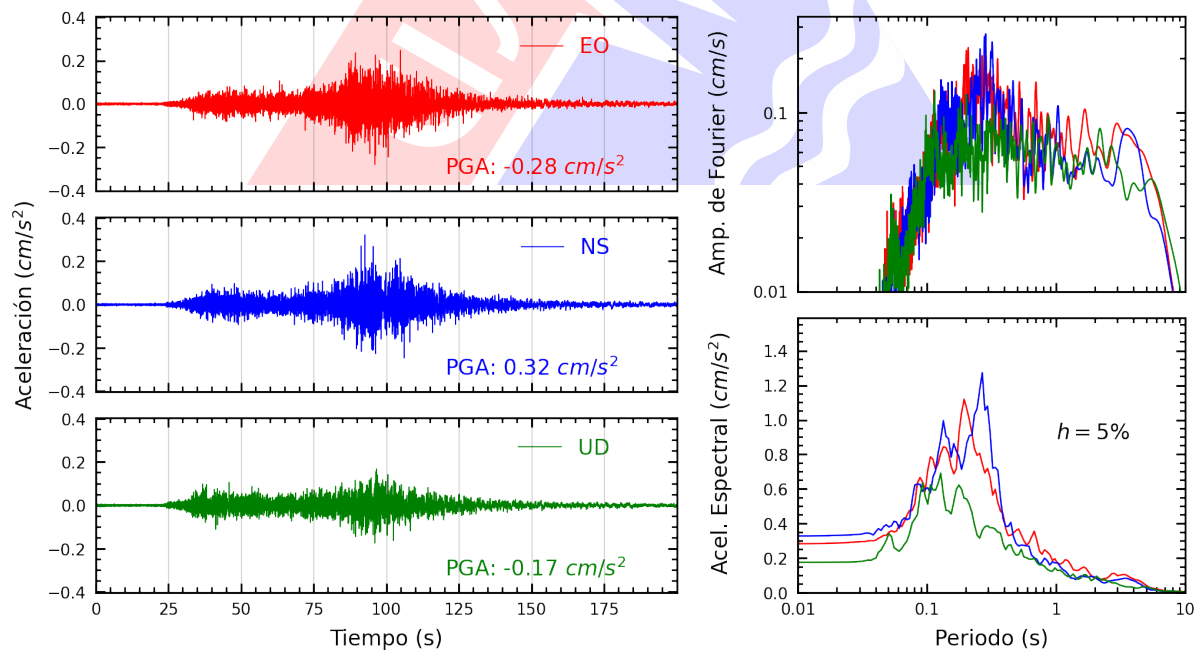
Figura A.36: Registros tiempo-historia, espectros de Fourier y de respuesta en las direcciones EO, NS y vertical de la estación JALV2. Sismo de Lomas, Caraveli - Arequipa del 2024-07-12, 04:30:32 (Hora local)
