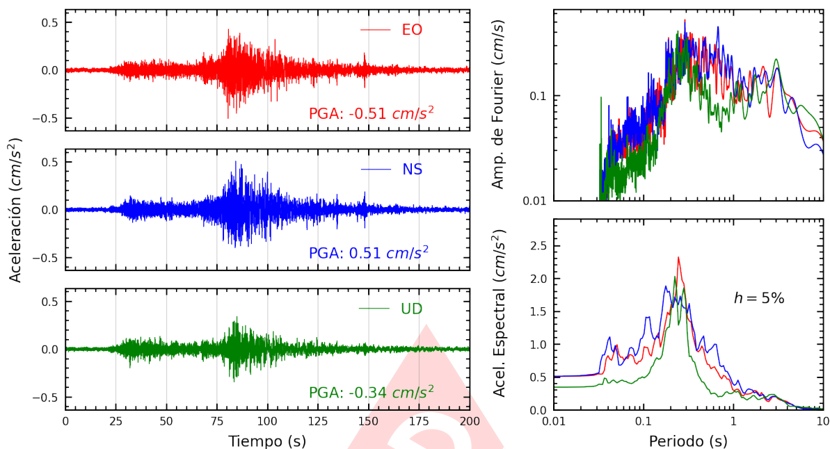
Figura A.23: Registros tiempo-historia, espectros de Fourier y de respuesta en las direcciones EO, NS y vertical de la estación UPCVI. Sismo de Lomas, Caraveli - Arequipa del 2024-07-12, 04:30:32 (Hora local)
