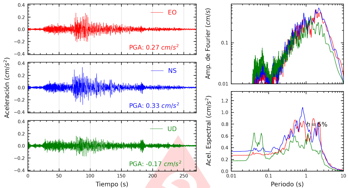
Figura A.35: Registros tiempo-historia, espectros de Fourier y de respuesta en las direcciones EO, NS y vertical de la estación SCHYO. Sismo de Lomas, Caraveli - Arequipa del 2024-07-12, 04:30:32 (Hora local)
