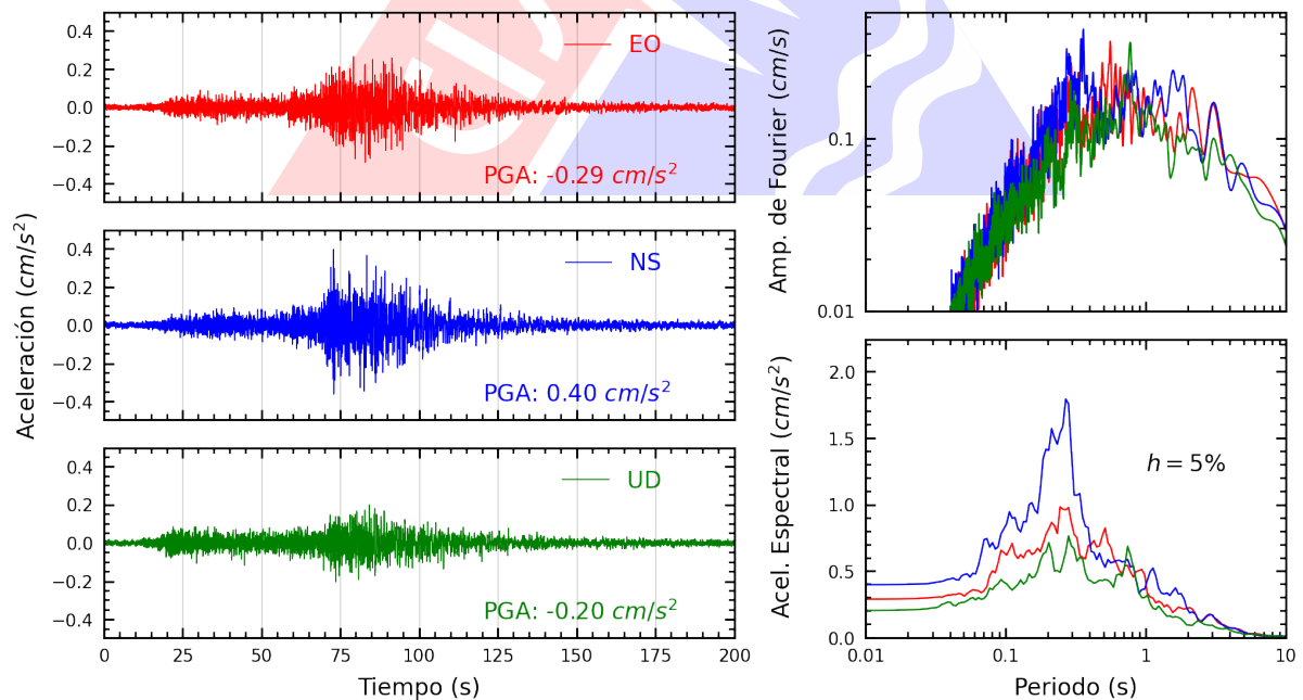
Figura A.28: Registros tiempo-historia, espectros de Fourier y de respuesta en las direcciones EO, NS y vertical de la estación SERVI. Sismo de Lomas, Caraveli - Arequipa del 2024-07-12, 04:30:32 (Hora local)
