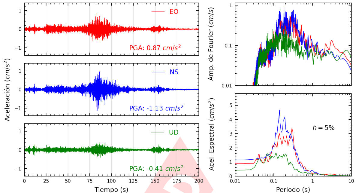
Figura A.9: Registros tiempo-historia, espectros de Fourier y de respuesta en las direcciones EO, NS y vertical de la estación CARAB. Sismo de Lomas, Caraveli - Arequipa del 2024-07-12, 04:30:32 (Hora local)
