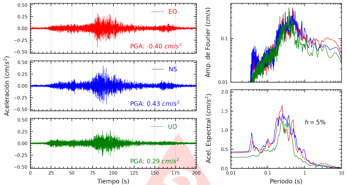
Figura A.25: Registros tiempo-historia, espectros de Fourier y de respuesta en las direcciones EO, NS y vertical de la estación COMAS. Sismo de Lomas, Caraveli - Arequipa del 2024-07-12, 04:30:32 (Hora local)
