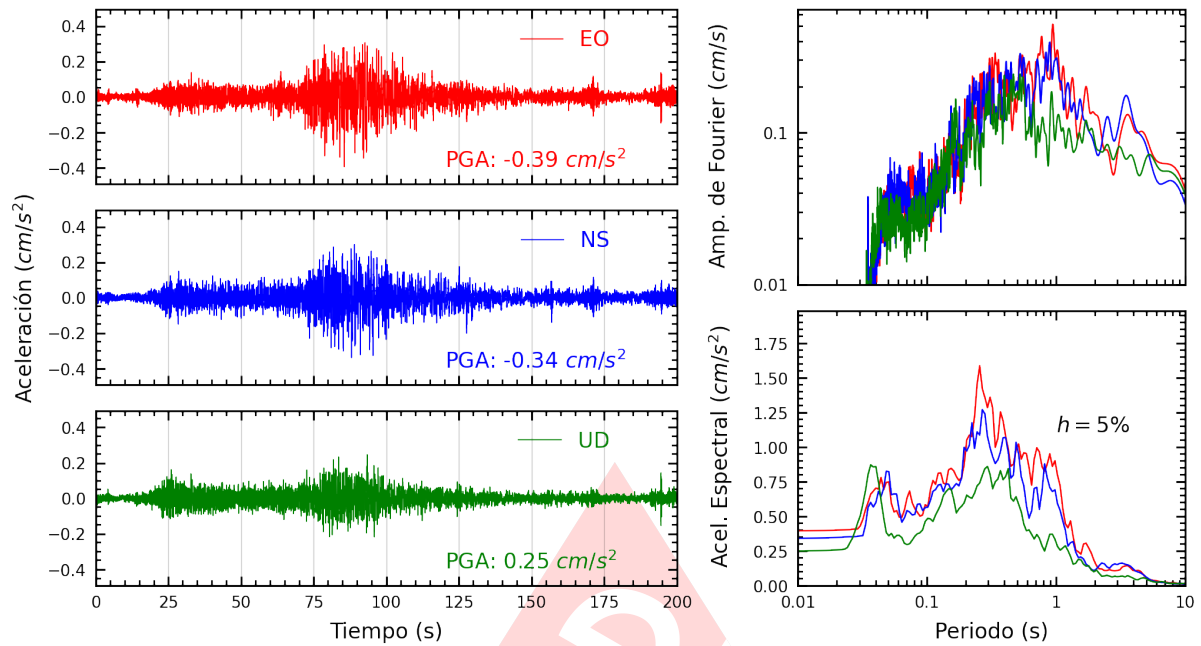
Figura A.29: Registros tiempo-historia, espectros de Fourier y de respuesta en las direcciones EO, NS y vertical de la estación UPCSM. Sismo de Lomas, Caraveli - Arequipa del 2024-07-12, 04:30:32 (Hora local)
