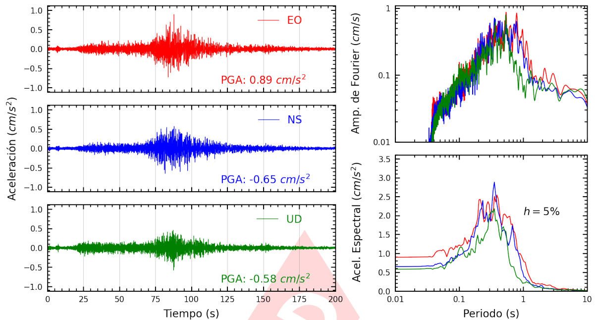
Figura A.11: Registros tiempo-historia, espectros de Fourier y de respuesta en las direcciones EO, NS y vertical de la estación UCV. Sismo de Lomas, Caraveli - Arequipa del 2024-07-12, 04:30:32 (Hora local)
