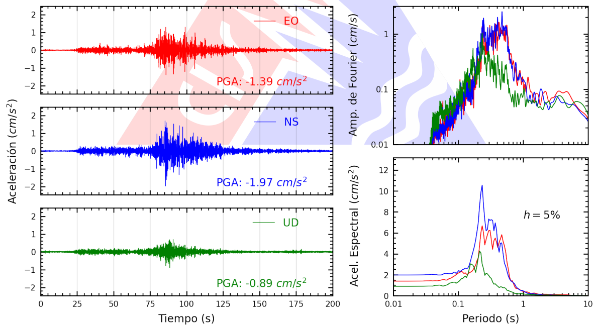
Figura A.2: Registros tiempo-historia, espectros de Fourier y de respuesta en las direcciones EO, NS y vertical de la estación MDPP. Sismo de Lomas, Caraveli - Arequipa del 2024-07-12, 04:30:32 (Hora local)
