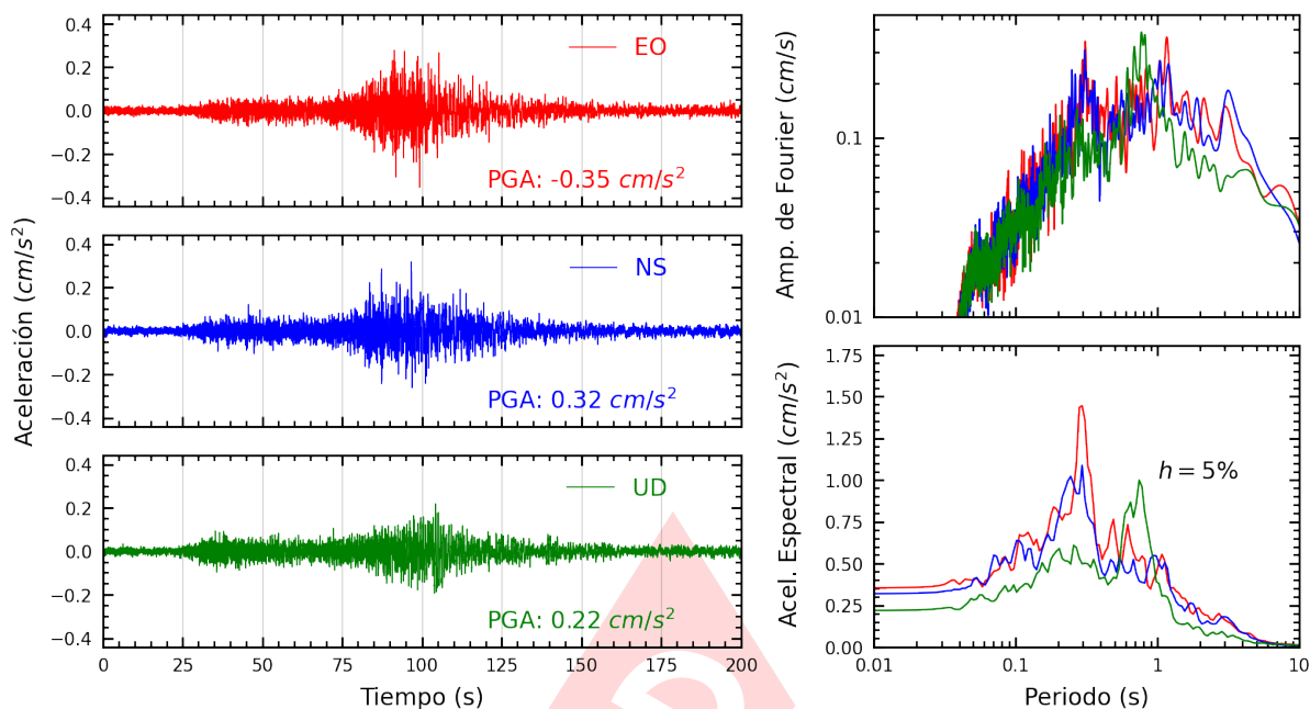
Figura A.33: Registros tiempo-historia, espectros de Fourier y de respuesta en las direcciones EO, NS y vertical de la estación CENEP. Sismo de Lomas, Caraveli - Arequipa del 2024-07-12, 04:30:32 (Hora local)
