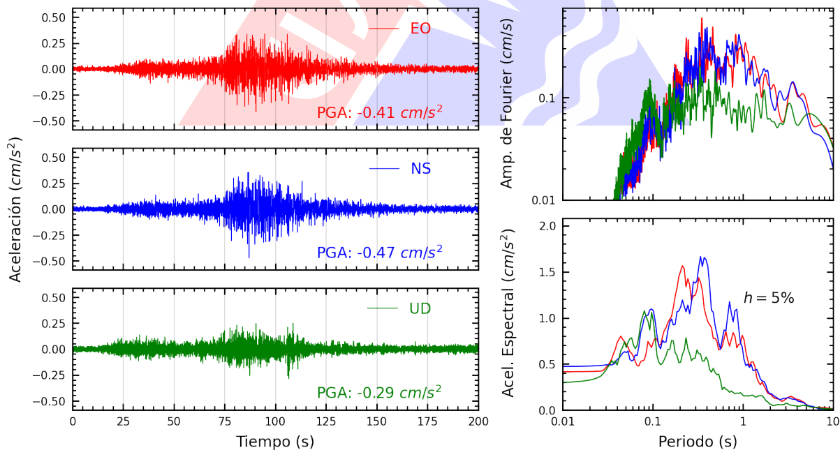
Figura A.24: Registros tiempo-historia, espectros de Fourier y de respuesta en las direcciones EO, NS y vertical de la estación RAMON. Sismo de Lomas, Caraveli - Arequipa del 2024-07-12, 04:30:32 (Hora local)
