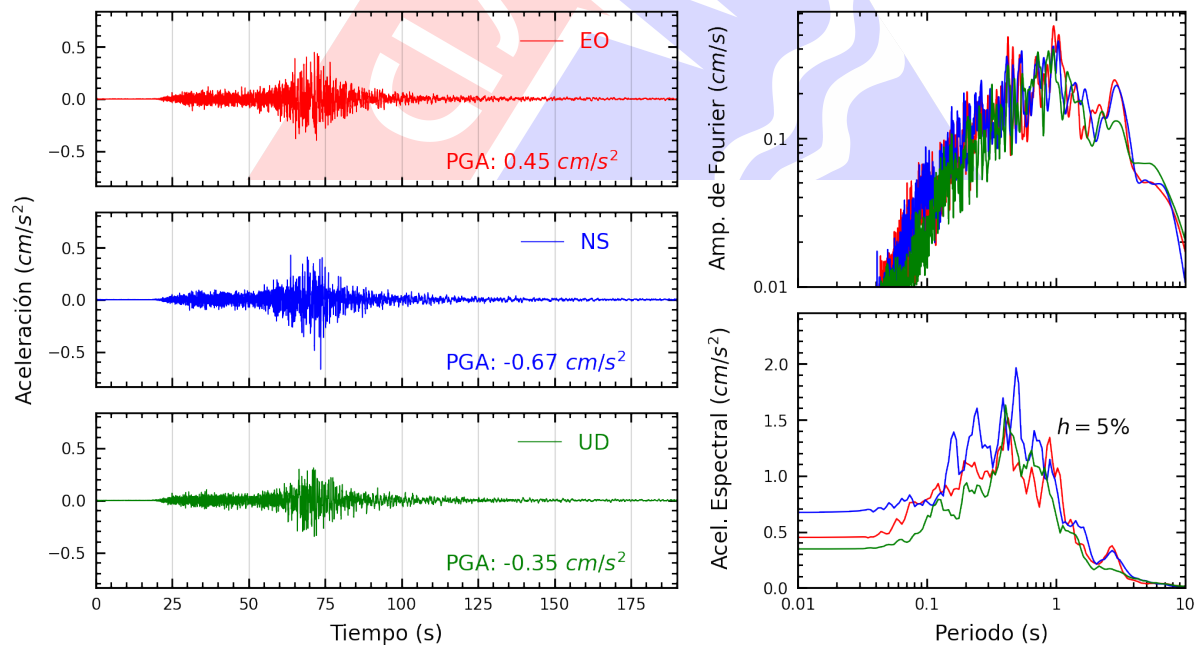
Figura A.20: Registros tiempo-historia, espectros de Fourier y de respuesta en las direcciones EO, NS y vertical de la estación UNSA. Sismo de Lomas, Caraveli - Arequipa del 2024-07-12, 04:30:32 (Hora local)
