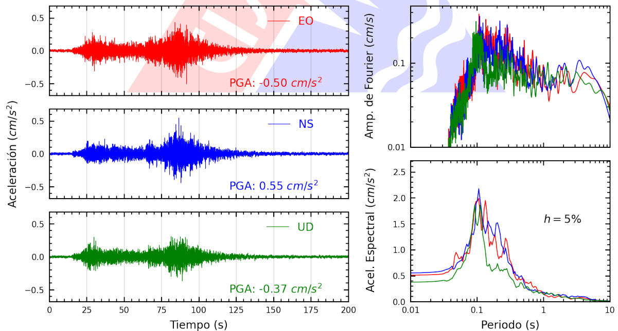
Figura A.22: Registros tiempo-historia, espectros de Fourier y de respuesta en las direcciones EO, NS y vertical de la estación AMORE. Sismo de Lomas, Caraveli - Arequipa del 2024-07-12, 04:30:32 (Hora local)
