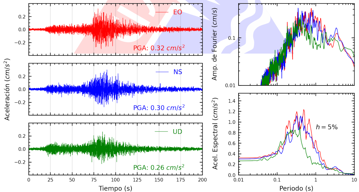
Figura A.38: Registros tiempo-historia, espectros de Fourier y de respuesta en las direcciones EO, NS y vertical de la estación UNFV. Sismo de Lomas, Caraveli - Arequipa del 2024-07-12, 04:30:32 (Hora local)
