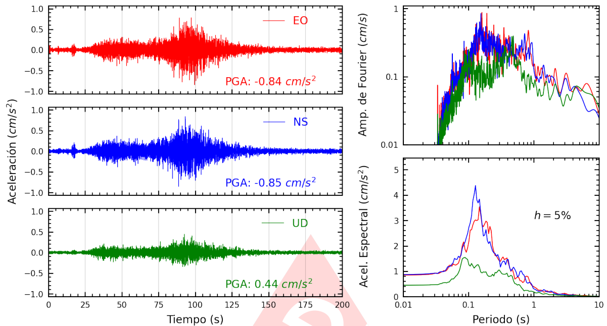
Figura A.13: Registros tiempo-historia, espectros de Fourier y de respuesta en las direcciones EO, NS y vertical de la estación USILM. Sismo de Lomas, Caraveli - Arequipa del 2024-07-12, 04:30:32 (Hora local)
