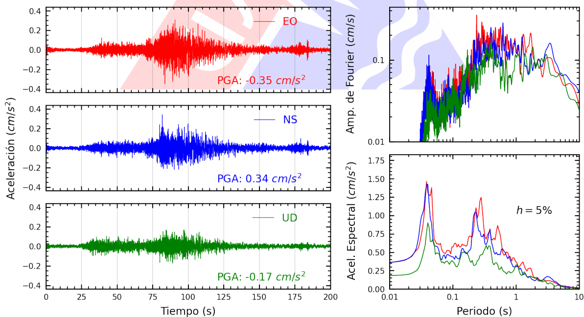
Figura A.34: Registros tiempo-historia, espectros de Fourier y de respuesta en las direcciones EO, NS y vertical de la estación CEPRE. Sismo de Lomas, Caraveli - Arequipa del 2024-07-12, 04:30:32 (Hora local)
