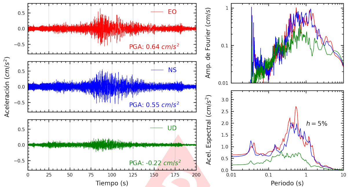
Figura A.21: Registros tiempo-historia, espectros de Fourier y de respuesta en las direcciones EO, NS y vertical de la estación DHNPE. Sismo de Lomas, Caraveli - Arequipa del 2024-07-12, 04:30:32 (Hora local)
