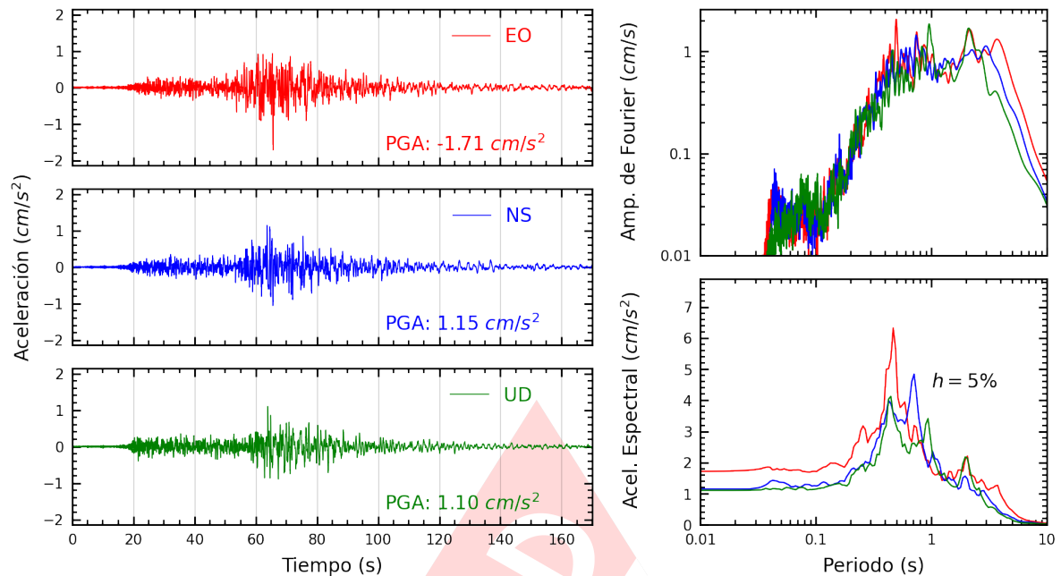
Figura A.3: Registros tiempo-historia, espectros de Fourier y de respuesta en las direcciones EO, NS y vertical de la estación SCAYA. Sismo de Lomas, Caraveli - Arequipa del 2024-07-12, 04:30:32 (Hora local)
