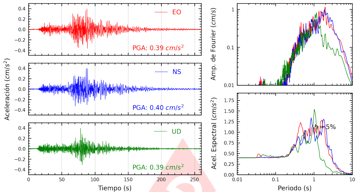
Figura A.27: Registros tiempo-historia, espectros de Fourier y de respuesta en las direcciones EO, NS y vertical de la estación UNCP. Sismo de Lomas, Caraveli - Arequipa del 2024-07-12, 04:30:32 (Hora local)
