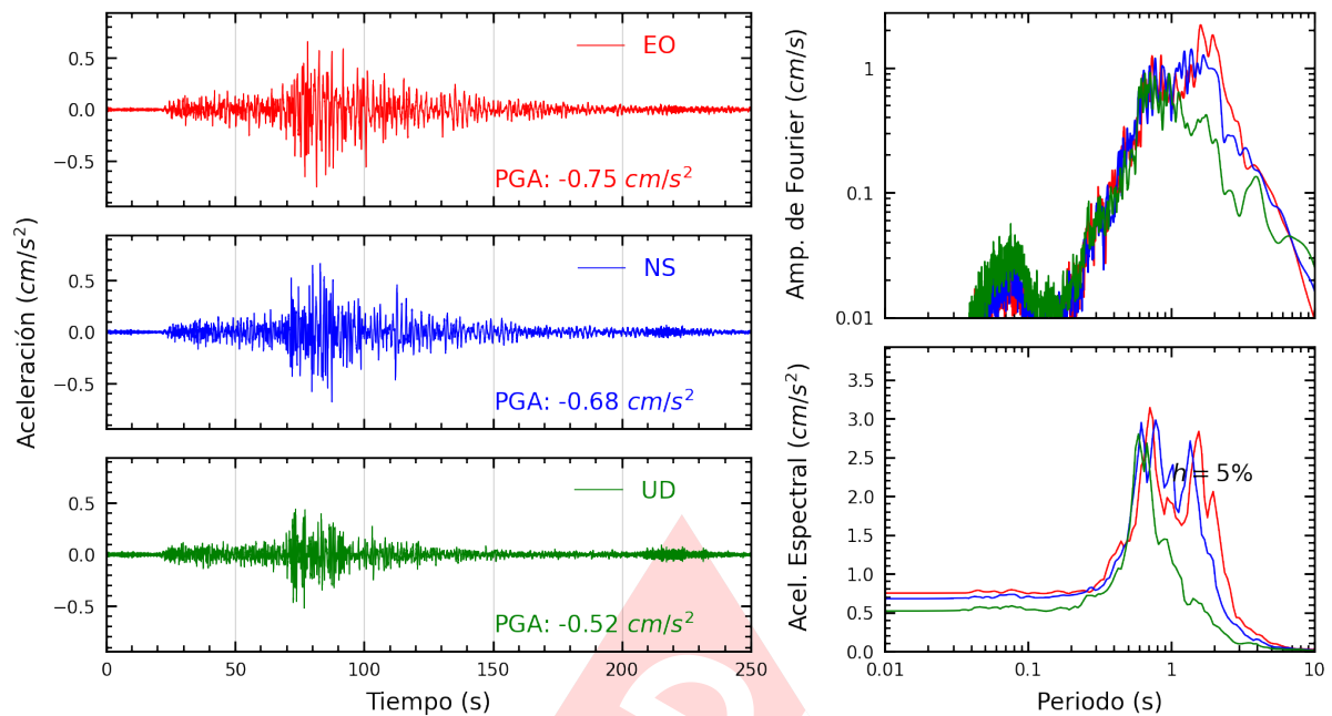
Figura A.17: Registros tiempo-historia, espectros de Fourier y de respuesta en las direcciones EO, NS y vertical de la estación SCCUS. Sismo de Lomas, Caraveli - Arequipa del 2024-07-12, 04:30:32 (Hora local)
