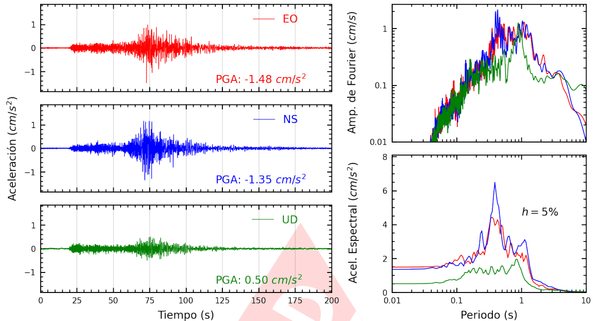
Figura A.5: Registros tiempo-historia, espectros de Fourier y de respuesta en las direcciones EO, NS y vertical de la estación SCARQ. Sismo de Lomas, Caraveli - Arequipa del 2024-07-12, 04:30:32 (Hora local)
