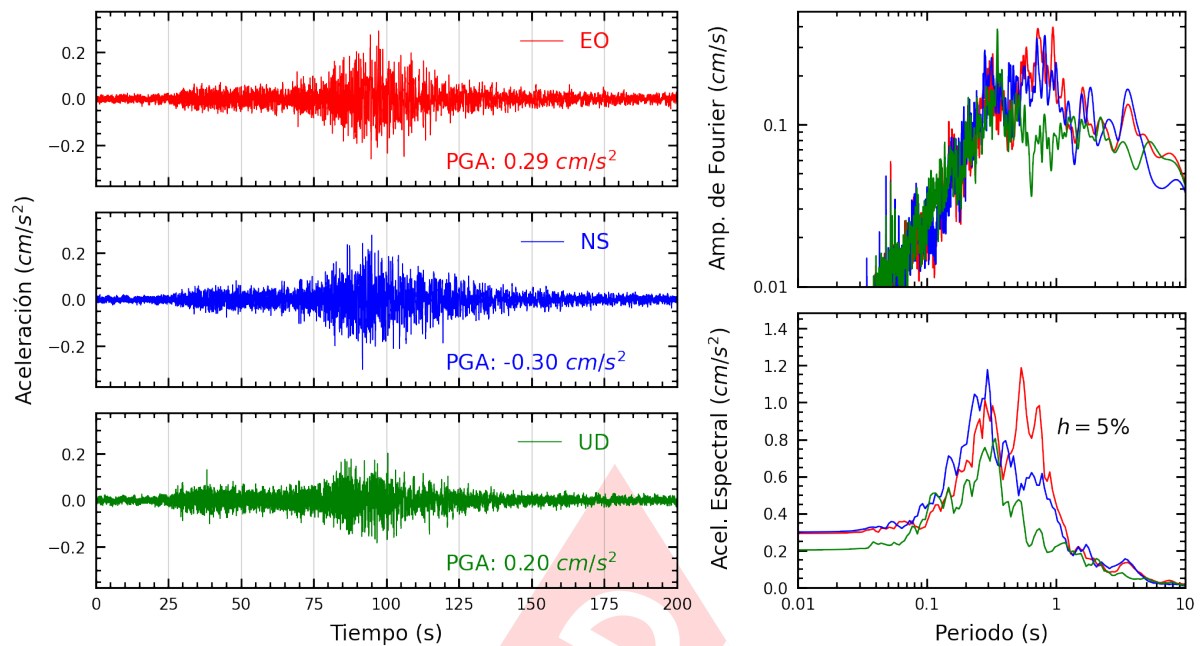
Figura A.41: Registros tiempo-historia, espectros de Fourier y de respuesta en las direcciones EO, NS y vertical de la estación UNMSM. Sismo de Lomas, Caraveli - Arequipa del 2024-07-12, 04:30:32 (Hora local)
