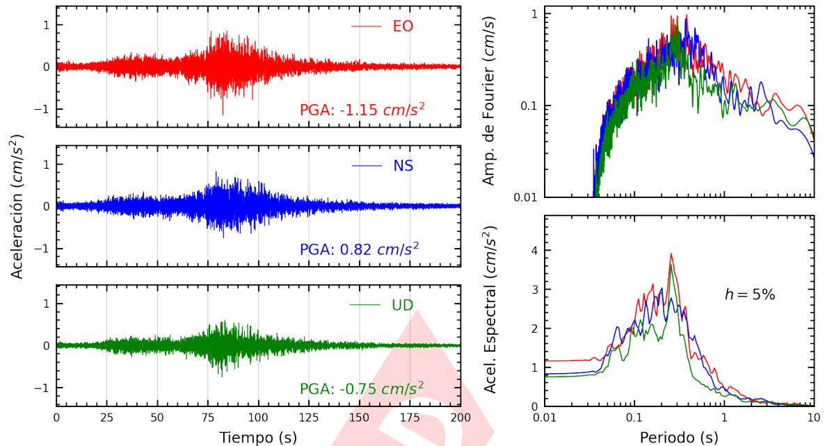
Figura A.7: Registros tiempo-historia, espectros de Fourier y de respuesta en las direcciones EO, NS y vertical de la estación PUNTA. Sismo de Lomas, Caraveli - Arequipa del 2024-07-12, 04:30:32 (Hora local)
