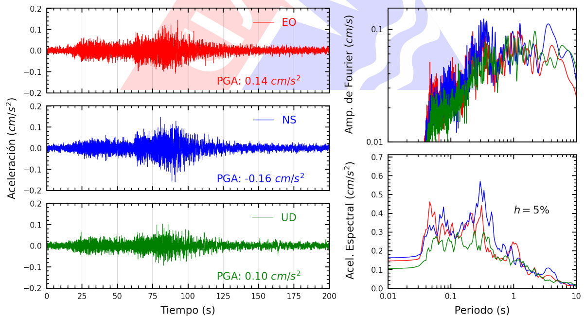
Figura A.42: Registros tiempo-historia, espectros de Fourier y de respuesta en las direcciones EO, NS y vertical de la estación UCSS. Sismo de Lomas, Caraveli - Arequipa del 2024-07-12, 04:30:32 (Hora local)
