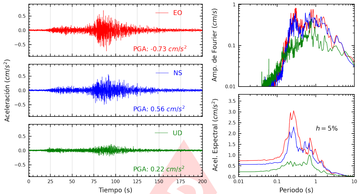
Figura A.19: Registros tiempo-historia, espectros de Fourier y de respuesta en las direcciones EO, NS y vertical de la estación DDMI. Sismo de Lomas, Caraveli - Arequipa del 2024-07-12, 04:30:32 (Hora local)
