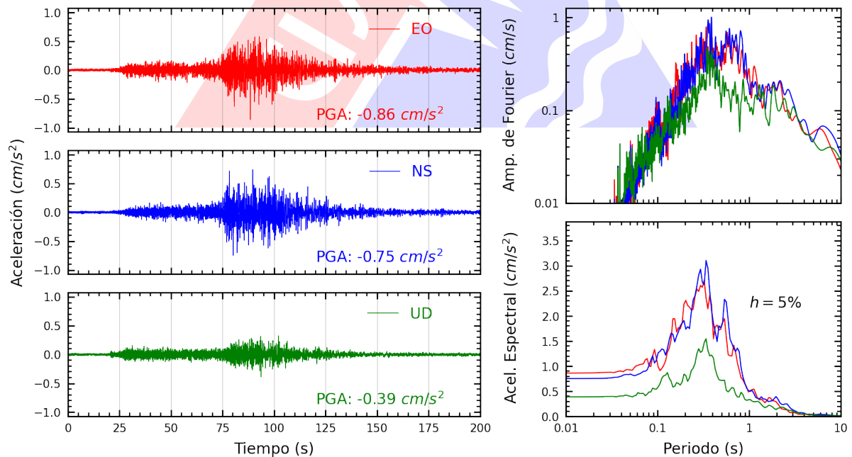
Figura A.12: Registros tiempo-historia, espectros de Fourier y de respuesta en las direcciones EO, NS y vertical de la estación USILP. Sismo de Lomas, Caraveli - Arequipa del 2024-07-12, 04:30:32 (Hora local)
