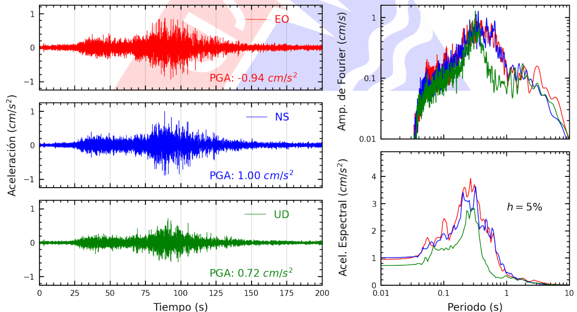
Figura A.10: Registros tiempo-historia, espectros de Fourier y de respuesta en las direcciones EO, NS y vertical de la estación UNTEL. Sismo de Lomas, Caraveli - Arequipa del 2024-07-12, 04:30:32 (Hora local)
