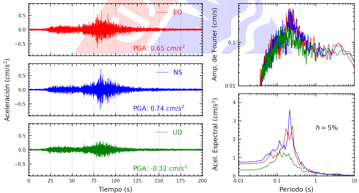
Figura A.18: Registros tiempo-historia, espectros de Fourier y de respuesta en las direcciones EO, NS y vertical de la estación INDEP. Sismo de Lomas, Caraveli - Arequipa del 2024-07-12, 04:30:32 (Hora local)
