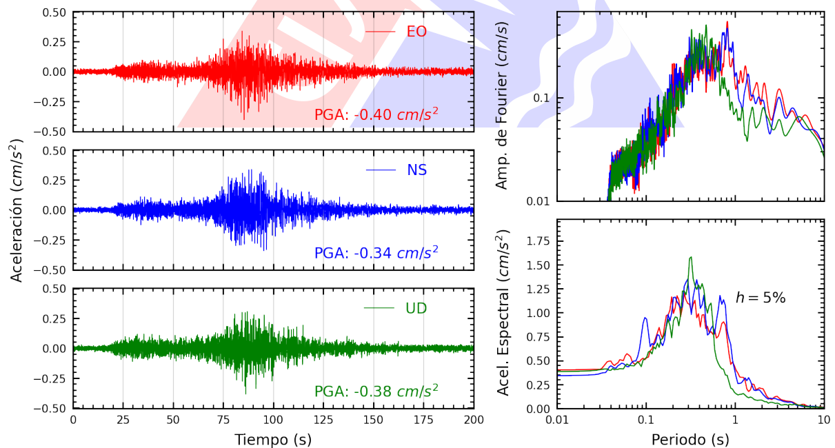
Figura A.26: Registros tiempo-historia, espectros de Fourier y de respuesta en las direcciones EO, NS y vertical de la estación IMCA. Sismo de Lomas, Caraveli - Arequipa del 2024-07-12, 04:30:32 (Hora local)
