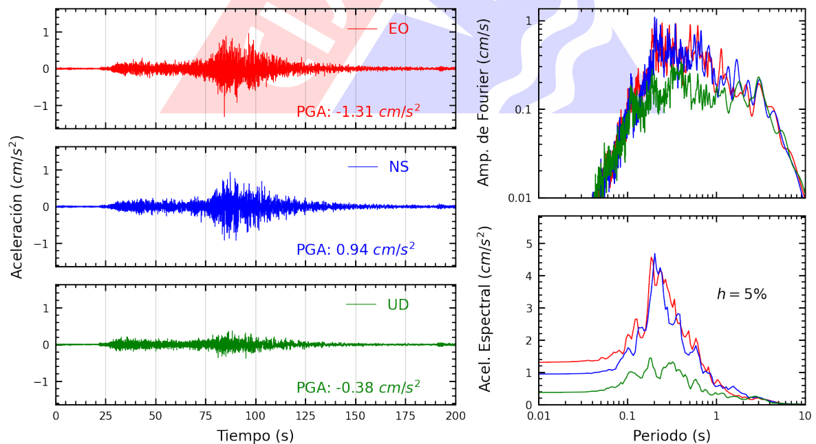
Figura A.6: Registros tiempo-historia, espectros de Fourier y de respuesta en las direcciones EO, NS y vertical de la estación SCCHO. Sismo de Lomas, Caraveli - Arequipa del 2024-07-12, 04:30:32 (Hora local)
