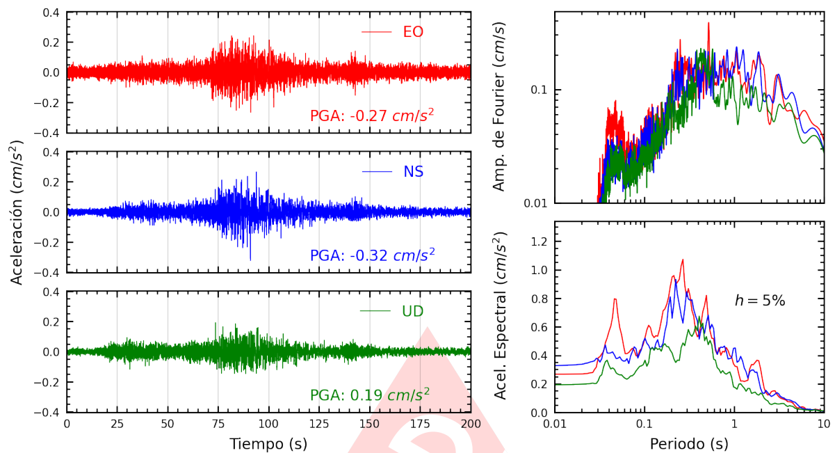
Figura A.37: Registros tiempo-historia, espectros de Fourier y de respuesta en las direcciones EO, NS y vertical de la estación INICT. Sismo de Lomas, Caraveli - Arequipa del 2024-07-12, 04:30:32 (Hora local)
