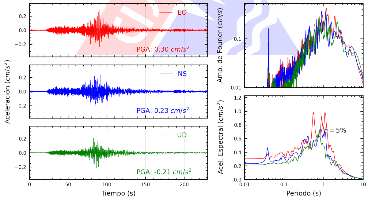
Figura A.40: Registros tiempo-historia, espectros de Fourier y de respuesta en las direcciones EO, NS y vertical de la estación UNAM. Sismo de Lomas, Caraveli - Arequipa del 2024-07-12, 04:30:32 (Hora local)
