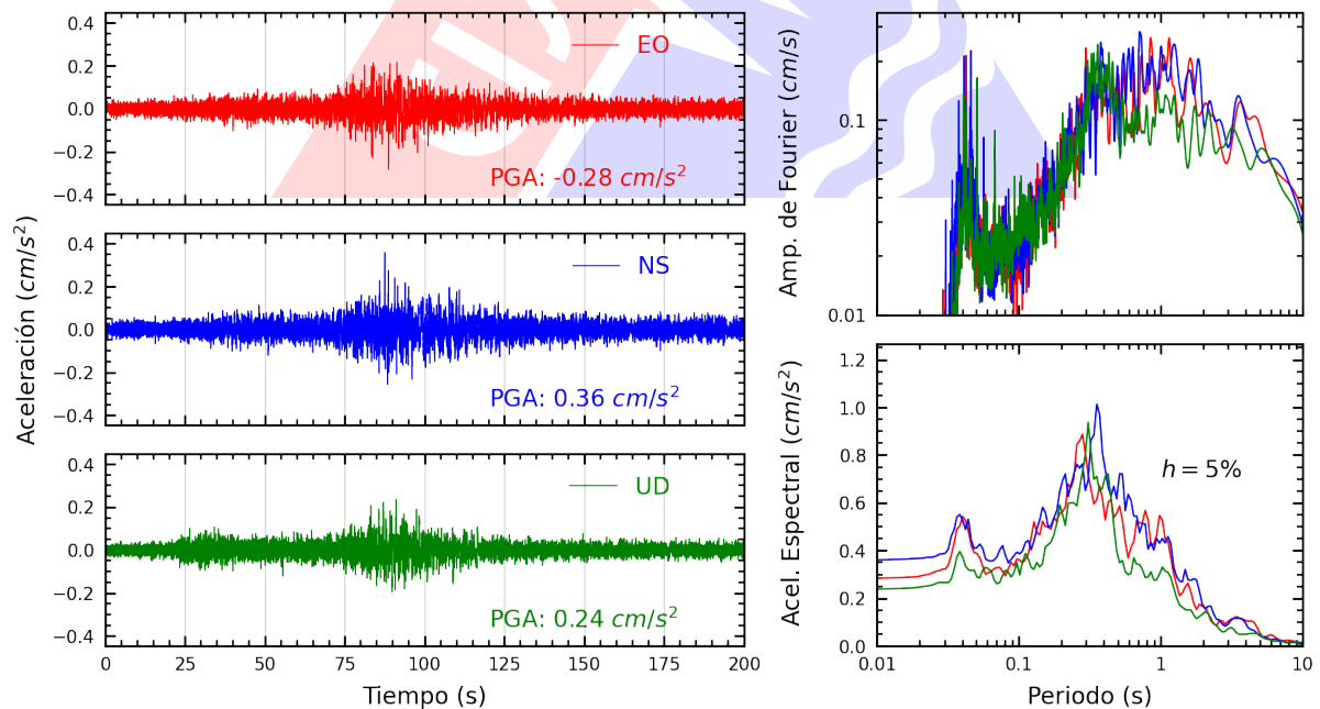
Figura A.32: Registros tiempo-historia, espectros de Fourier y de respuesta en las direcciones EO, NS y vertical de la estación BONDY. Sismo de Lomas, Caraveli - Arequipa del 2024-07-12, 04:30:32 (Hora local)
