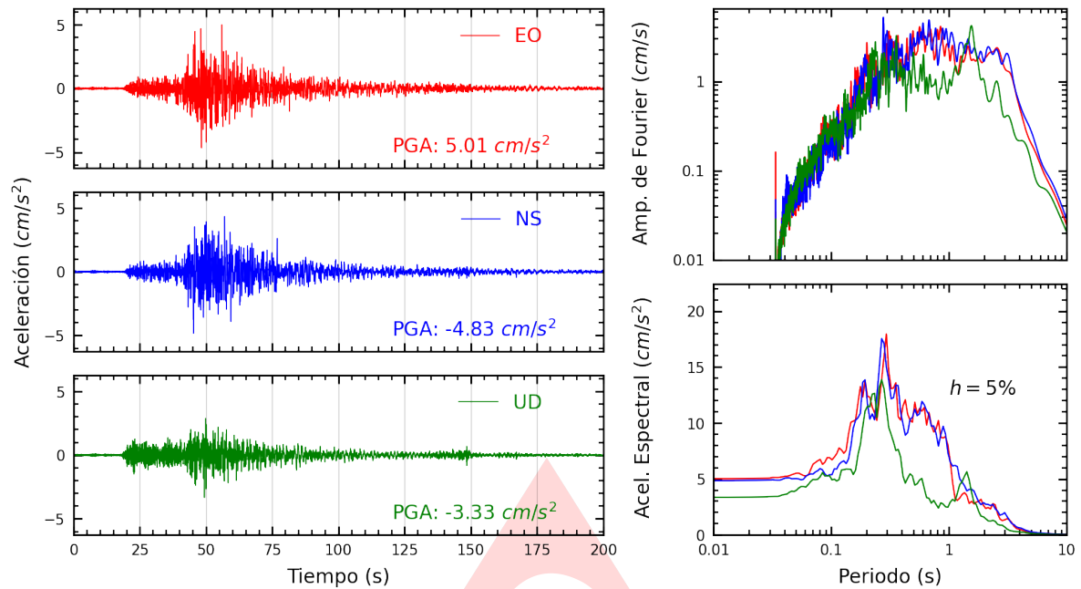
Figura A.1: Registros tiempo-historia, espectros de Fourier y de respuesta en las direcciones EO, NS y vertical de la estación SCICA. Sismo de Lomas, Caraveli - Arequipa del 2024-07-12, 04:30:32 (Hora local)
