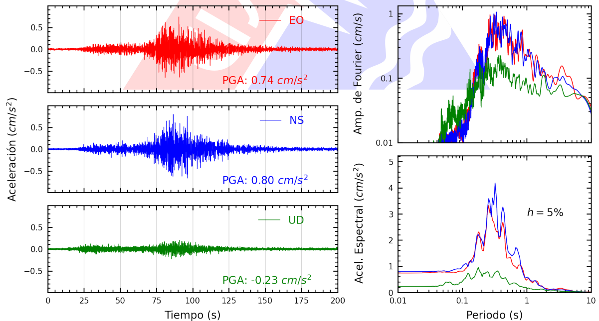
Figura A.16: Registros tiempo-historia, espectros de Fourier y de respuesta en las direcciones EO, NS y vertical de la estación ACAPU. Sismo de Lomas, Caraveli - Arequipa del 2024-07-12, 04:30:32 (Hora local)
