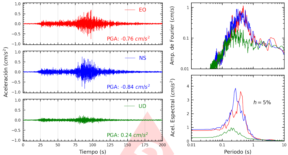
Figura A.15: Registros tiempo-historia, espectros de Fourier y de respuesta en las direcciones EO, NS y vertical de la estación VHAYA. Sismo de Lomas, Caraveli - Arequipa del 2024-07-12, 04:30:32 (Hora local)
