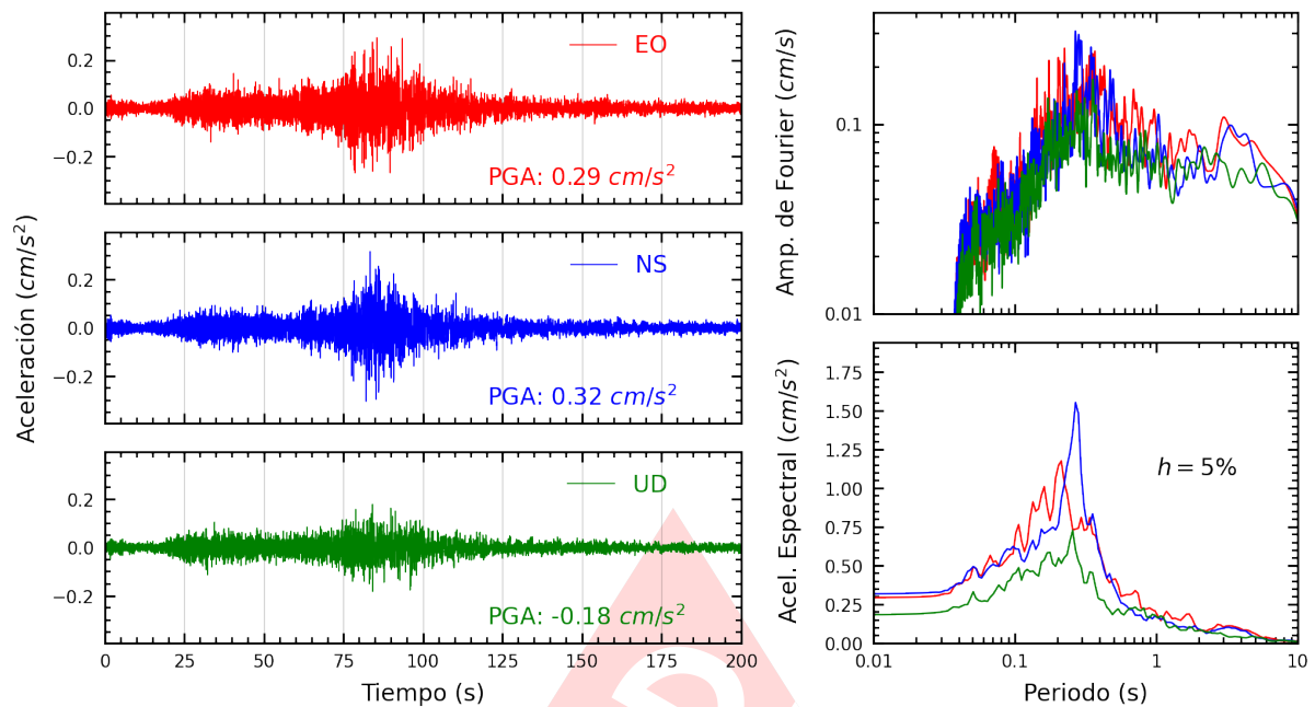
Figura A.39: Registros tiempo-historia, espectros de Fourier y de respuesta en las direcciones EO, NS y vertical de la estación FICPE. Sismo de Lomas, Caraveli - Arequipa del 2024-07-12, 04:30:32 (Hora local)
