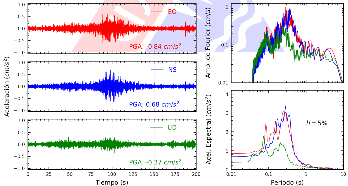
Figura A.14: Registros tiempo-historia, espectros de Fourier y de respuesta en las direcciones EO, NS y vertical de la estación SCOLI. Sismo de Lomas, Caraveli - Arequipa del 2024-07-12, 04:30:32 (Hora local)
