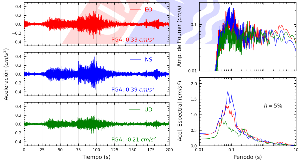
Figura A.30: Registros tiempo-historia, espectros de Fourier y de respuesta en las direcciones EO, NS y vertical de la estación JOSEO. Sismo de Lomas, Caraveli - Arequipa del 2024-07-12, 04:30:32 (Hora local)
