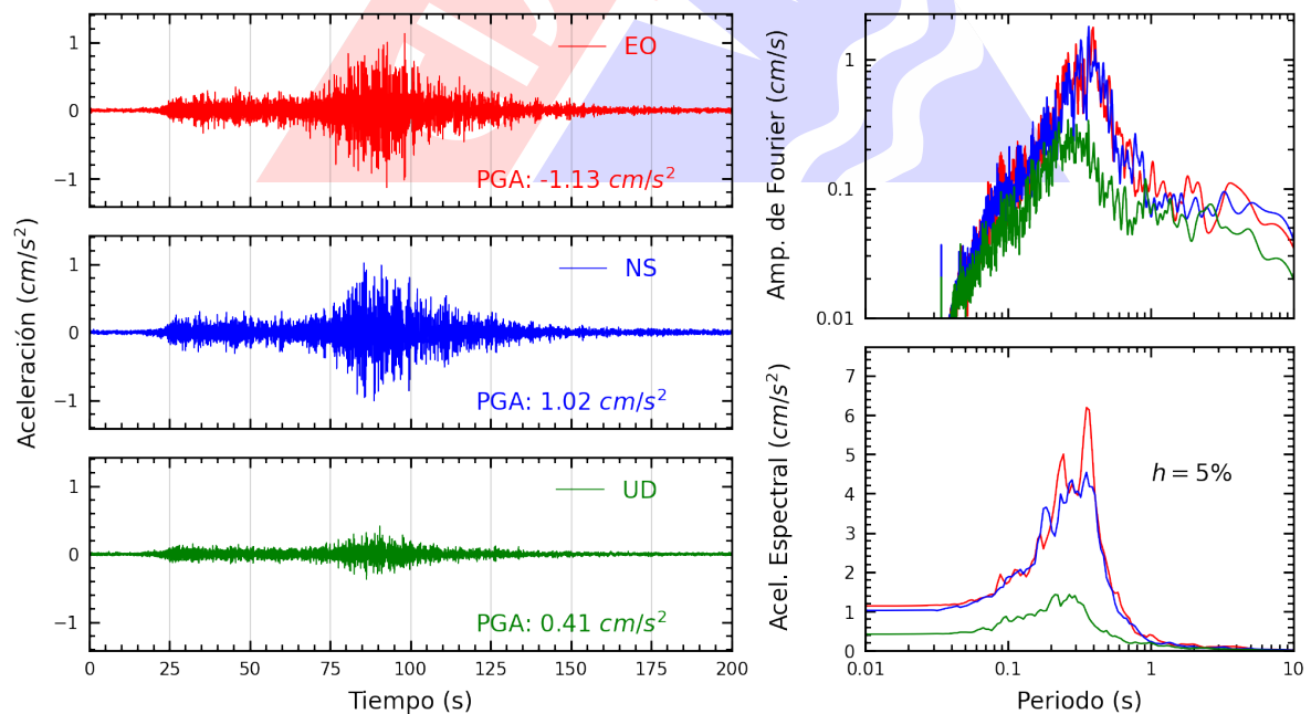
Figura A.8: Registros tiempo-historia, espectros de Fourier y de respuesta en las direcciones EO, NS y vertical de la estación DEFEN. Sismo de Lomas, Caraveli - Arequipa del 2024-07-12, 04:30:32 (Hora local)
