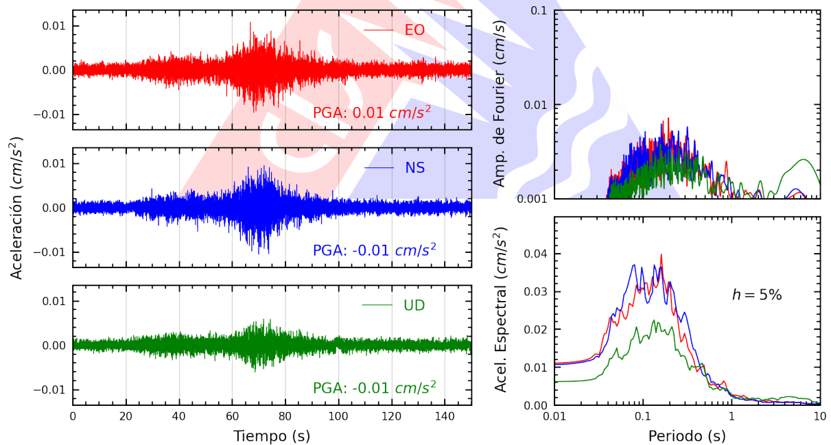
Figura A.2: Registros tiempo-historia, espectros de Fourier y de respuesta en las direcciones EO, NS y vertical de la estación UNSA. Sismo de Lomas, Caraveli - Arequipa del 2024-07-13, 09:02:32 (Hora local)
