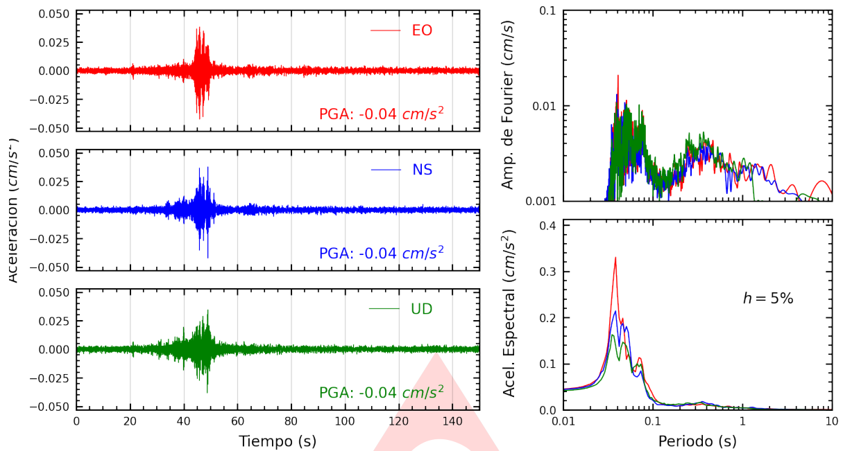
Figura A.1: Registros tiempo-historia, espectros de Fourier y de respuesta en las direcciones EO, NS y vertical de la estación UNCP. Sismo de Lomas, Caraveli - Arequipa del 2024-07-13, 09:02:32 (Hora local)
