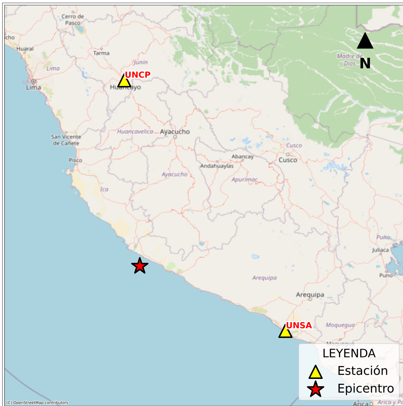
Figura 2: Mapa de ubicación de la(s) estación(es) acelerográfica(s) correspondiente(s) al Sismo de Lomas, Caraveli - Arequipa del 13 de julio de 2024 a las 09:02:32 (hora local)
