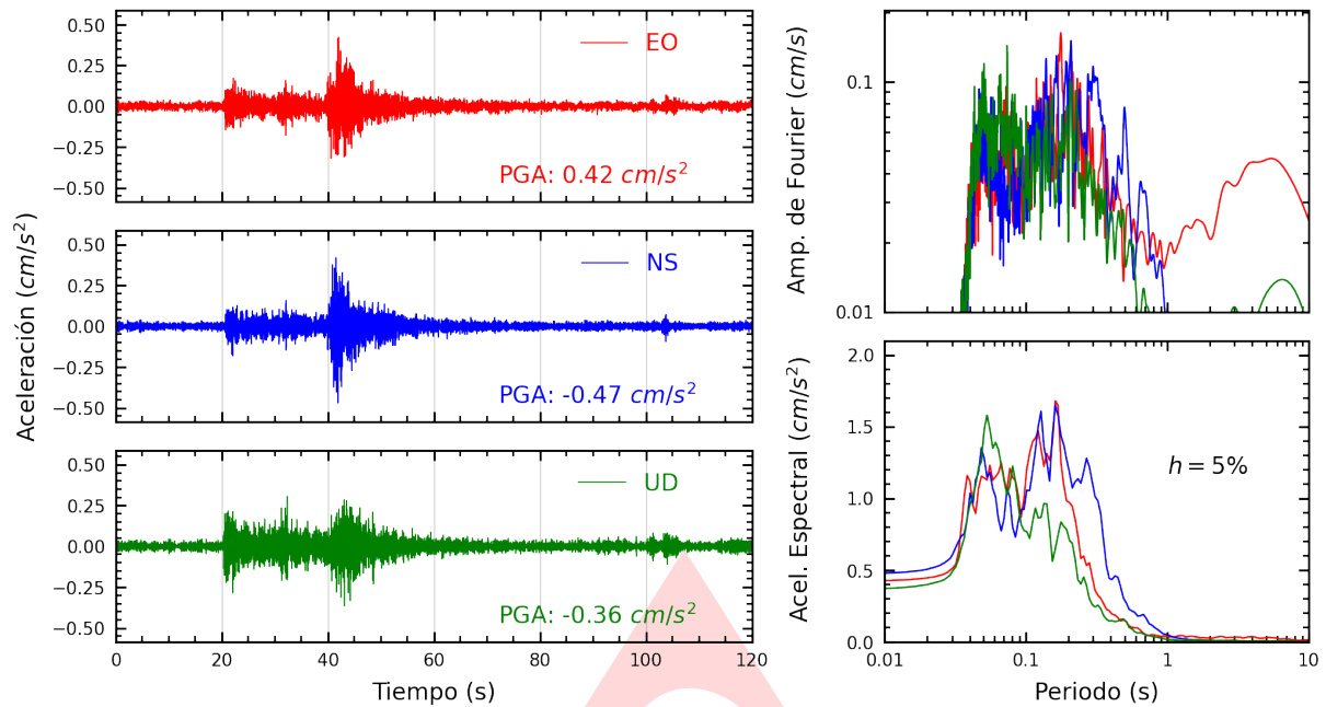
Figura A.1: Registros tiempo-historia, espectros de Fourier y de respuesta en las direcciones EO, NS y vertical de la estación UJBG3. Sismo de Capaso, El Collao - Puno del 2024-07-13, 20:13:23 (Hora local)
