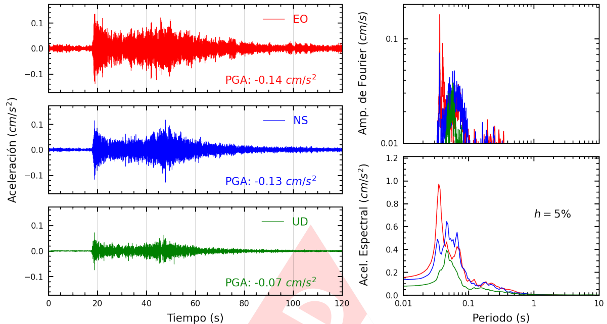
Figura A.3: Registros tiempo-historia, espectros de Fourier y de respuesta en las direcciones EO, NS y vertical de la estación UNAM. Sismo de Capaso, El Collao - Puno del 2024-07-13, 20:13:23 (Hora local)
