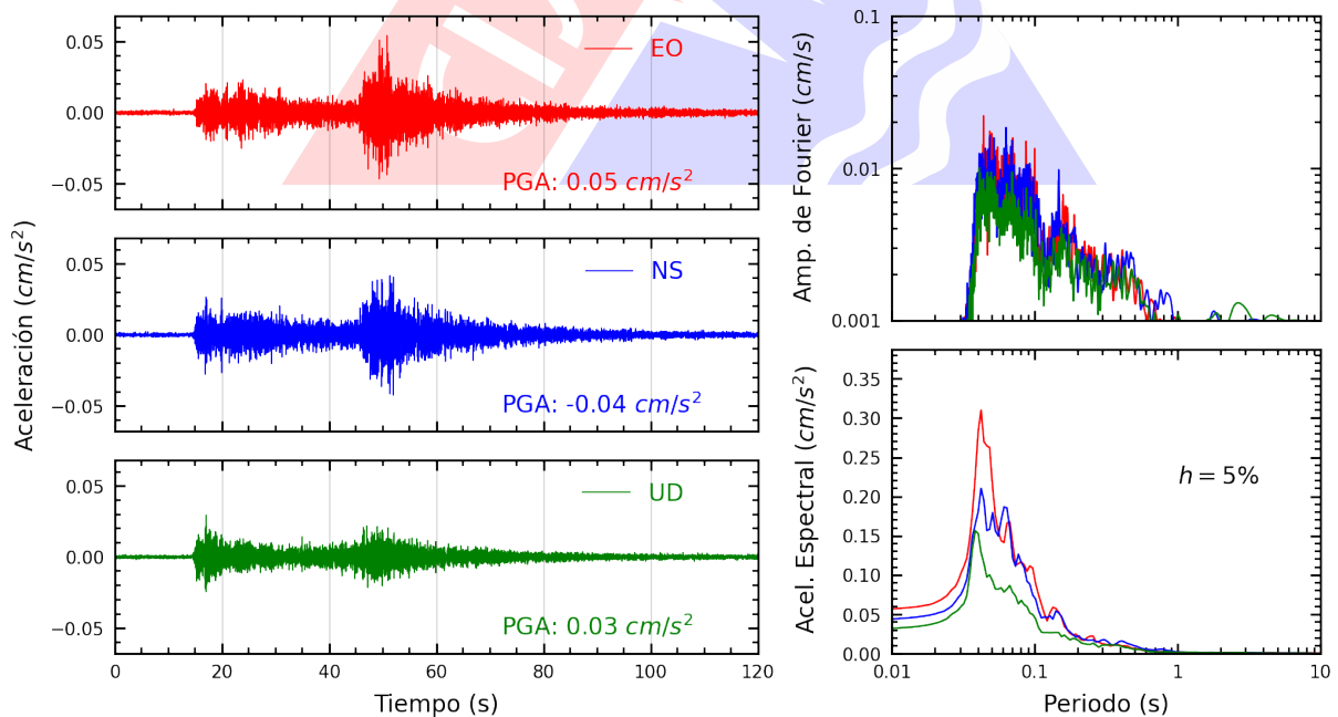
Figura A.4: Registros tiempo-historia, espectros de Fourier y de respuesta en las direcciones EO, NS y vertical de la estación UNSA. Sismo de Capaso, El Collao - Puno del 2024-07-13, 20:13:23 (Hora local)
