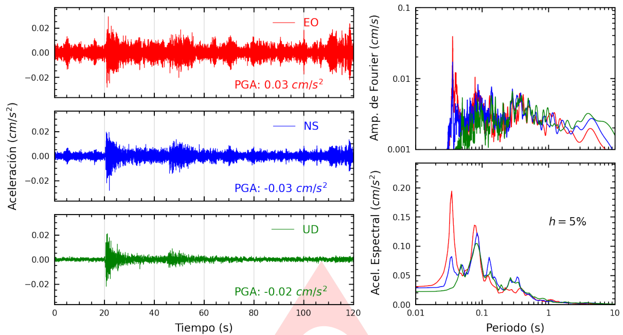
Figura A.1: Registros tiempo-historia, espectros de Fourier y de respuesta en las direcciones EO, NS y vertical de la estación UNAM. Sismo de Santa Lucía, Lampa - Puno del 2024-07-13, 20:45:23 (Hora local)
