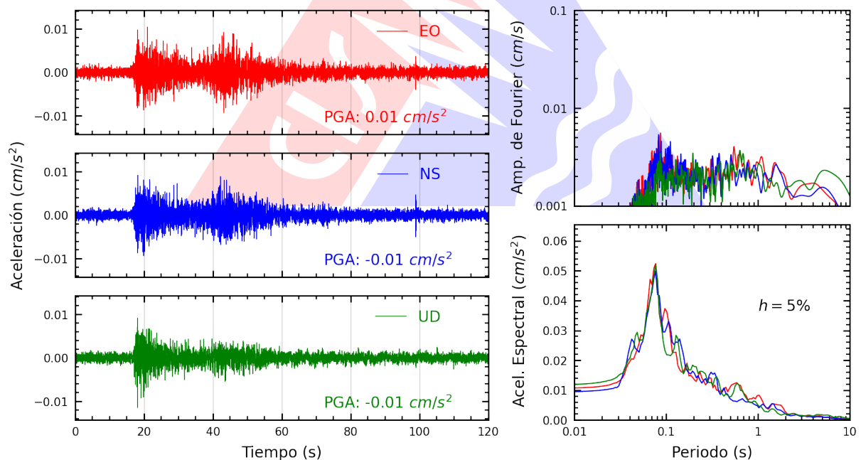
Figura A.2: Registros tiempo-historia, espectros de Fourier y de respuesta en las direcciones EO, NS y vertical de la estación UNSA. Sismo de Santa Lucía, Lampa - Puno del 2024-07-13, 20:45:23 (Hora local)
