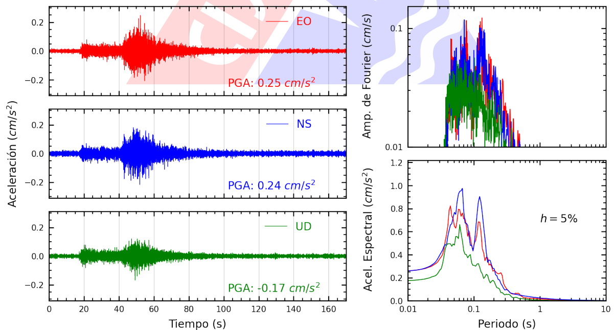
Figura A.16: Registros tiempo-historia, espectros de Fourier y de respuesta en las direcciones EO, NS y vertical de la estación ATARJ. Sismo de Pisco, Pisco - Ica del 2024-07-19, 08:54:25 (Hora local)
