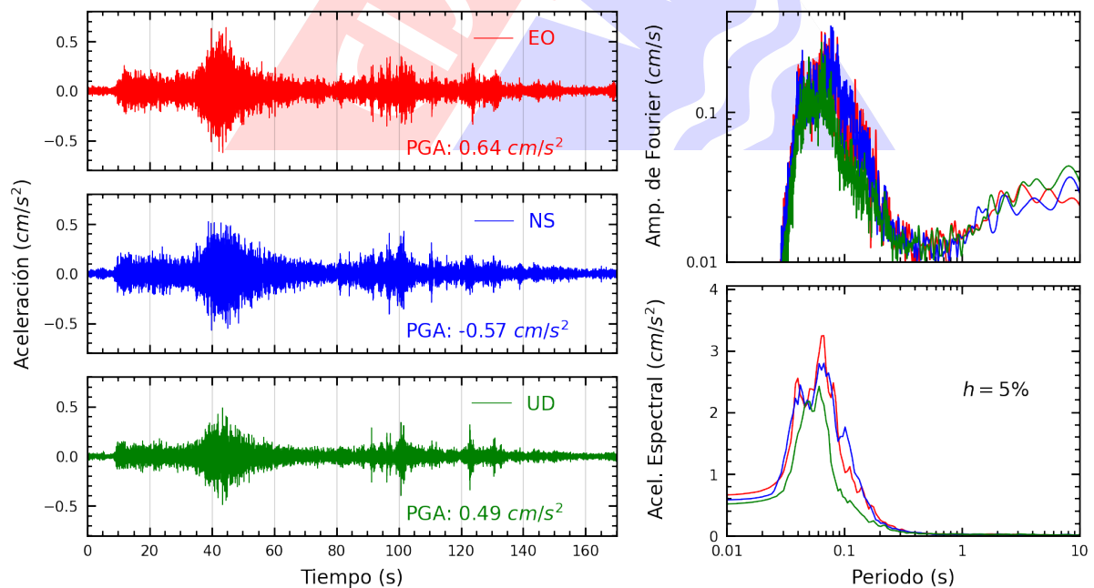
Figura A.4: Registros tiempo-historia, espectros de Fourier y de respuesta en las direcciones EO, NS y vertical de la estación JOSEO. Sismo de Pisco, Pisco - Ica del 2024-07-19, 08:54:25 (Hora local)
