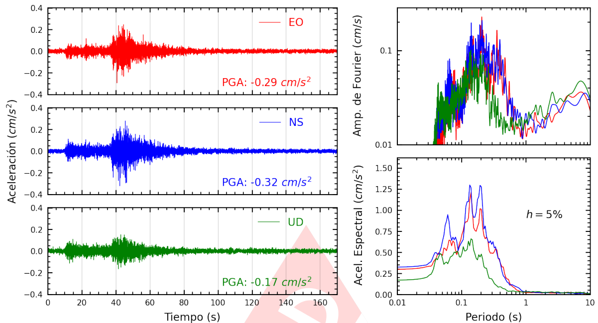
Figura A.9: Registros tiempo-historia, espectros de Fourier y de respuesta en las direcciones EO, NS y vertical de la estación VHAYA. Sismo de Pisco, Pisco - Ica del 2024-07-19, 08:54:25 (Hora local)
