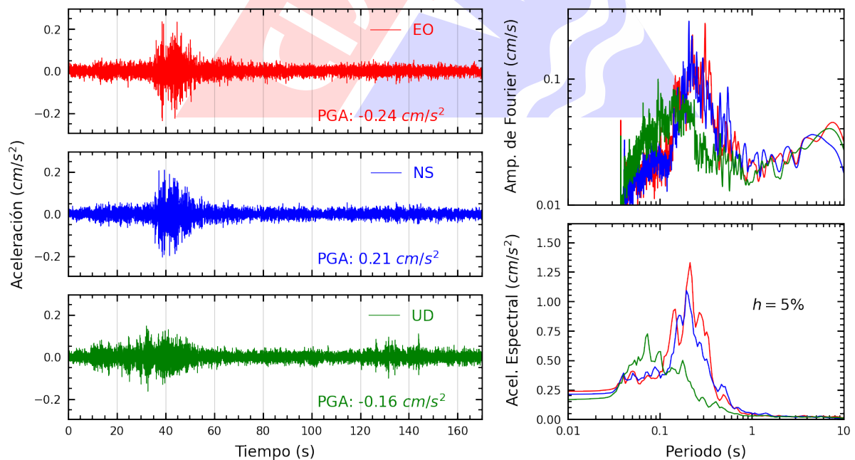
Figura A.18: Registros tiempo-historia, espectros de Fourier y de respuesta en las direcciones EO, NS y vertical de la estación DSMI. Sismo de Pisco, Pisco - Ica del 2024-07-19, 08:54:25 (Hora local)
