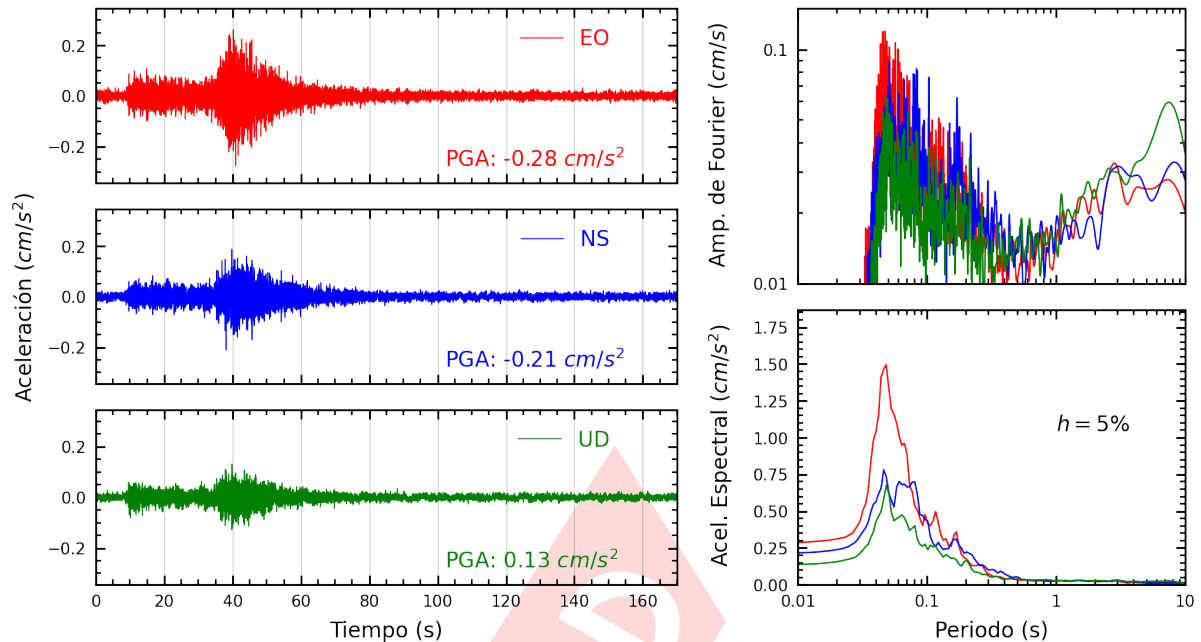
Figura A.13: Registros tiempo-historia, espectros de Fourier y de respuesta en las direcciones EO, NS y vertical de la estación UCSS. Sismo de Pisco, Pisco - Ica del 2024-07-19, 08:54:25 (Hora local)
