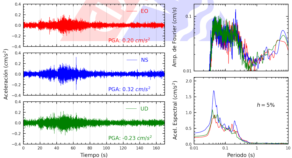
Figura A.10: Registros tiempo-historia, espectros de Fourier y de respuesta en las direcciones EO, NS y vertical de la estación USMP. Sismo de Pisco, Pisco - Ica del 2024-07-19, 08:54:25 (Hora local)
