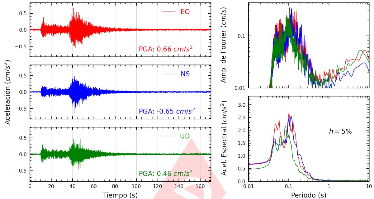
Figura A.3: Registros tiempo-historia, espectros de Fourier y de respuesta en las direcciones EO, NS y vertical de la estación AMORE. Sismo de Pisco, Pisco - Ica del 2024-07-19, 08:54:25 (Hora local)
