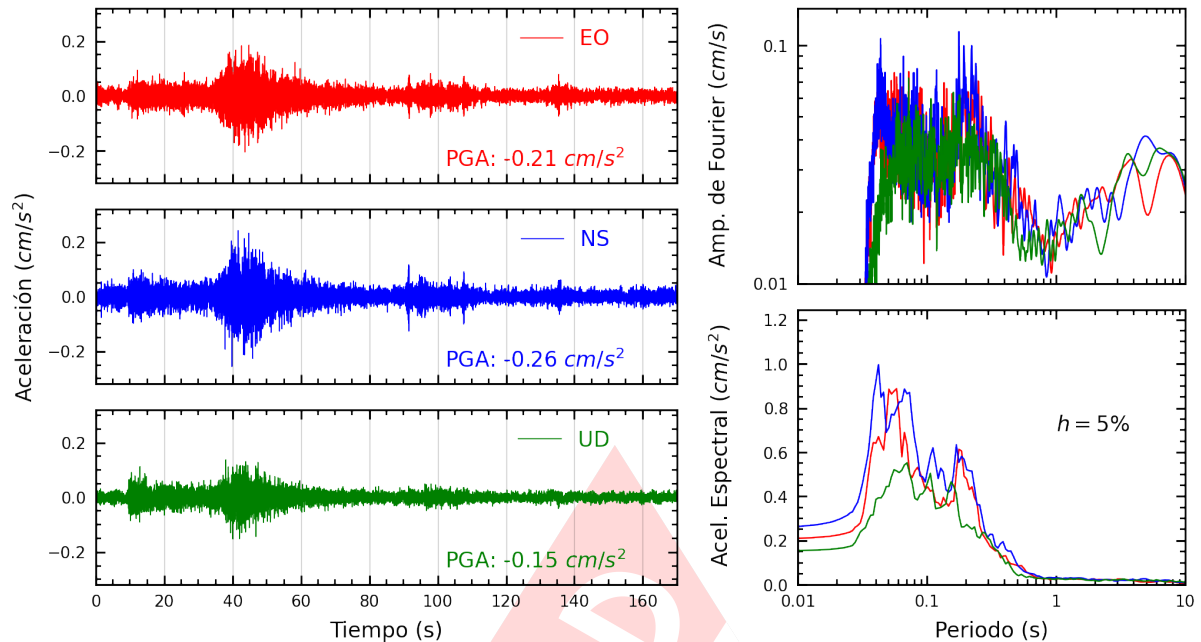
Figura A.15: Registros tiempo-historia, espectros de Fourier y de respuesta en las direcciones EO, NS y vertical de la estación COMAS. Sismo de Pisco, Pisco - Ica del 2024-07-19, 08:54:25 (Hora local)
