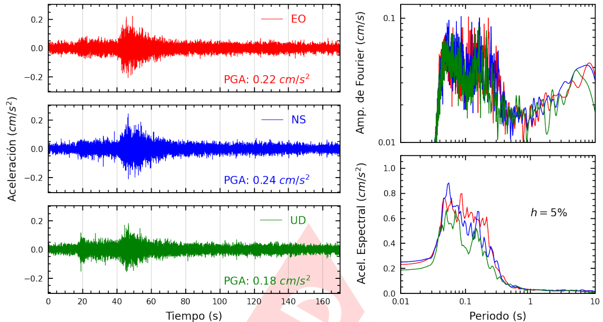
Figura A.17: Registros tiempo-historia, espectros de Fourier y de respuesta en las direcciones EO, NS y vertical de la estación CENEP. Sismo de Pisco, Pisco - Ica del 2024-07-19, 08:54:25 (Hora local)
