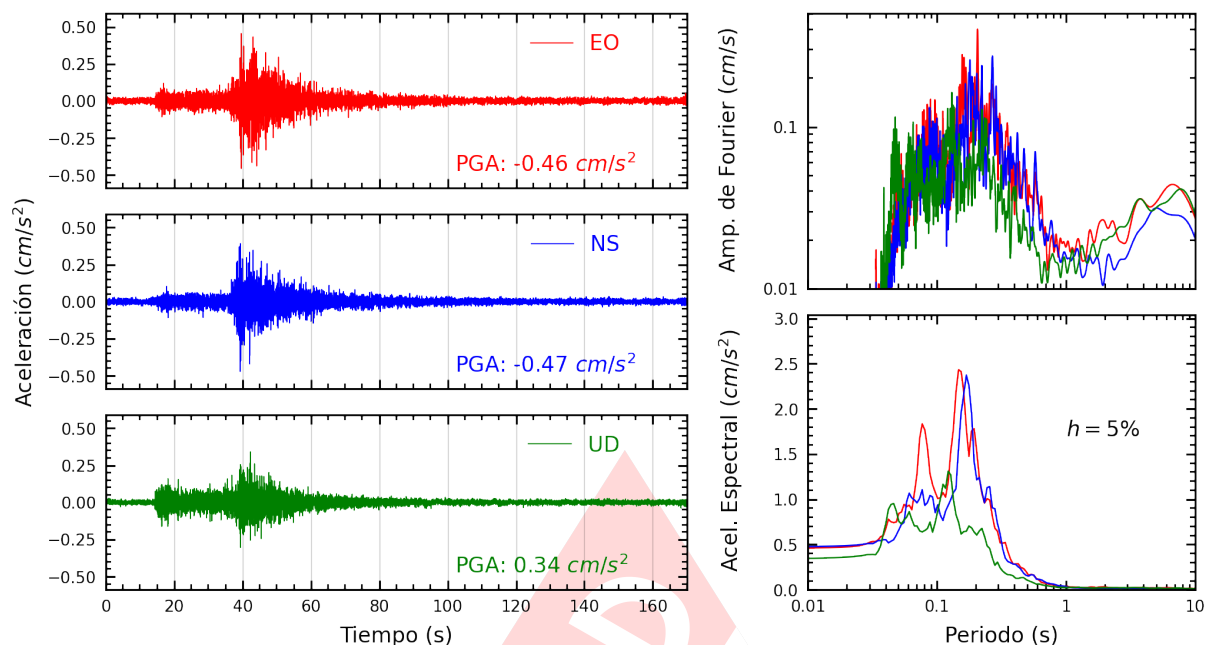
Figura A.7: Registros tiempo-historia, espectros de Fourier y de respuesta en las direcciones EO, NS y vertical de la estación USILP. Sismo de Pisco, Pisco - Ica del 2024-07-19, 08:54:25 (Hora local)
