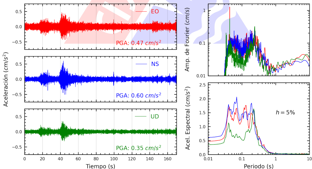
Figura A.6: Registros tiempo-historia, espectros de Fourier y de respuesta en las direcciones EO, NS y vertical de la estación UPCVI. Sismo de Pisco, Pisco - Ica del 2024-07-19, 08:54:25 (Hora local)
