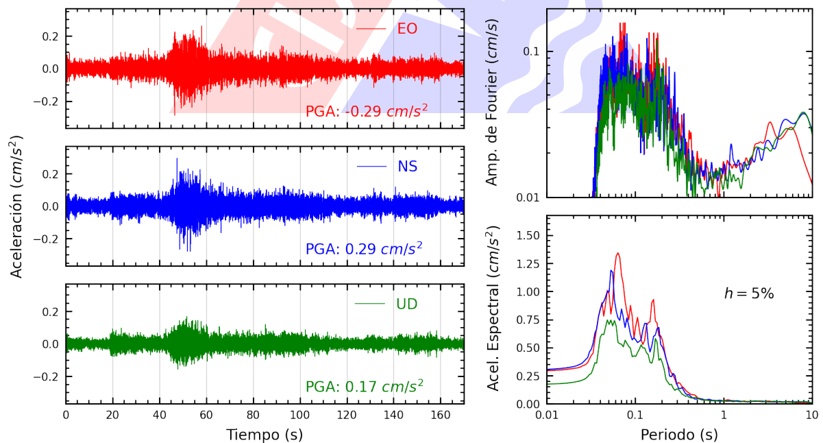
Figura A.12: Registros tiempo-historia, espectros de Fourier y de respuesta en las direcciones EO, NS y vertical de la estación FICPE. Sismo de Pisco, Pisco - Ica del 2024-07-19, 08:54:25 (Hora local)
