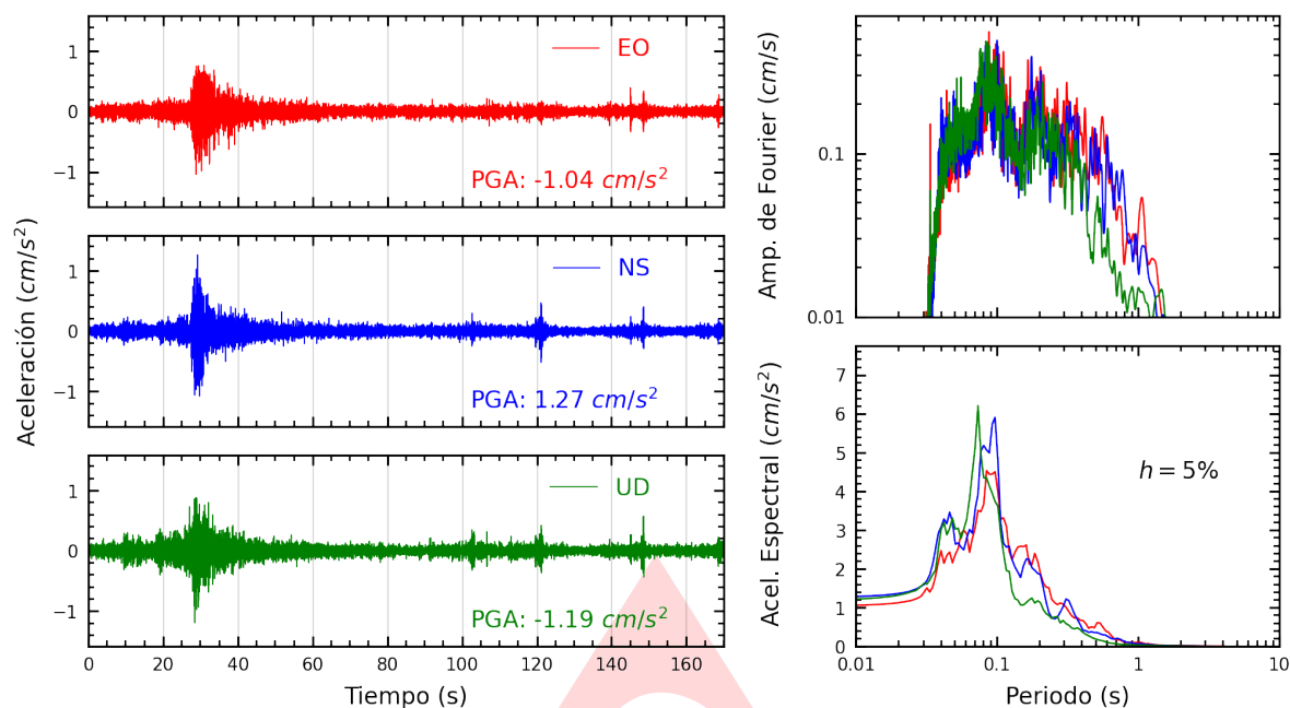
Figura A.1: Registros tiempo-historia, espectros de Fourier y de respuesta en las direcciones EO, NS y vertical de la estación SCICA. Sismo de Pisco, Pisco - Ica del 2024-07-19, 08:54:25 (Hora local)
