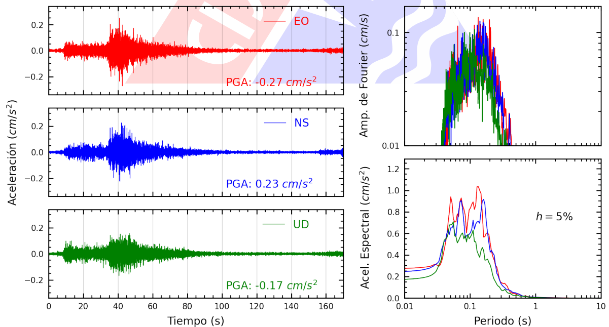
Figura A.14: Registros tiempo-historia, espectros de Fourier y de respuesta en las direcciones EO, NS y vertical de la estación JALV2. Sismo de Pisco, Pisco - Ica del 2024-07-19, 08:54:25 (Hora local)
