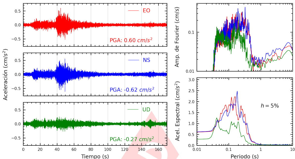
Figura A.5: Registros tiempo-historia, espectros de Fourier y de respuesta en las direcciones EO, NS y vertical de la estación DEFEN. Sismo de Pisco, Pisco - Ica del 2024-07-19, 08:54:25 (Hora local)
