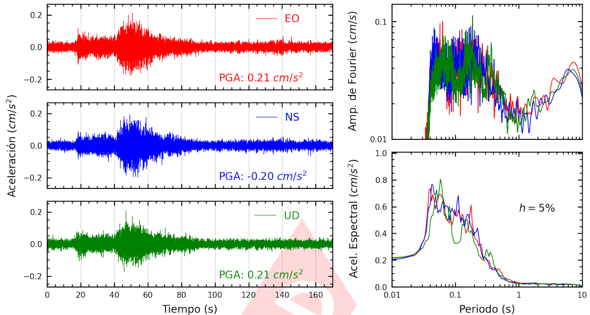
Figura A.21: Registros tiempo-historia, espectros de Fourier y de respuesta en las direcciones EO, NS y vertical de la estación IMCA. Sismo de Pisco, Pisco - Ica del 2024-07-19, 08:54:25 (Hora local)
