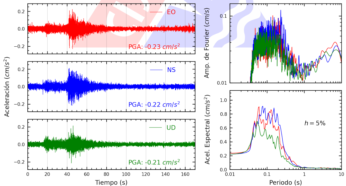
Figura A.20: Registros tiempo-historia, espectros de Fourier y de respuesta en las direcciones EO, NS y vertical de la estación SERVI. Sismo de Pisco, Pisco - Ica del 2024-07-19, 08:54:25 (Hora local)
