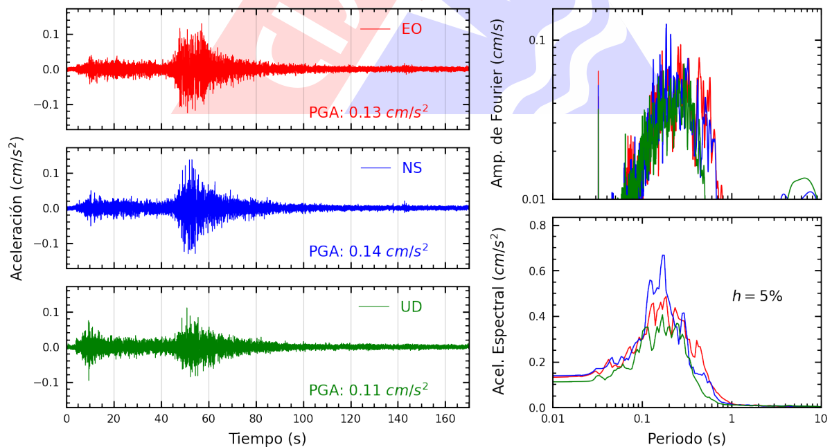
Figura A.22: Registros tiempo-historia, espectros de Fourier y de respuesta en las direcciones EO, NS y vertical de la estación CARAL. Sismo de Pisco, Pisco - Ica del 2024-07-19, 08:54:25 (Hora local)
