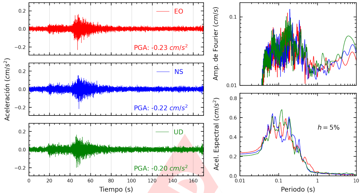
Figura A.19: Registros tiempo-historia, espectros de Fourier y de respuesta en las direcciones EO, NS y vertical de la estación UNFV. Sismo de Pisco, Pisco - Ica del 2024-07-19, 08:54:25 (Hora local)
