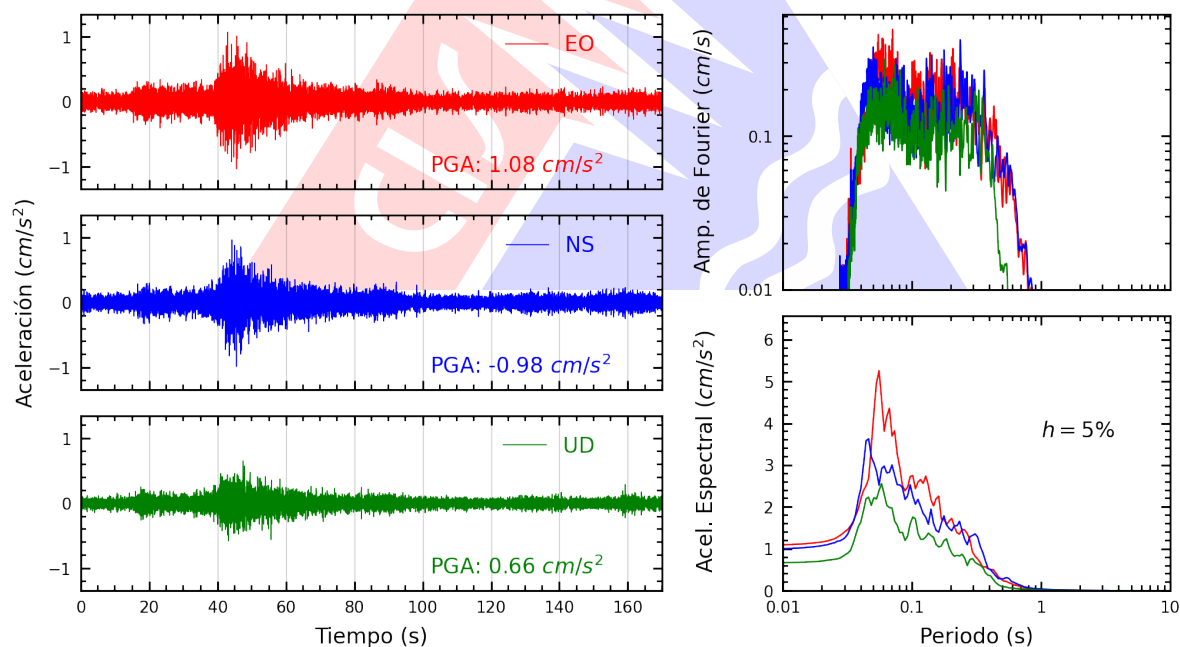
Figura A.2: Registros tiempo-historia, espectros de Fourier y de respuesta en las direcciones EO, NS y vertical de la estación UNTEL. Sismo de Pisco, Pisco - Ica del 2024-07-19, 08:54:25 (Hora local)
