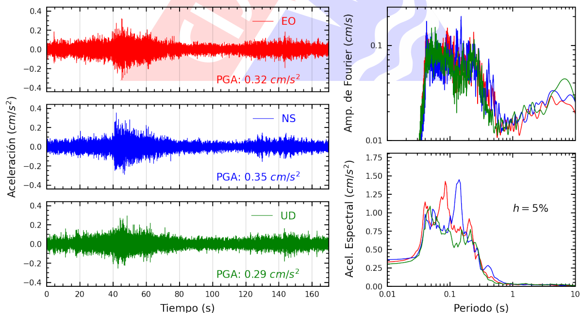
Figura A.8: Registros tiempo-historia, espectros de Fourier y de respuesta en las direcciones EO, NS y vertical de la estación URPPE. Sismo de Pisco, Pisco - Ica del 2024-07-19, 08:54:25 (Hora local)
