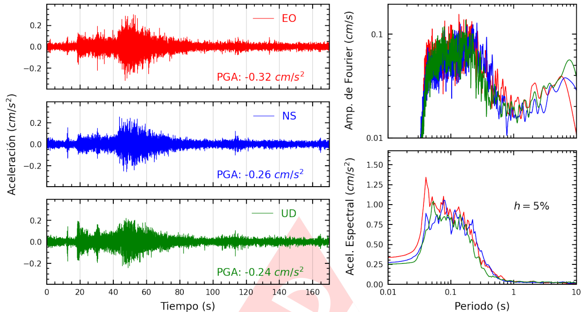
Figura A.11: Registros tiempo-historia, espectros de Fourier y de respuesta en las direcciones EO, NS y vertical de la estación UCV. Sismo de Pisco, Pisco - Ica del 2024-07-19, 08:54:25 (Hora local)
