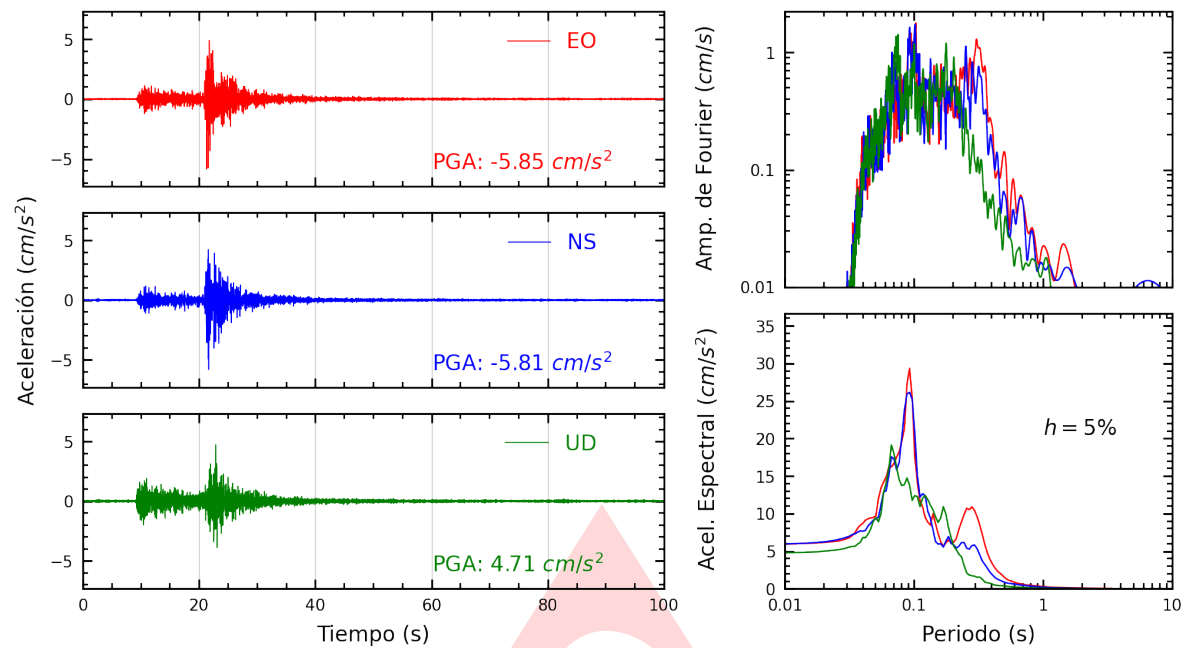
Figura A.1: Registros tiempo-historia, espectros de Fourier y de respuesta en las direcciones EO, NS y vertical de la estación SCTAC. Sismo de Calana, Tacna - Tacna del 2024-07-20, 21:53:43 (Hora local)
