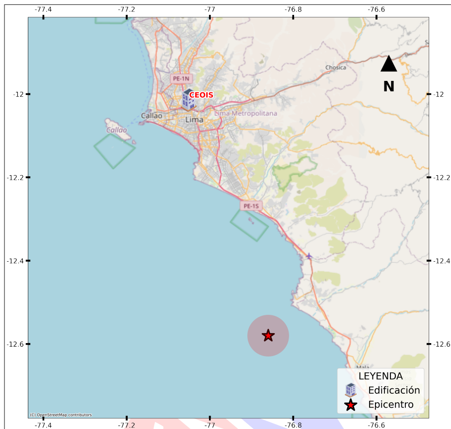
Figura 2: Mapa de ubicación de la edificación monitoreada a nivel nacional correspondiente(s) al Sismo de Chilca, Cañete - Lima del 23 de julio de 2024 a las 12:34:55 (hora local)
