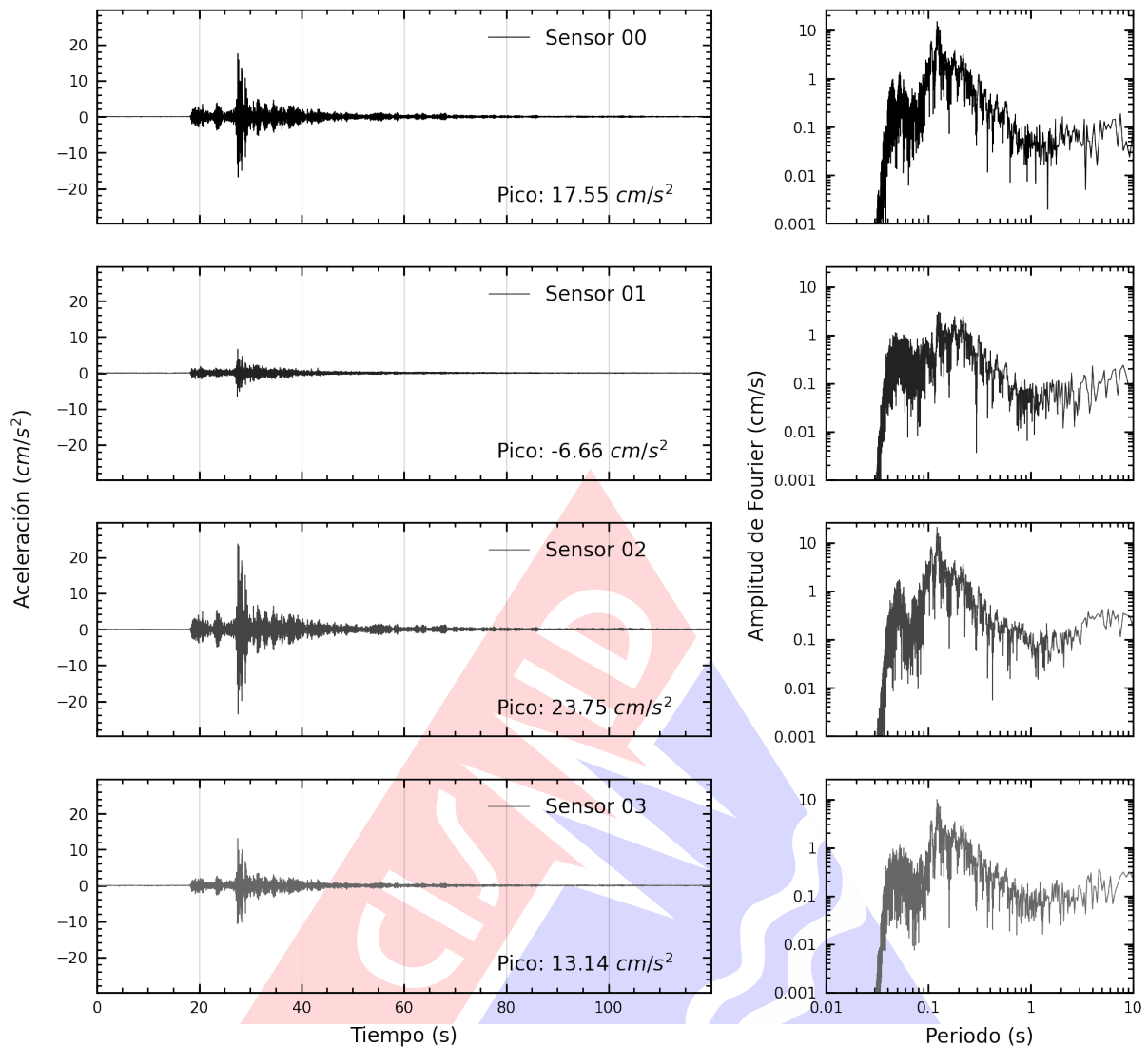
Figura A.3: Registros tiempo-historia y espectros de Fourier en la dirección vertical de la edificación Centro de Información e Investigación de la FIC-UNI. Sismo de Chilca, Cañete - Lima del 2024-07-23, 12:34:55 (Hora local)
