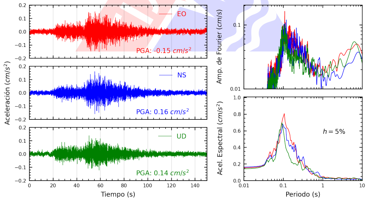
Figura A.20: Registros tiempo-historia, espectros de Fourier y de respuesta en las direcciones EO, NS y vertical de la estación AMORE. Sismo de Pisco, Pisco - Ica del 2024-07-24, 05:40:17 (Hora local)
