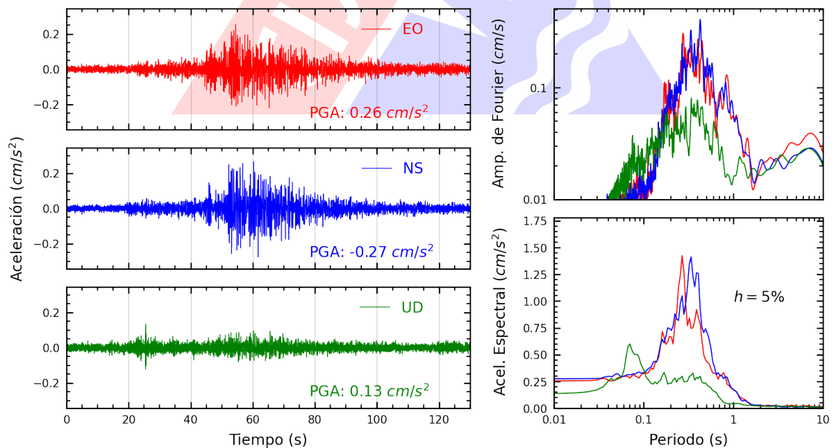
Figura A.8: Registros tiempo-historia, espectros de Fourier y de respuesta en las direcciones EO, NS y vertical de la estación ACAPU. Sismo de Pisco, Pisco - Ica del 2024-07-24, 05:40:17 (Hora local)
