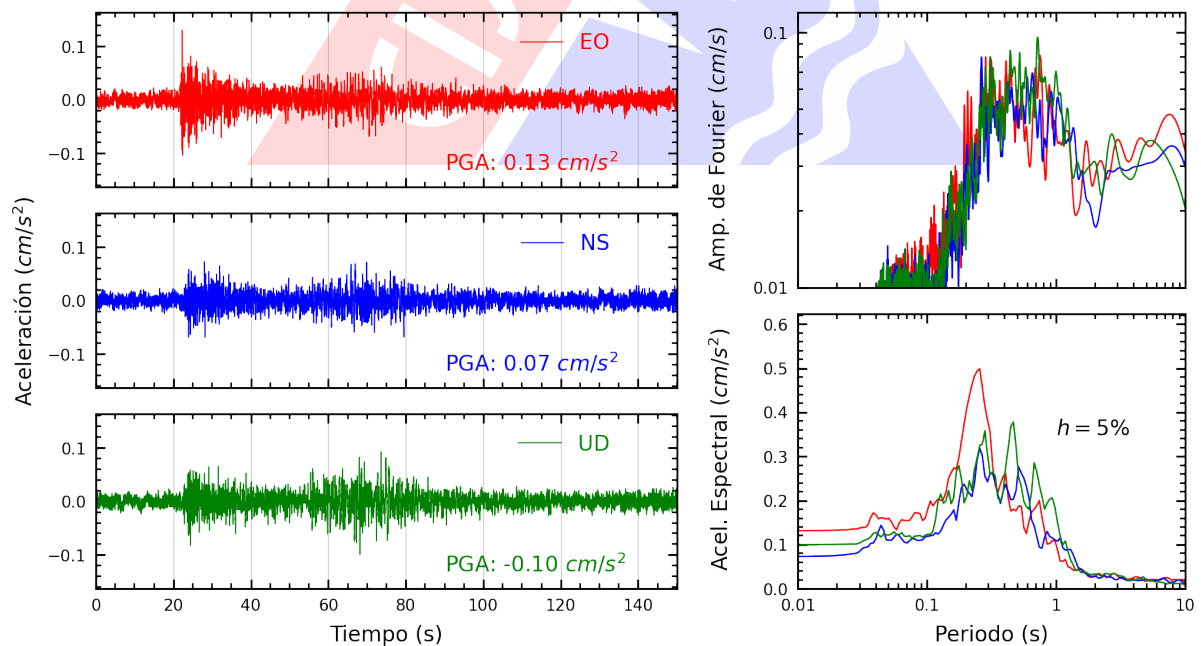
Figura A.22: Registros tiempo-historia, espectros de Fourier y de respuesta en las direcciones EO, NS y vertical de la estación UNSCH. Sismo de Pisco, Pisco - Ica del 2024-07-24, 05:40:17 (Hora local)
