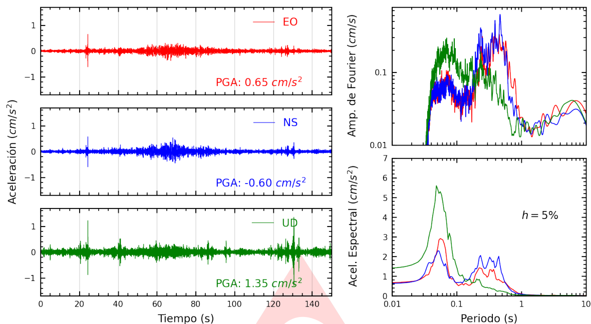
Figura A.1: Registros tiempo-historia, espectros de Fourier y de respuesta en las direcciones EO, NS y vertical de la estación MDPP. Sismo de Pisco, Pisco - Ica del 2024-07-24, 05:40:17 (Hora local)
