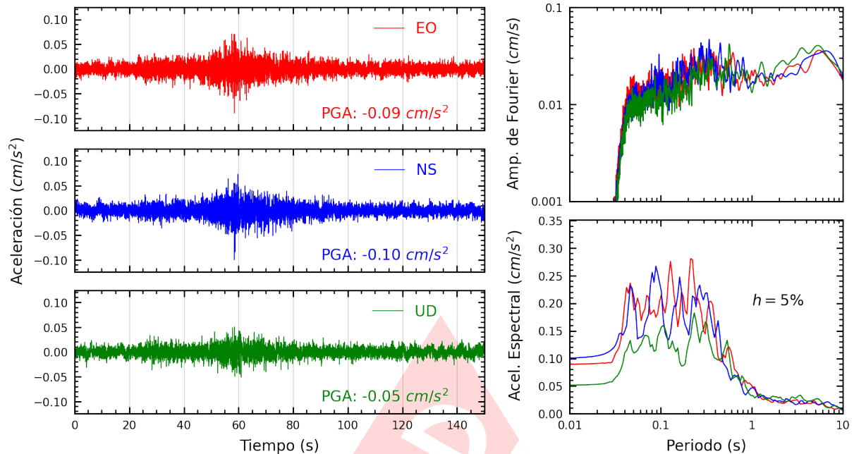
Figura A.23: Registros tiempo-historia, espectros de Fourier y de respuesta en las direcciones EO, NS y vertical de la estación UCSS. Sismo de Pisco, Pisco - Ica del 2024-07-24, 05:40:17 (Hora local)
