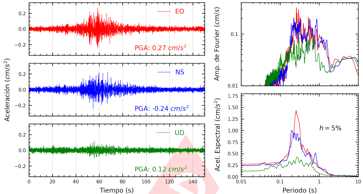
Figura A.9: Registros tiempo-historia, espectros de Fourier y de respuesta en las direcciones EO, NS y vertical de la estación DSMI. Sismo de Pisco, Pisco - Ica del 2024-07-24, 05:40:17 (Hora local)
