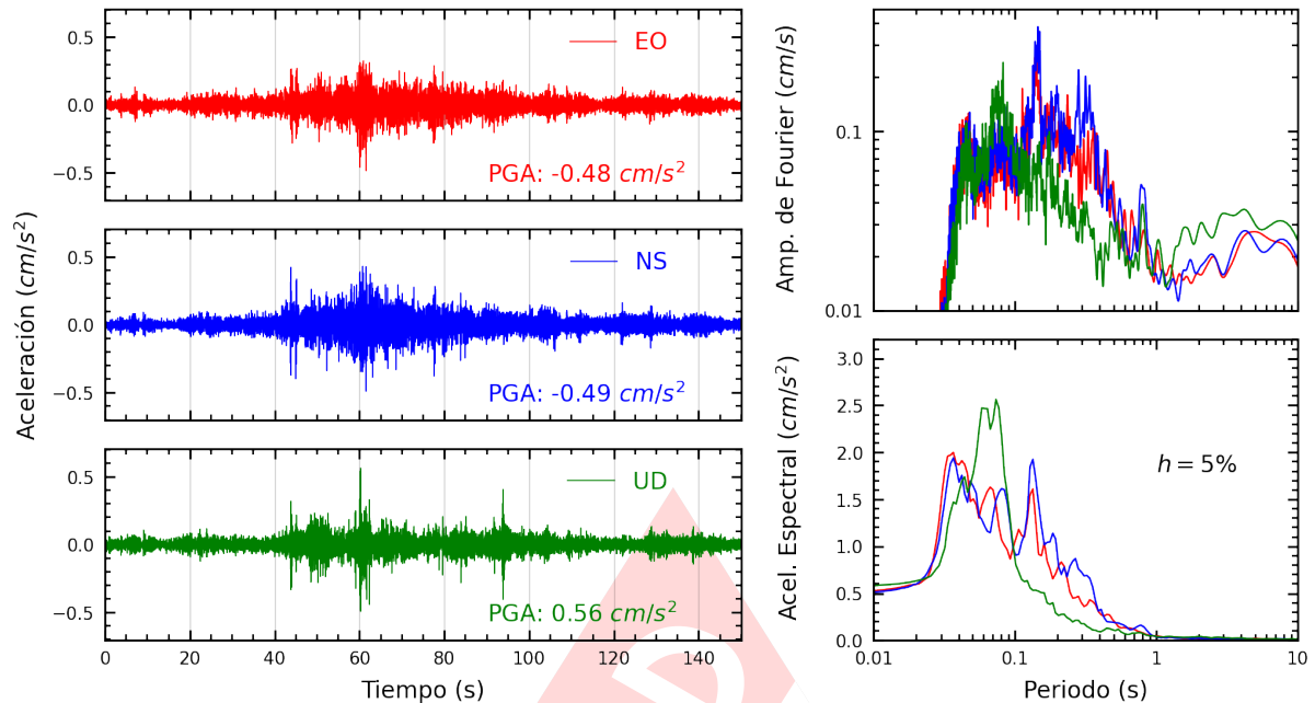
Figura A.3: Registros tiempo-historia, espectros de Fourier y de respuesta en las direcciones EO, NS y vertical de la estación CARAB. Sismo de Pisco, Pisco - Ica del 2024-07-24, 05:40:17 (Hora local)
