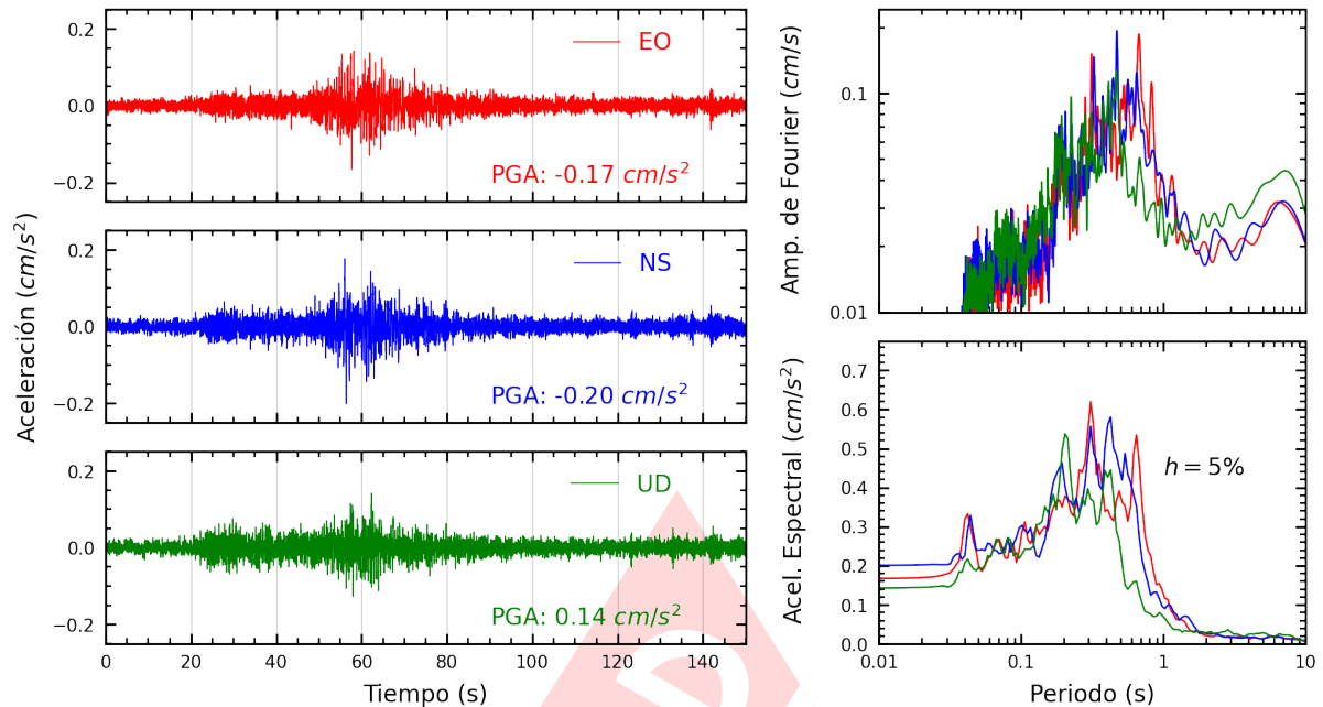
Figura A.15: Registros tiempo-historia, espectros de Fourier y de respuesta en las direcciones EO, NS y vertical de la estación UNFV. Sismo de Pisco, Pisco - Ica del 2024-07-24, 05:40:17 (Hora local)
