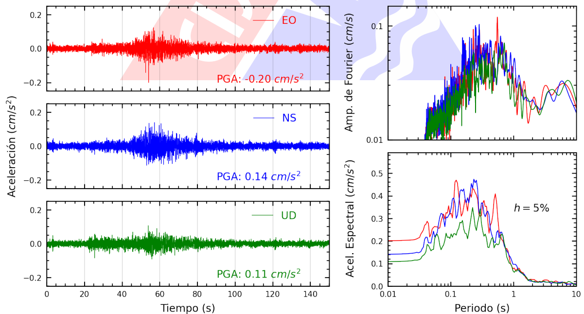
Figura A.16: Registros tiempo-historia, espectros de Fourier y de respuesta en las direcciones EO, NS y vertical de la estación SERVI. Sismo de Pisco, Pisco - Ica del 2024-07-24, 05:40:17 (Hora local)
