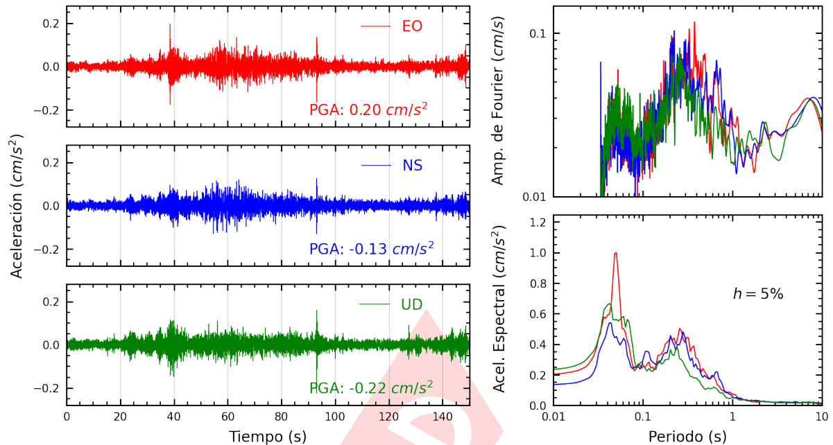
Figura A.11: Registros tiempo-historia, espectros de Fourier y de respuesta en las direcciones EO, NS y vertical de la estación USMP. Sismo de Pisco, Pisco - Ica del 2024-07-24, 05:40:17 (Hora local)
