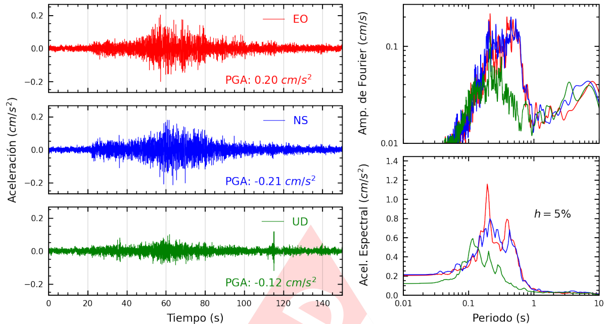
Figura A.13: Registros tiempo-historia, espectros de Fourier y de respuesta en las direcciones EO, NS y vertical de la estación VHAYA. Sismo de Pisco, Pisco - Ica del 2024-07-24, 05:40:17 (Hora local)
