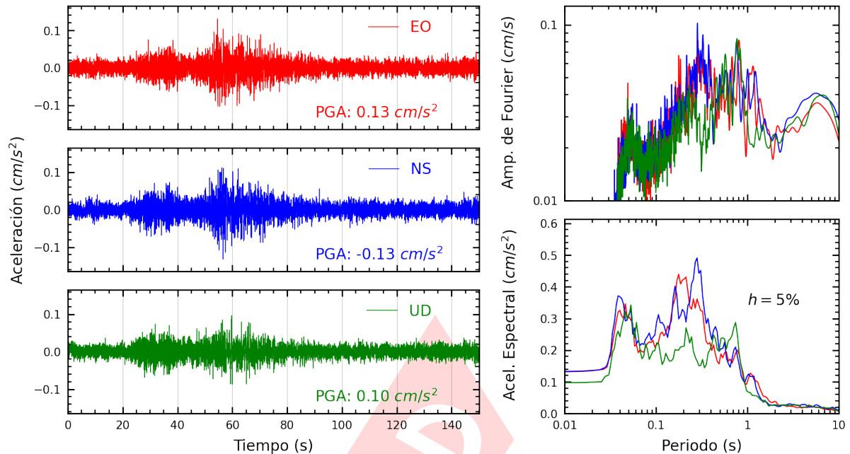
Figura A.21: Registros tiempo-historia, espectros de Fourier y de respuesta en las direcciones EO, NS y vertical de la estación CENEP. Sismo de Pisco, Pisco - Ica del 2024-07-24, 05:40:17 (Hora local)
