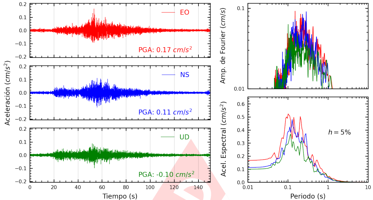
Figura A.17: Registros tiempo-historia, espectros de Fourier y de respuesta en las direcciones EO, NS y vertical de la estación JALV2. Sismo de Pisco, Pisco - Ica del 2024-07-24, 05:40:17 (Hora local)
