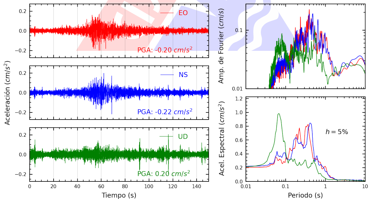
Figura A.12: Registros tiempo-historia, espectros de Fourier y de respuesta en las direcciones EO, NS y vertical de la estación RAMON. Sismo de Pisco, Pisco - Ica del 2024-07-24, 05:40:17 (Hora local)
