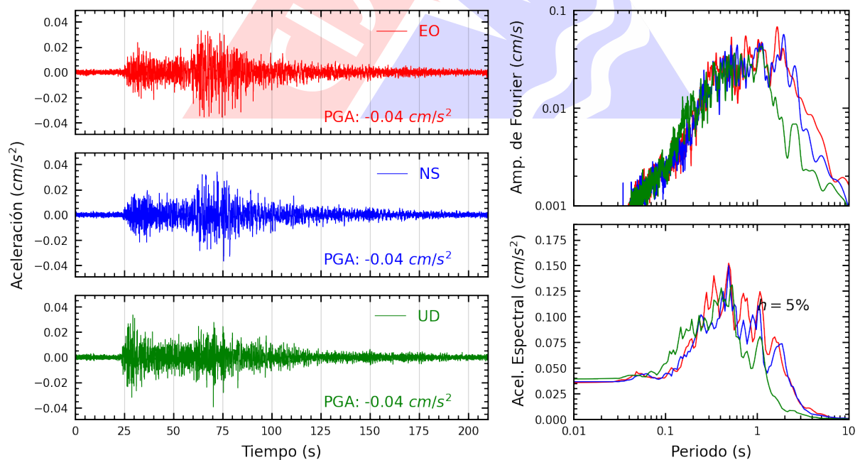
Figura A.24: Registros tiempo-historia, espectros de Fourier y de respuesta en las direcciones EO, NS y vertical de la estación UNCP. Sismo de Pisco, Pisco - Ica del 2024-07-24, 05:40:17 (Hora local)
