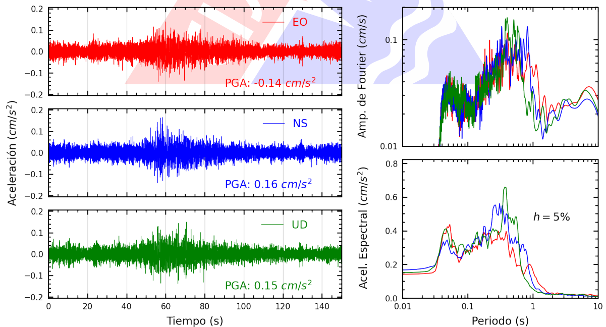
Figura A.18: Registros tiempo-historia, espectros de Fourier y de respuesta en las direcciones EO, NS y vertical de la estación IMCA. Sismo de Pisco, Pisco - Ica del 2024-07-24, 05:40:17 (Hora local)
