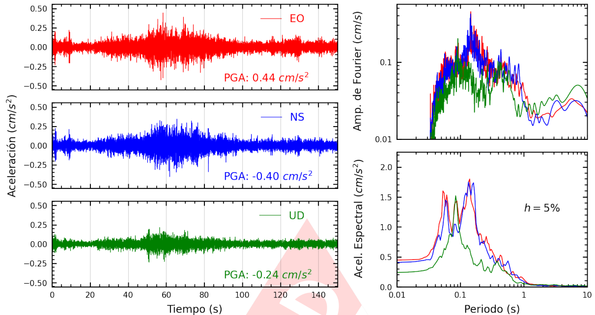
Figura A.5: Registros tiempo-historia, espectros de Fourier y de respuesta en las direcciones EO, NS y vertical de la estación USILM. Sismo de Pisco, Pisco - Ica del 2024-07-24, 05:40:17 (Hora local)
