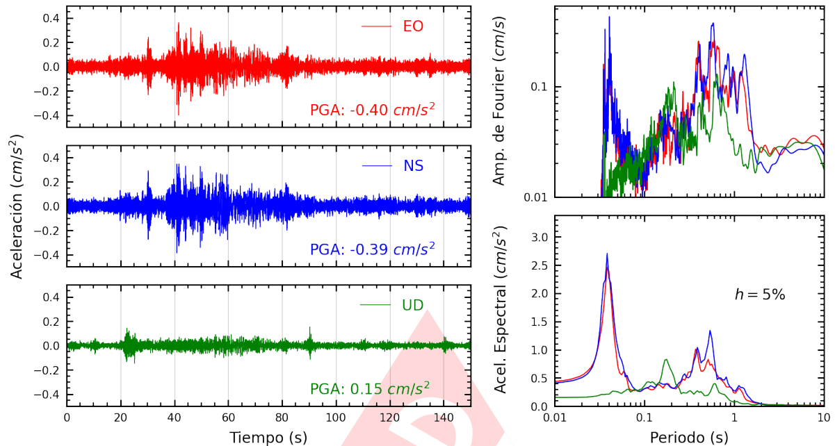
Figura A.7: Registros tiempo-historia, espectros de Fourier y de respuesta en las direcciones EO, NS y vertical de la estación DHNPE. Sismo de Pisco, Pisco - Ica del 2024-07-24, 05:40:17 (Hora local)
