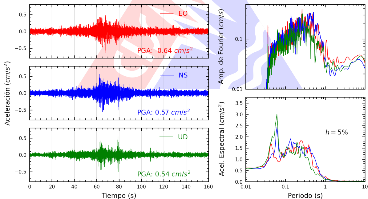
Figura A.2: Registros tiempo-historia, espectros de Fourier y de respuesta en las direcciones EO, NS y vertical de la estación PUNTA. Sismo de Pisco, Pisco - Ica del 2024-07-24, 05:40:17 (Hora local)
