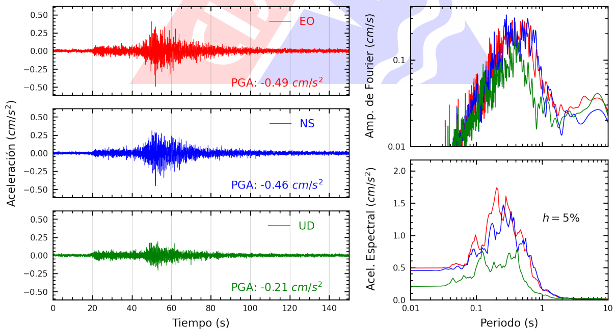
Figura A.4: Registros tiempo-historia, espectros de Fourier y de respuesta en las direcciones EO, NS y vertical de la estación USILP. Sismo de Pisco, Pisco - Ica del 2024-07-24, 05:40:17 (Hora local)
