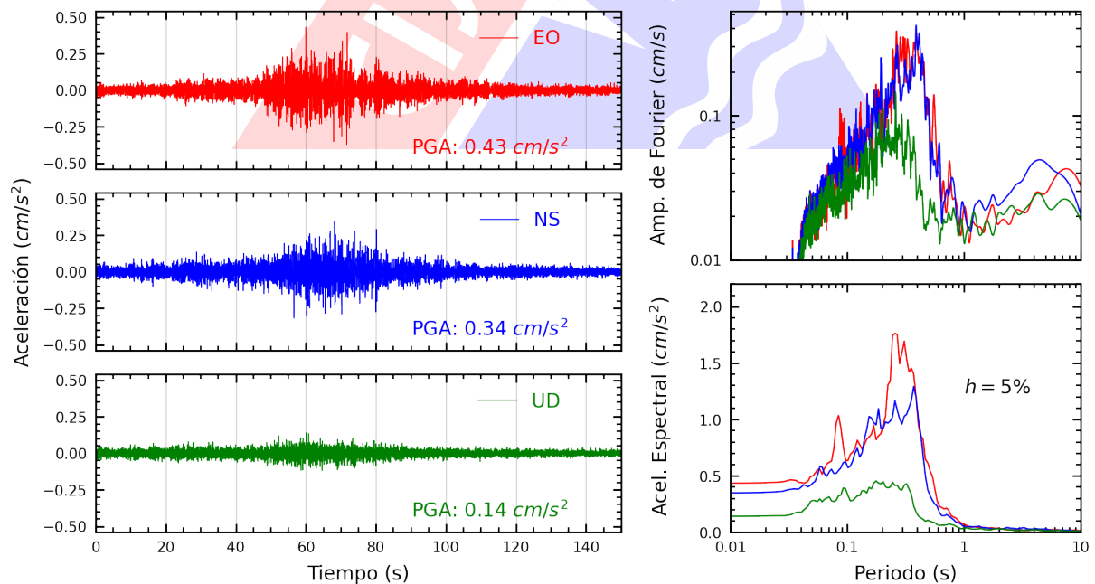
Figura A.6: Registros tiempo-historia, espectros de Fourier y de respuesta en las direcciones EO, NS y vertical de la estación DEFEN. Sismo de Pisco, Pisco - Ica del 2024-07-24, 05:40:17 (Hora local)
