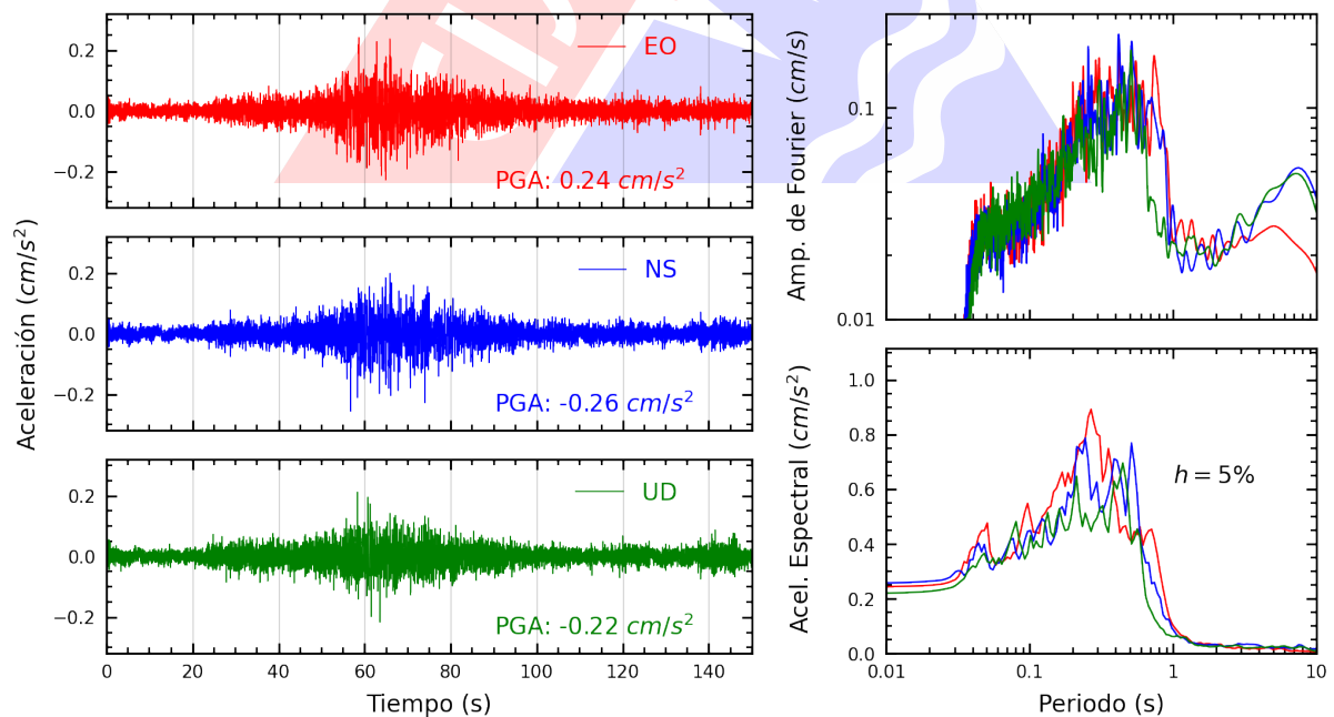
Figura A.10: Registros tiempo-historia, espectros de Fourier y de respuesta en las direcciones EO, NS y vertical de la estación UCV. Sismo de Pisco, Pisco - Ica del 2024-07-24, 05:40:17 (Hora local)
