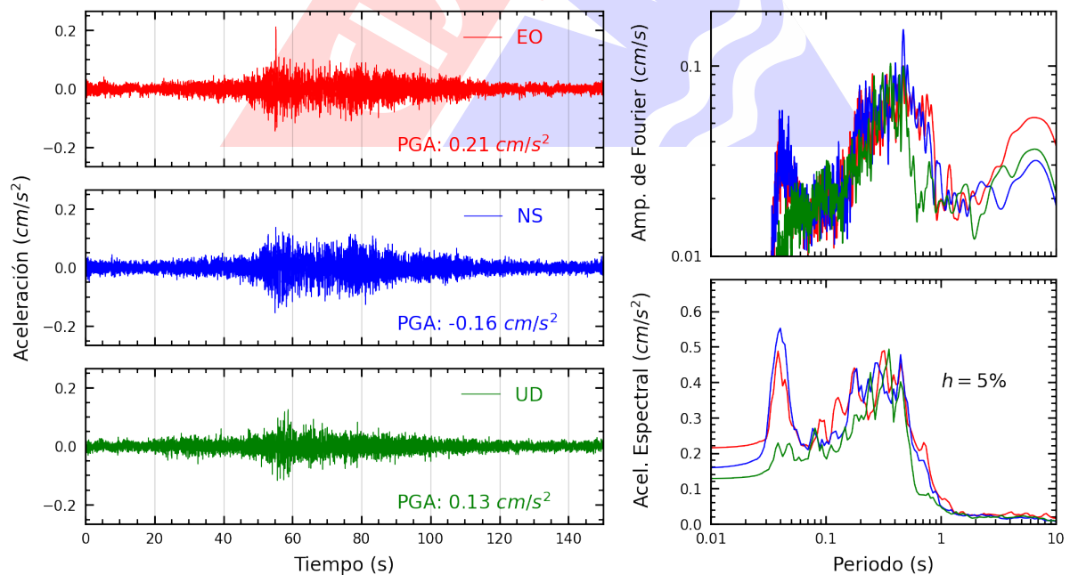
Figura A.14: Registros tiempo-historia, espectros de Fourier y de respuesta en las direcciones EO, NS y vertical de la estación COMAS. Sismo de Pisco, Pisco - Ica del 2024-07-24, 05:40:17 (Hora local)
