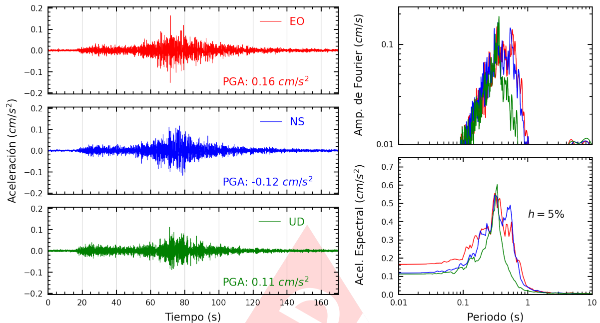
Figura A.19: Registros tiempo-historia, espectros de Fourier y de respuesta en las direcciones EO, NS y vertical de la estación CARAL. Sismo de Pisco, Pisco - Ica del 2024-07-24, 05:40:17 (Hora local)
