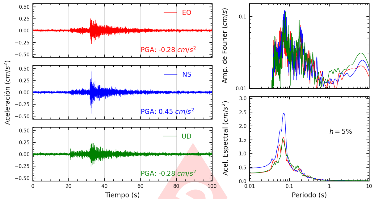
Figura A.25: Registros tiempo-historia, espectros de Fourier y de respuesta en las direcciones EO, NS y vertical de la estación UNFV. Sismo de Mala, Cañete - Lima del 2024-07-28, 19:05:18 (Hora local)
