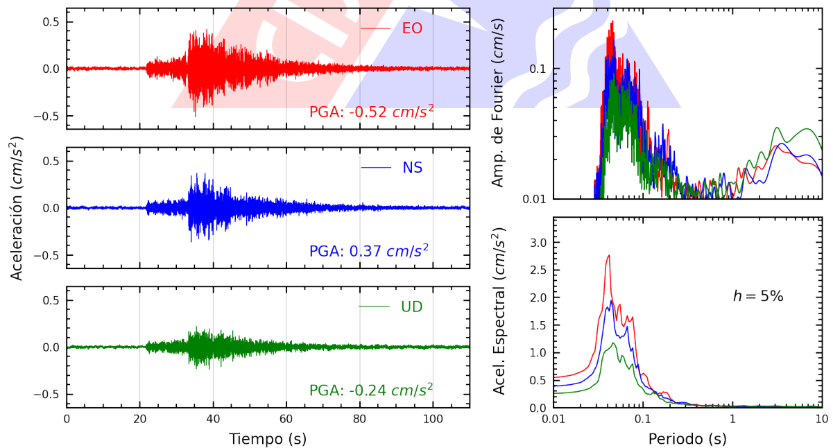
Figura A.20: Registros tiempo-historia, espectros de Fourier y de respuesta en las direcciones EO, NS y vertical de la estación UCSS. Sismo de Mala, Cañete - Lima del 2024-07-28, 19:05:18 (Hora local)
