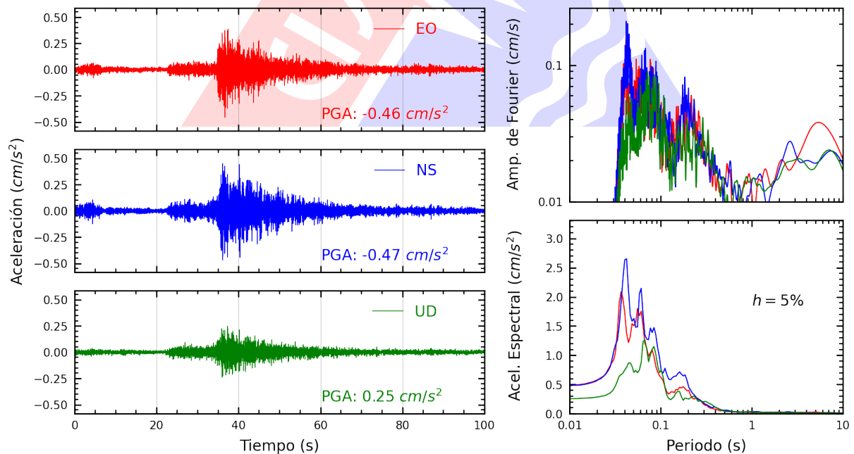
Figura A.22: Registros tiempo-historia, espectros de Fourier y de respuesta en las direcciones EO, NS y vertical de la estación COMAS. Sismo de Mala, Cañete - Lima del 2024-07-28, 19:05:18 (Hora local)
