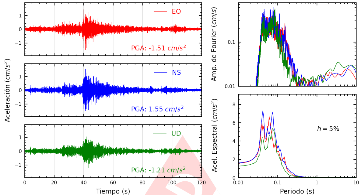
Figura A.3: Registros tiempo-historia, espectros de Fourier y de respuesta en las direcciones EO, NS y vertical de la estación SROSA. Sismo de Mala, Cañete - Lima del 2024-07-28, 19:05:18 (Hora local)
