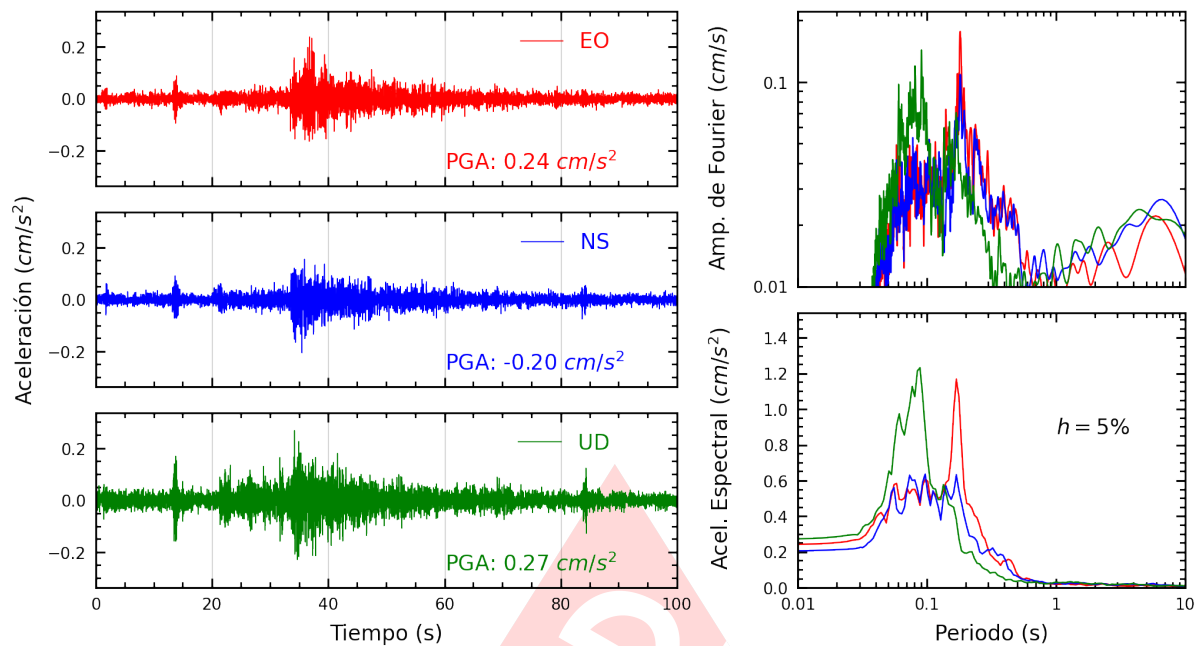
Figura A.31: Registros tiempo-historia, espectros de Fourier y de respuesta en las direcciones EO, NS y vertical de la estación RAMON. Sismo de Mala, Cañete - Lima del 2024-07-28, 19:05:18 (Hora local)
