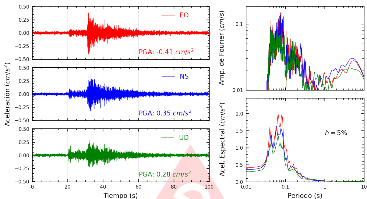
Figura A.27: Registros tiempo-historia, espectros de Fourier y de respuesta en las direcciones EO, NS y vertical de la estación CENEP. Sismo de Mala, Cañete - Lima del 2024-07-28, 19:05:18 (Hora local)
