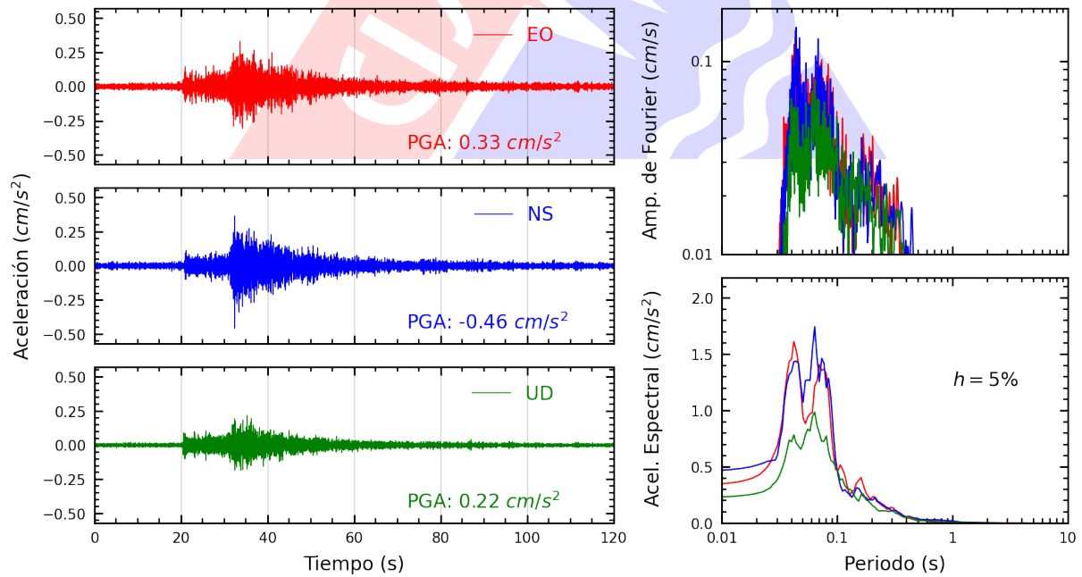
Figura A.24: Registros tiempo-historia, espectros de Fourier y de respuesta en las direcciones EO, NS y vertical de la estación BORJA. Sismo de Mala, Cañete - Lima del 2024-07-28, 19:05:18 (Hora local)
