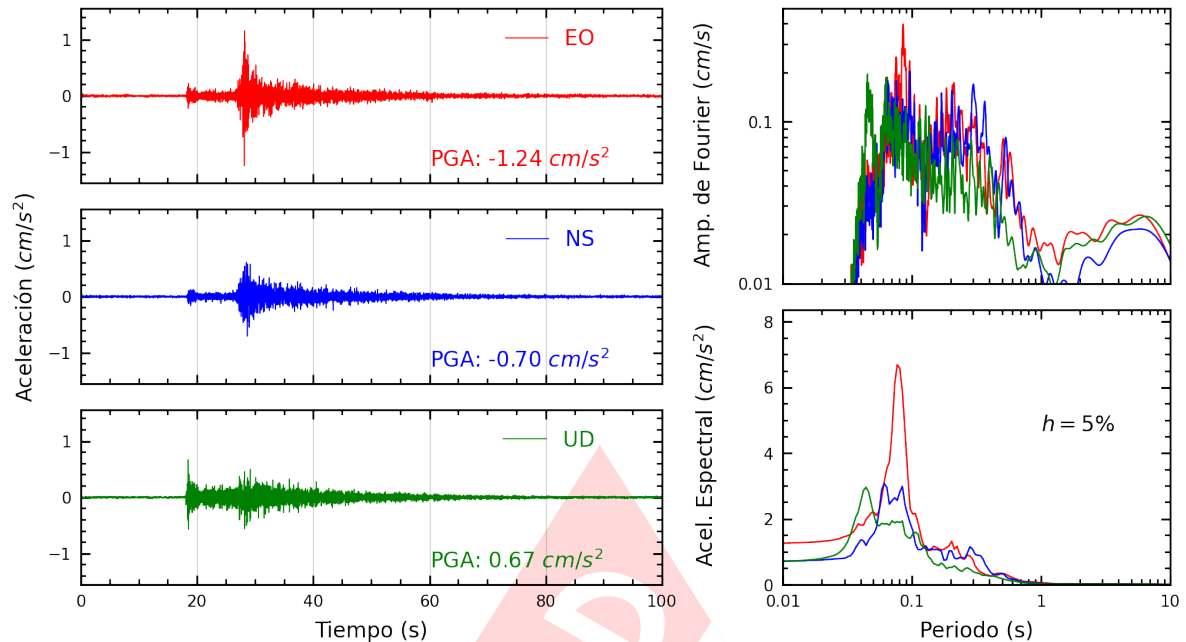
Figura A.7: Registros tiempo-historia, espectros de Fourier y de respuesta en las direcciones EO, NS y vertical de la estación USILP. Sismo de Mala, Cañete - Lima del 2024-07-28, 19:05:18 (Hora local)
