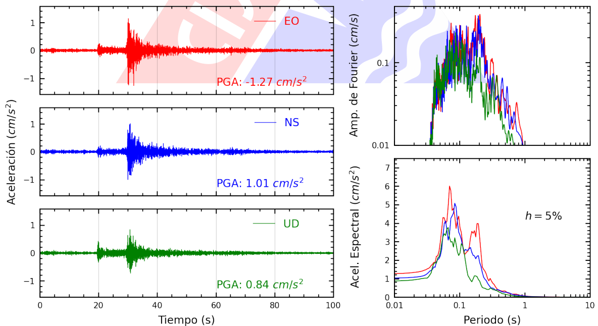
Figura A.6: Registros tiempo-historia, espectros de Fourier y de respuesta en las direcciones EO, NS y vertical de la estación SCCHO. Sismo de Mala, Cañete - Lima del 2024-07-28, 19:05:18 (Hora local)
