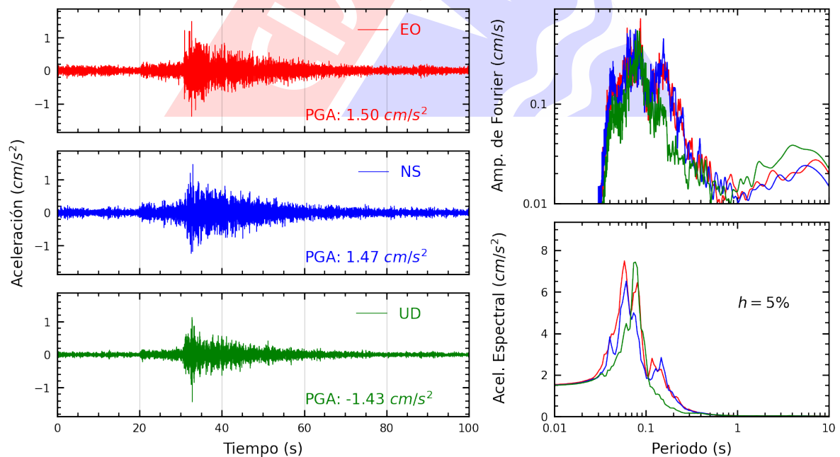
Figura A.4: Registros tiempo-historia, espectros de Fourier y de respuesta en las direcciones EO, NS y vertical de la estación USILM. Sismo de Mala, Cañete - Lima del 2024-07-28, 19:05:18 (Hora local)
