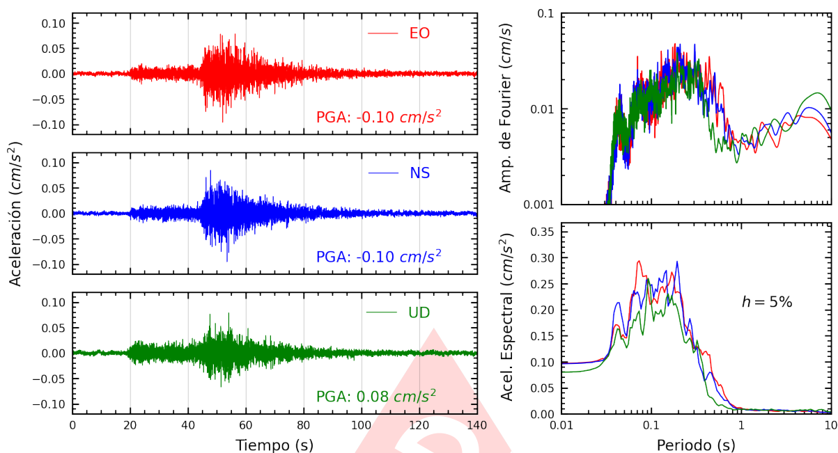
Figura A.33: Registros tiempo-historia, espectros de Fourier y de respuesta en las direcciones EO, NS y vertical de la estación CARAL. Sismo de Mala, Cañete - Lima del 2024-07-28, 19:05:18 (Hora local)
