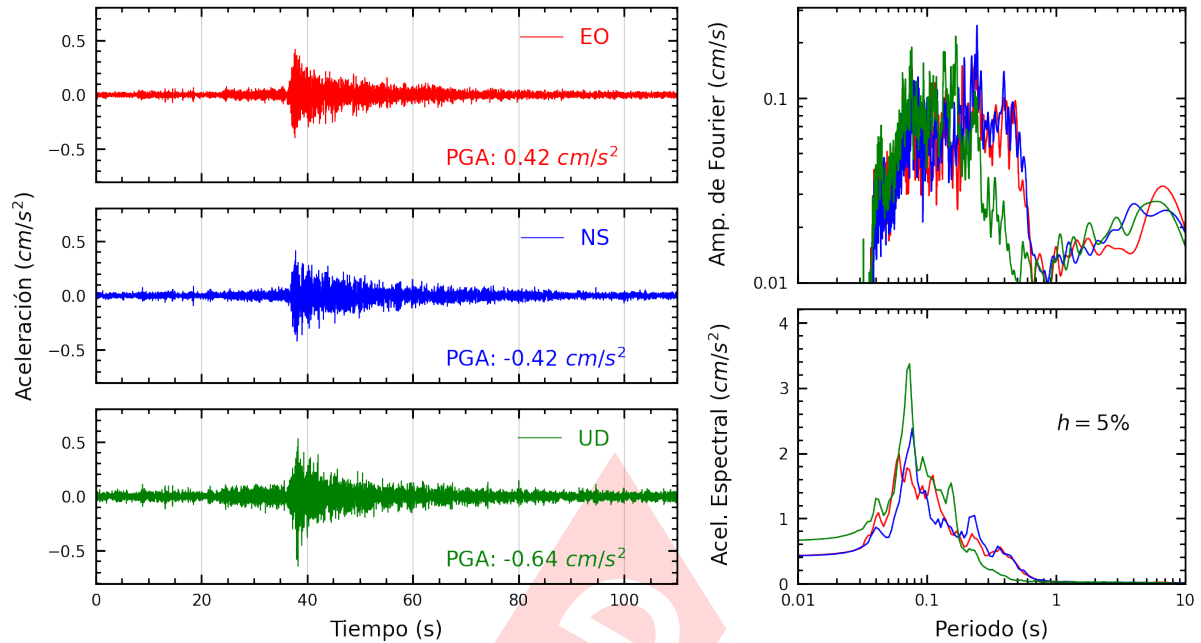
Figura A.19: Registros tiempo-historia, espectros de Fourier y de respuesta en las direcciones EO, NS y vertical de la estación MDPP. Sismo de Mala, Cañete - Lima del 2024-07-28, 19:05:18 (Hora local)
