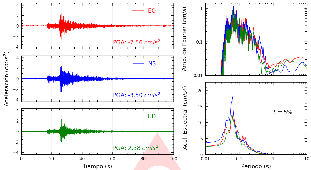
Figura A.1: Registros tiempo-historia, espectros de Fourier y de respuesta en las direcciones EO, NS y vertical de la estación PUNTA. Sismo de Mala, Cañete - Lima del 2024-07-28, 19:05:18 (Hora local)
