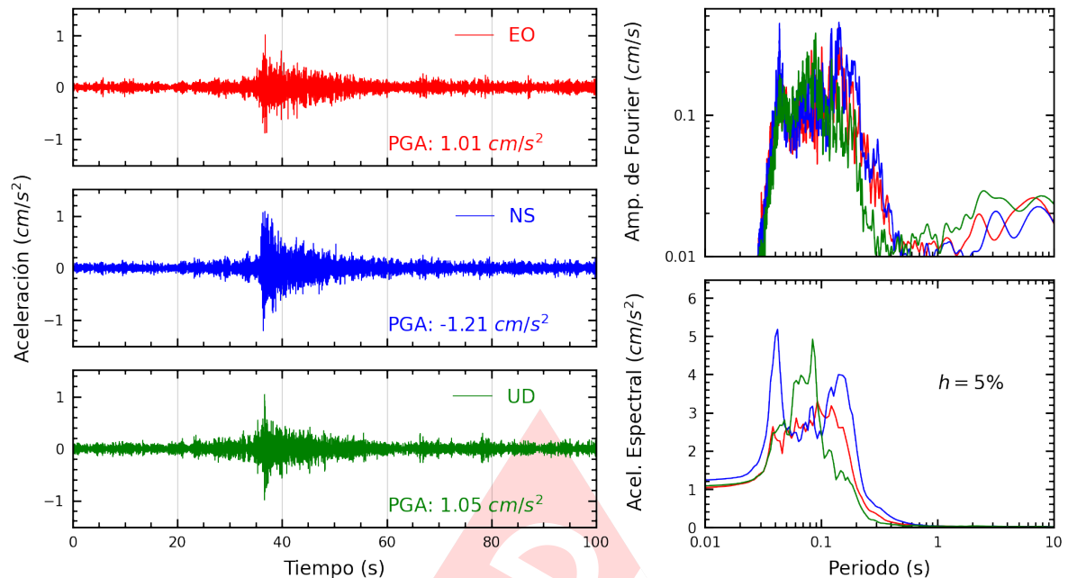
Figura A.9: Registros tiempo-historia, espectros de Fourier y de respuesta en las direcciones EO, NS y vertical de la estación CARAB. Sismo de Mala, Cañete - Lima del 2024-07-28, 19:05:18 (Hora local)
