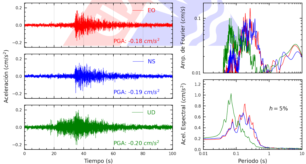
Figura A.32: Registros tiempo-historia, espectros de Fourier y de respuesta en las direcciones EO, NS y vertical de la estación ACAPU. Sismo de Mala, Cañete - Lima del 2024-07-28, 19:05:18 (Hora local)
