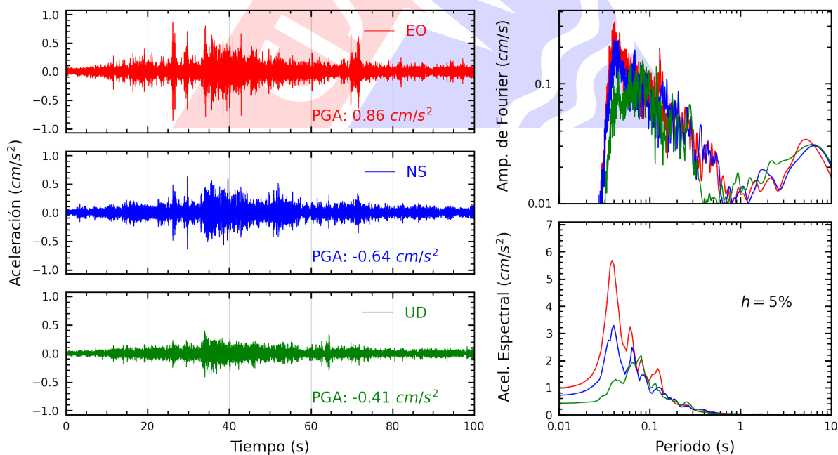
Figura A.14: Registros tiempo-historia, espectros de Fourier y de respuesta en las direcciones EO, NS y vertical de la estación OLIVO. Sismo de Mala, Cañete - Lima del 2024-07-28, 19:05:18 (Hora local)
