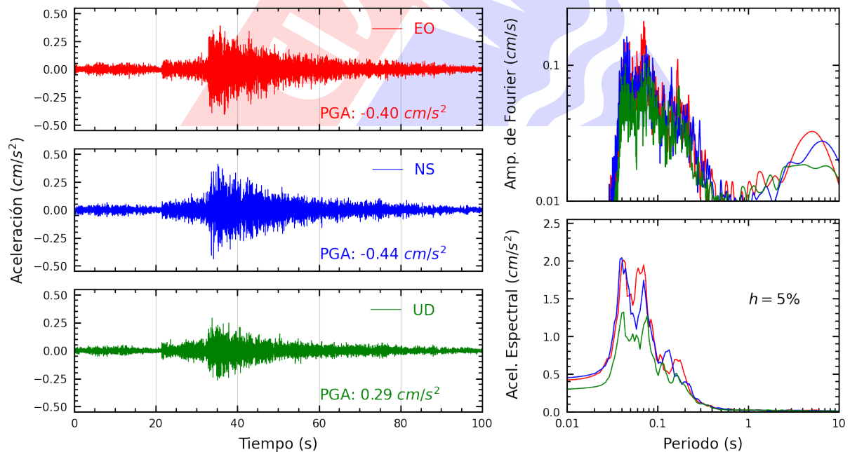
Figura A.26: Registros tiempo-historia, espectros de Fourier y de respuesta en las direcciones EO, NS y vertical de la estación FICPE. Sismo de Mala, Cañete - Lima del 2024-07-28, 19:05:18 (Hora local)
