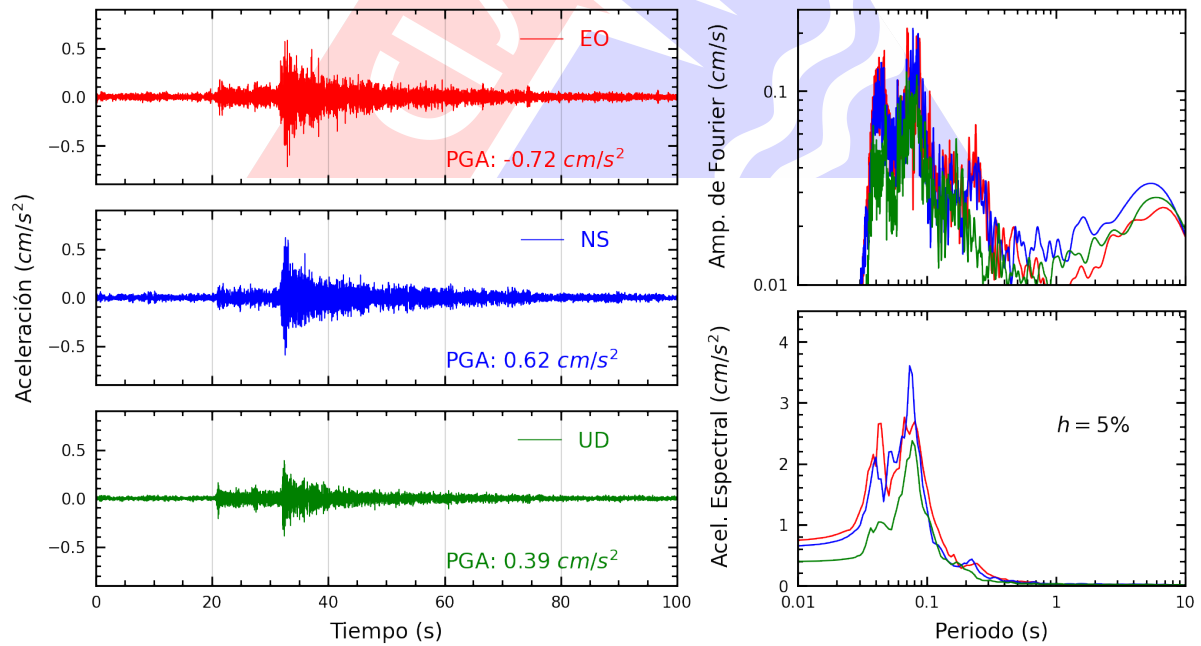
Figura A.16: Registros tiempo-historia, espectros de Fourier y de respuesta en las direcciones EO, NS y vertical de la estación CEPRE. Sismo de Mala, Cañete - Lima del 2024-07-28, 19:05:18 (Hora local)
