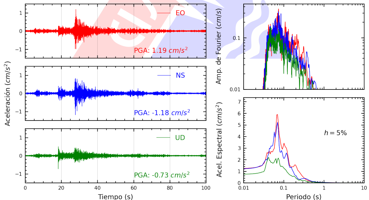
Figura A.10: Registros tiempo-historia, espectros de Fourier y de respuesta en las direcciones EO, NS y vertical de la estación PACHA. Sismo de Mala, Cañete - Lima del 2024-07-28, 19:05:18 (Hora local)
