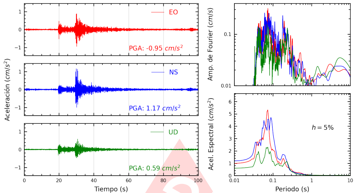
Figura A.11: Registros tiempo-historia, espectros de Fourier y de respuesta en las direcciones EO, NS y vertical de la estación UPCVI. Sismo de Mala, Cañete - Lima del 2024-07-28, 19:05:18 (Hora local)
