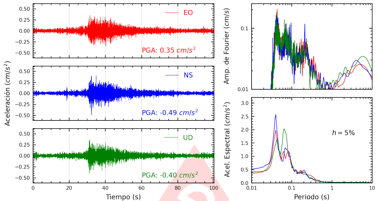
Figura A.21: Registros tiempo-historia, espectros de Fourier y de respuesta en las direcciones EO, NS y vertical de la estación USMP. Sismo de Mala, Cañete - Lima del 2024-07-28, 19:05:18 (Hora local)
