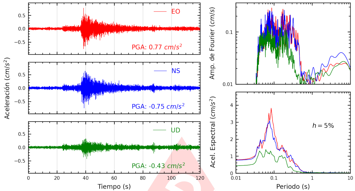
Figura A.15: Registros tiempo-historia, espectros de Fourier y de respuesta en las direcciones EO, NS y vertical de la estación DEFEN. Sismo de Mala, Cañete - Lima del 2024-07-28, 19:05:18 (Hora local)
