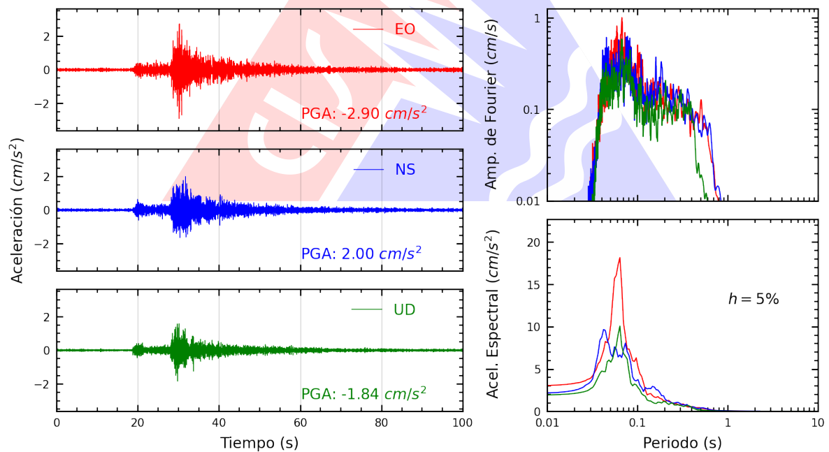
Figura A.2: Registros tiempo-historia, espectros de Fourier y de respuesta en las direcciones EO, NS y vertical de la estación UNTEL. Sismo de Mala, Cañete - Lima del 2024-07-28, 19:05:18 (Hora local)
