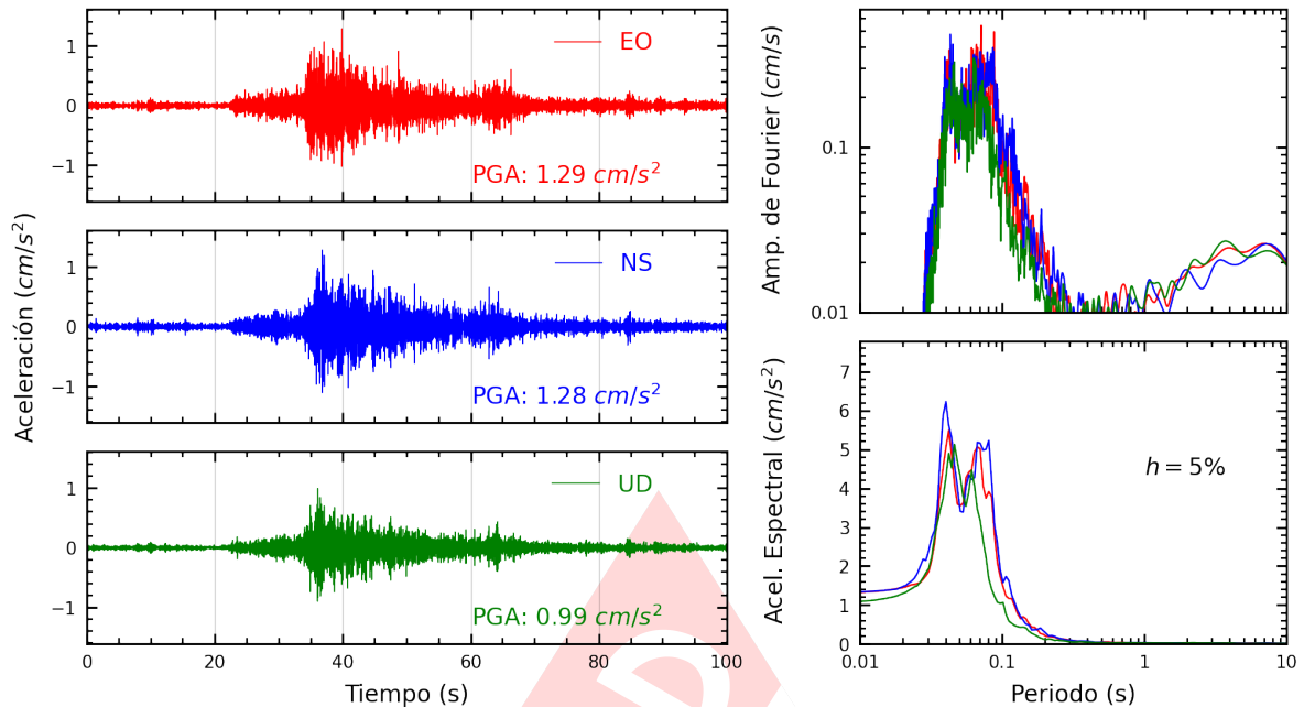
Figura A.5: Registros tiempo-historia, espectros de Fourier y de respuesta en las direcciones EO, NS y vertical de la estación JOSEO. Sismo de Mala, Cañete - Lima del 2024-07-28, 19:05:18 (Hora local)
