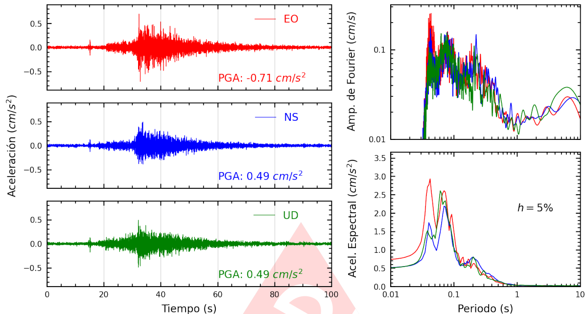
Figura A.17: Registros tiempo-historia, espectros de Fourier y de respuesta en las direcciones EO, NS y vertical de la estación UCV. Sismo de Mala, Cañete - Lima del 2024-07-28, 19:05:18 (Hora local)
