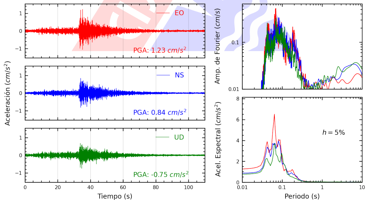
Figura A.8: Registros tiempo-historia, espectros de Fourier y de respuesta en las direcciones EO, NS y vertical de la estación INDEP. Sismo de Mala, Cañete - Lima del 2024-07-28, 19:05:18 (Hora local)
