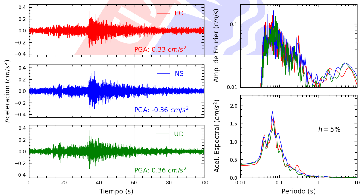
Figura A.28: Registros tiempo-historia, espectros de Fourier y de respuesta en las direcciones EO, NS y vertical de la estación MADRE. Sismo de Mala, Cañete - Lima del 2024-07-28, 19:05:18 (Hora local)
