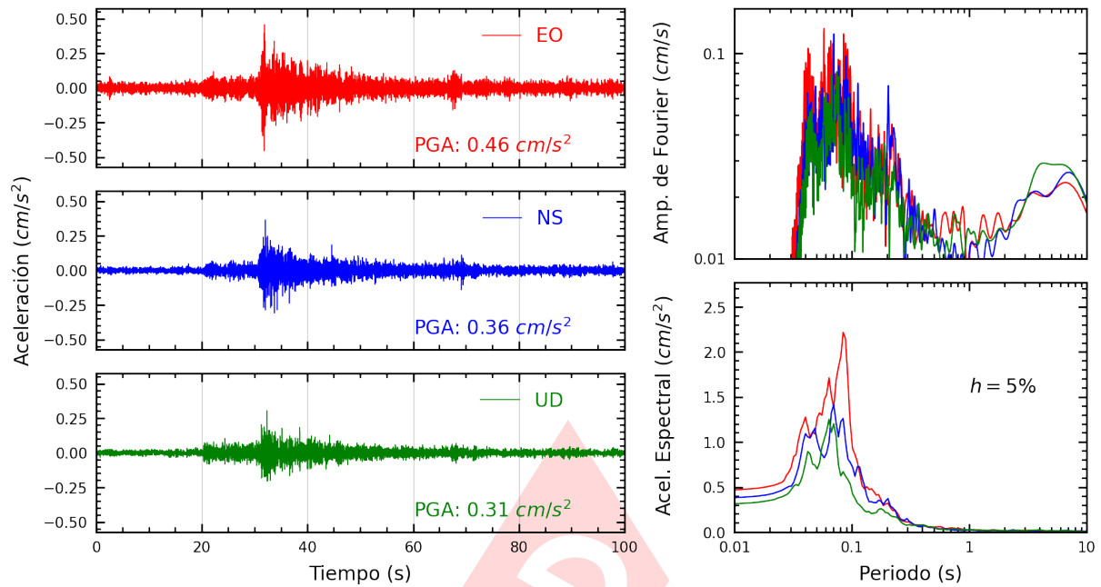
Figura A.23: Registros tiempo-historia, espectros de Fourier y de respuesta en las direcciones EO, NS y vertical de la estación INICT. Sismo de Mala, Cañete - Lima del 2024-07-28, 19:05:18 (Hora local)
