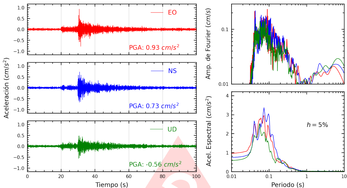
Figura A.13: Registros tiempo-historia, espectros de Fourier y de respuesta en las direcciones EO, NS y vertical de la estación URPE. Sismo de Mala, Cañete - Lima del 2024-07-28, 19:05:18 (Hora local)
