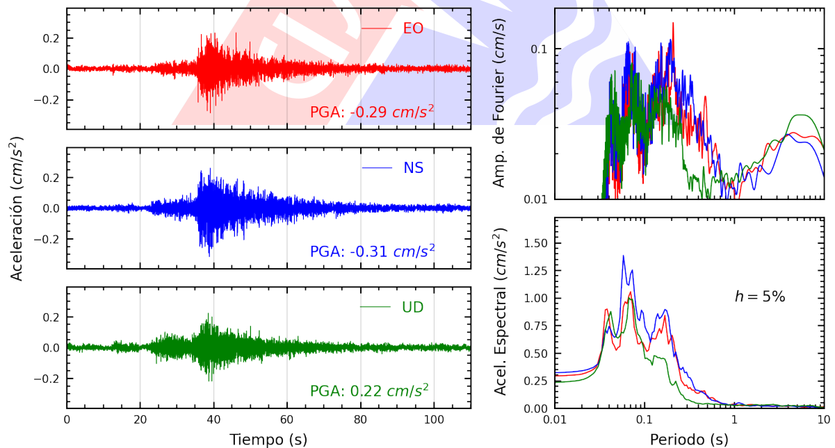
Figura A.30: Registros tiempo-historia, espectros de Fourier y de respuesta en las direcciones EO, NS y vertical de la estación VHAYA. Sismo de Mala, Cañete - Lima del 2024-07-28, 19:05:18 (Hora local)
