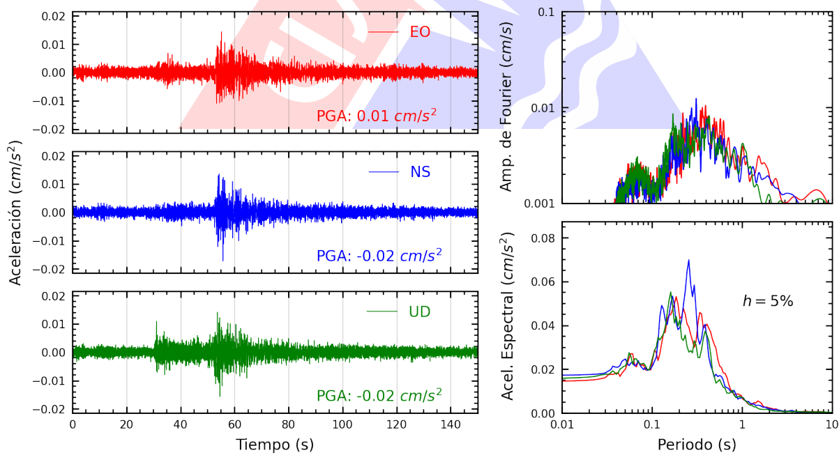
Figura A.34: Registros tiempo-historia, espectros de Fourier y de respuesta en las direcciones EO, NS y vertical de la estación UNCP. Sismo de Mala, Cañete - Lima del 2024-07-28, 19:05:18 (Hora local)
