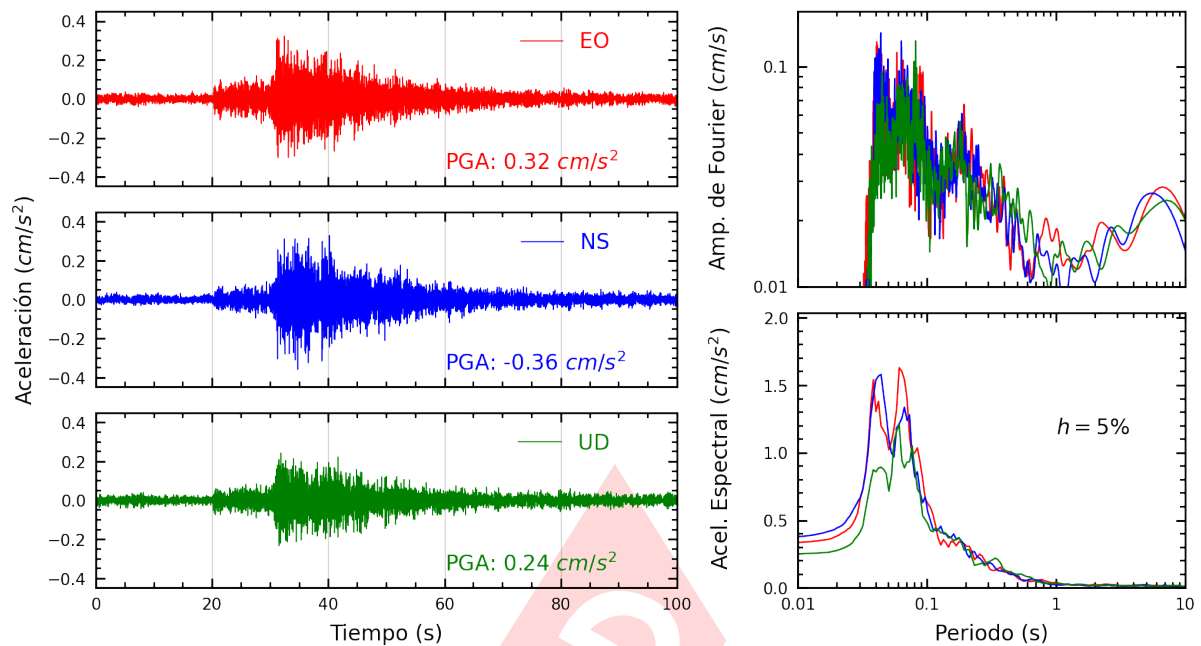
Figura A.29: Registros tiempo-historia, espectros de Fourier y de respuesta en las direcciones EO, NS y vertical de la estación IMCA. Sismo de Mala, Cañete - Lima del 2024-07-28, 19:05:18 (Hora local)
