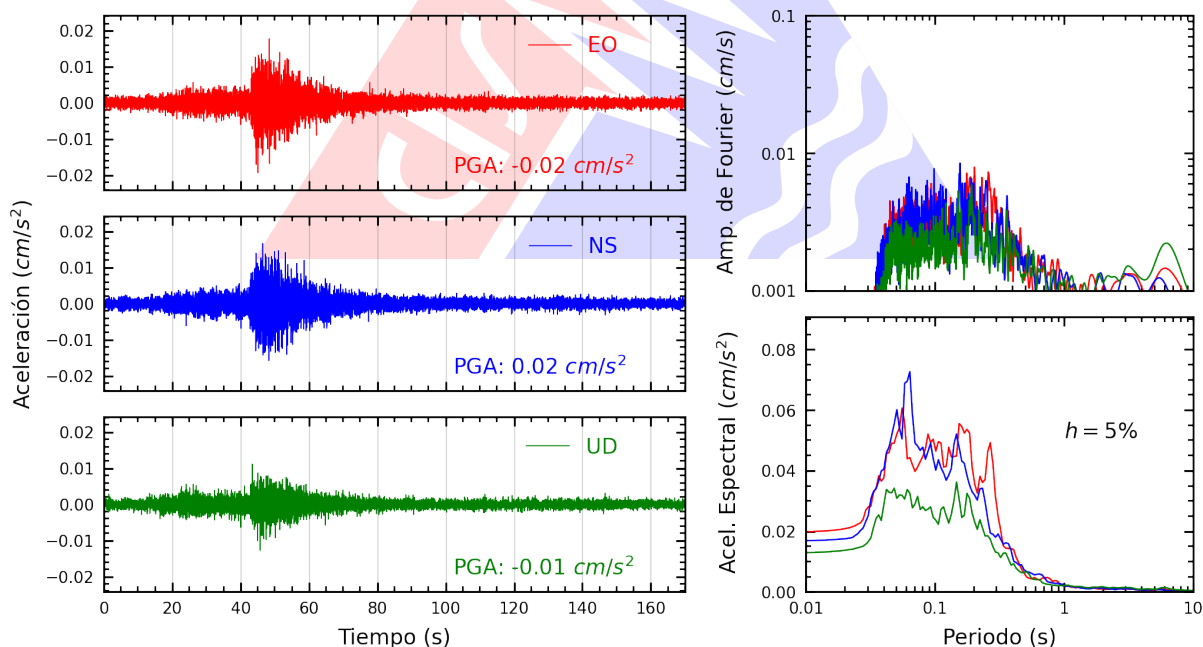
Figura A.2: Registros tiempo-historia, espectros de Fourier y de respuesta en las direcciones EO, NS y vertical de la estación UNSA. Sismo de Pullo, Parinacochas - Ayacucho del 2024-07-30, 22:34:30 (Hora local)
