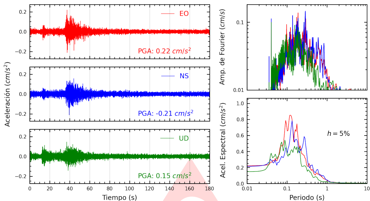
Figura A.1: Registros tiempo-historia, espectros de Fourier y de respuesta en las direcciones EO, NS y vertical de la estación UNICA. Sismo de Pullo, Parinacochas - Ayacucho del 2024-07-30, 22:34:30 (Hora local)
