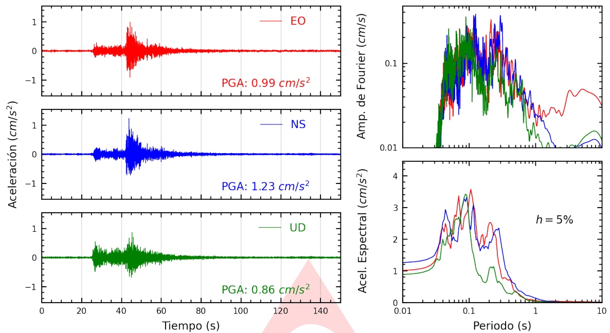
Figura A.1: Registros tiempo-historia, espectros de Fourier y de respuesta en las direcciones EO, NS y vertical de la estación UJBG3. Sismo de Candarave, Candarave - Tacna del 2024-08-06, 06:33:43 (Hora local)
