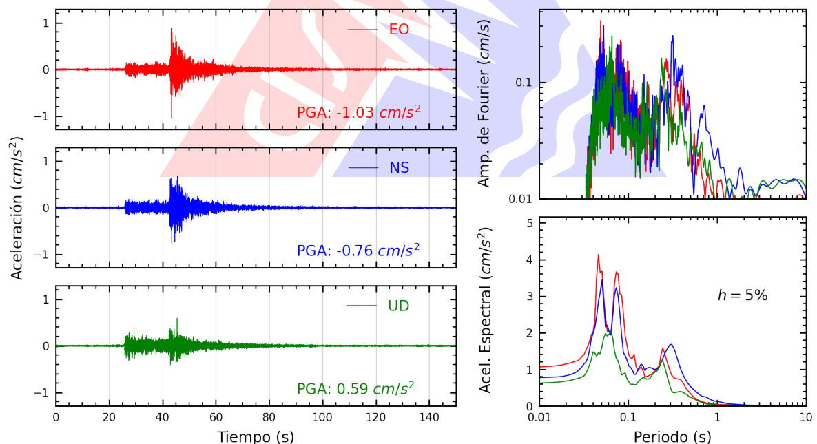
Figura A.2: Registros tiempo-historia, espectros de Fourier y de respuesta en las direcciones EO, NS y vertical de la estación CREY. Sismo de Candarave, Candarave - Tacna del 2024-08-06, 06:33:43 (Hora local)
