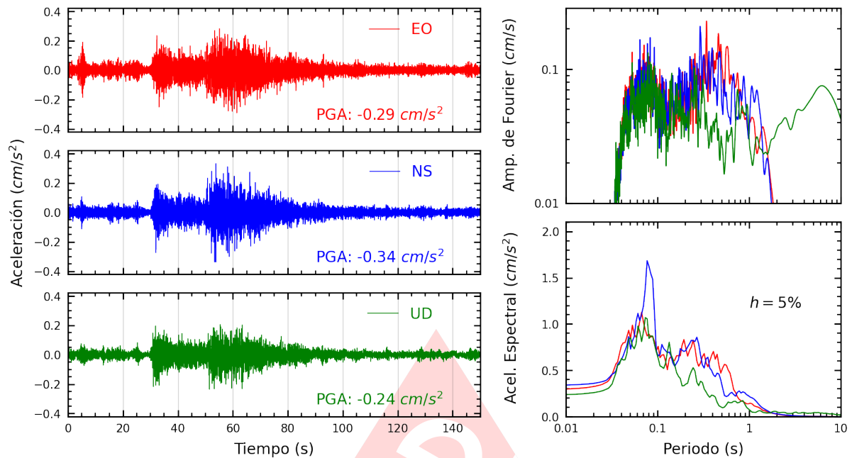
Figura A.5: Registros tiempo-historia, espectros de Fourier y de respuesta en las direcciones EO, NS y vertical de la estación SCARQ. Sismo de Candarave, Candarave - Tacna del 2024-08-06, 06:33:43 (Hora local)
