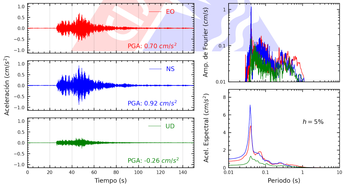
Figura A.4: Registros tiempo-historia, espectros de Fourier y de respuesta en las direcciones EO, NS y vertical de la estación UNAM. Sismo de Candarave, Candarave - Tacna del 2024-08-06, 06:33:43 (Hora local)
