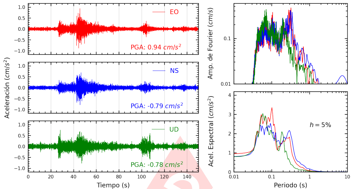
Figura A.3: Registros tiempo-historia, espectros de Fourier y de respuesta en las direcciones EO, NS y vertical de la estación SCTAC. Sismo de Candarave, Candarave - Tacna del 2024-08-06, 06:33:43 (Hora local)
