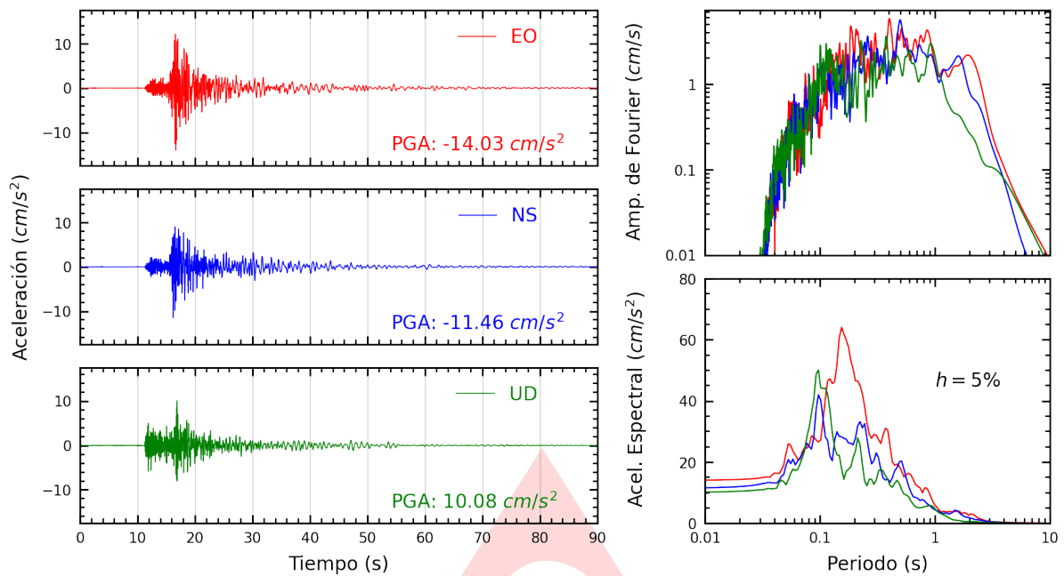
Figura A.1: Registros tiempo-historia, espectros de Fourier y de respuesta en las direcciones EO, NS y vertical de la estación SCCUS. Sismo de Lucre, Quispicanchi - Cusco del 2024-08-13, 01:36:17 (Hora local)
