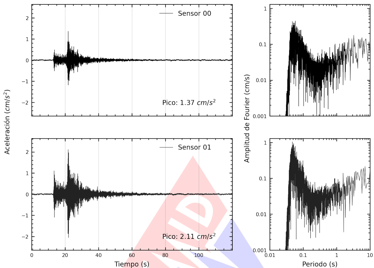
Figura A.3: Registros tiempo-historia y espectros de Fourier en la dirección vertical de la edificación Laboratorio de Estructuras del CISMID-FIC-UNI. Sismo de Chilca, Cañete - Lima del 2024-08-13, 02:05:30 (Hora local)
