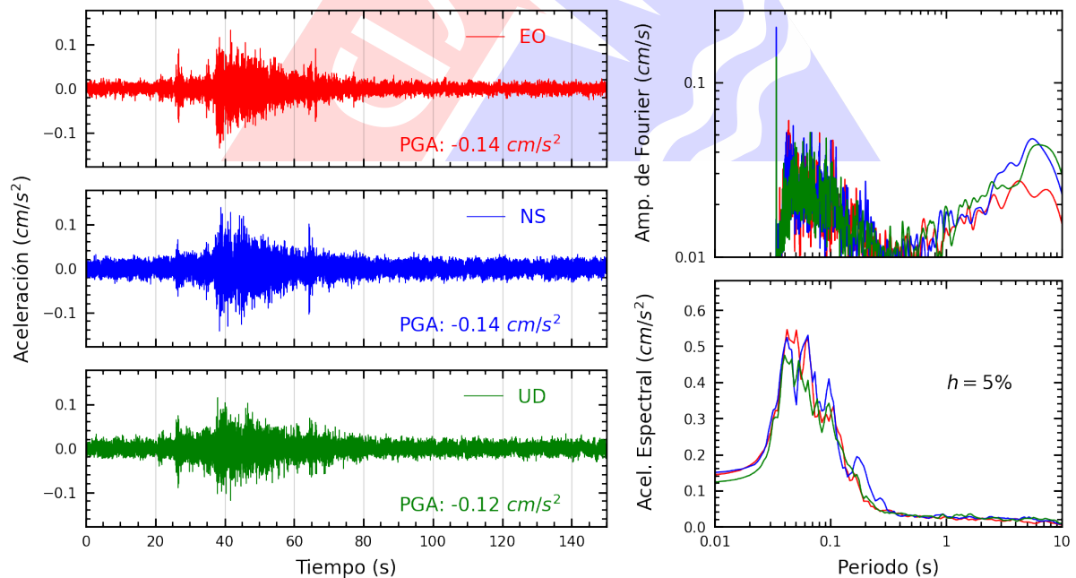
Figura A.20: Registros tiempo-historia, espectros de Fourier y de respuesta en las direcciones EO, NS y vertical de la estación USMP. Sismo de Mala, Cañete - Lima del 2024-08-15, 04:38:57 (Hora local)
