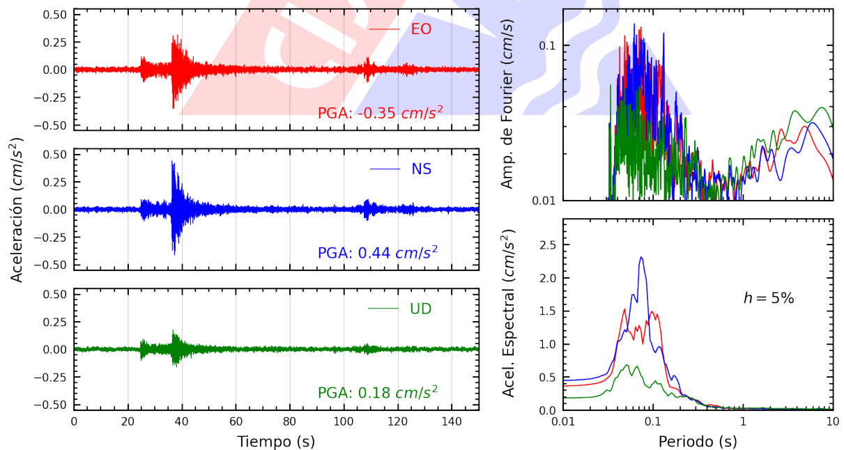
Figura A.6: Registros tiempo-historia, espectros de Fourier y de respuesta en las direcciones EO, NS y vertical de la estación UPCVI. Sismo de Mala, Cañete - Lima del 2024-08-15, 04:38:57 (Hora local)
