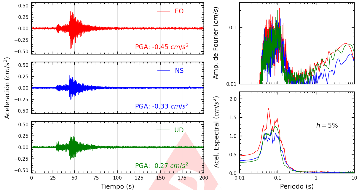
Figura A.5: Registros tiempo-historia, espectros de Fourier y de respuesta en las direcciones EO, NS y vertical de la estación AMORE. Sismo de Mala, Cañete - Lima del 2024-08-15, 04:38:57 (Hora local)
