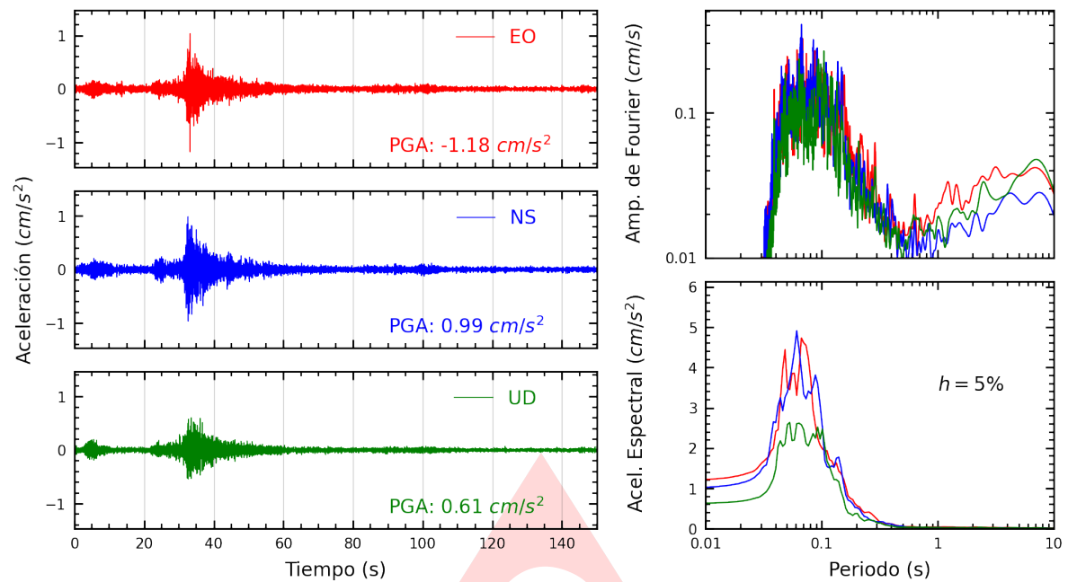
Figura A.1: Registros tiempo-historia, espectros de Fourier y de respuesta en las direcciones EO, NS y vertical de la estación PUNTA. Sismo de Mala, Cañete - Lima del 2024-08-15, 04:38:57 (Hora local)
