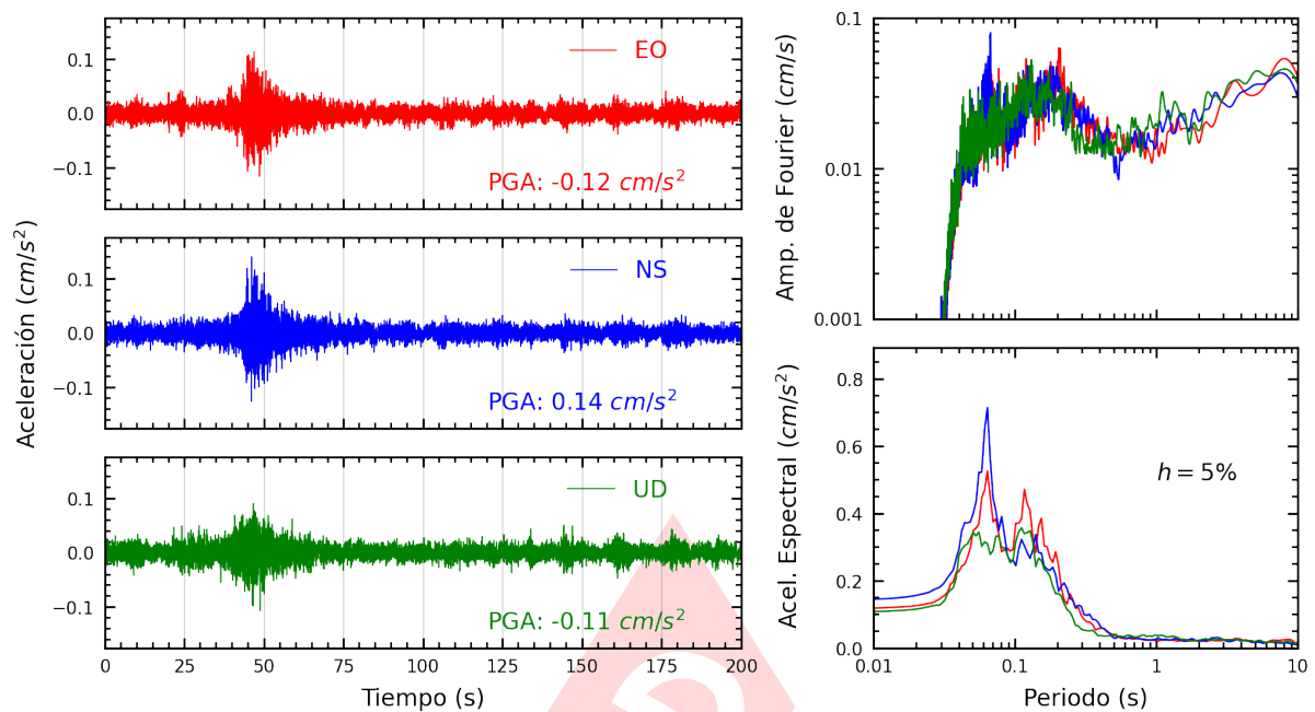
Figura A.21: Registros tiempo-historia, espectros de Fourier y de respuesta en las direcciones EO, NS y vertical de la estación VHAYA. Sismo de Mala, Cañete - Lima del 2024-08-15, 04:38:57 (Hora local)
