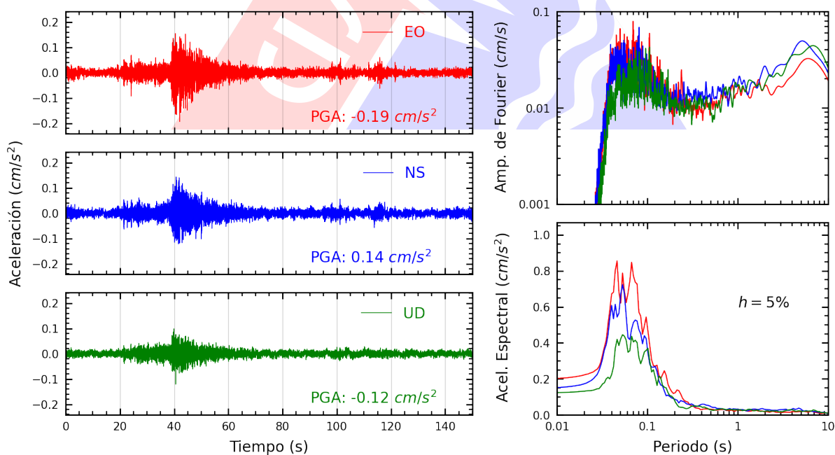
Figura A.16: Registros tiempo-historia, espectros de Fourier y de respuesta en las direcciones EO, NS y vertical de la estación CEPRE. Sismo de Mala, Cañete - Lima del 2024-08-15, 04:38:57 (Hora local)
