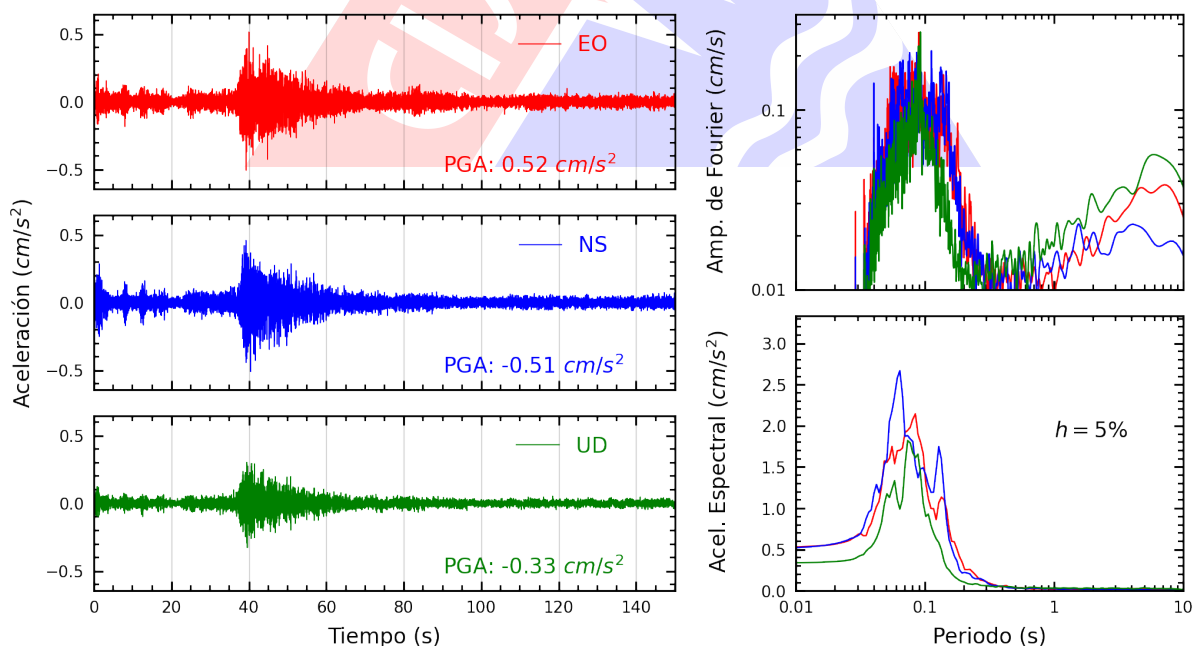
Figura A.4: Registros tiempo-historia, espectros de Fourier y de respuesta en las direcciones EO, NS y vertical de la estación USILM. Sismo de Mala, Cañete - Lima del 2024-08-15, 04:38:57 (Hora local)
