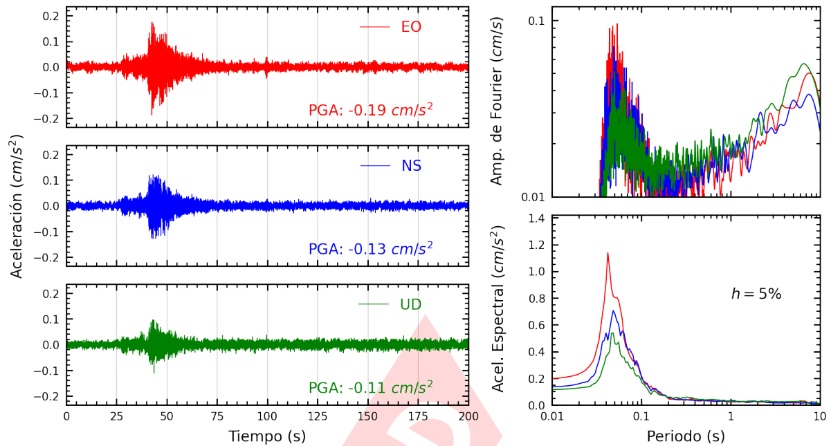
Figura A.17: Registros tiempo-historia, espectros de Fourier y de respuesta en las direcciones EO, NS y vertical de la estación UCSS. Sismo de Mala, Cañete - Lima del 2024-08-15, 04:38:57 (Hora local)
