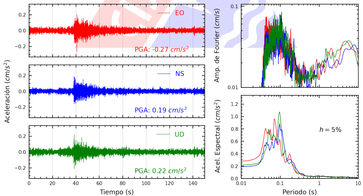
Figura A.12: Registros tiempo-historia, espectros de Fourier y de respuesta en las direcciones EO, NS y vertical de la estación UCV. Sismo de Mala, Cañete - Lima del 2024-08-15, 04:38:57 (Hora local)
