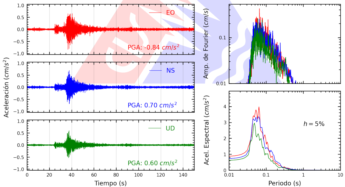
Figura A.2: Registros tiempo-historia, espectros de Fourier y de respuesta en las direcciones EO, NS y vertical de la estación UNTEL. Sismo de Mala, Cañete - Lima del 2024-08-15, 04:38:57 (Hora local)
