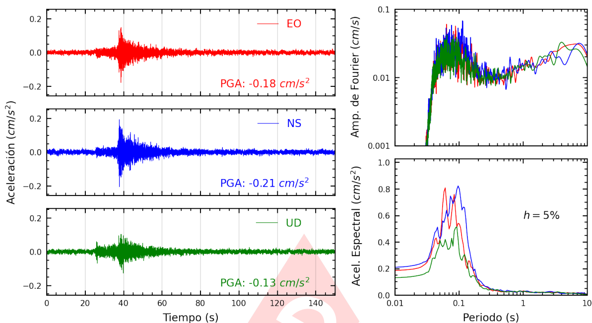
Figura A.15: Registros tiempo-historia, espectros de Fourier y de respuesta en las direcciones EO, NS y vertical de la estación SERVI. Sismo de Mala, Cañete - Lima del 2024-08-15, 04:38:57 (Hora local)
