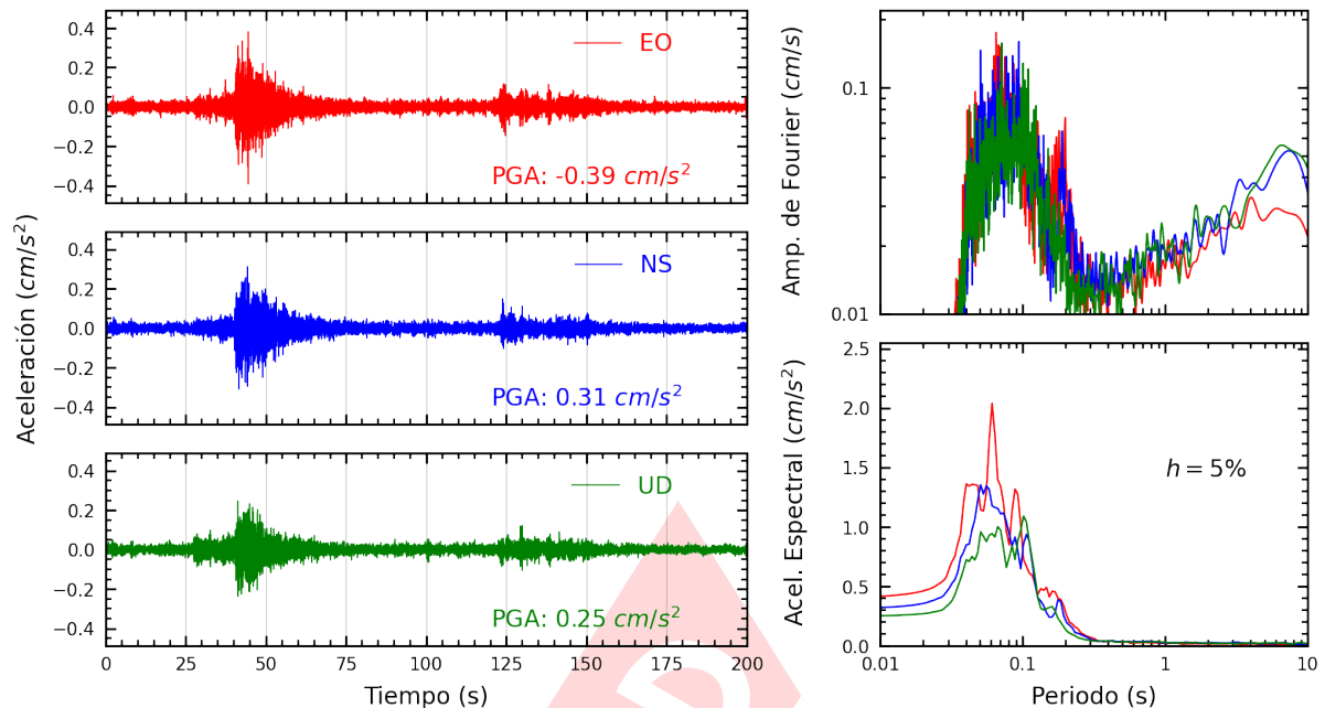
Figura A.9: Registros tiempo-historia, espectros de Fourier y de respuesta en las direcciones EO, NS y vertical de la estación INDEP. Sismo de Mala, Cañete - Lima del 2024-08-15, 04:38:57 (Hora local)
