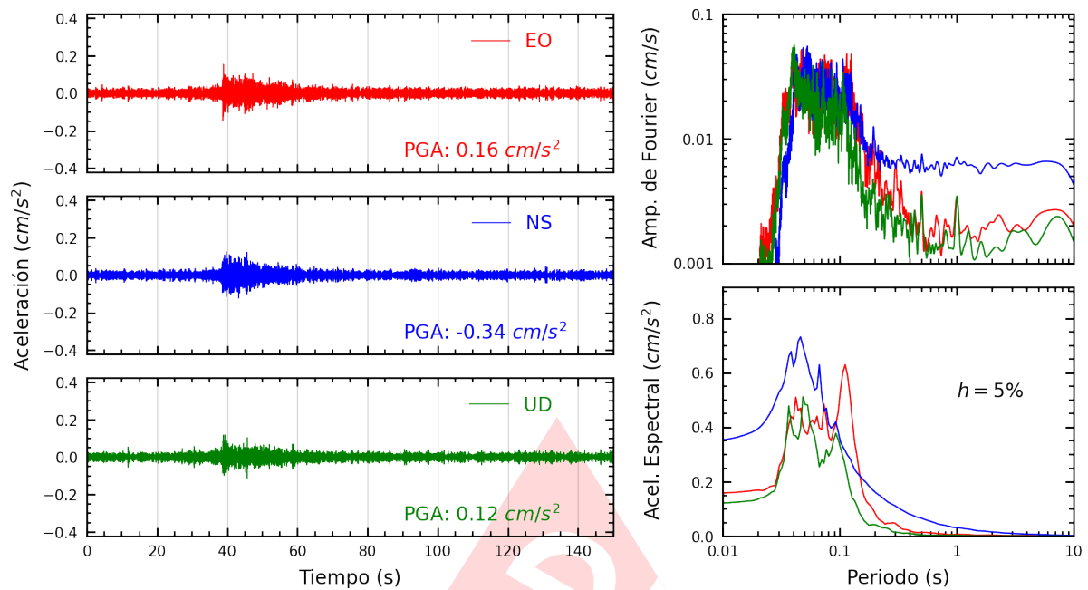
Figura A.11: Registros tiempo-historia, espectros de Fourier y de respuesta en las direcciones EO, NS y vertical de la estación ATARJ. Sismo de Mala, Cañete - Lima del 2024-08-15, 04:38:57 (Hora local)
