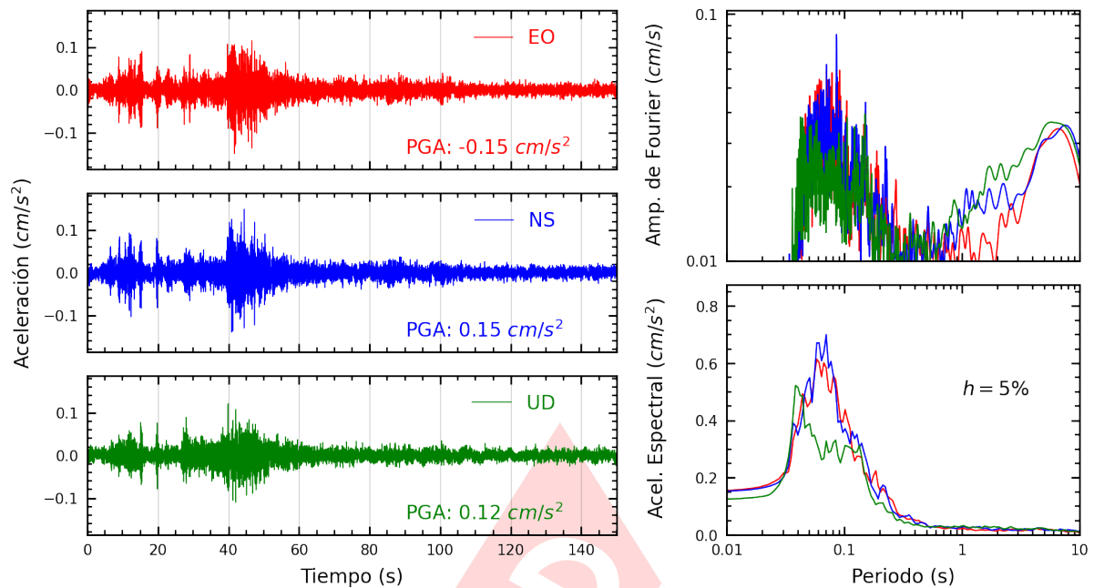
Figura A.19: Registros tiempo-historia, espectros de Fourier y de respuesta en las direcciones EO, NS y vertical de la estación UPCSM. Sismo de Mala, Cañete - Lima del 2024-08-15, 04:38:57 (Hora local)
