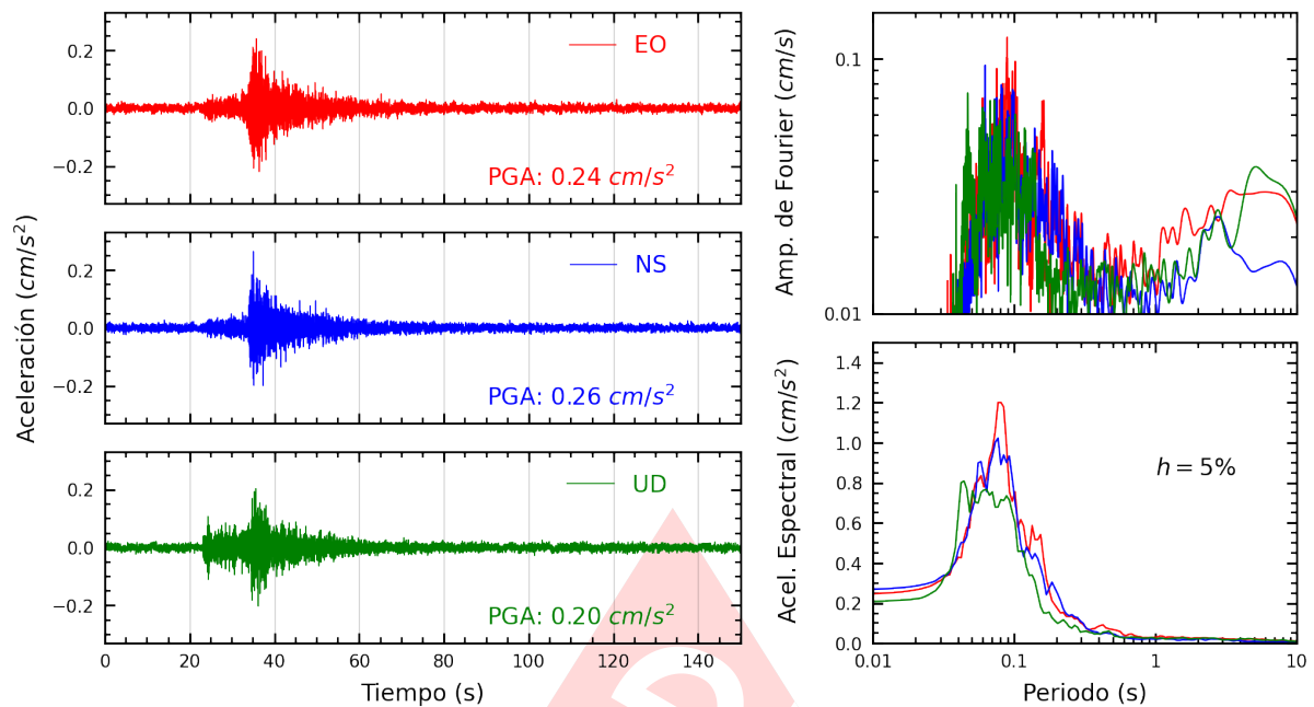
Figura A.13: Registros tiempo-historia, espectros de Fourier y de respuesta en las direcciones EO, NS y vertical de la estación USILP. Sismo de Mala, Cañete - Lima del 2024-08-15, 04:38:57 (Hora local)
