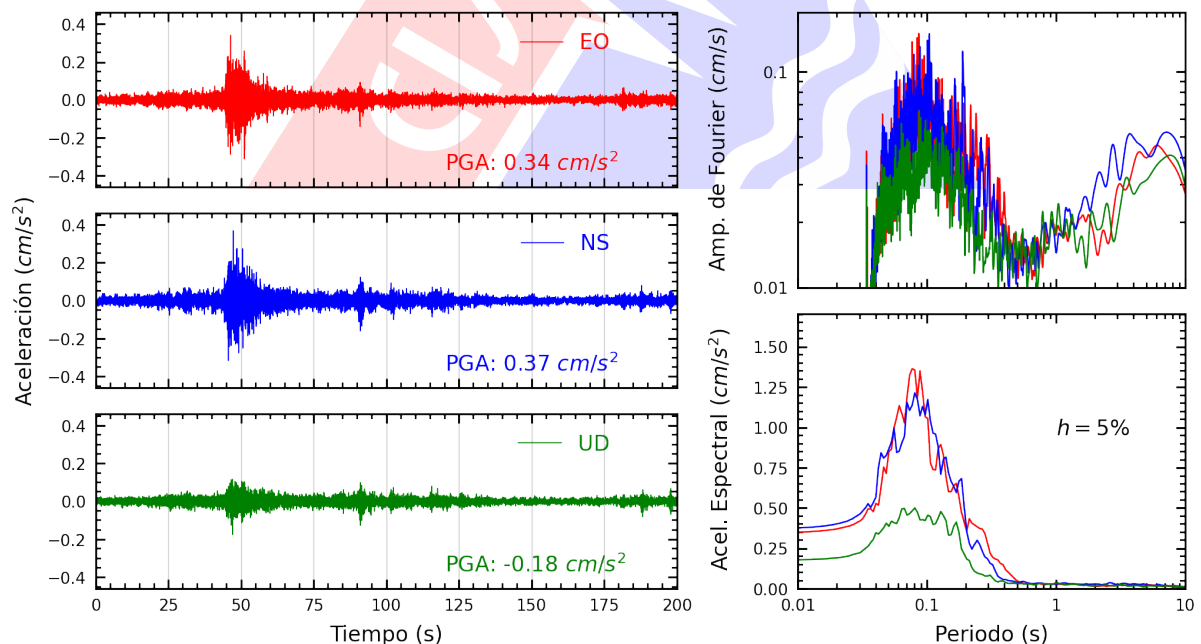
Figura A.10: Registros tiempo-historia, espectros de Fourier y de respuesta en las direcciones EO, NS y vertical de la estación DEFEN. Sismo de Mala, Cañete - Lima del 2024-08-15, 04:38:57 (Hora local)
