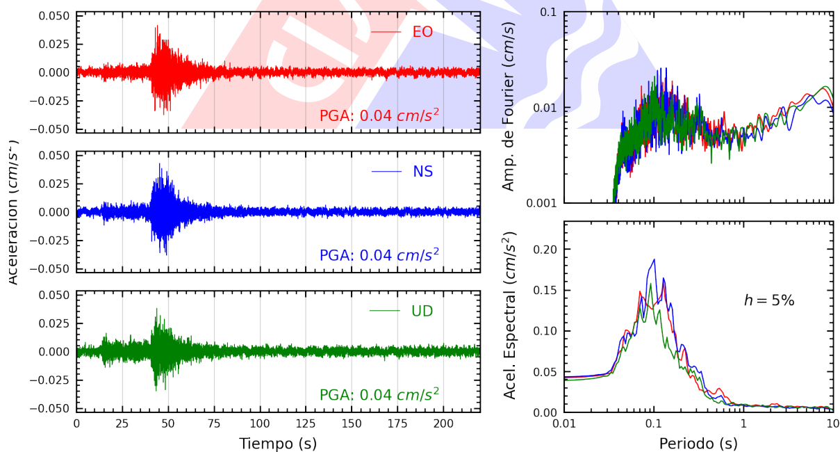
Figura A.24: Registros tiempo-historia, espectros de Fourier y de respuesta en las direcciones EO, NS y vertical de la estación CARAL. Sismo de Mala, Cañete - Lima del 2024-08-15, 04:38:57 (Hora local)
