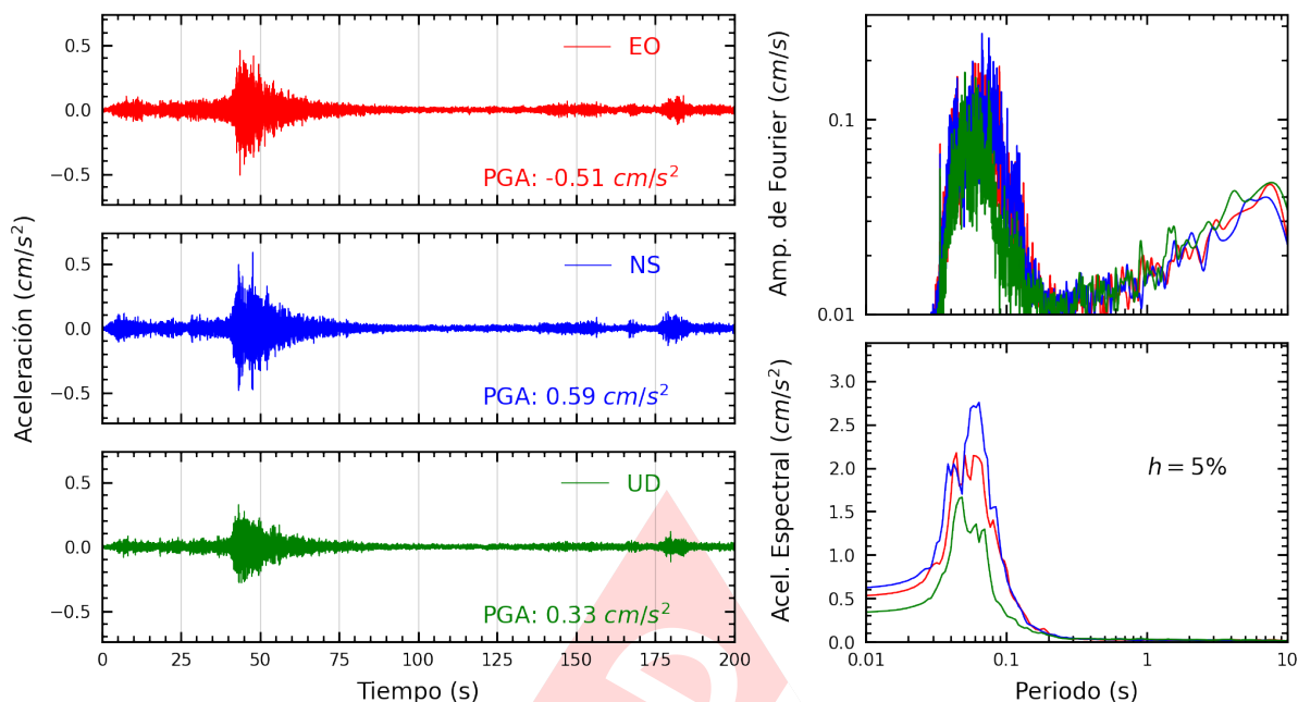
Figura A.3: Registros tiempo-historia, espectros de Fourier y de respuesta en las direcciones EO, NS y vertical de la estación JOSEO. Sismo de Mala, Cañete - Lima del 2024-08-15, 04:38:57 (Hora local)
