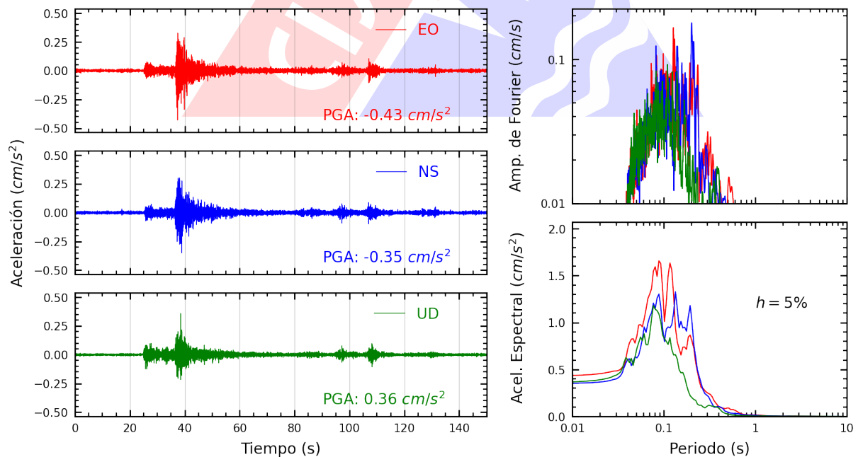
Figura A.8: Registros tiempo-historia, espectros de Fourier y de respuesta en las direcciones EO, NS y vertical de la estación SCCHO. Sismo de Mala, Cañete - Lima del 2024-08-15, 04:38:57 (Hora local)
