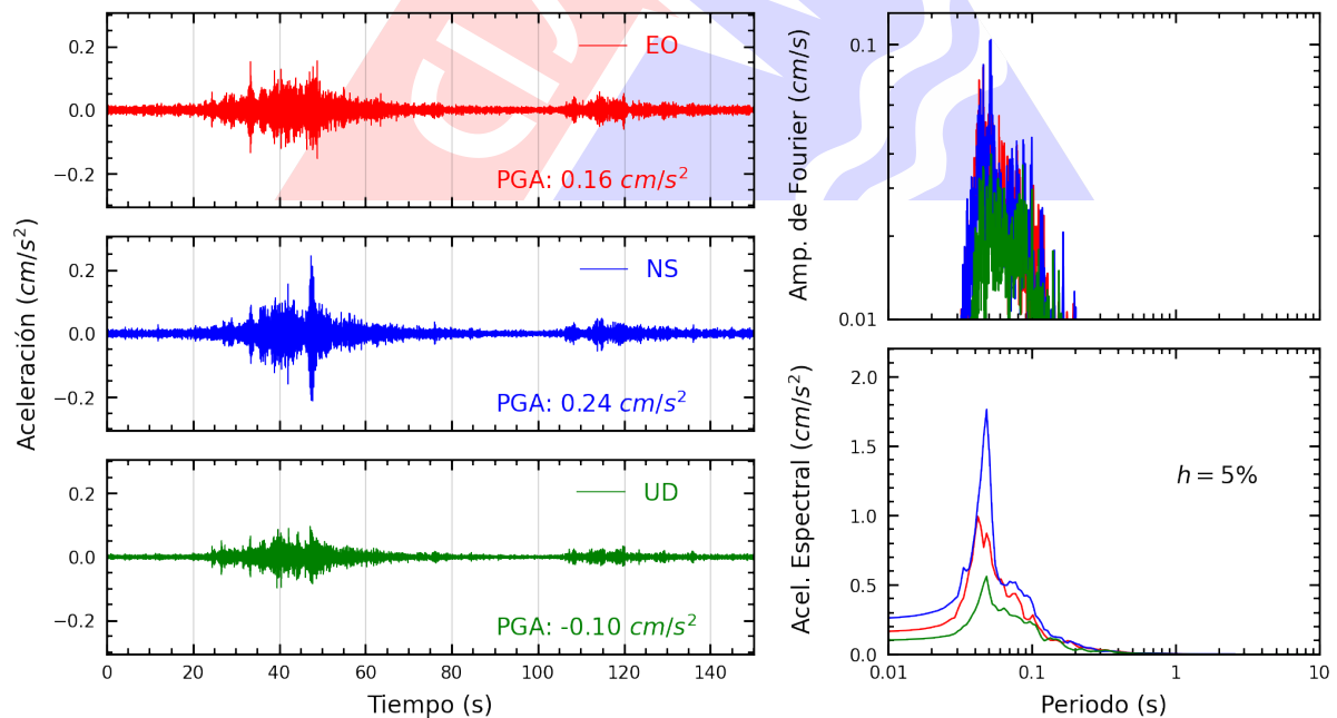
Figura A.14: Registros tiempo-historia, espectros de Fourier y de respuesta en las direcciones EO, NS y vertical de la estación BORJA. Sismo de Mala, Cañete - Lima del 2024-08-15, 04:38:57 (Hora local)
