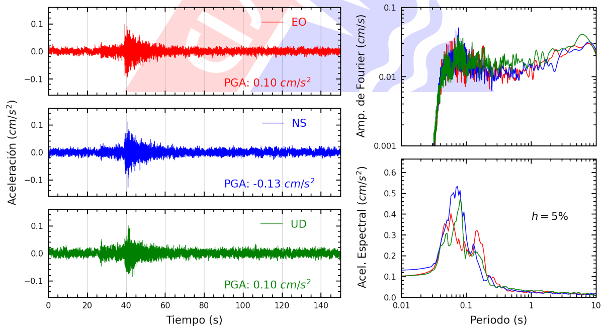
Figura A.22: Registros tiempo-historia, espectros de Fourier y de respuesta en las direcciones EO, NS y vertical de la estación UNFV. Sismo de Mala, Cañete - Lima del 2024-08-15, 04:38:57 (Hora local)
