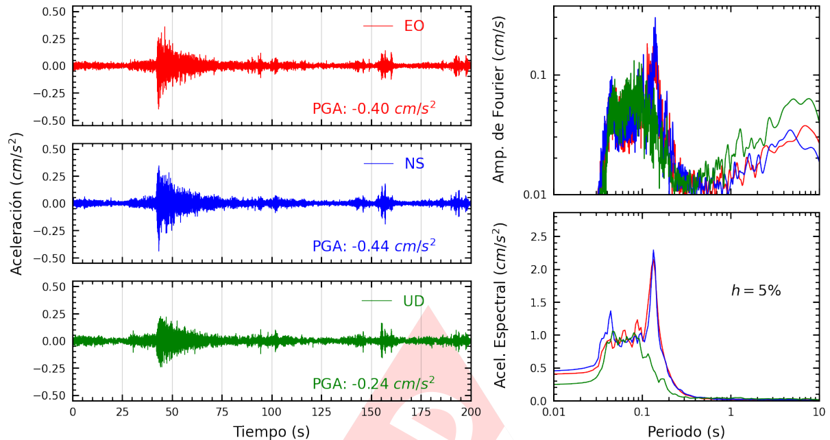
Figura A.7: Registros tiempo-historia, espectros de Fourier y de respuesta en las direcciones EO, NS y vertical de la estación CARAB. Sismo de Mala, Cañete - Lima del 2024-08-15, 04:38:57 (Hora local)
