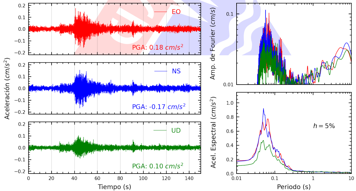
Figura A.18: Registros tiempo-historia, espectros de Fourier y de respuesta en las direcciones EO, NS y vertical de la estación FICPE. Sismo de Mala, Cañete - Lima del 2024-08-15, 04:38:57 (Hora local)
