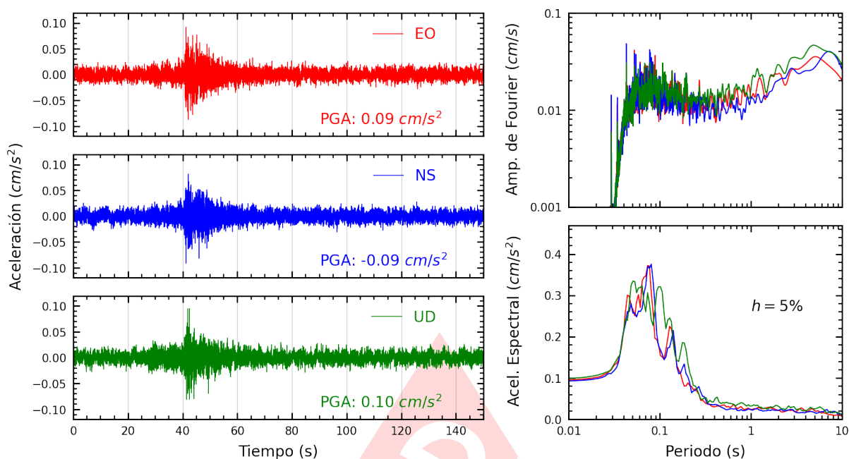
Figura A.23: Registros tiempo-historia, espectros de Fourier y de respuesta en las direcciones EO, NS y vertical de la estación UNMSM. Sismo de Mala, Cañete - Lima del 2024-08-15, 04:38:57 (Hora local)
