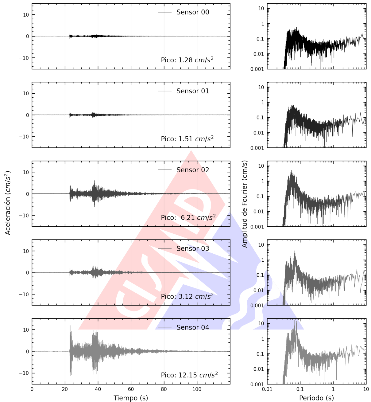
Figura A.3: Registros tiempo-historia y espectros de Fourier en la dirección vertical de la edificación Centro de Observación para la Ingeniería Sísmica del CISMID-FIC-UNI. Sismo de Huacho, Huaura - Lima del 2024-08-17, 03:04:02 (Hora local)
