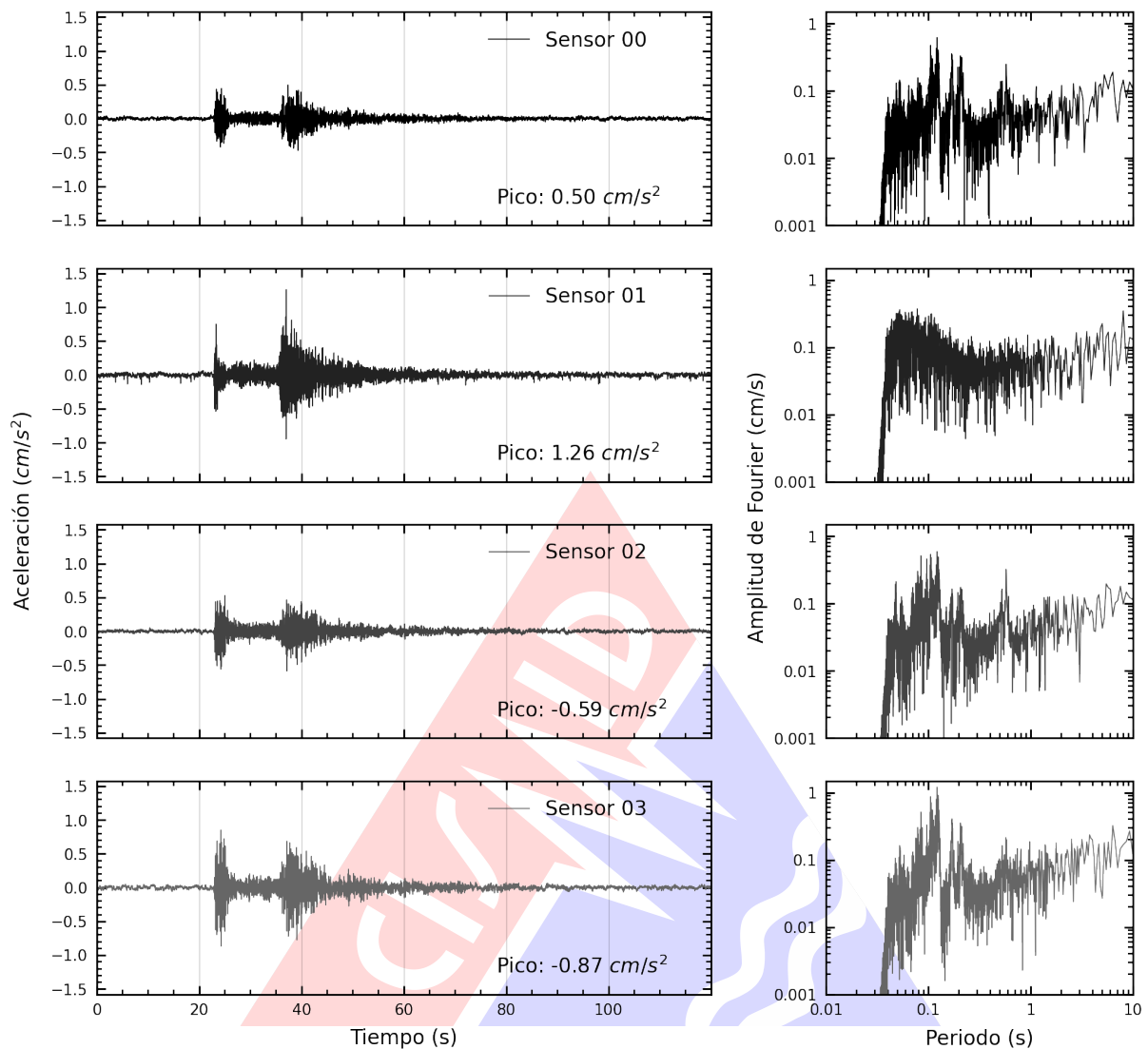
Figura A.2: Registros tiempo-historia y espectros de Fourier en la dirección NS de la edificación Centro de Información e Investigación de la FIC-UNI. Sismo de Huacho, Huaura - Lima del 2024-08-17, 03:04:02 (Hora local)
