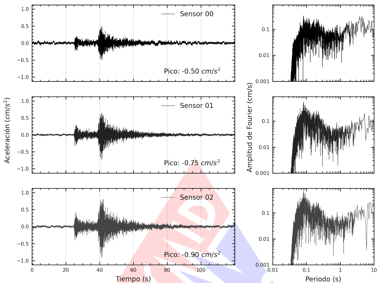
Figura A.1: Registros tiempo-historia y espectros de Fourier en la dirección EW de la edificación Vivienda. Sismo de Huacho, Huaura - Lima del 2024-08-17, 03:04:02 (Hora local)
