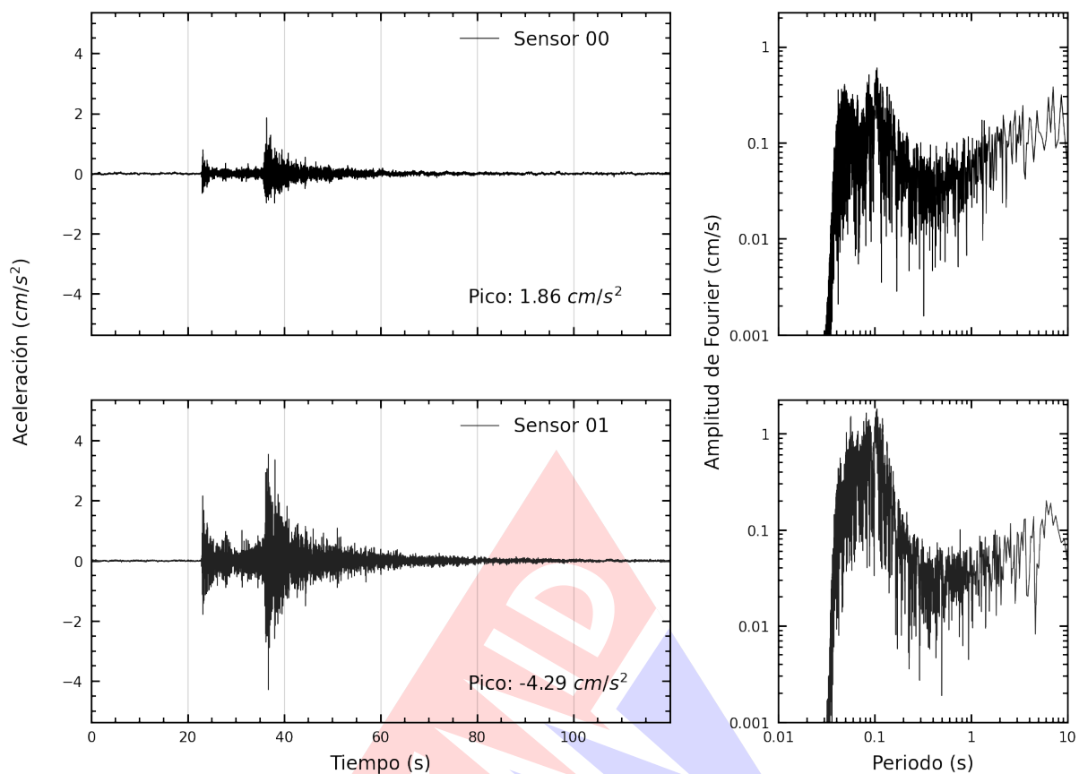
Figura A.2: Registros tiempo-historia y espectros de Fourier en la dirección NS de la edificación Laboratorio de Estructuras del CISMID-FIC-UNI. Sismo de Huacho, Huaura - Lima del 2024-08-17, 03:04:02 (Hora local)
