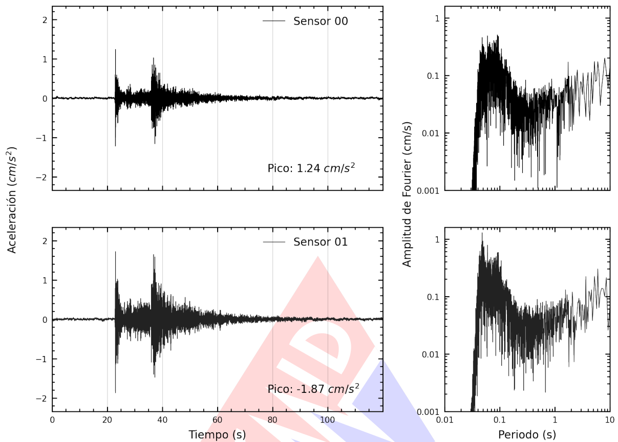
Figura A.3: Registros tiempo-historia y espectros de Fourier en la dirección vertical de la edificación Laboratorio de Estructuras del CISMID-FIC-UNI. Sismo de Huacho, Huaura - Lima del 2024-08-17, 03:04:02 (Hora local)
