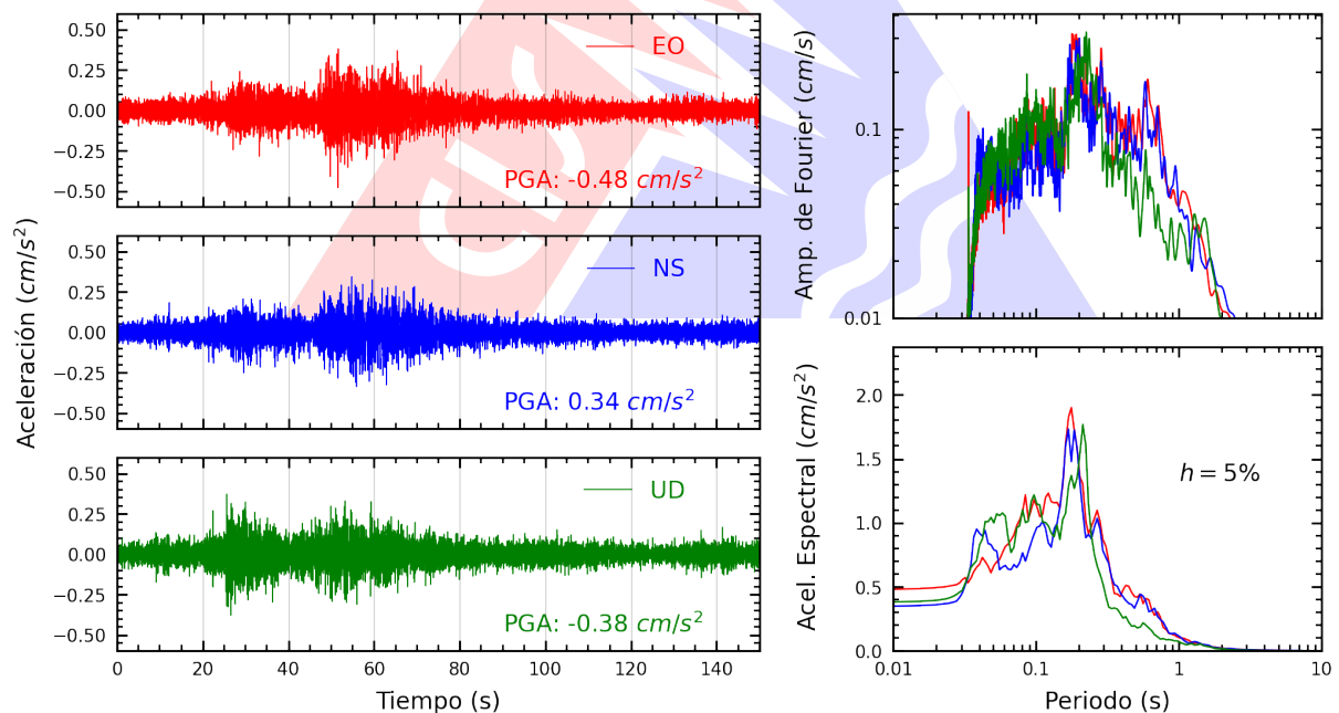
Figura A.2: Registros tiempo-historia, espectros de Fourier y de respuesta en las direcciones EO, NS y vertical de la estación SCICA. Sismo de Acari, Caraveli - Arequipa del 2024-08-17, 21:47:55 (Hora local)
