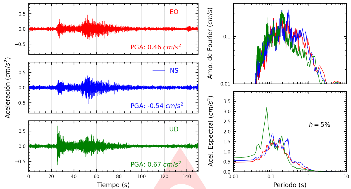
Figura A.1: Registros tiempo-historia, espectros de Fourier y de respuesta en las direcciones EO, NS y vertical de la estación UNICA. Sismo de Acari, Caraveli - Arequipa del 2024-08-17, 21:47:55 (Hora local)
