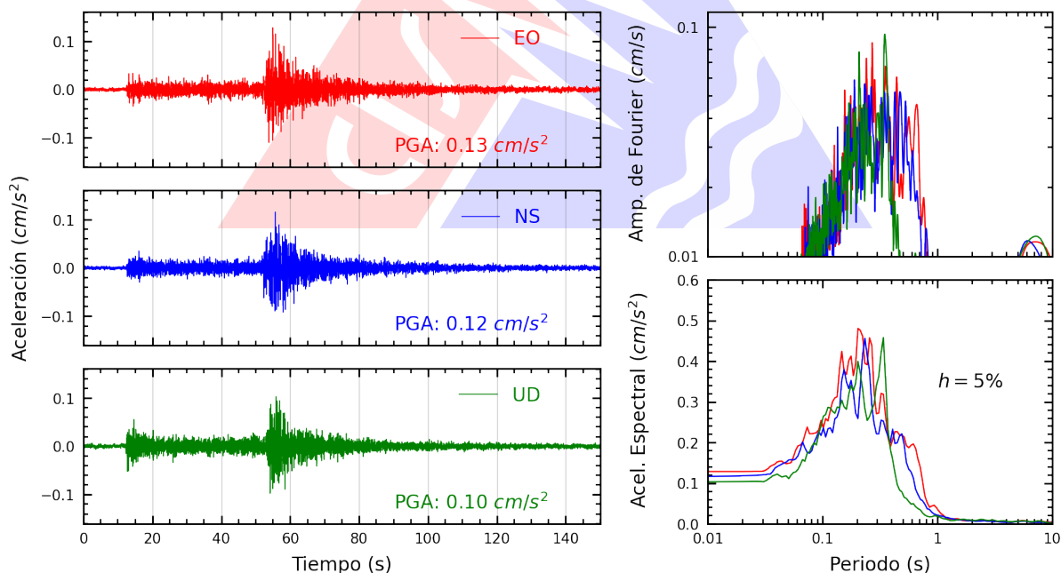
Figura A.2: Registros tiempo-historia, espectros de Fourier y de respuesta en las direcciones EO, NS y vertical de la estación CARAL. Sismo de Pucallpa, Coronel Portillo - Ucayali del 2024-08-17, 23:10:17 (Hora local)
