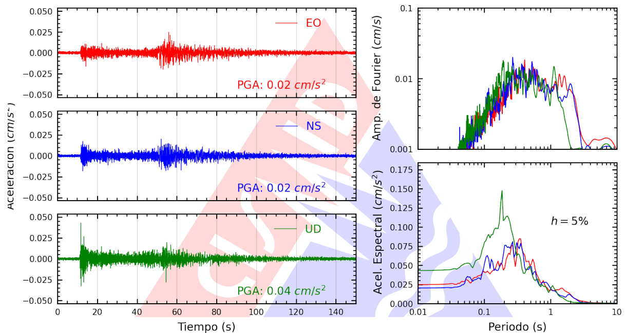
Figura A.3: Registros tiempo-historia, espectros de Fourier y de respuesta en las direcciones EO, NS y vertical de la estación UNCP. Sismo de Pucallpa, Coronel Portillo - Ucayali del 2024-08-17, 23:10:17 (Hora local)
