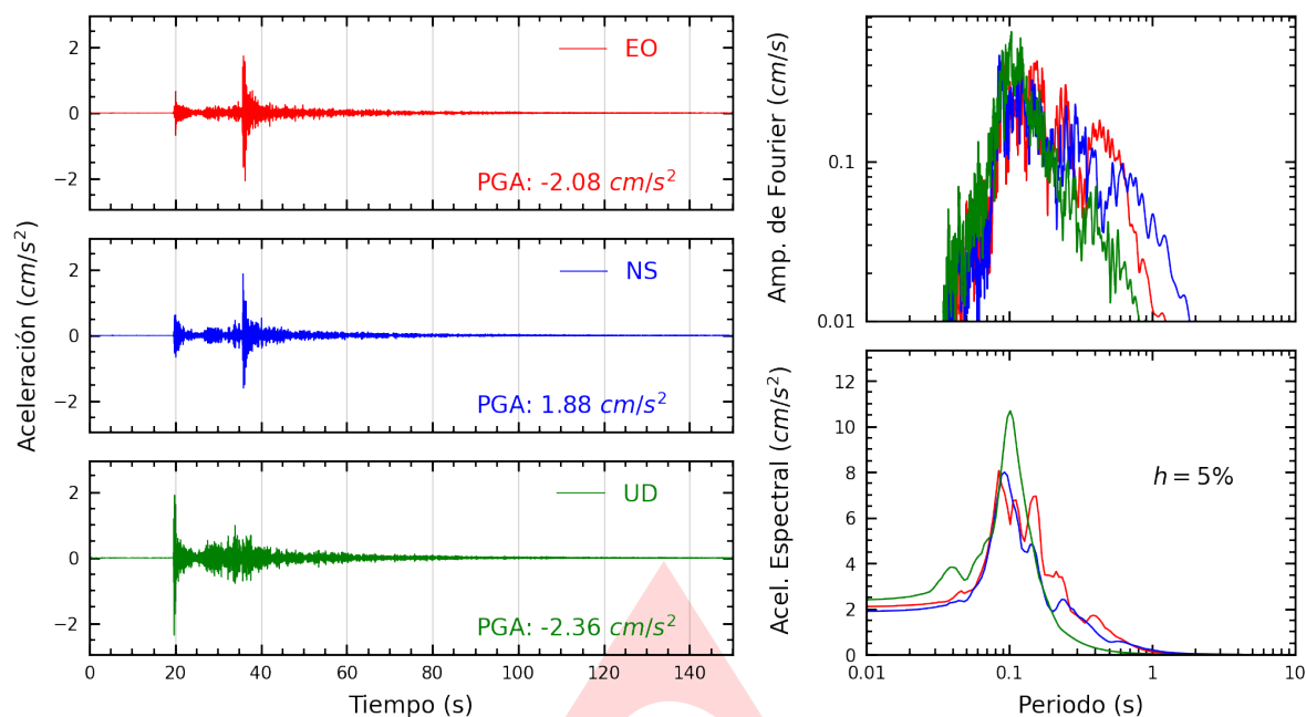
Figura A.1: Registros tiempo-historia, espectros de Fourier y de respuesta en las direcciones EO, NS y vertical de la estación UNIA. Sismo de Pucallpa, Coronel Portillo - Ucayali del 2024-08-17, 23:10:17 (Hora local)
