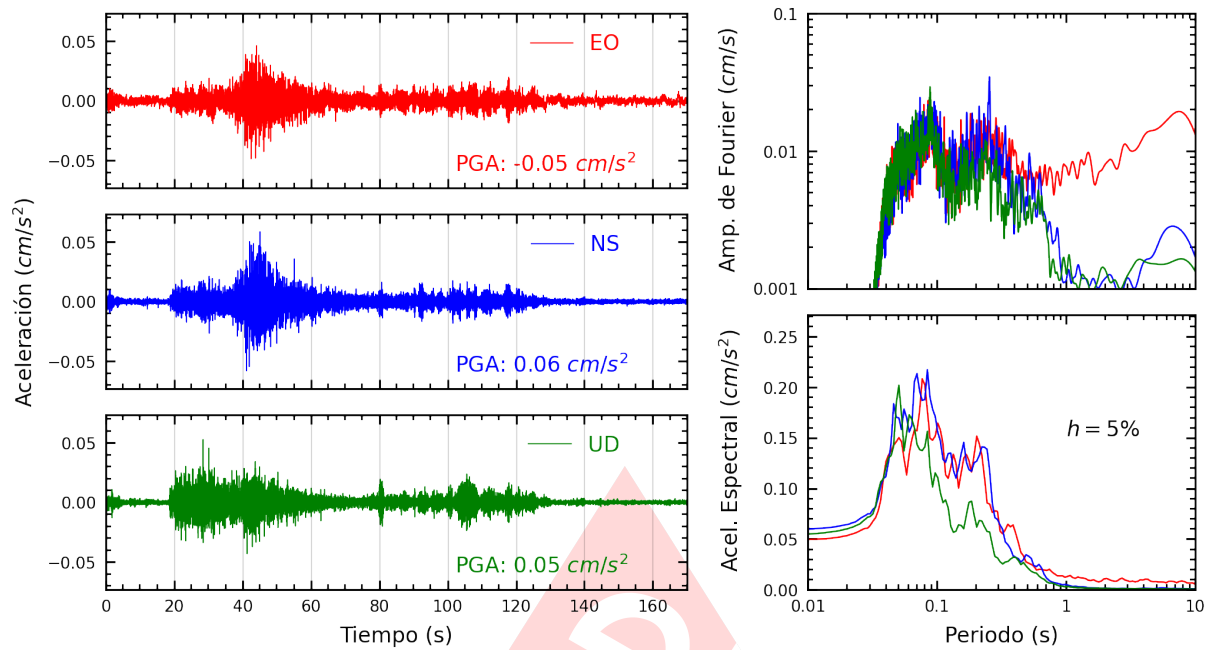
Figura A.3: Registros tiempo-historia, espectros de Fourier y de respuesta en las direcciones EO, NS y vertical de la estación SCCHI. Sismo de Trujillo, Trujillo - La Libertad del 2024-08-27, 04:55:11 (Hora local)
