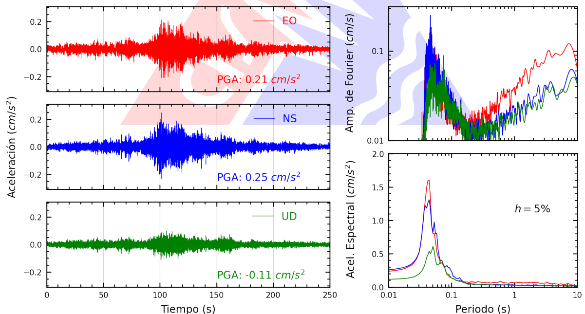
Figura A.2: Registros tiempo-historia, espectros de Fourier y de respuesta en las direcciones EO, NS y vertical de la estación UNAB. Sismo de Trujillo, Trujillo - La Libertad del 2024-08-27, 04:55:11 (Hora local)
