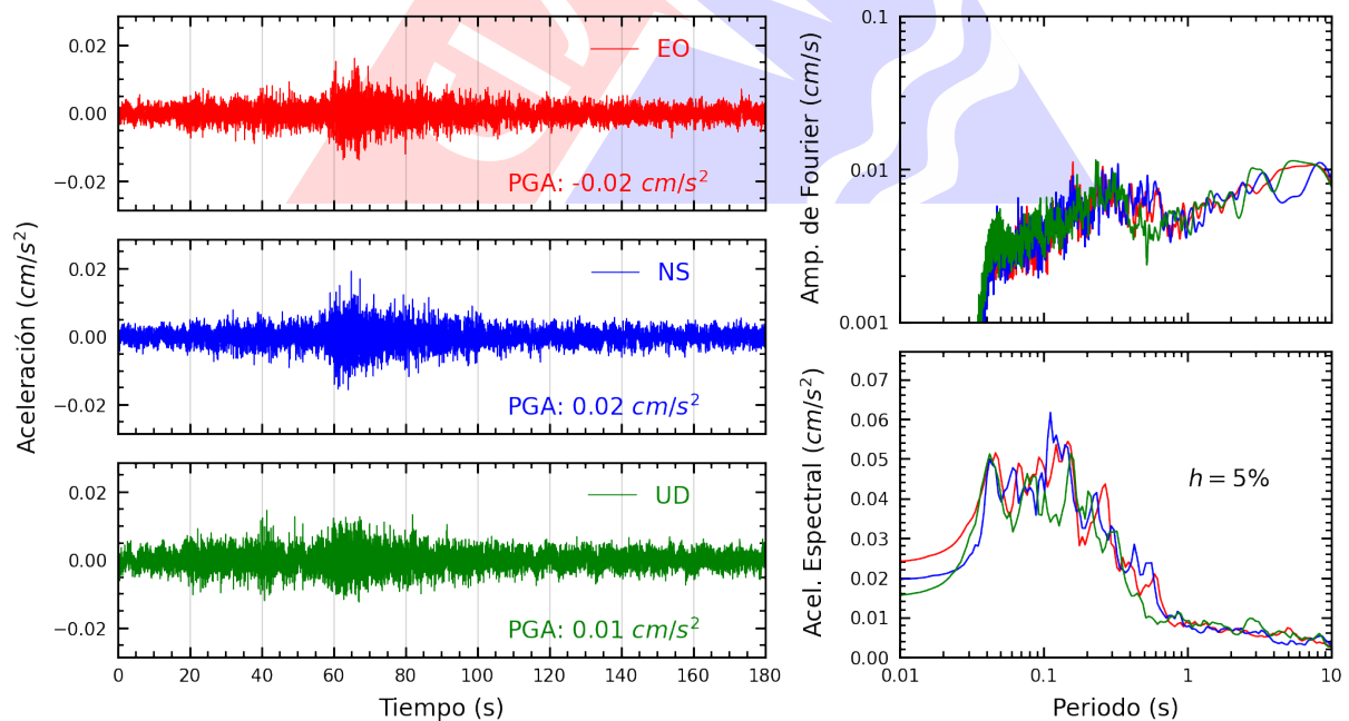
Figura A.4: Registros tiempo-historia, espectros de Fourier y de respuesta en las direcciones EO, NS y vertical de la estación CARAL. Sismo de Trujillo, Trujillo - La Libertad del 2024-08-27, 04:55:11 (Hora local)
