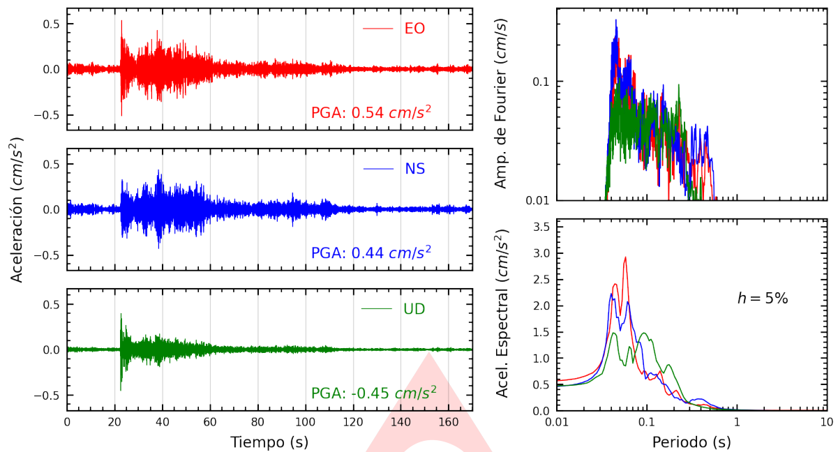
Figura A.1: Registros tiempo-historia, espectros de Fourier y de respuesta en las direcciones EO, NS y vertical de la estación SCTRU. Sismo de Trujillo, Trujillo - La Libertad del 2024-08-27, 04:55:11 (Hora local)
