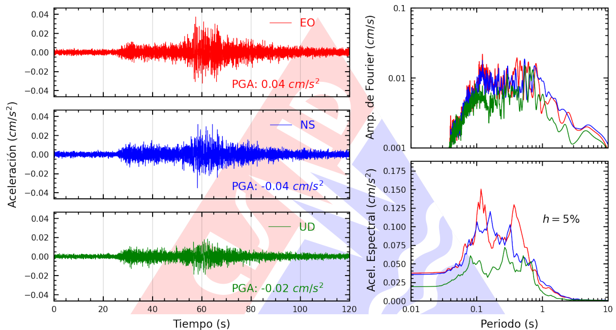
Figura A.3: Registros tiempo-historia, espectros de Fourier y de respuesta en las direcciones EO, NS y vertical de la estación ATARJ. Sismo de Huancabamba, Oxapampa - Pasco del 2024-04-01, 08:23:27 (Hora local)
