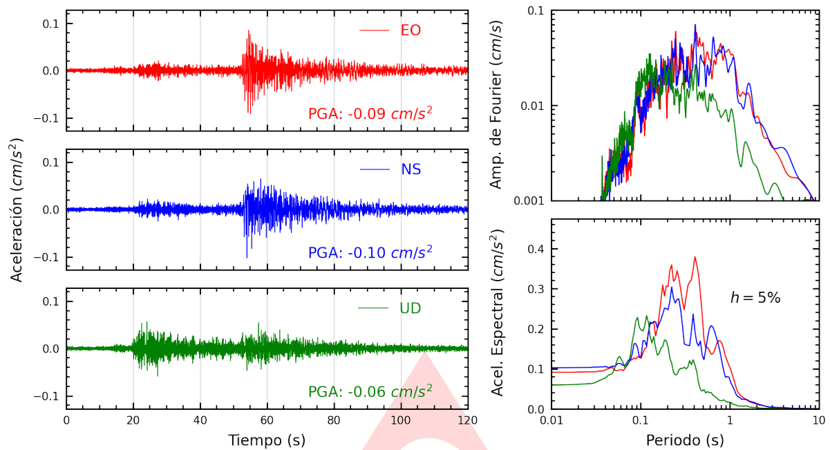
Figura A.1: Registros tiempo-historia, espectros de Fourier y de respuesta en las direcciones EO, NS y vertical de la estación UNIA. Sismo de Huancabamba, Oxapampa - Pasco del 2024-04-01, 08:23:27 (Hora local)
