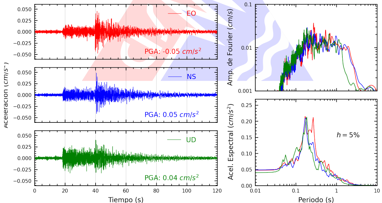
Figura A.2: Registros tiempo-historia, espectros de Fourier y de respuesta en las direcciones EO, NS y vertical de la estación UNCP. Sismo de Huancabamba, Oxapampa - Pasco del 2024-04-01, 08:23:27 (Hora local)
