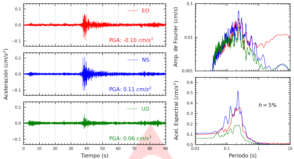
Figura A.1: Registros tiempo-historia, espectros de Fourier y de respuesta en las direcciones EO, NS y vertical de la estación SCCHI. Sismo de Sihuas, Sihuas - Ancash del 2024-04-11, 08:59:04 (Hora local)
